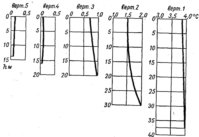
Распределение температуры воды по глубине в преддоставный период на разных участках вдхр Куйбышевское, 16/XII.
