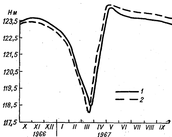
Рис. 7. Ход уровня вдхр Ивановское — г. Конаково.
