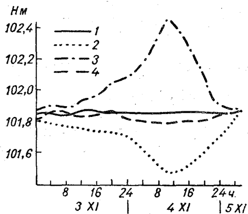
Рис. 11. Изменение уровня на постах при ветровой денивелизации на вдхр Рыбинском.
