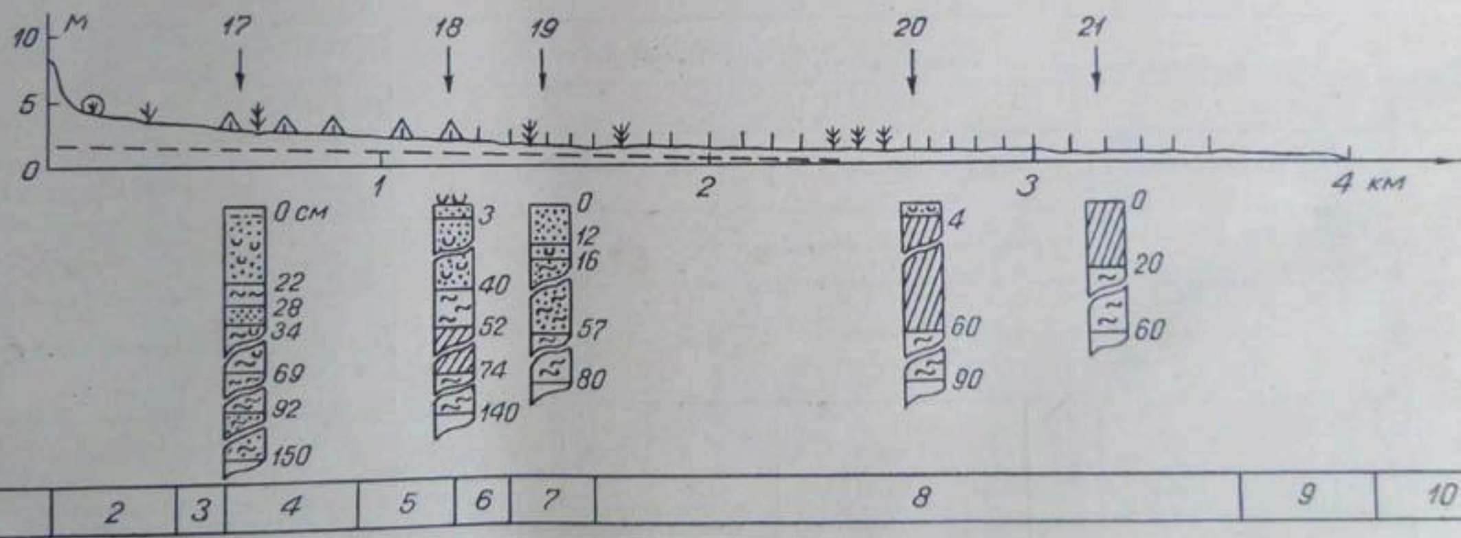
Рис. 32. Физико-географический профиль обсохшей части дна залива Аджибай (см. схему 6). Усл. обозн. см. на рис. 29.
