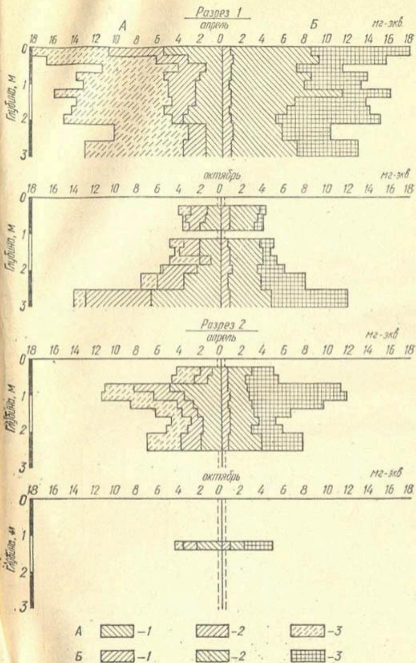
рис. 5. Изменение солевого профиля почвогрунтов при орошении риса (очвы междурядных отложений). "А—1— \text{Ca}^{++} , 2— \text{Mg}^{++} , 3— \text{Na} ; Б—1— \text{HCO}_3^- , 2— \text{Cl}^- , 3— \text{SO}_4^{--} .
