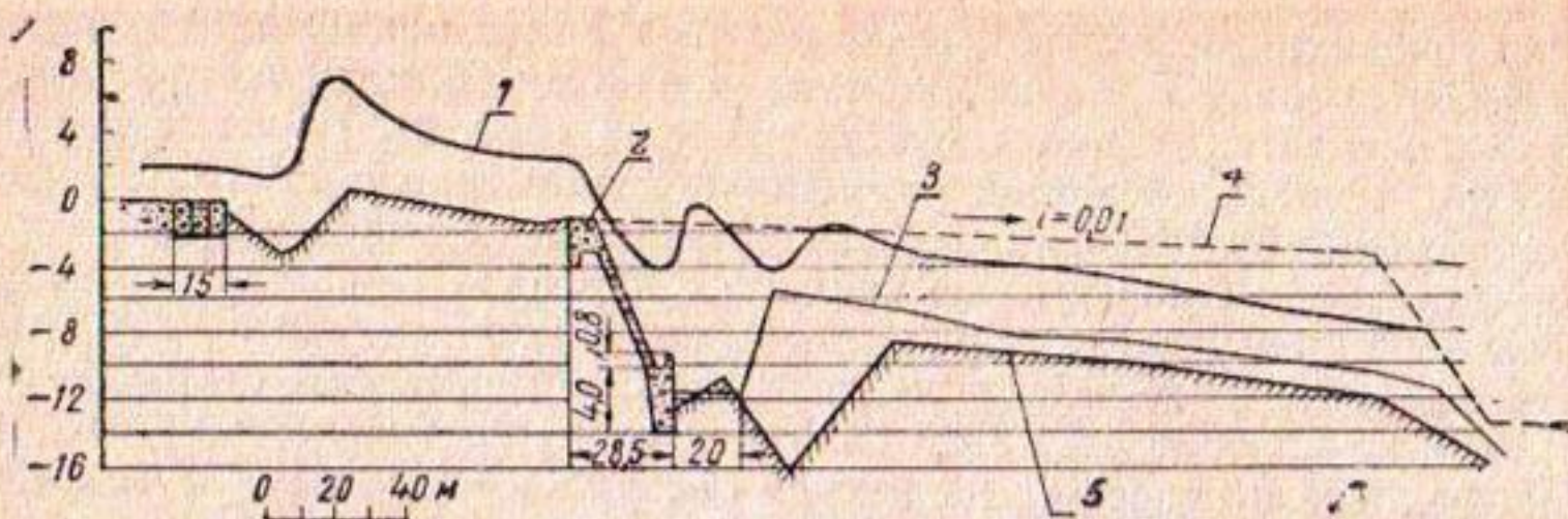
Рис. 4. Продольные профили отводящего канала (при наличии концевого перепада с удлиненным носком) и русла реки за ним по моделированию паводка 1%-ной обеспеченности:
