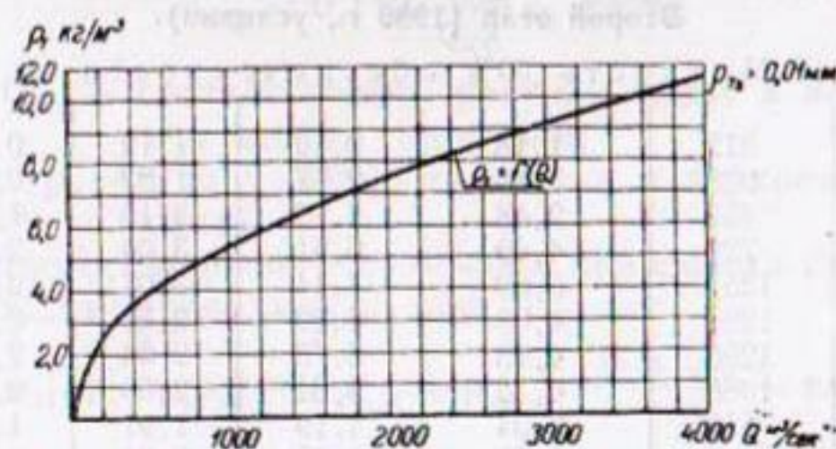
Рис. 7 Кривая \rho_T = f(Q) для фракции наносов d > 0,01 мм, р. Амударья, нижний бьеф Кизыл-Аякского гидроузла.
