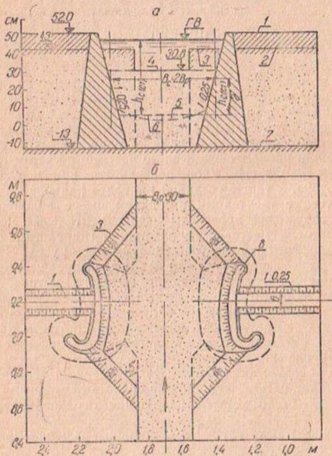
Рис. 1. Поперечный разрез (а) и план модели (б) искусственно сжатого русла (I и II цикл опытов):
