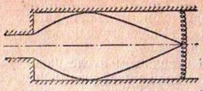
Рис. 4. Фронт гидравлического прыжка ниже «листа» растекающегося бурного потока.
