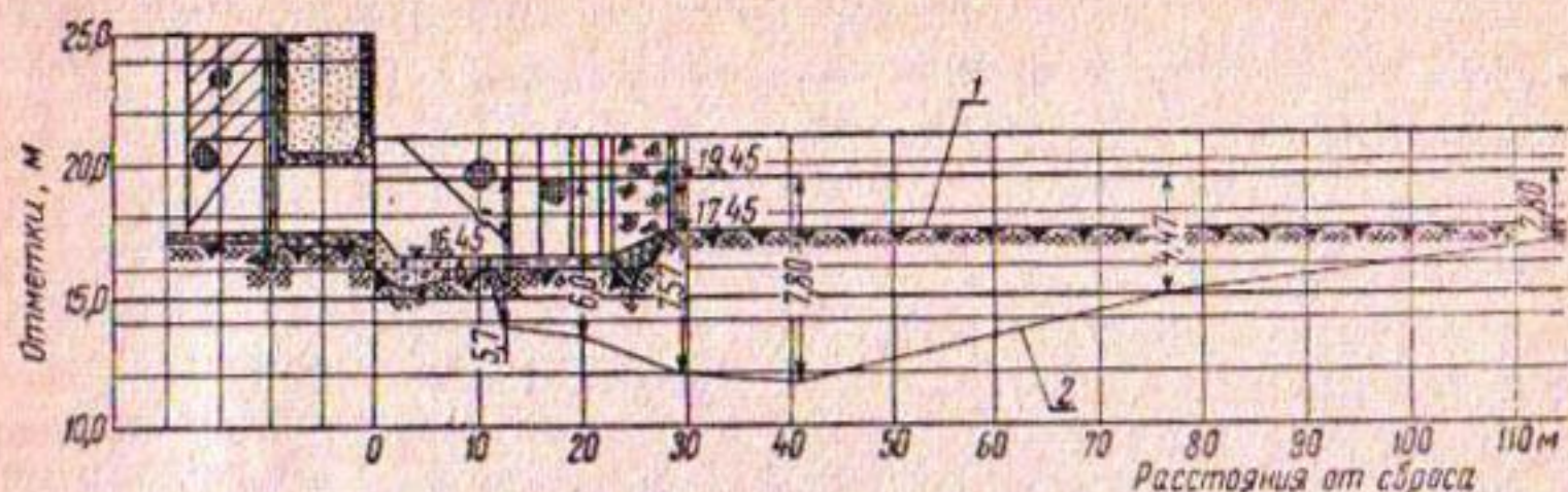
Рис. 3. Продольный профиль нижнего бьефа сбросного сооружения на ПК 469 БФК;
