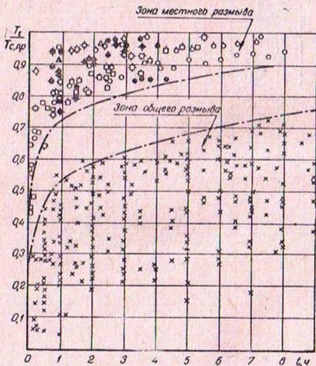
Рис. 10. График относительной глубины размыва во времени (данные опытов по общему размыву обозначены X, по местному размыву обозначения те же, что и на рисунке 8, б).
