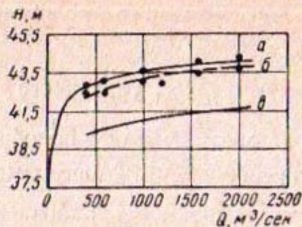
Рис. 5. Кривые зависимости Q=f(H) в створе за плотиной.
