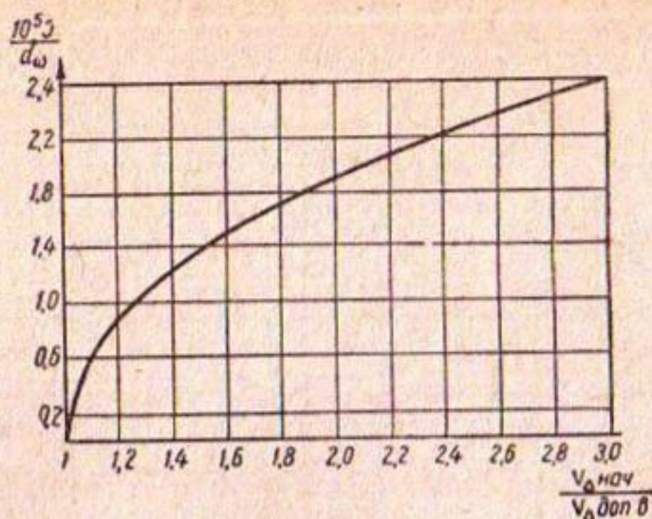
Рис. 5. Кривая зависимости средней интенсивности размыва I от отношения начальной донной скорости v_{\Delta \text{нач}} к допускаемой (неразмывающей) донной скорости в воронке размыва v_{\Delta \text{доп.в}} .
