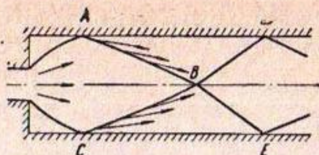
Рис. 2. Линии ударных волн при бурном состоянии потока в отводящем русле.
