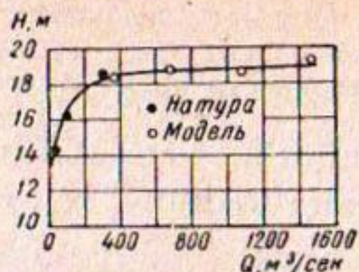
Рис. 6. Кривая зависимости Q=f(H) в створе моста.
