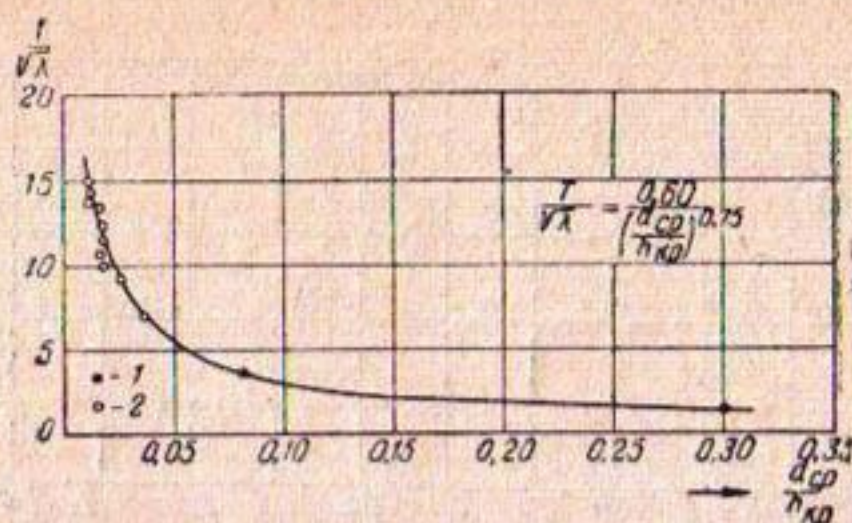
Рис. 9. График зависимости \frac{T}{\sqrt{\lambda}} = f\left(\frac{d_{cp}}{h_{kp}}\right) :
