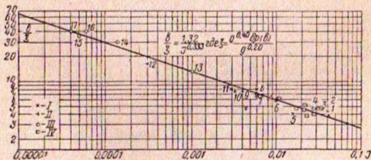
Рис. 12. Зависимость относительной ширины русла \frac{b}{\xi} от гидравлического уклона потока I :
