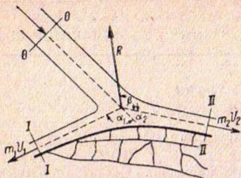
Рис. 1. Расчетная схема объема жидкости, заключенного между поверхностью тела, свободной поверхностью струи и сечениями 0—0, I—I и II—II.
