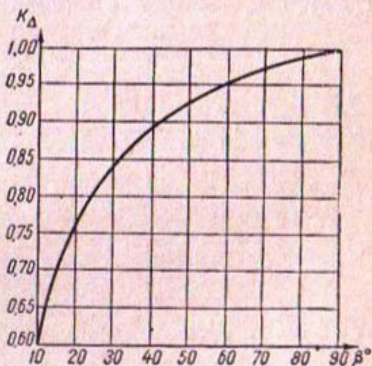
Рис. 1. Кривая зависимости относительной величины допускаемой (неразрывающей) донной скорости в воронке размыва K_{\Delta} от угла наклона входа струи \beta .
