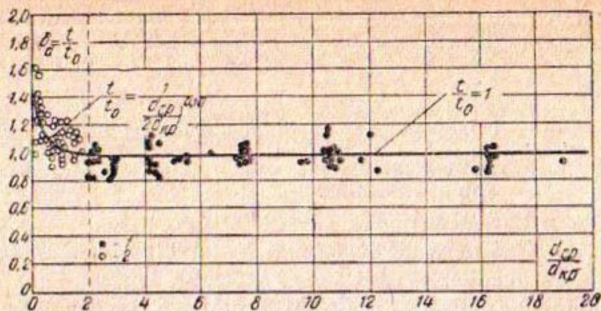
Рис. 6. График зависимости \frac{t}{t_0} = f\left(\frac{d_{cp}}{d_{кр}}\right) — среднее значение фактической глубины, полученной в опытах на модели в условиях плоской задачи; t_0 — расчетная глубина, определенная по формуле (14): 1 — опыты при d_{cp} > 2 мм; 2 — опыты при d_{cp} < 2 мм.
