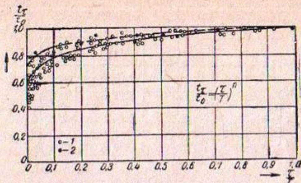
Рис. 10. График зависимости \frac{t_\tau}{t_0} = f\left(\frac{\tau}{T}\right) : 1 — опыты при d_{\text{ср}} < 2 мм, n = 0,11 ; 2 — опыты при d_{\text{ср}} > 2 мм, n = 0,06 .
