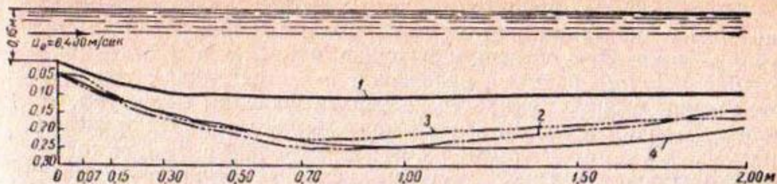
Рис. 1. Совмещенные профили местного размыва при различных гидравлических режимах в конце крепления. Опыты в лотке шириной 1,5 м с Q=0,090 \text{ м}^3/\text{сек} :
