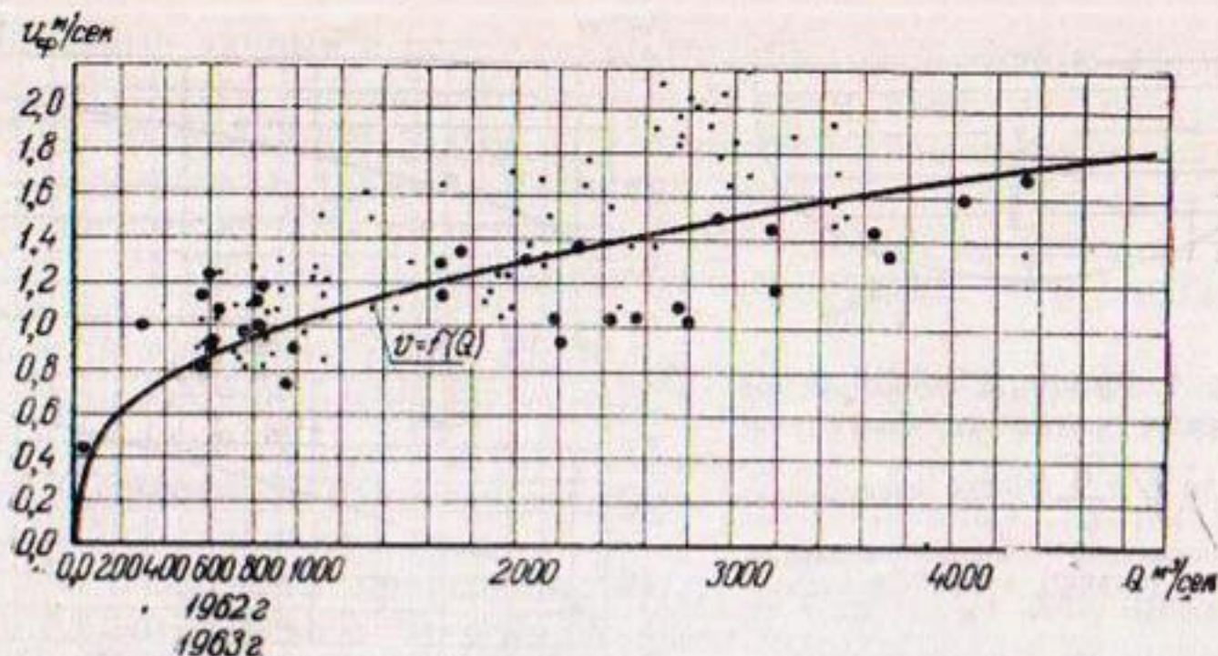
Рис. 3. Кривая v=f(Q) для расчетного формируемого русла при i=\text{const}=0,000238 (створ Пулизиндан) и данные наблюдений.
