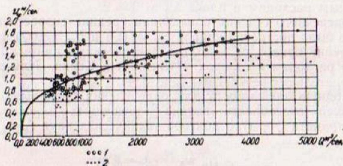
Рис. 4. Кривая v=f(Q) для расчетного формируемого русла, 1955 г.:
