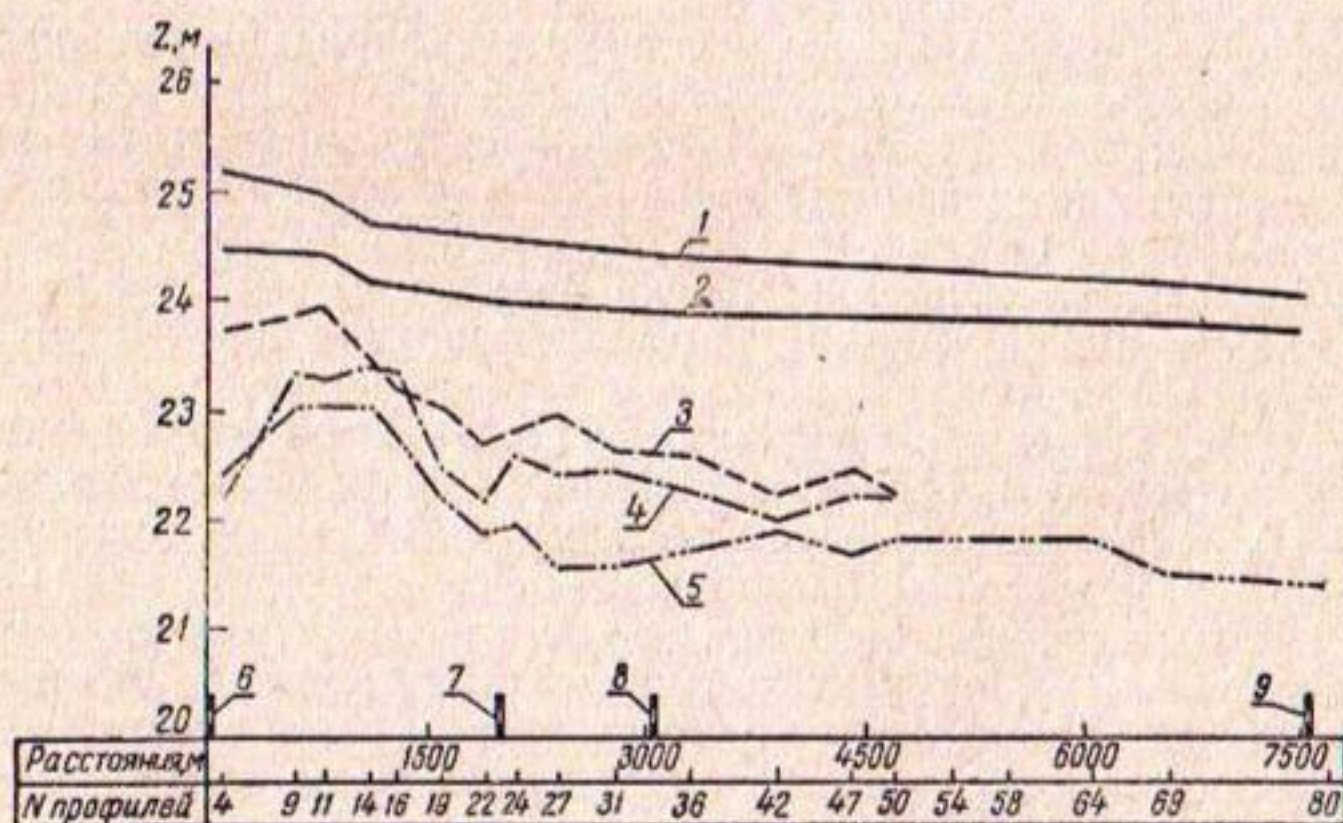
Рис. 5. Продольный профиль р. Неман по средним отметкам дна и уровням воды: 1 — уровень воды в 1955—1959 гг. при Q=300 m^3/сек ; 2 — то же, в 1963 г. при Q=300 m^3/сек ; 3 — профиль дна в 1959 г.; 4 — то же, в 1960 г.; 5 — то же, в 1963 г.; 6 — створ ГЭС; 7 — в/п Петрошюнай; 8 — в/п Вичунай № 18; 9 — в/п Панемуне.
