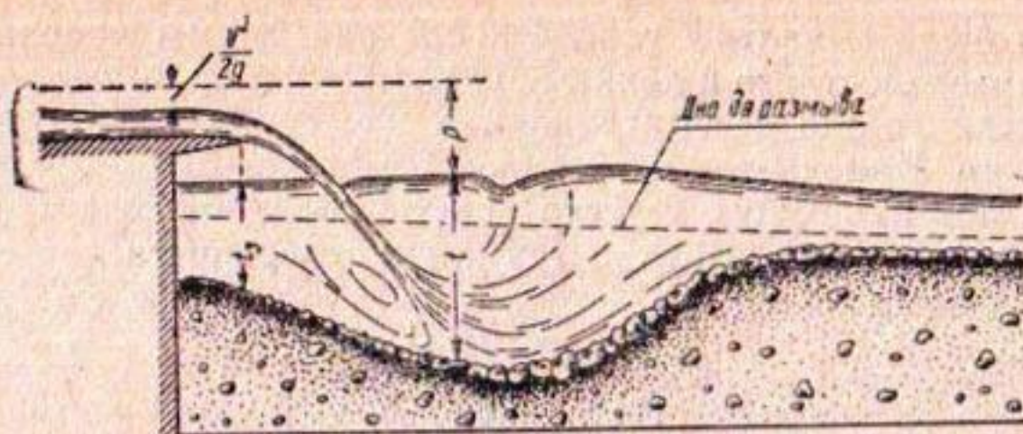
Рис. 2. Схема сопрягающего сооружения, исследованного в лабораторном лотке.
