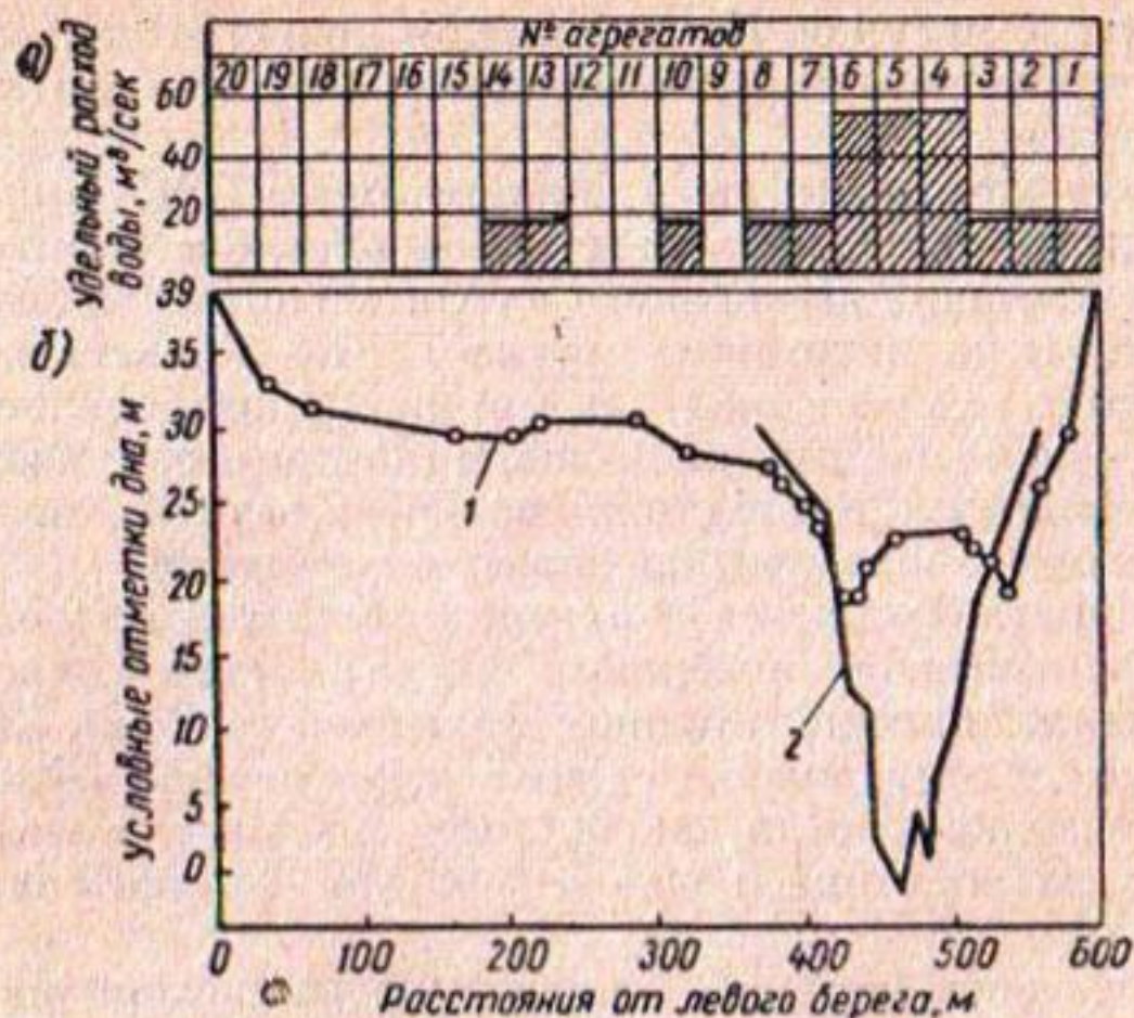
Рис. 3. Схемы к пропуску расходов воды через турбины и водосбросные отверстия ГЭС:
