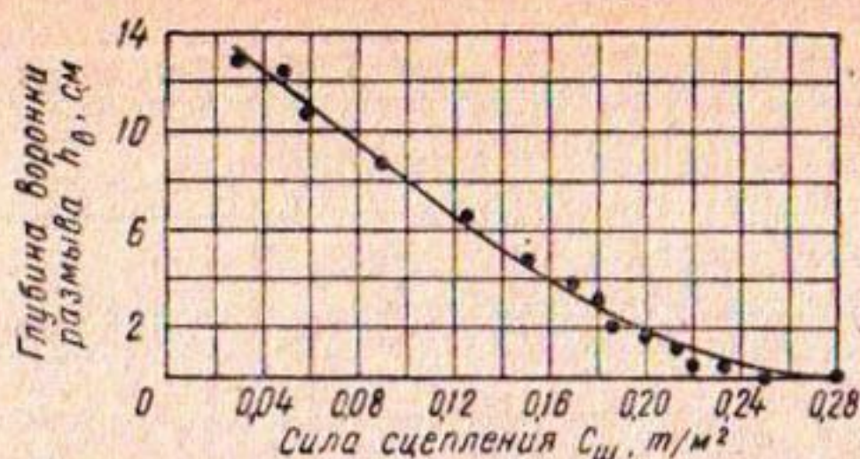
Рис. 1. Кривая сопротивляемости полностью водонасыщенных грунтов размыву в зависимости от величины сил сцепления.
