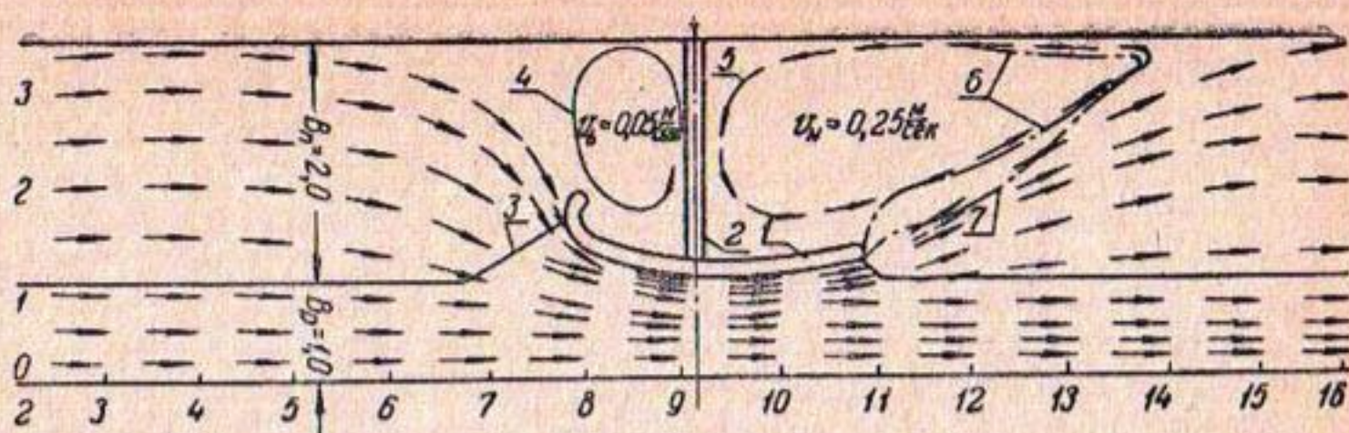
Рис. 4. Картина растекания поверхностных токов в третьем цикле опытов:
