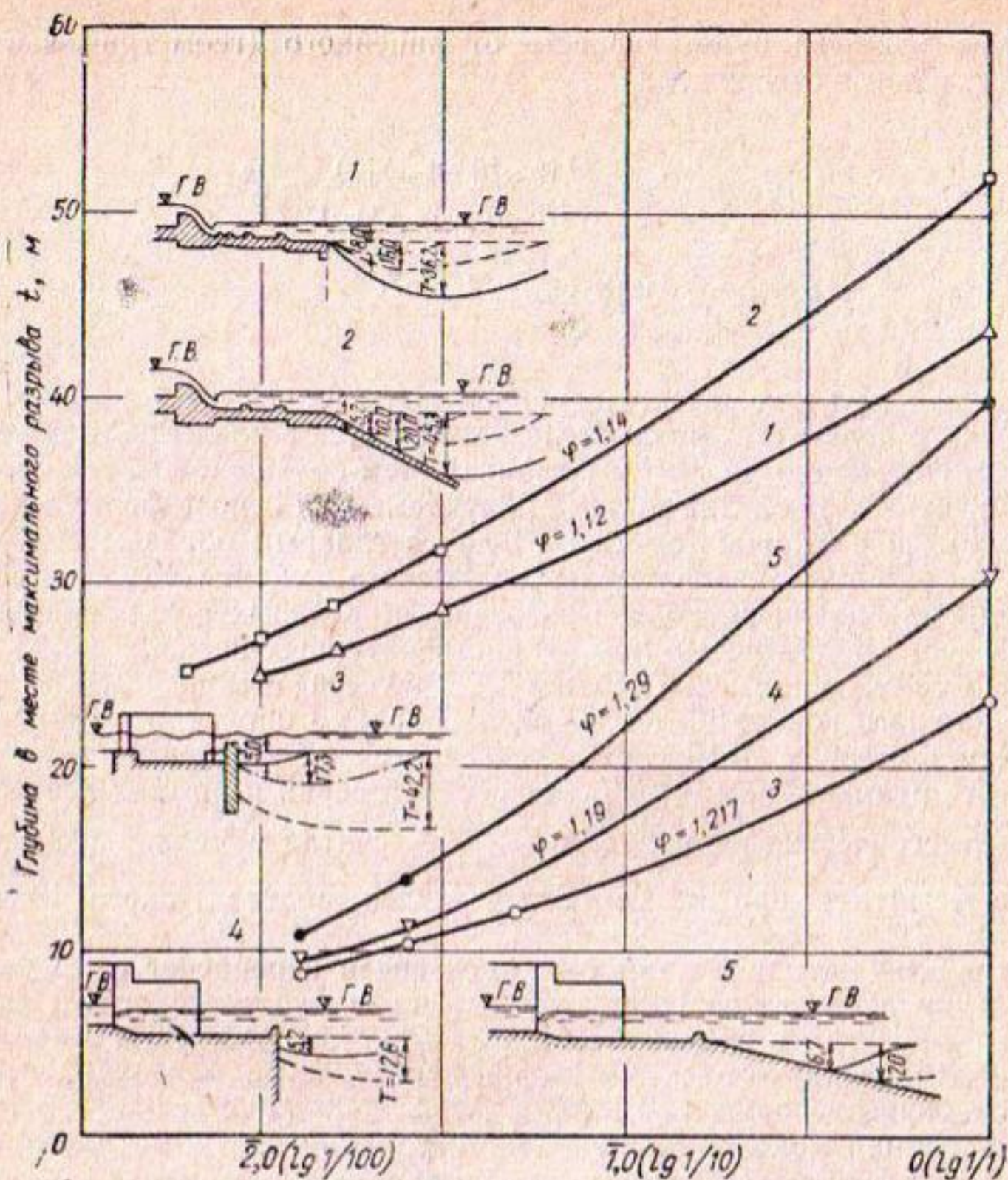
Рис. 1. Результаты исследований на моделях различных конструкций и прогнозирование глубины размыва в натуре:
