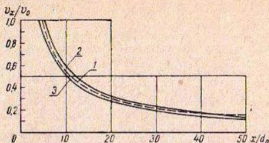
Рис. 1. Кривые изменения максимальной скорости (по оси) в осесимметричной (круглой) струе в зависимости от изменения расстояния от начального сечения: 1 — по Теперину; 2 — по Абрамовичу, при a=0,076 ; 3 — то же, при a=0,066 .
