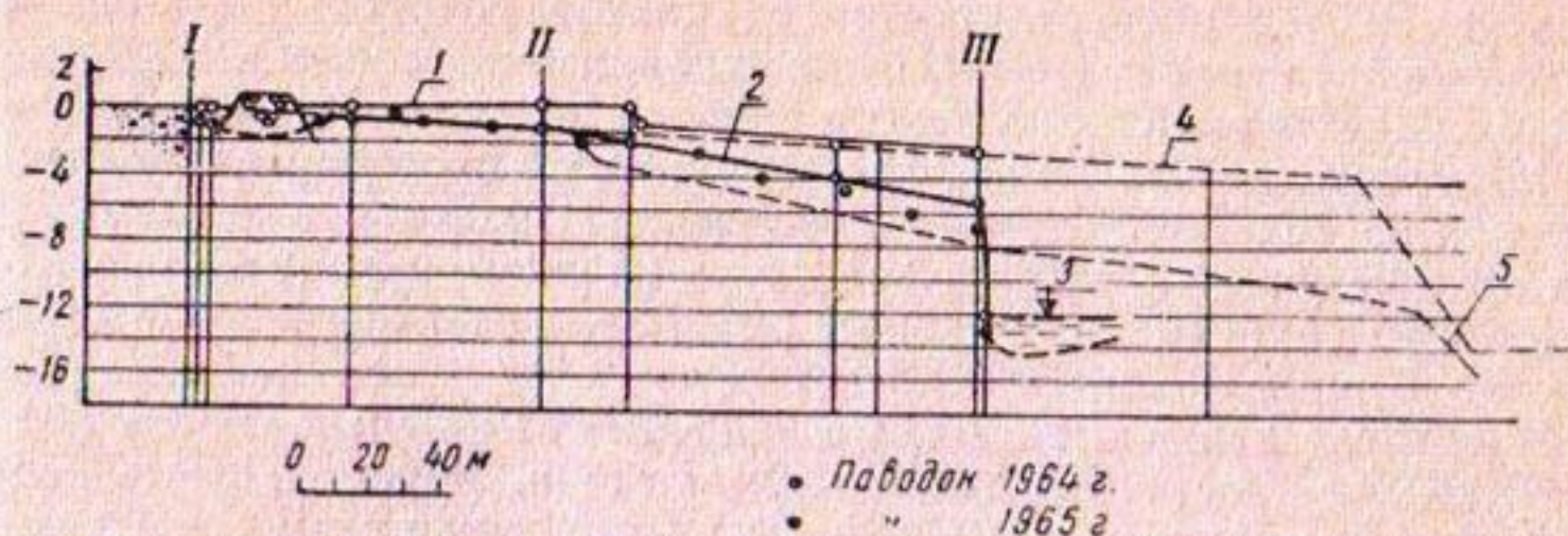
Рис. 2. Продольные профили отводящего канала и русло реки за ним:
