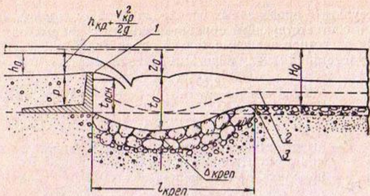
Рис. 13. Схема воронки размыва за перепадом:
