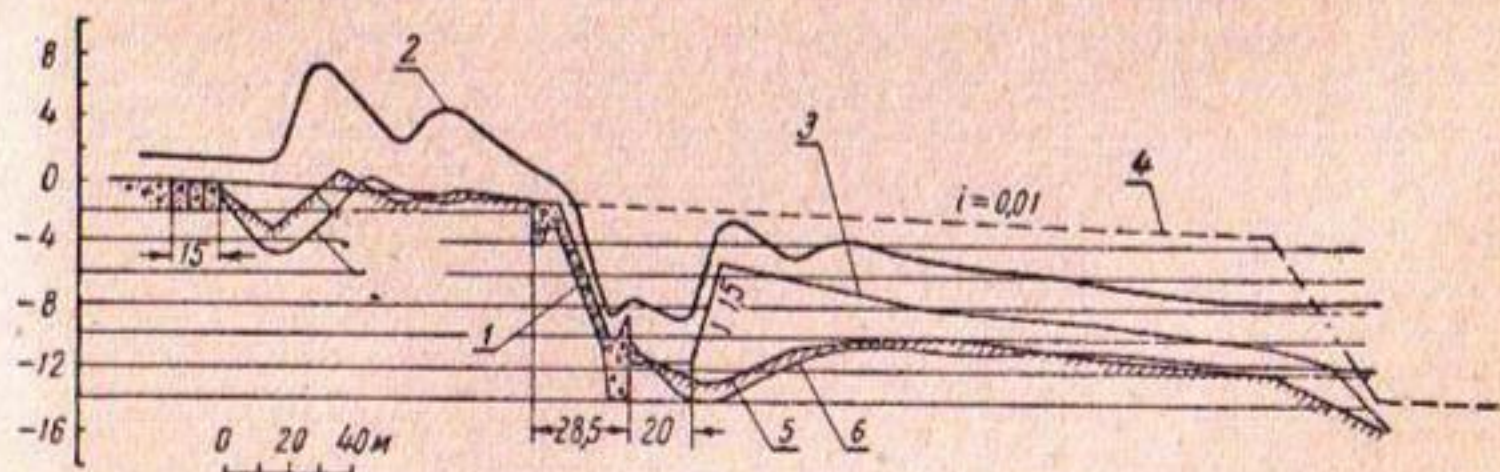
Рис. 5. Продольные профили отводящего канала (при наличии концевого перепада с удлиненным носком и расщепителями на нем) и русло реки за ним по моделированию паводков 1%-ной и 0,1%-ной обеспеченности:
