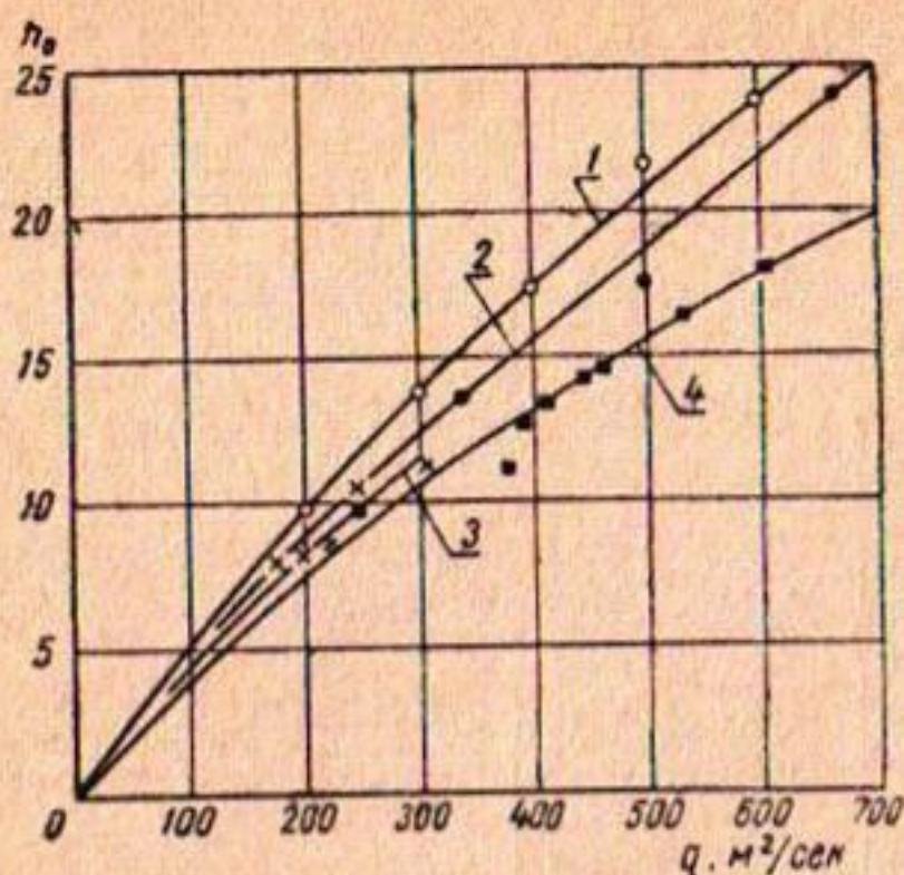
Рис. 2. Кривые h_0 = f(q) :
