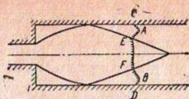
Рис. 5. Фронт гидравлического прыжка в пределах сужающейся части «листа» растекающегося бурного потока.
