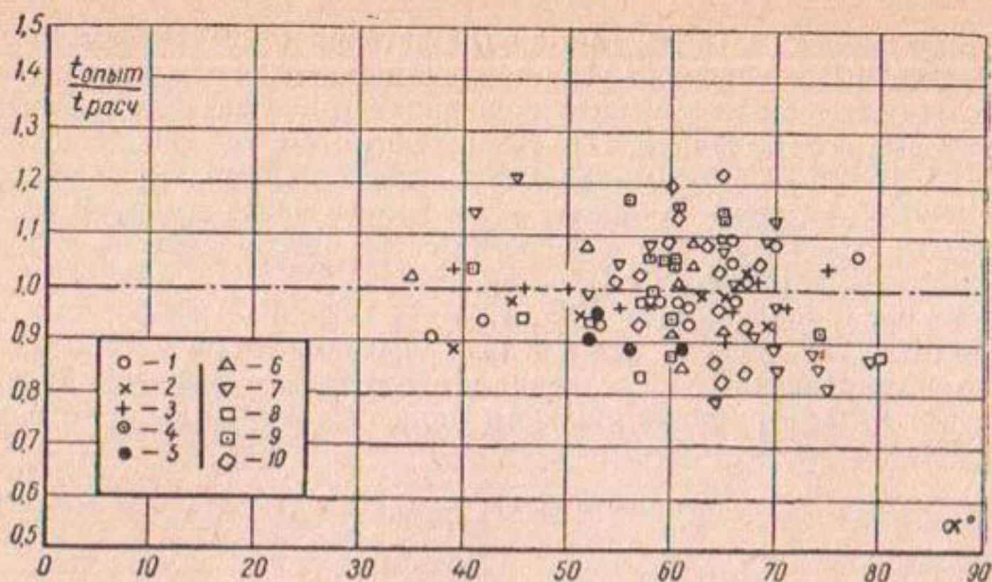
Рис. 8. График зависимости \frac{t_{\text{опыт}}}{t_{\text{расч}}} = f(\alpha^\circ) . t_{\text{расч}} — расчетная глубина, полученная по формуле (14);
