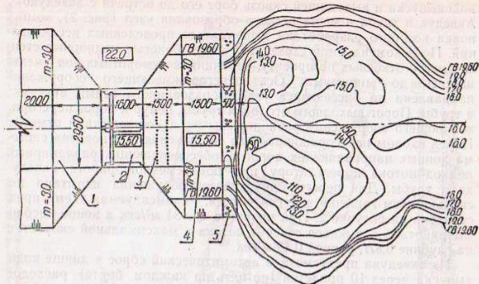
Рис. 3. Подпорное сооружение на 397 км канала:
