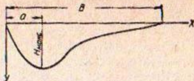
Рис. 4. Расчетная схема поперечного профиля русла в створе полузапруды:
