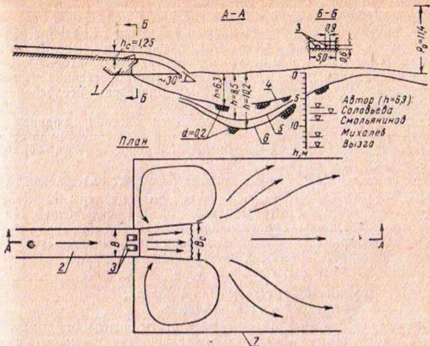
Рис. 1. Консольный водосброс Кондопожской ГЭС. Размывы русла в нижнем бьефе:
