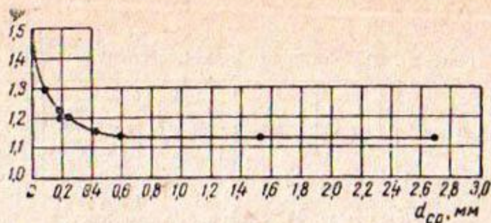
Рис. 3 Кривая зависимости \varphi = f(d_{cp}) .
