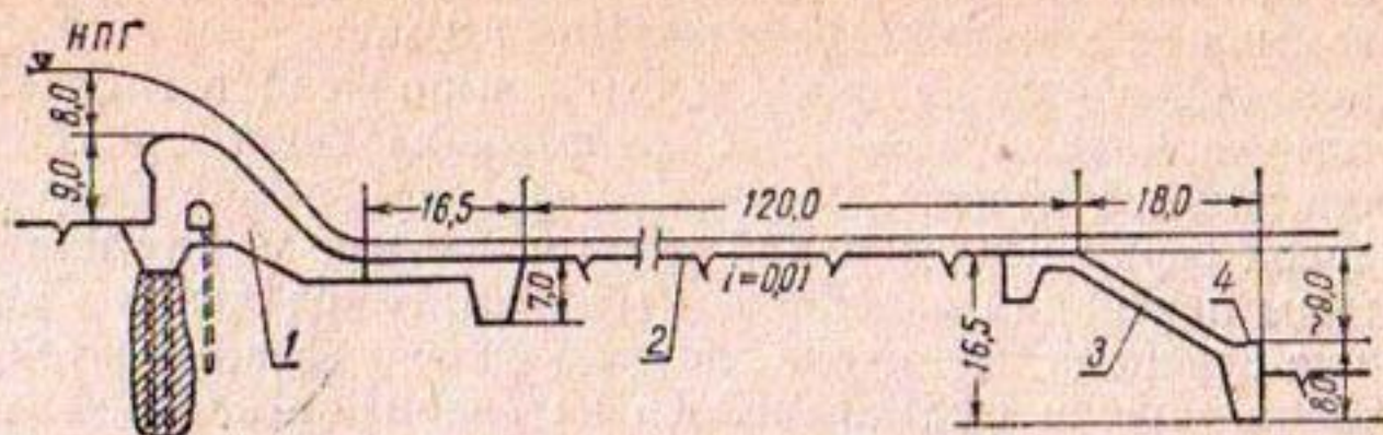
Рис. 1. Водосброс плотины:
