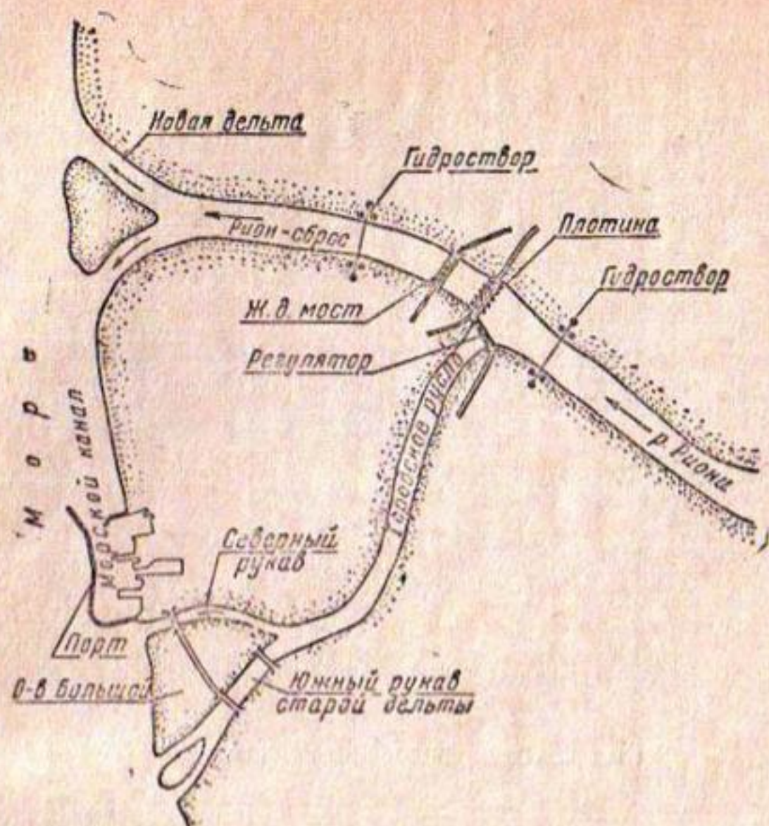
Рис. 1. Схематический план района вододелительного узла
