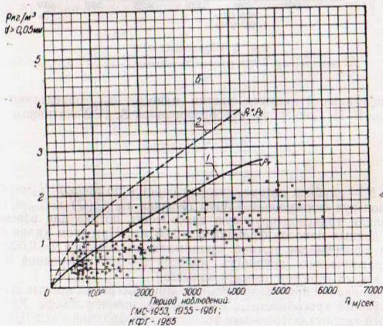
Рис. 5. Транспортирующая способность \rho . Амударьи для фракций d > 0,05 мм и данные наблюдений:
