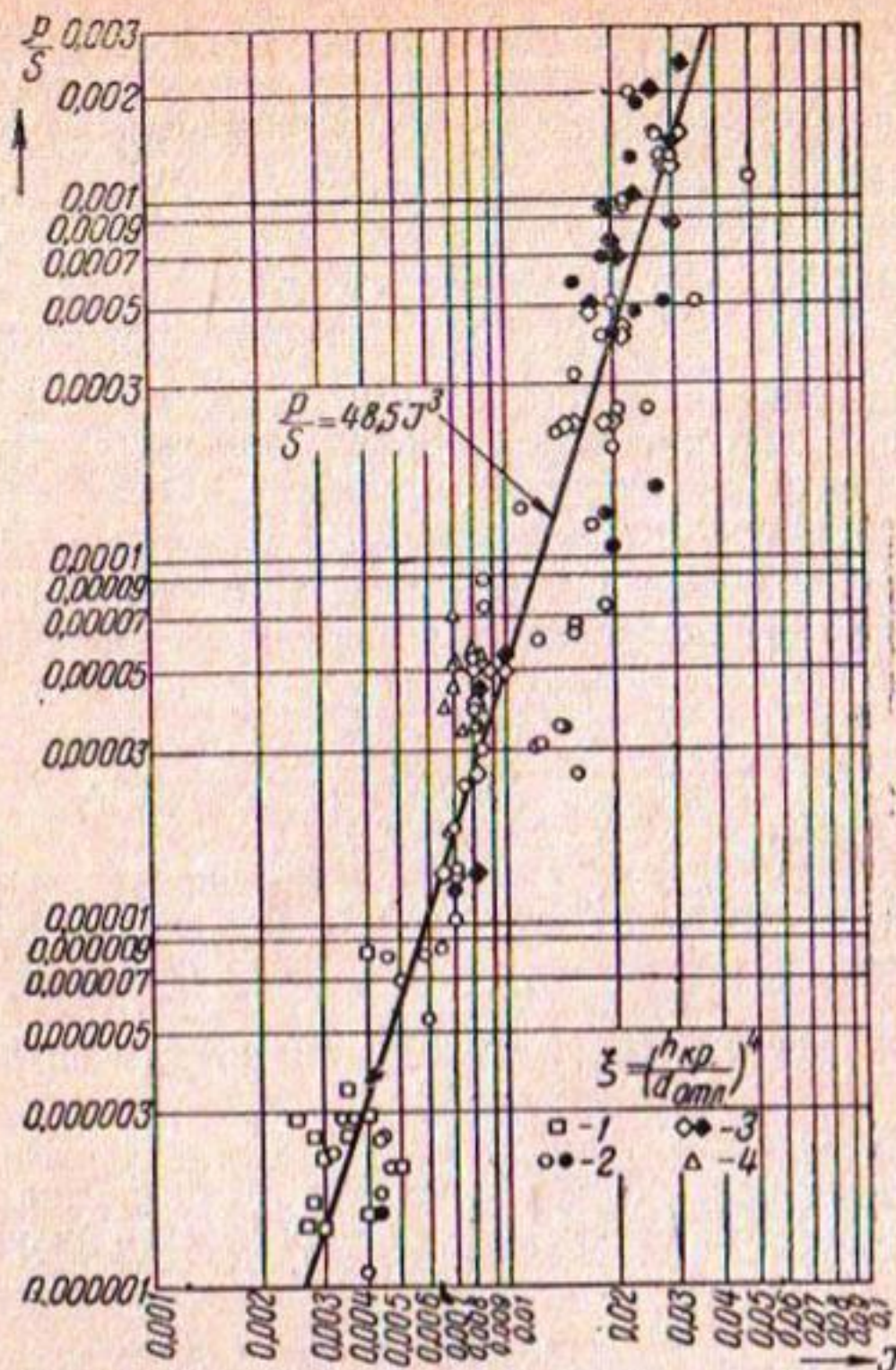
Рис. 11. Зависимость величины \frac{P}{S} от уклона потока I :
