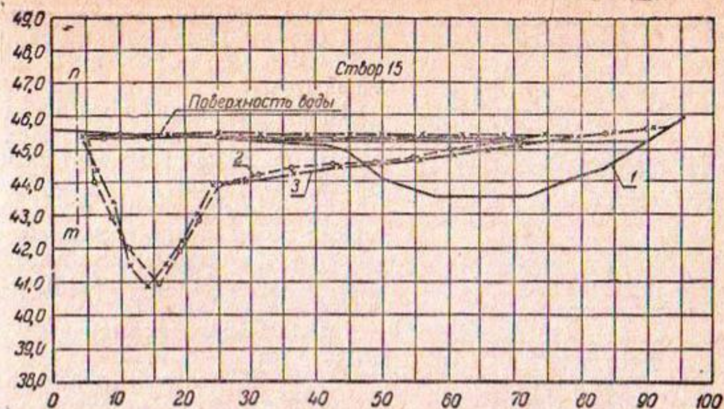
Рис. 2. Изменение поперечного профиля русла:
