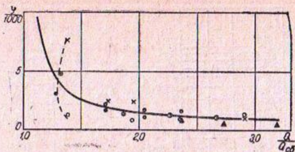
Рис. 9. График \varphi = \varphi \left( \frac{Q}{Q_{сб}} \right) .
