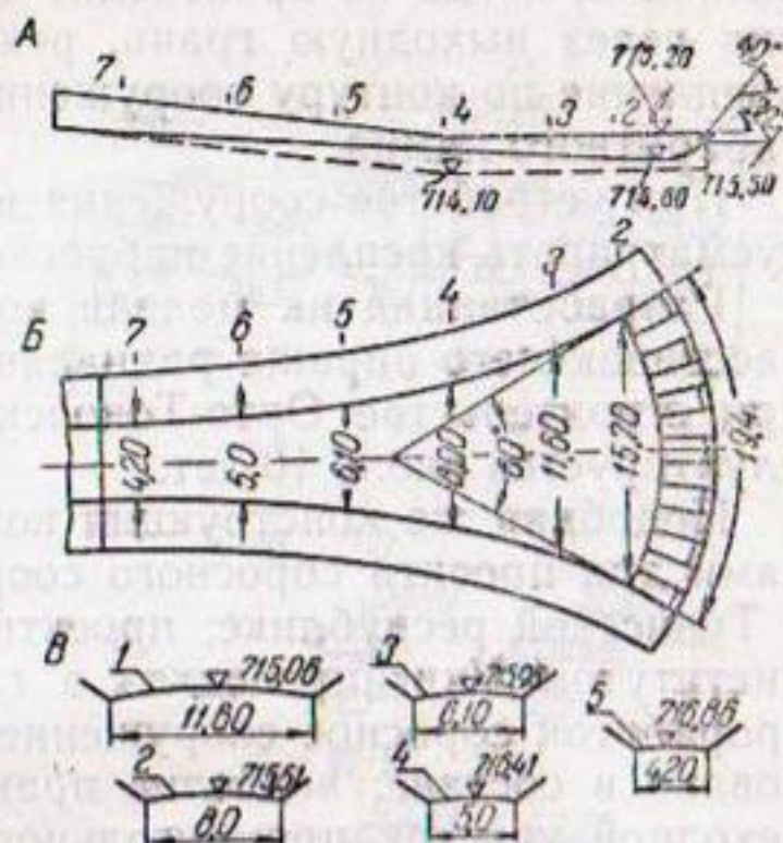
Рис. 1. Конструкция рассеивающего виража Орто-Токойского водохранилища: А — продольный разрез по оси; Б — план; В — поперечные профили:
