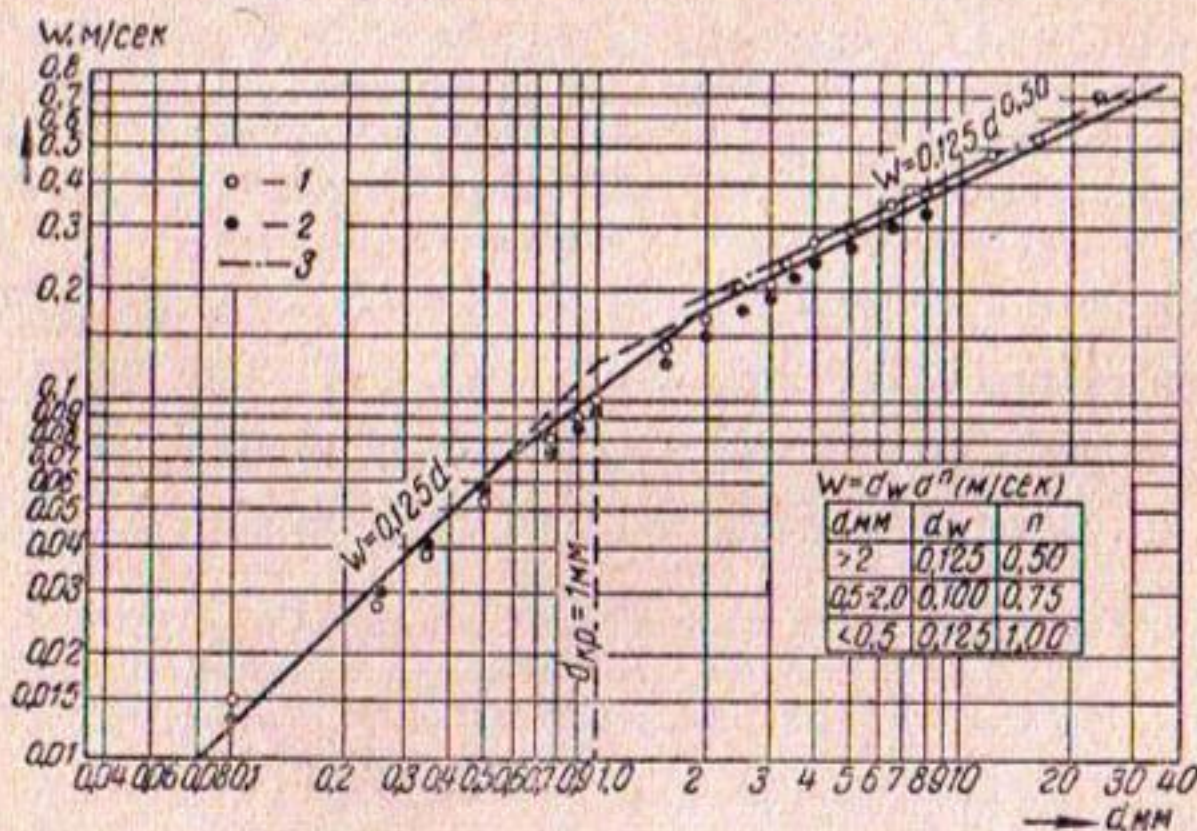
Рис. 7. График зависимости W=f(d) для гравелисто-песчаных частиц грунта ( \gamma \approx 2,65 \text{ т/м}^3 ). Гидравлическую крупность измеряли при температуре воды t^\circ = 10-12^\circ :
