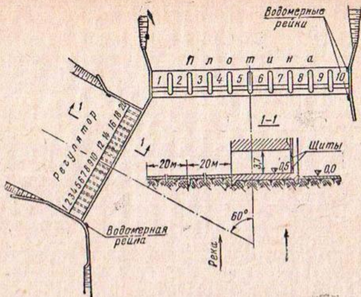
Рис. 2. Схема вододелительного узла.
