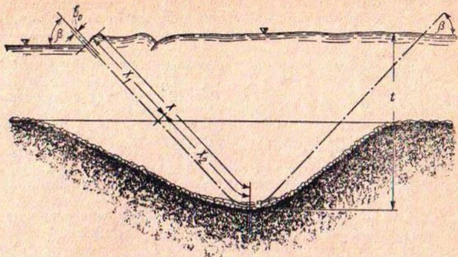
Рис. 1. Схема размыва несвязных грунтов падающей струей воды.
