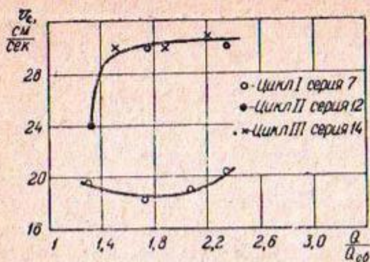
Рис. 5. График зависимости v_c от \frac{Q}{Q_{сб}} на период полуразмыва при d = 0,24 м.
