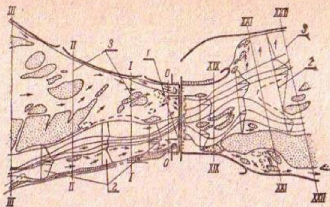
Рис. 3. План русла р. Зеравшан у плотины до ее реконструкции при проходе расхода 412 м³/сек:
