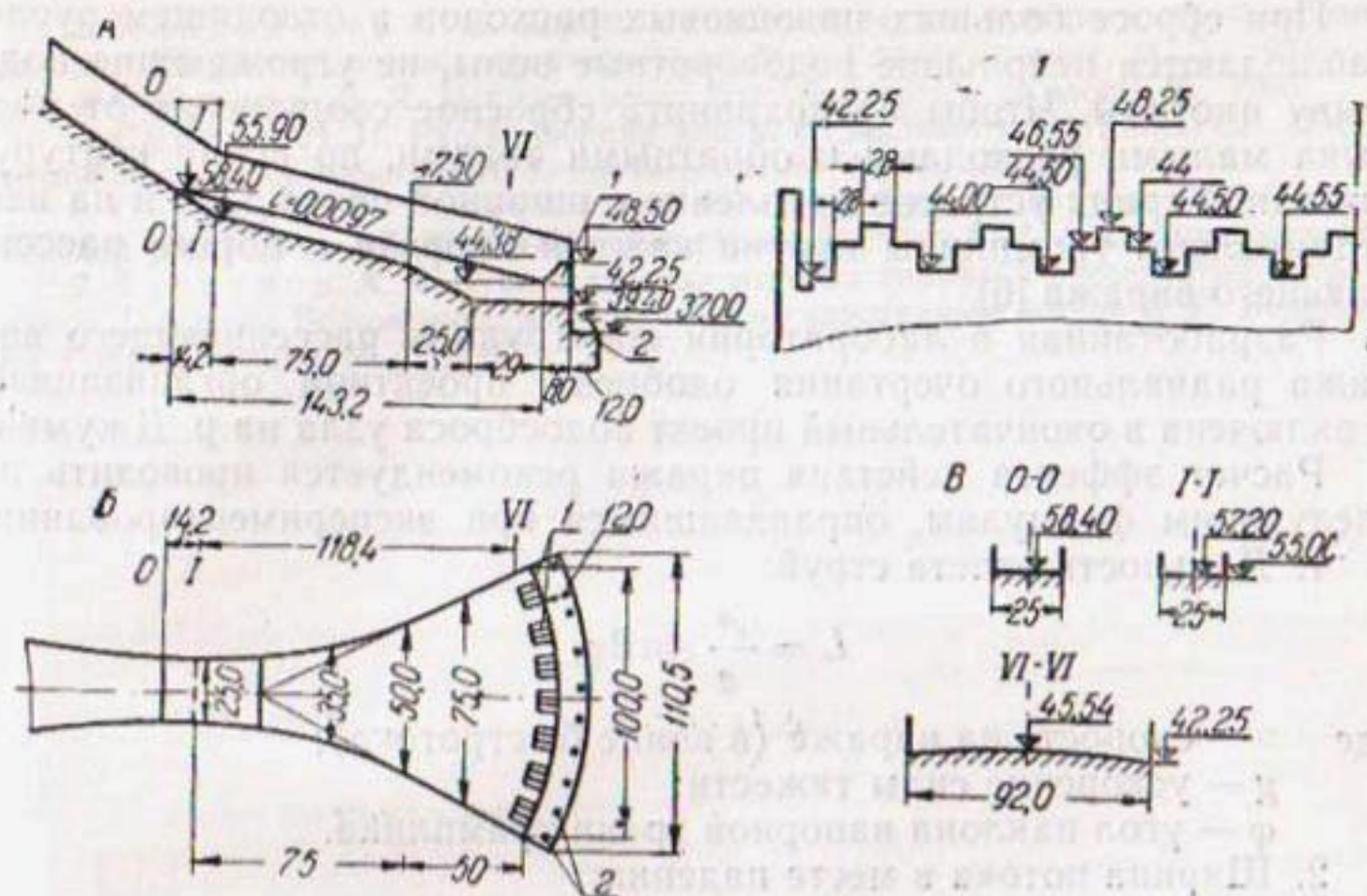
Рис. 3. Конструкция рассеивающего виажа водохранилища на р. Джумини: А — продольный разрез; Б — план; В — поперечные сечения.
