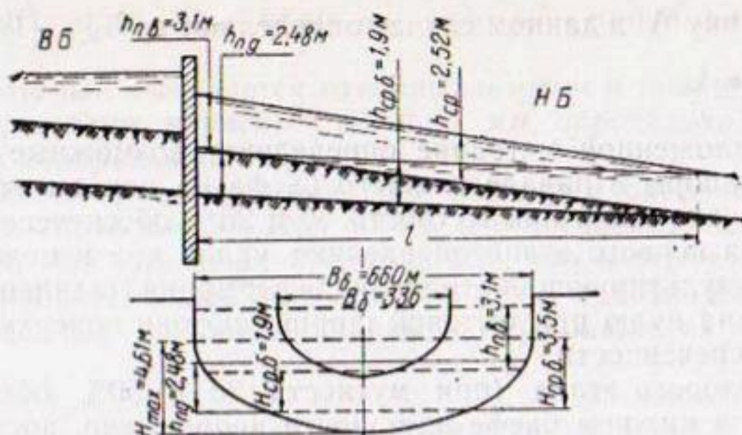
Рис. 8. Подъем дна и уровня воды на втором этапе эксплуатации гидроузла.
