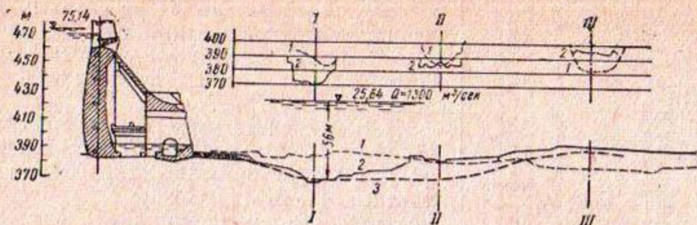
Рис. 4. Плотина Пикоти на р. Дуэро в Португалии. Размывы дна в натуре и на модели:
