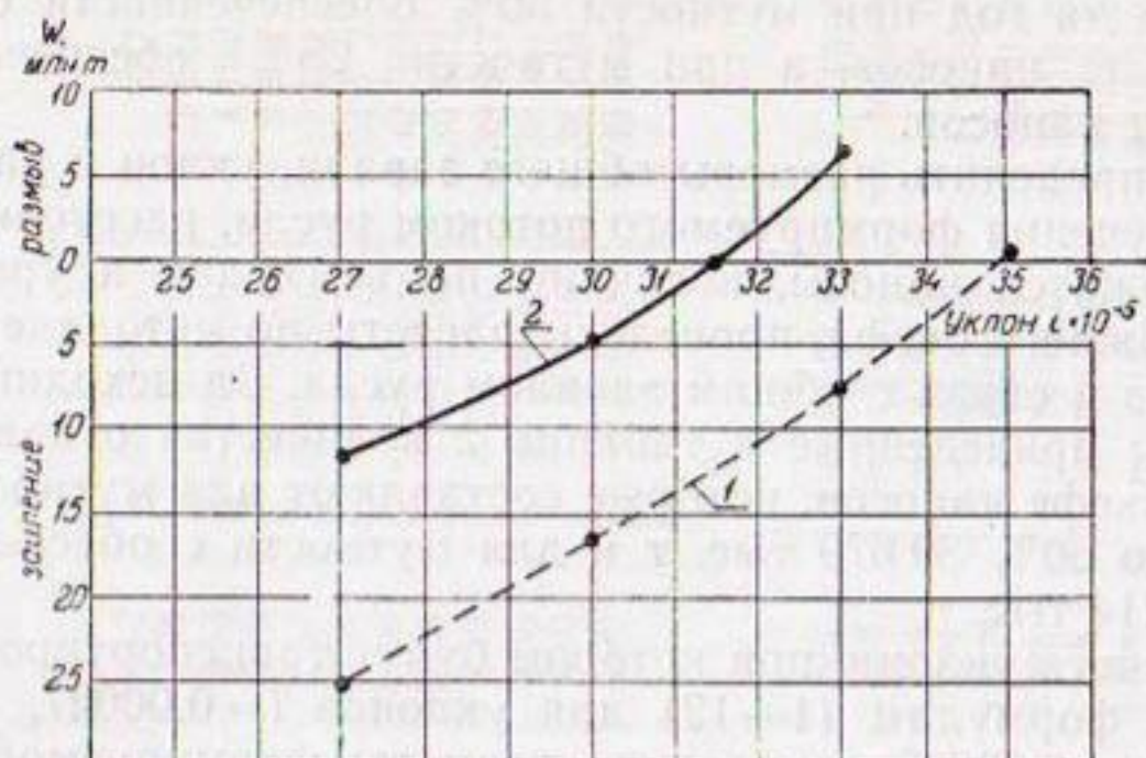
Рис. 10. Кривые изменения результирующих объемов заиления и размыва в зависимости от уклона русла на втором этапе развития:
