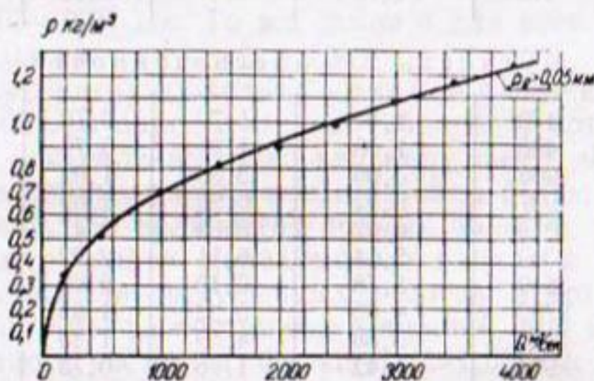
Рис. 6. Транспортирующая способность р. Амударья в районе Кизыл-Аяка (донные наносы).
