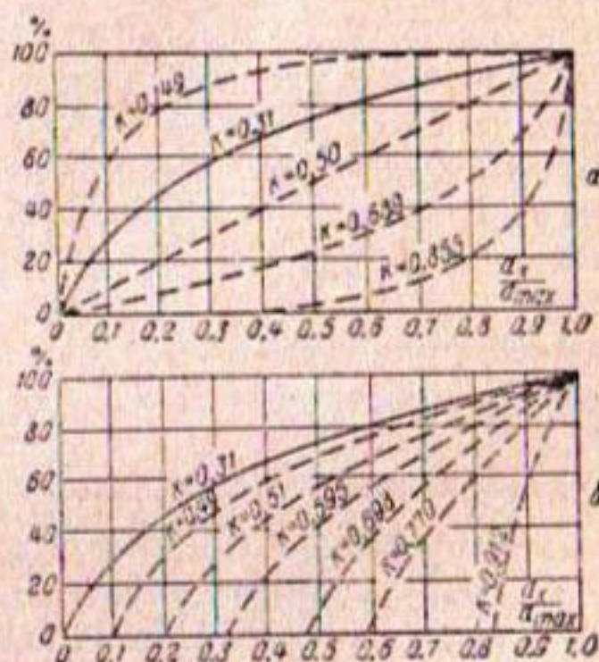
Рис. 3. Смеси частиц грунта, испытанные в опытах ( d_x — диаметр сита, через которое прошла данная фракция; d_{\text{max}} — максимальный диаметр частиц данной смеси грунта):
