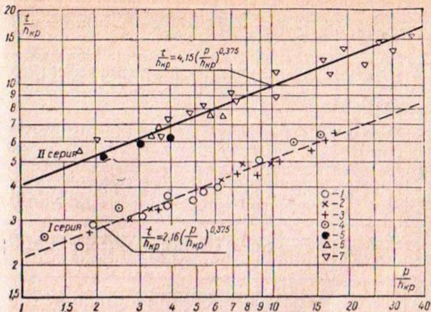
Рис. 4. График зависимости \frac{t}{h_{кр}} = f\left(\frac{p}{h_{кр}}\right) :
