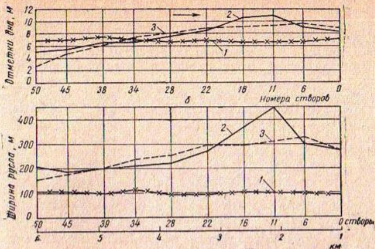
Рис. 4. Продольные профили дна и соответствующая им ширина русла Волго-Ахтубинского канала (1953 г.) (течение слева направо):
