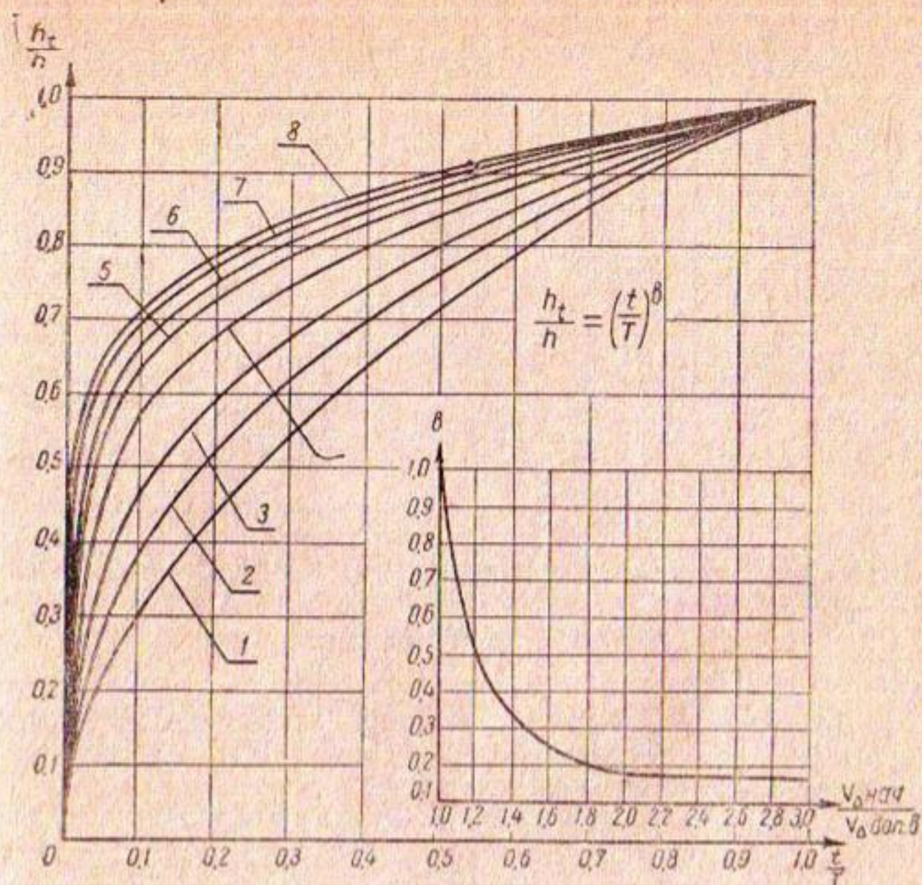
Рис. 4. Кривые зависимости относительной глубины размыва \frac{h_t}{h} от относительного времени размыва \frac{t}{T} для различных значений отношения \frac{v_{\Delta \text{нач}}}{v_{\Delta \text{доп.в}}} : 1 — \frac{v_{\Delta \text{нач}}}{v_{\Delta \text{доп.в}}} = 1,2 ; 2 — то же, = 1,3 ; 3 — то же, = 1,4 ; 4 — то же, = 1,6 ; 5 — то же, = 1,8 ; 6 — то же, = 2,0 ; 7 — то же, = 3 .
