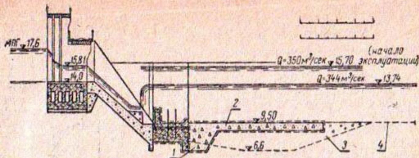
Рис. 1. Дамходжинский гидроузел. Разрез по водосливу:
