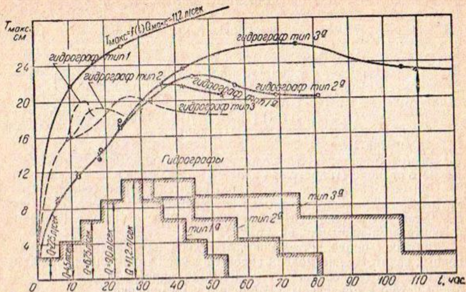
Рис. 7. График T_{\max} = T_{\max}(t) при пропуске различных типов гидрографов в выходном русле типа 1.
