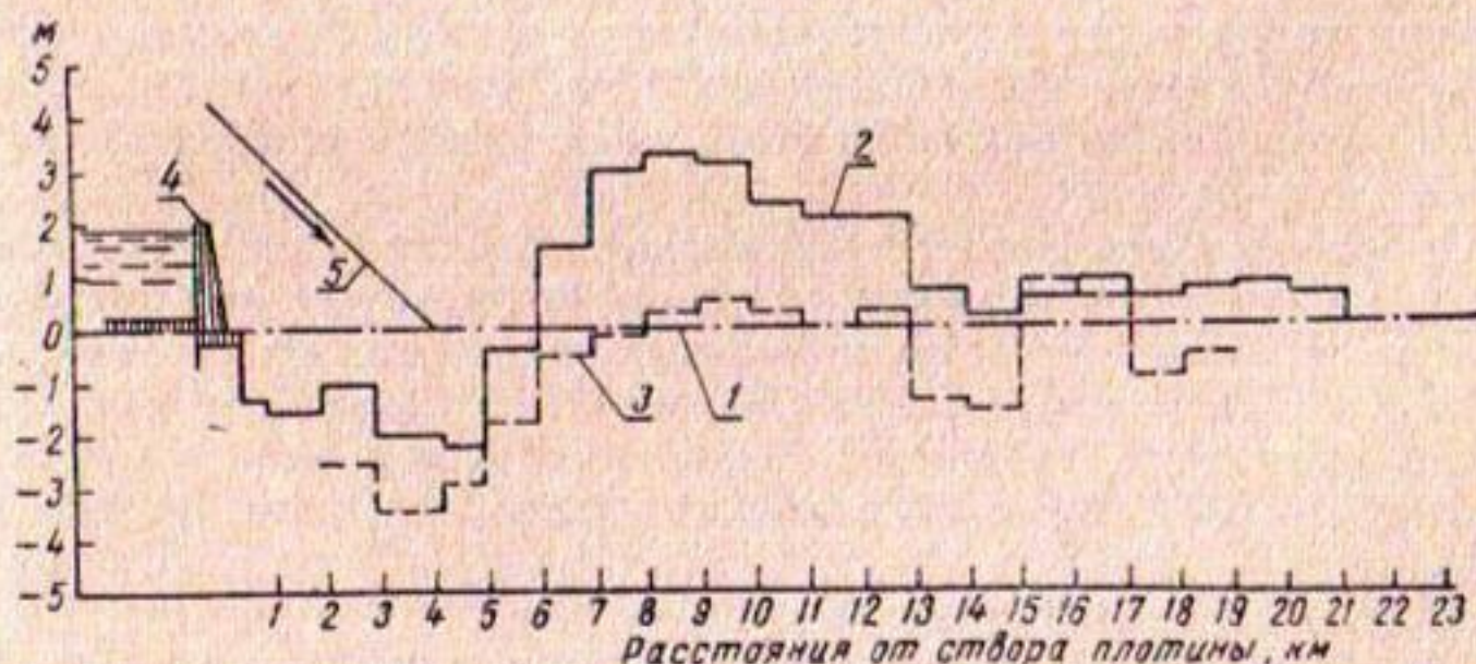
Рис. 3. График движения деформаций русла р. Волги в нижнем бьефе Волжской ГЭС имени В. И. Ленина:
