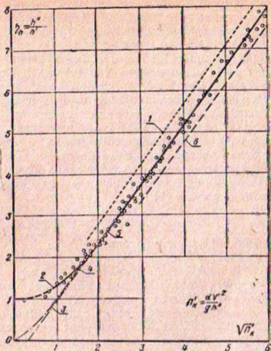
Рис. 1. Сравнение точности определения коэффициента сопряжения взаимных глубин \eta_m = \frac{h''}{h'} по различным формулам (опытные данные Бахметева, Гибсона, Эйнвахтера, Сметаны и др.):
