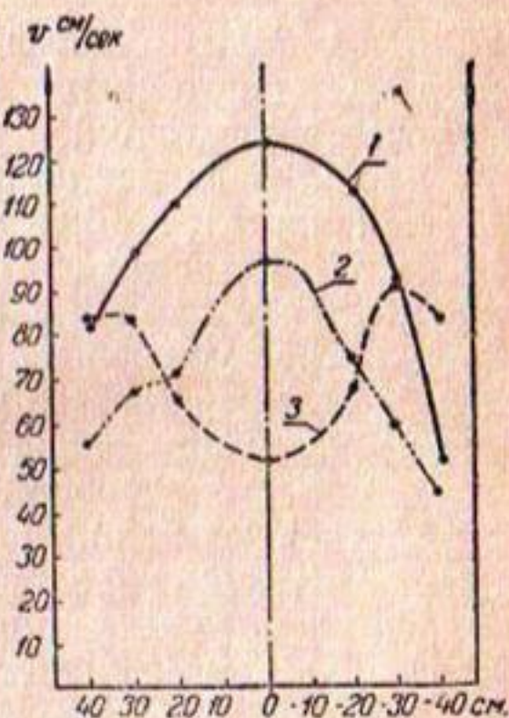
Рис. 6. Эпиюры скоростей на удалении x = 350 м от сооружения при постоянном расходе и бытовых глубинах: 1 — при 12,8 м; 2 — при 15,0 м; 3 — при 16,0 м.
