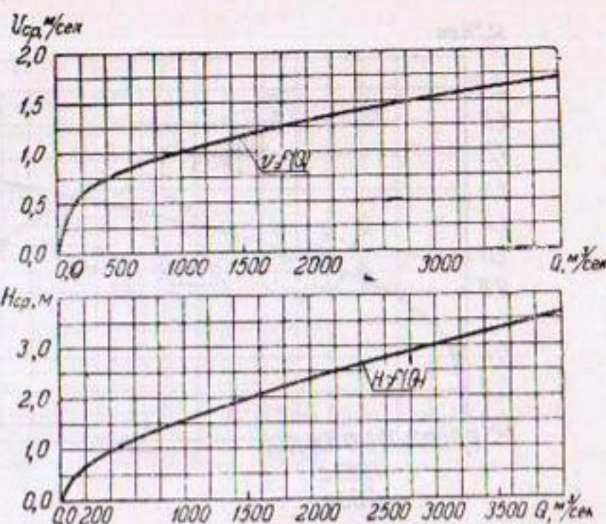
Рис. 2. Кривые v = f(Q) и H = f(Q) для расчетного формируемого потоком русла.
