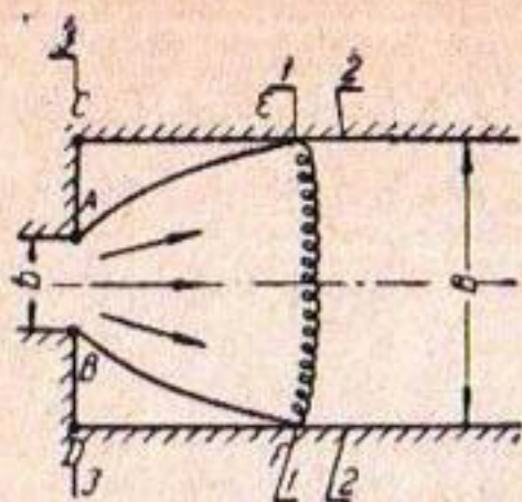
Рис. 1. Предельное положение гидравлического прыжка при переходе от свободного растекания потока к сбойному течению:
