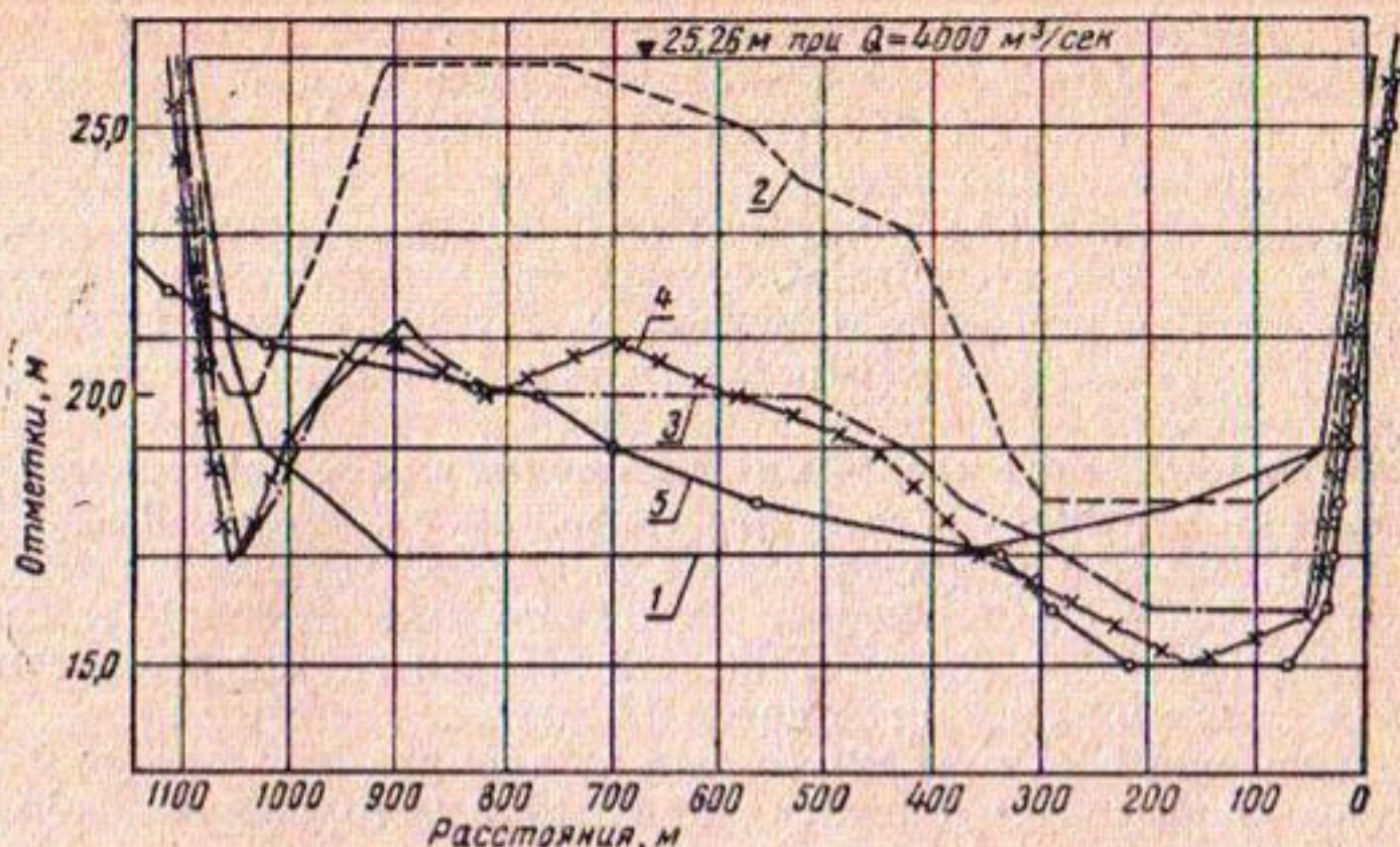
Рис. 2. Совмещенные поперечники русла р. Волги в 7 км ниже створа Волжской ГЭС имени В. И. Ленина, замеренные за ряд лет (отметки условные):
