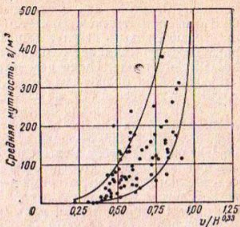
Рис. 1. Зависимость между средней мутностью (руслоформирующих фракций) и величиной \frac{u}{H^{0.33}}
