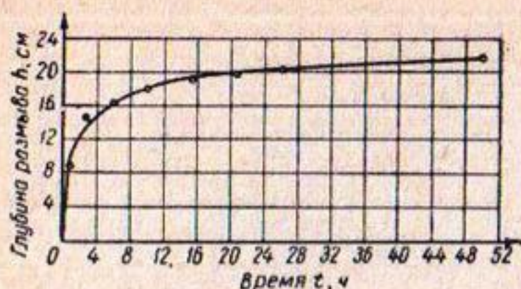
Рис. 3. Кривая зависимости глубины размыва от времени.
