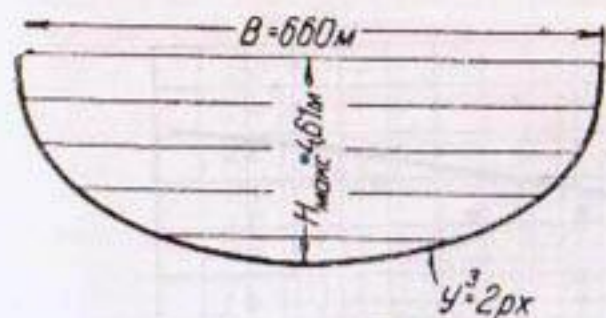
Рис. 1. Расчетное формируемое потоком русло р. Амударьи:
