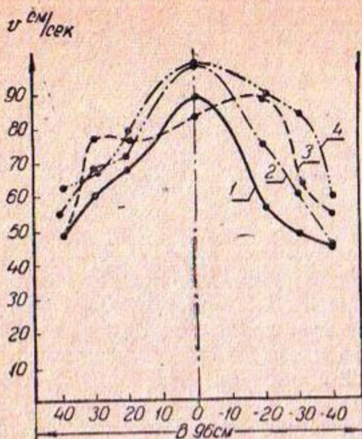
Рис. 3. Эпюры поверхностных скоростей на разном удалении от сооружения:
