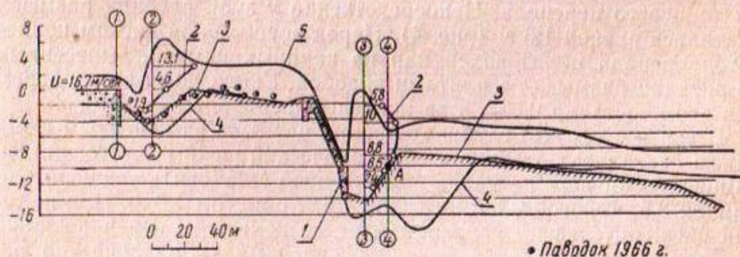
Рис. 3. Продольные профили отводящего канала и русла реки за ним (при наличии концевого перепада) по моделированию паводков 1%-ной и 0,1%-ной обеспеченности:
