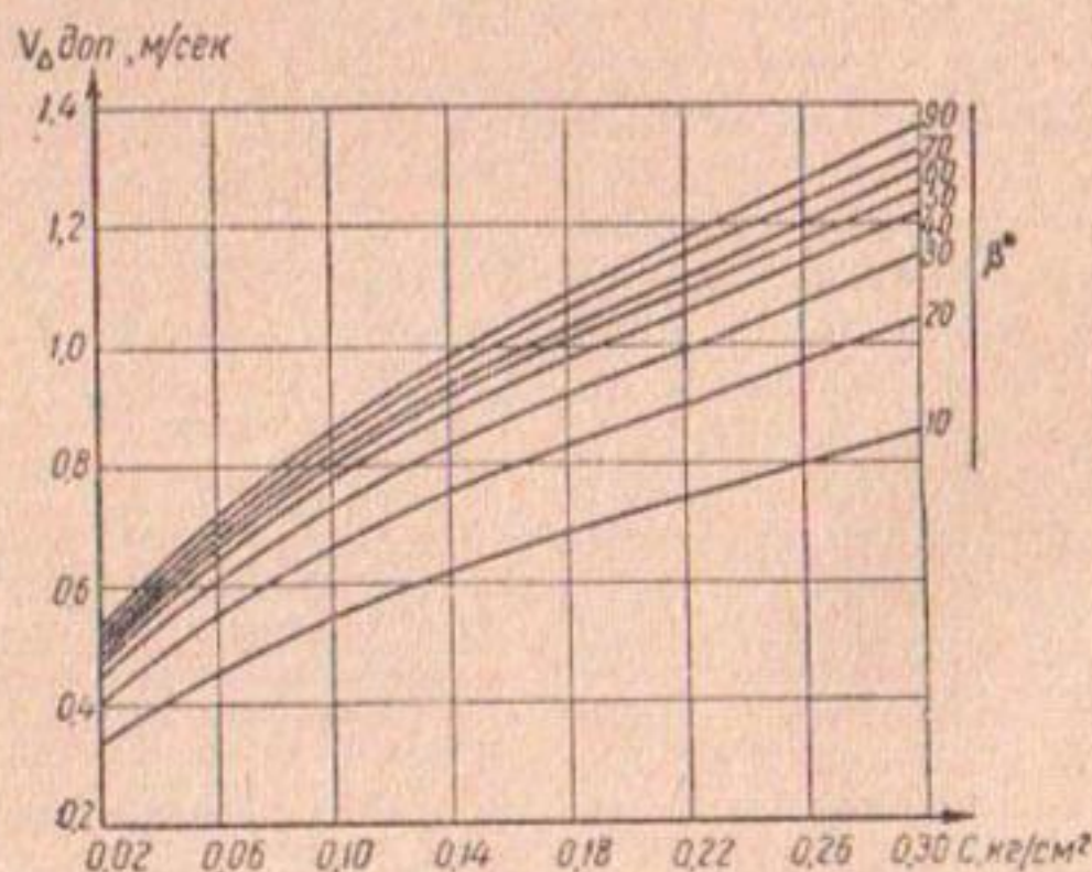
Рис. 2. Кривые зависимости допускаемой (неразмывающей) донной скорости в воронке размыва v_{\Delta \text{доп.в}} от сцепления c и угла наклона входа струи \beta .
