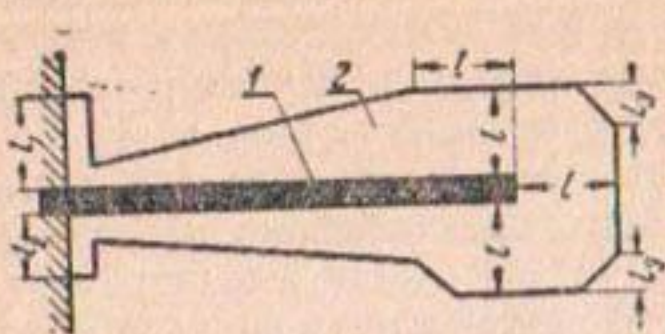
Рис. 5. Схема туюфячного крепления полузапруды:
