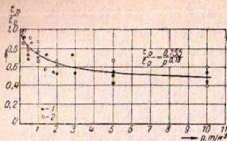
Рис. 5. График зависимости \frac{t_p}{t_0} = f(\rho) :
