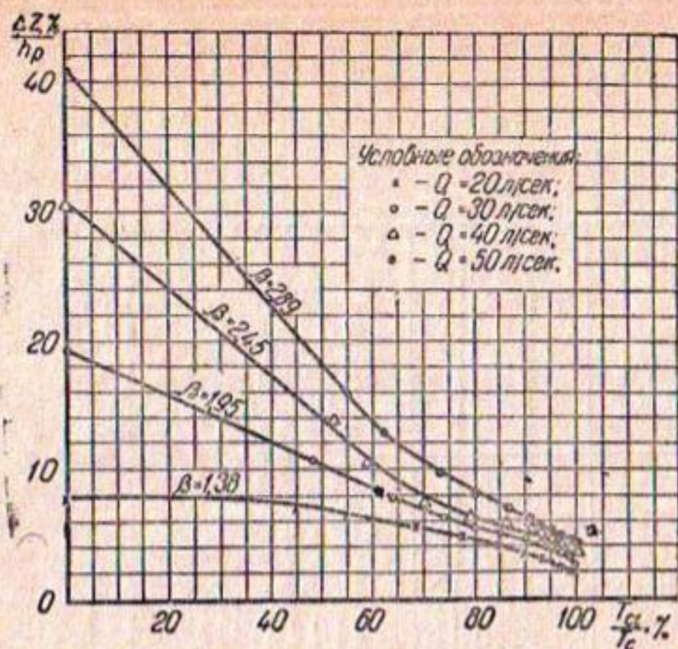
Рис. 3. График зависимости \frac{\Delta z}{h_p} от относительной глу-
