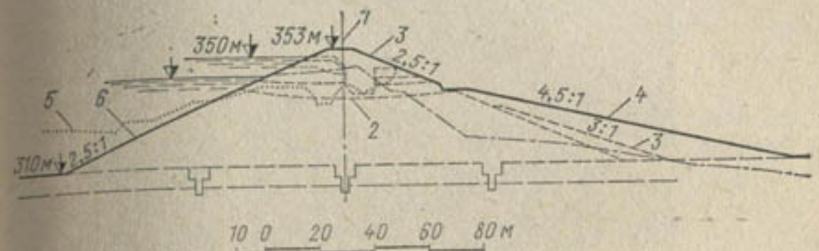
Рис. 18. Поперечное сечение плотины Сен-Фернандо.
