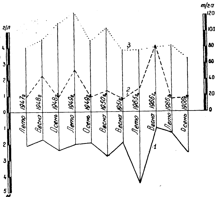
Рис. 1. Глубина залегания, степень минерализации грунтовых вод и запасы солей в аллювиально-луговых (тугайных) почвах.
