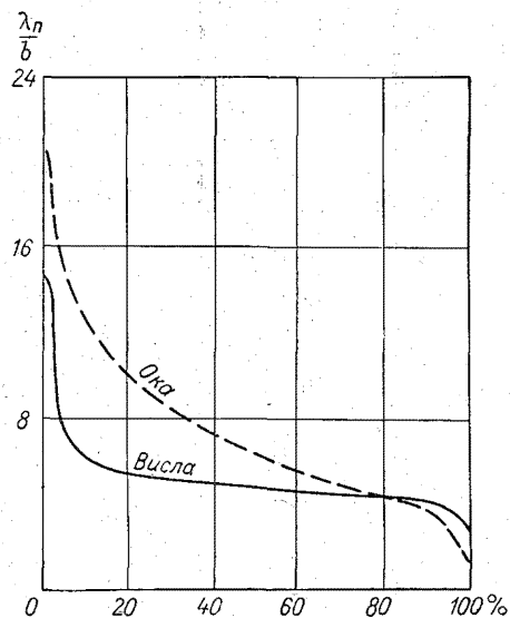
Рис. 38. Кривые обеспеченности относительных шагов — побочней рек Оки и Вислы.
