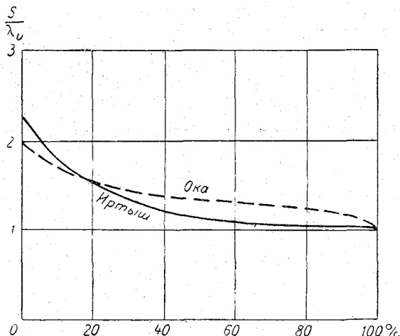
Рис. 42. Кривые обеспеченности степени выраженности ограниченно меандрирующих излучин рек Оки и Иртыша.
