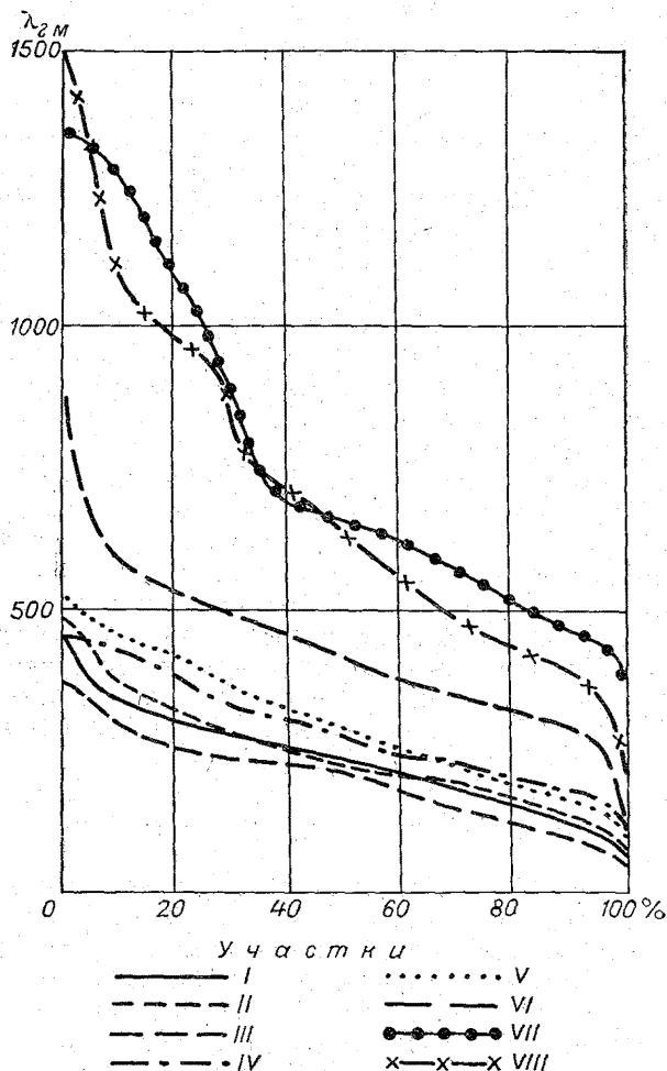
Рис. 30. Кривые обеспеченности шагов ленточных гряд для бесприточных участков.
