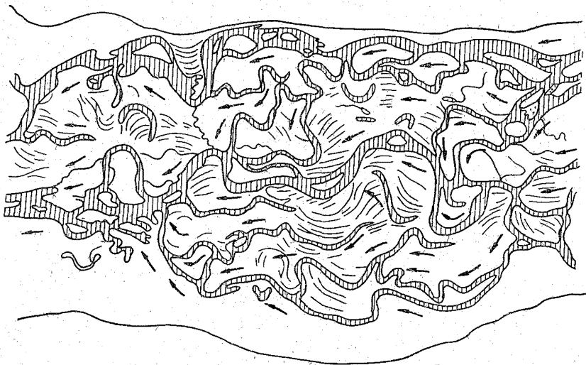
Рис. 69. Участок реки с пойменной многорукавностью. Течения на затопленной пойме хорошо согласуются с направлением протоков во все фазы половодья.
