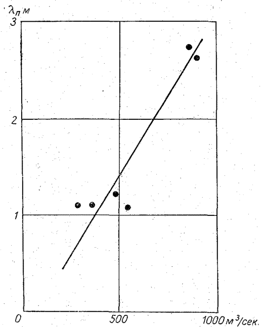
Рис. 39. Связь шагов побочней на р. Оке со средними годовыми расходами воды.
