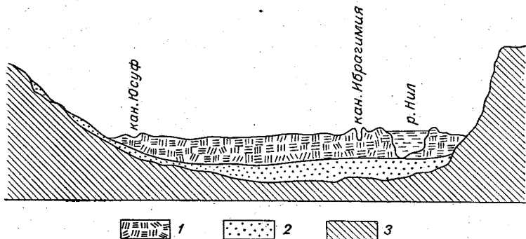
Рис. 59. Поперечный разрез долины р. Нила.
