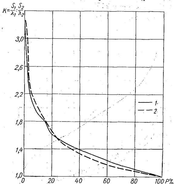
Рис. 45. Кривые обеспеченности параметра K = \frac{S_1}{\lambda_1} : \frac{S_2}{\lambda_2} .
