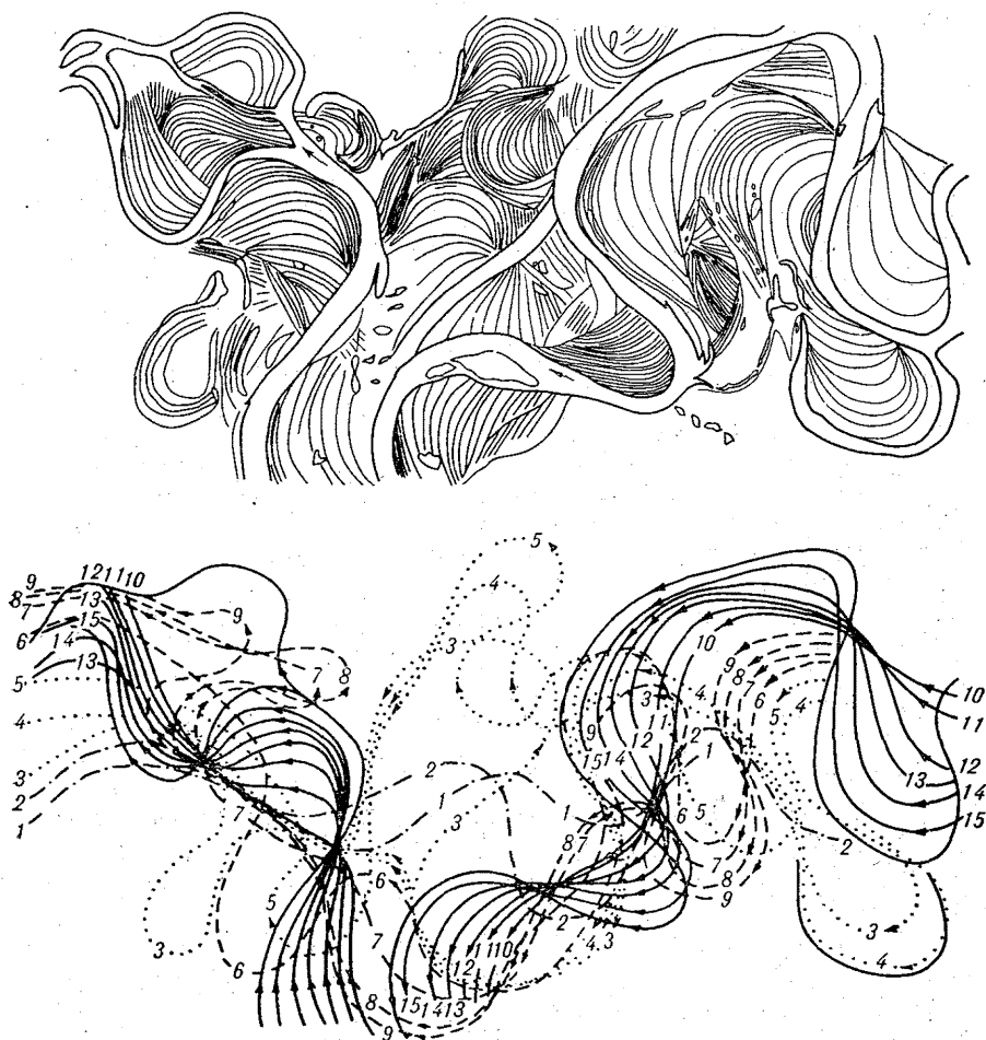
Рис. 56. Веера перемещения русла р. Оки.
