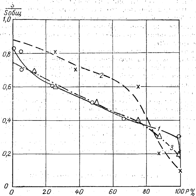
Рис. 53. Кривые обеспеченности \frac{S}{S_{\text{общ}}} для одноплёсовых (1), двухплёсовых (2) и многoplёсовых (3) излучин.
