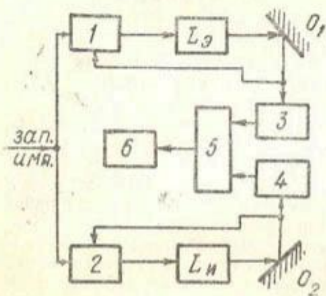
Рис. 1. Блок-схема акустического измерителя уровня жидкостей.
