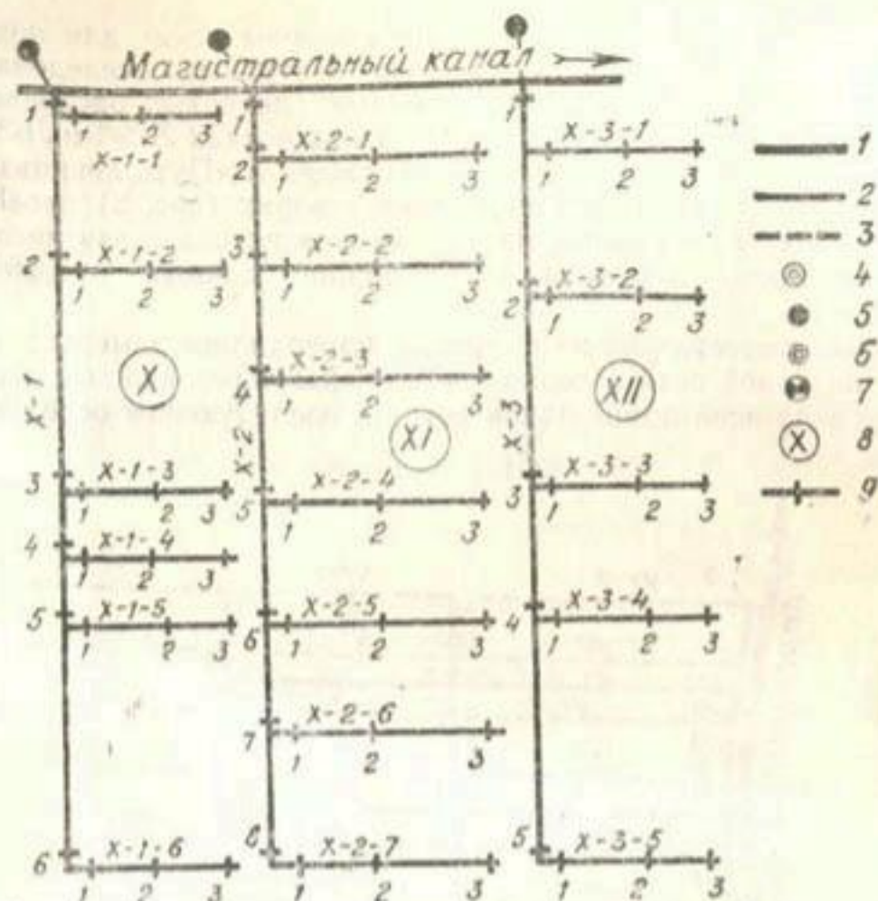
Рис. 1. Выборочная схема оросительной сети хлопководческого совхоза «Теджен» в зоне орошения Каракумского канала: 1—бетонный канал; 2—лотковый распределитель; 3—трубопровод; 4—водозабор из Каракумского канала в бетонный канал; 5—водозабор из бетонного канала в лоток; 6—водозабор из лотка в трубопровод; 7—насосная станция; 8—номер поливного массива; 9—закрепленный гидрометрический створ и его номер.
