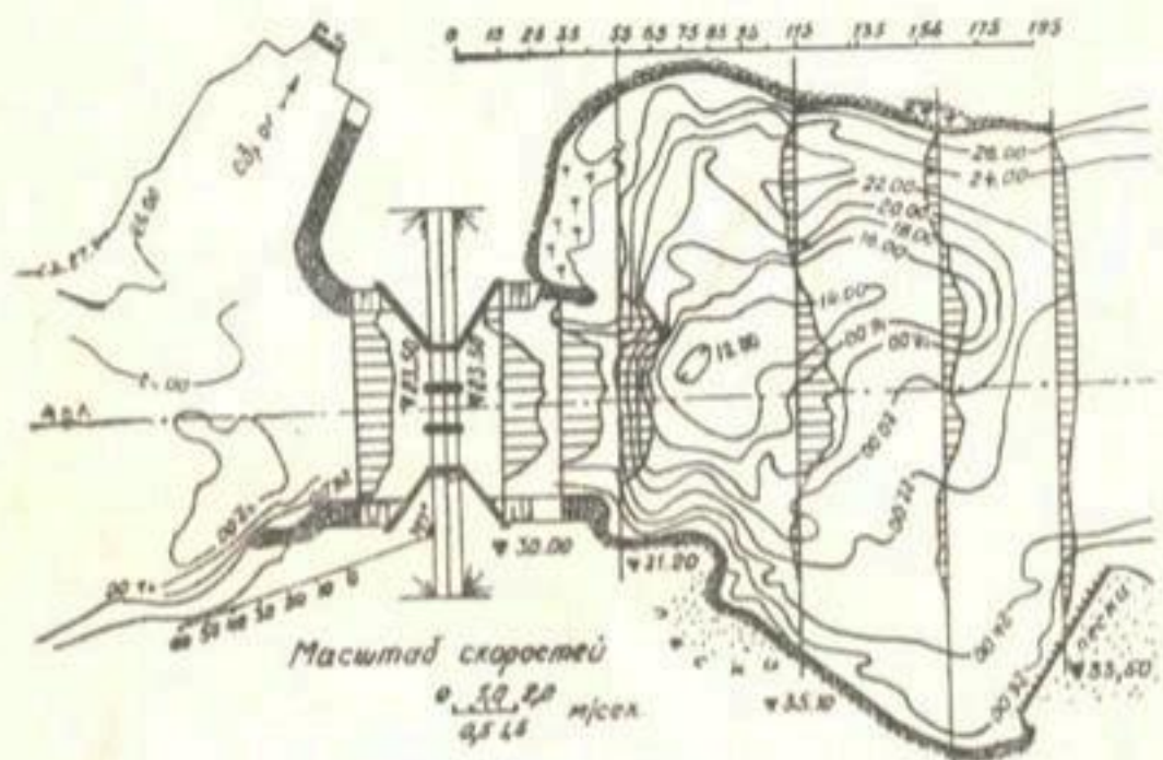
Рис. 1. Донные, боковые размывы и распределение скоростей потока в нижнем бьефе перегораживающего сооружения на Каракумском канале.
