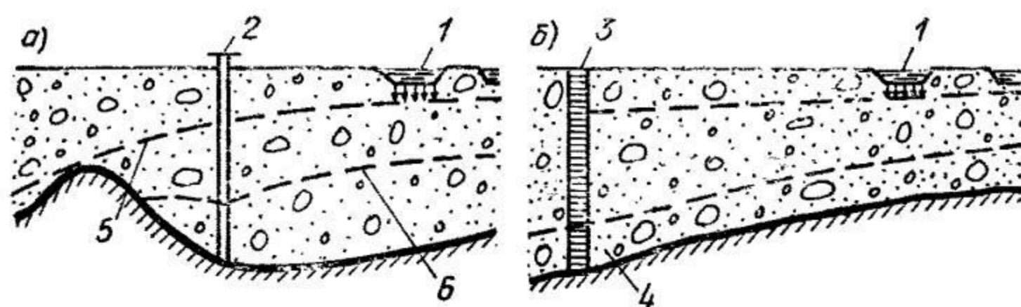
Рис. 13.1. Схемы подземных водохранилищ
