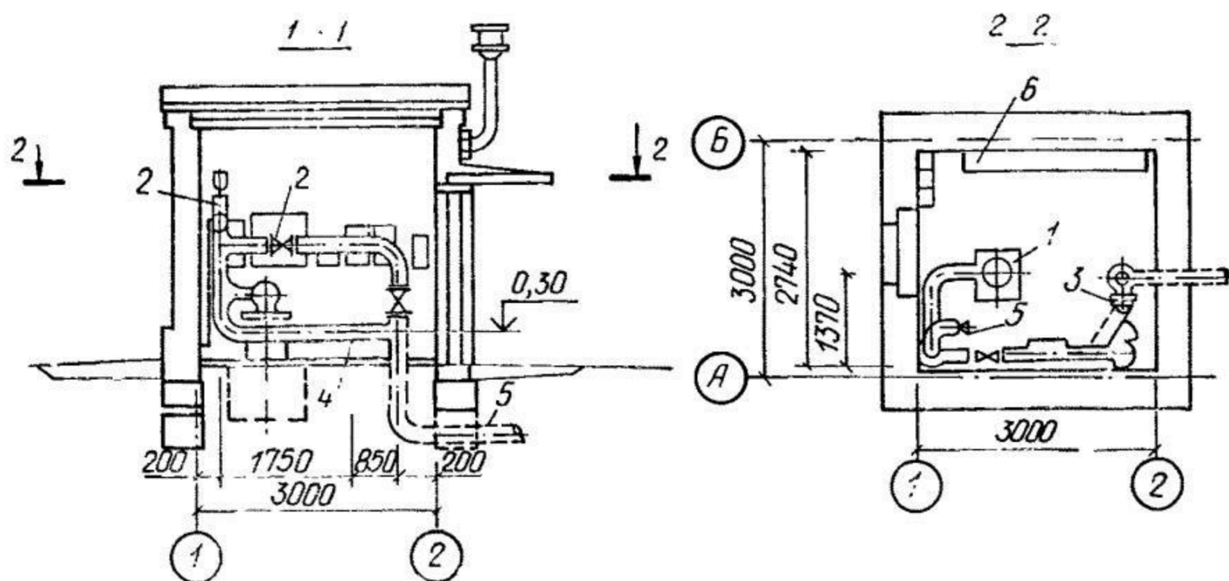
Рис. 5.1. Насосная станция над скважиной (наземная)
