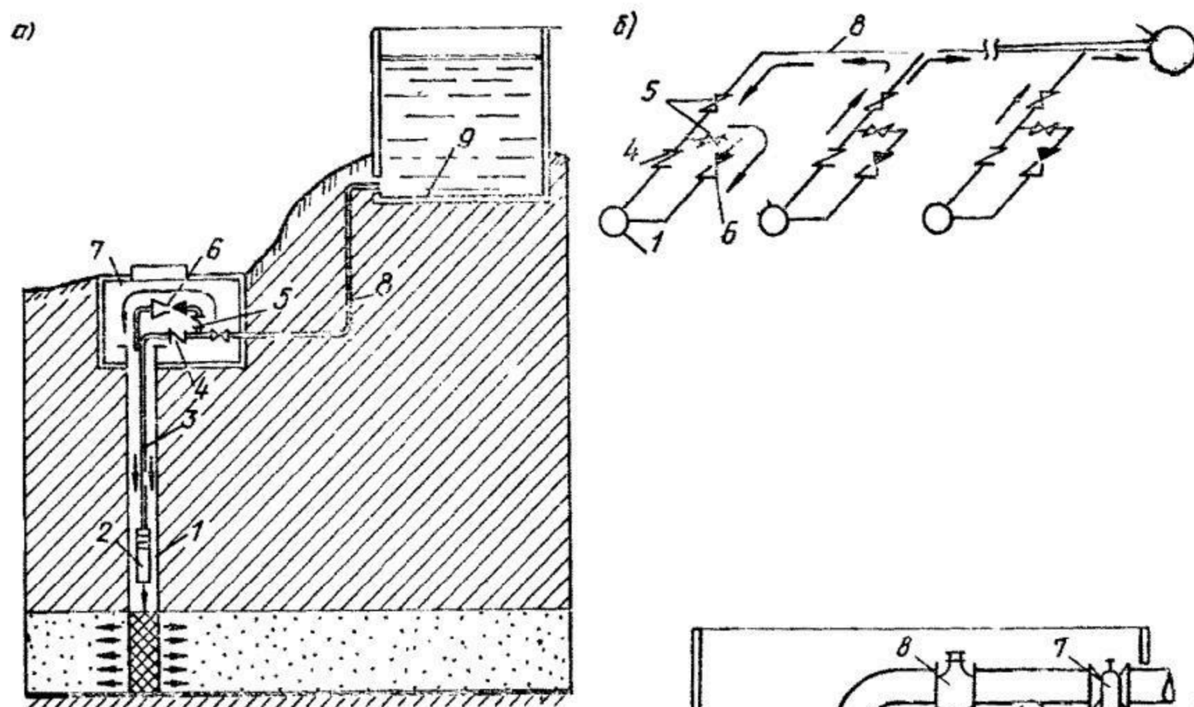
Рис. 21.3. Система водоснабжения (а, б) с установками обезжелезивания циклического типа
