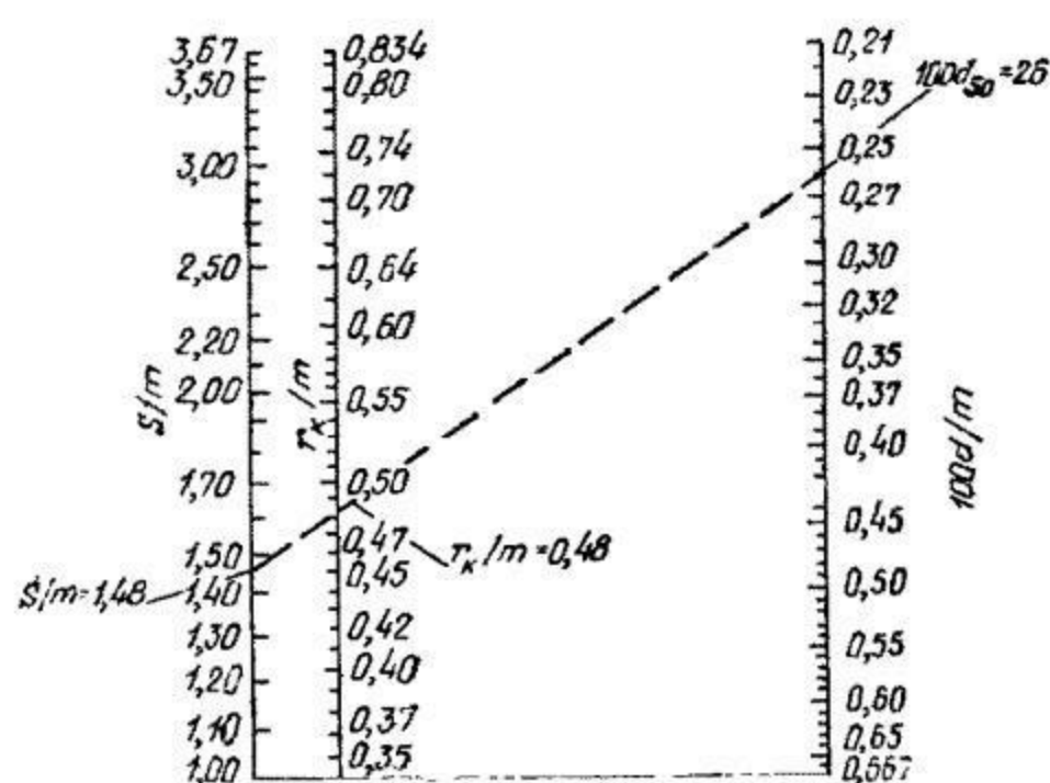
Рис. 14.2. Номограмма к определению радиуса каверны бесфильтровой скважины
