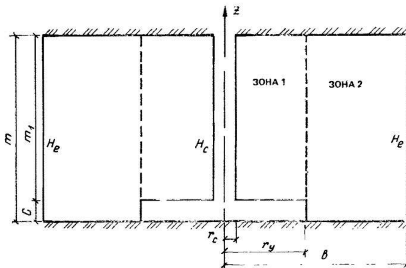
Рис. 14.5. Схема к расчету скважины с уширенным основанием
