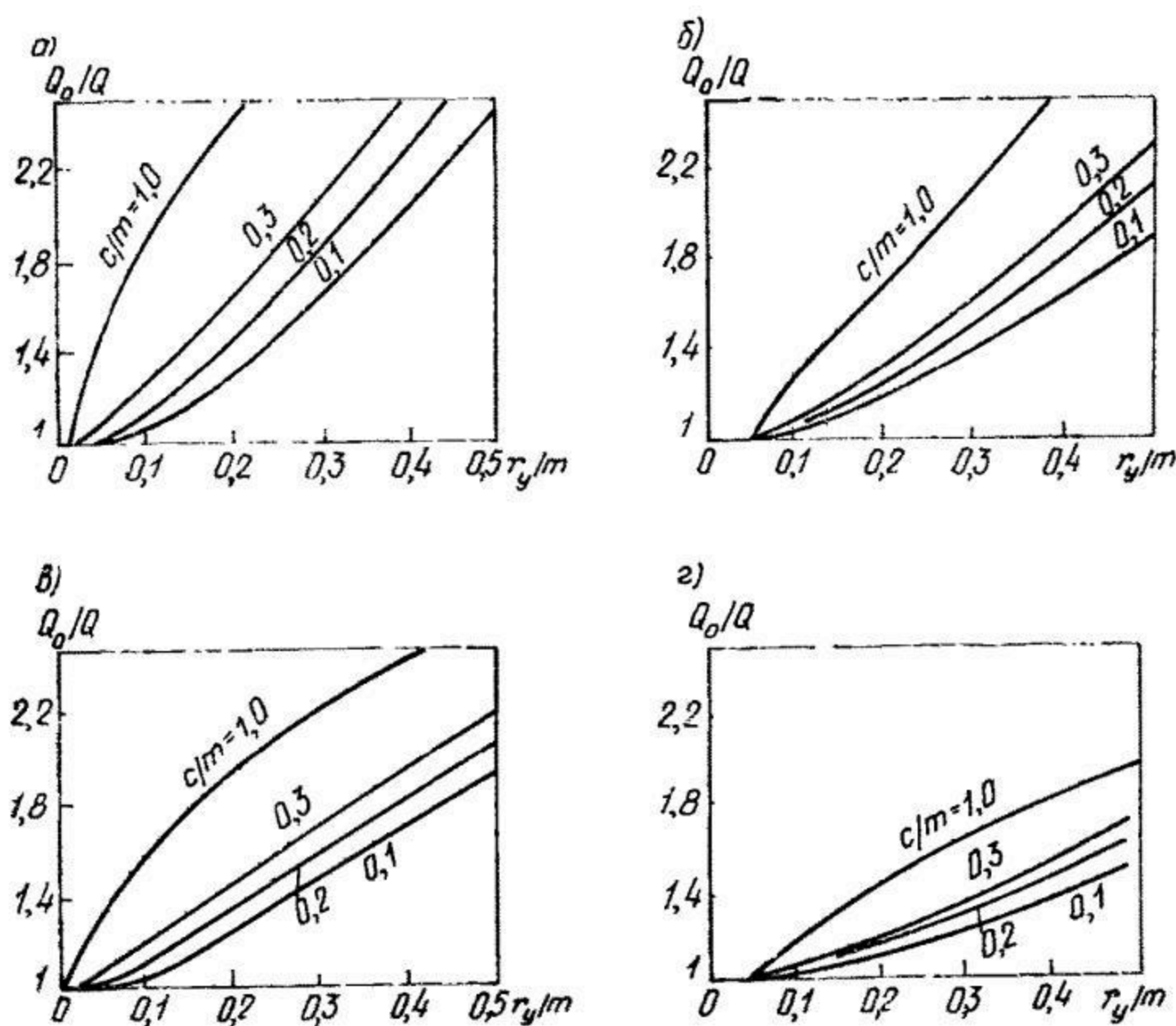
Рис. 14.6. Влияние радиального уширения на производительность скважин
