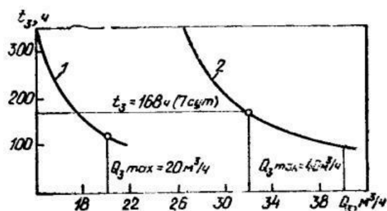
Рис. 21.24. Зависимости t_3 = f(Q_3) 1 — схема со свободным наливом: N=7 , Q_s=315 м³/ч; 2 — схема с принудительной закачкой: N=14 , Q_s=630 м³/ч
