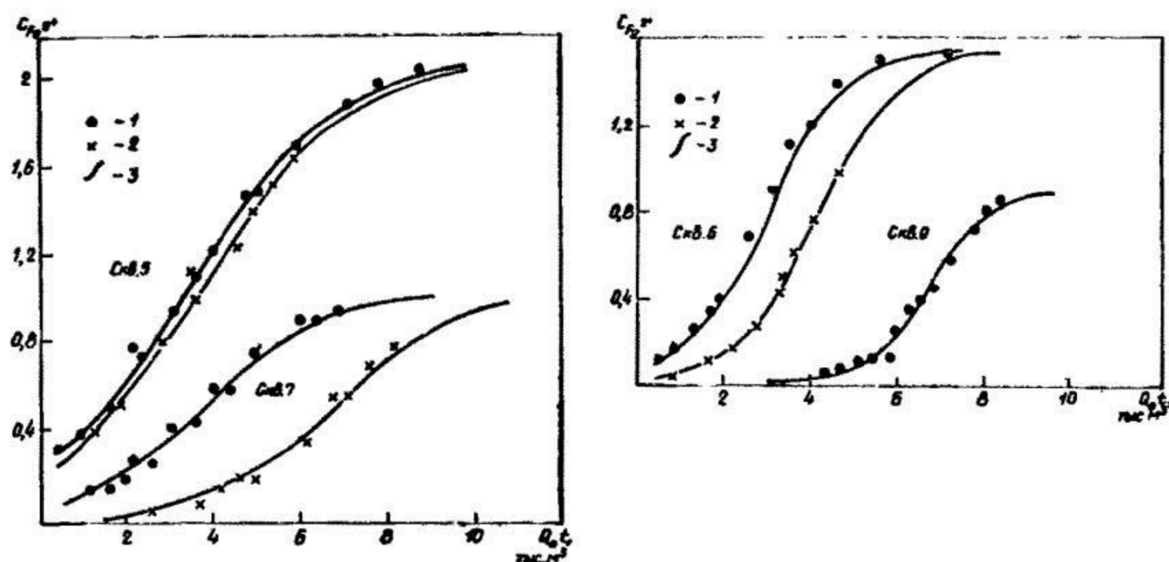
Рис. 21.9. Выходные кривые
