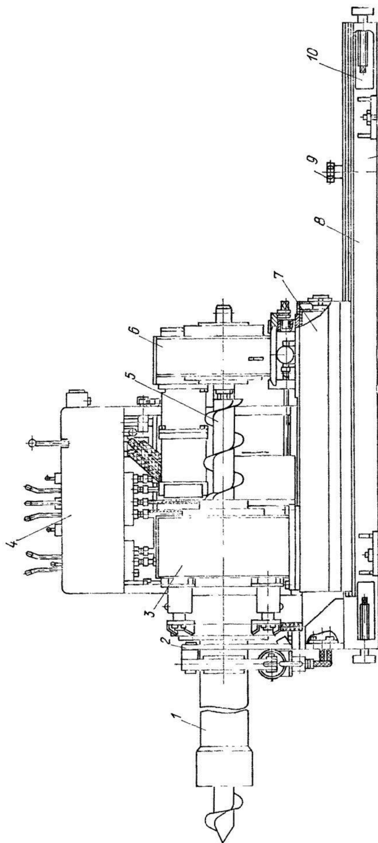
Рис. 10.1. Буровой агрегат установки лучевого бурения УЛБ-130
