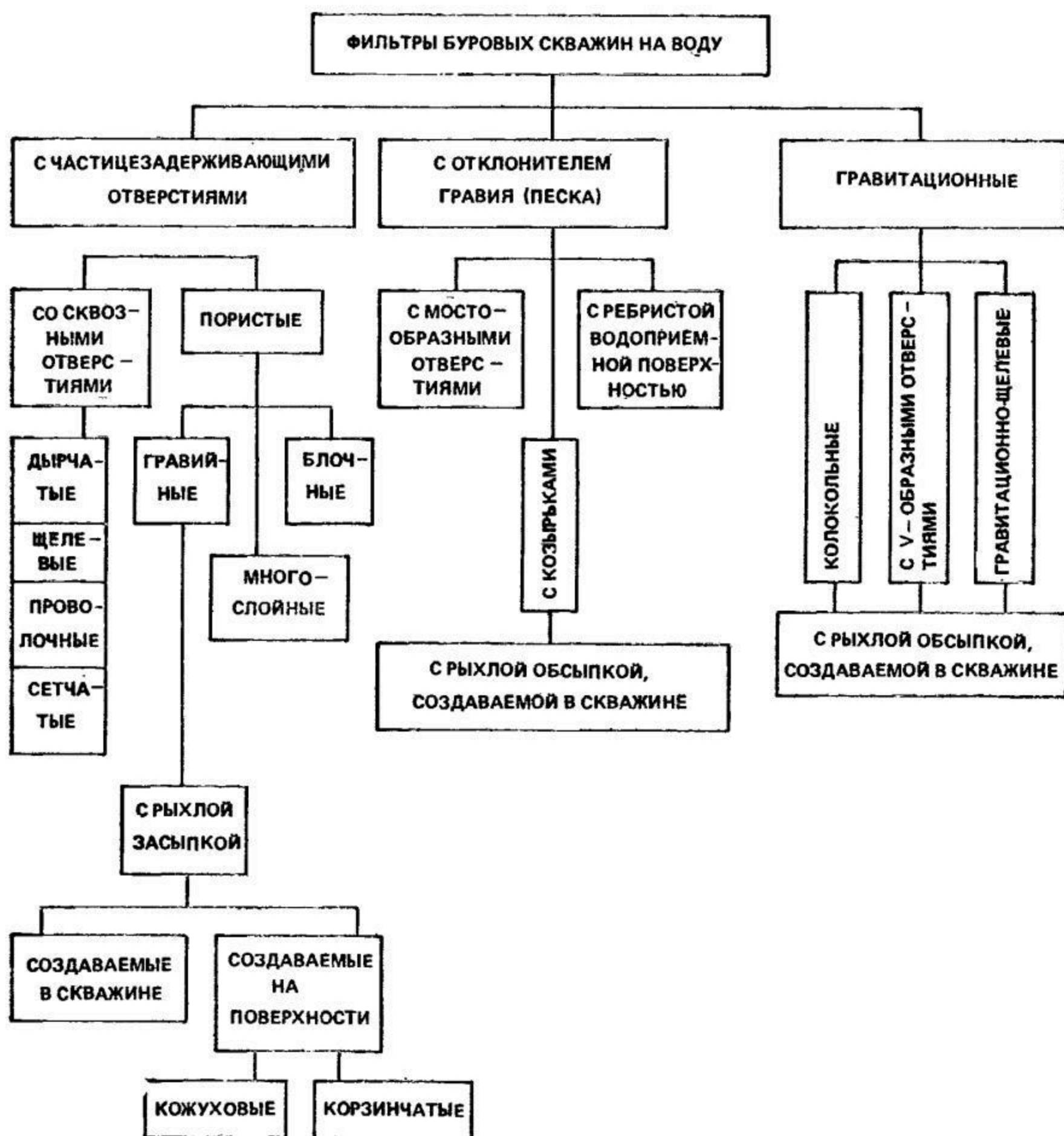
Рис. 4.1. Классификация фильтров водозаборных скважин
