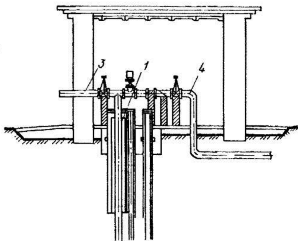
Рис. 13.13. Схема входного узла скважины двойного назначения
