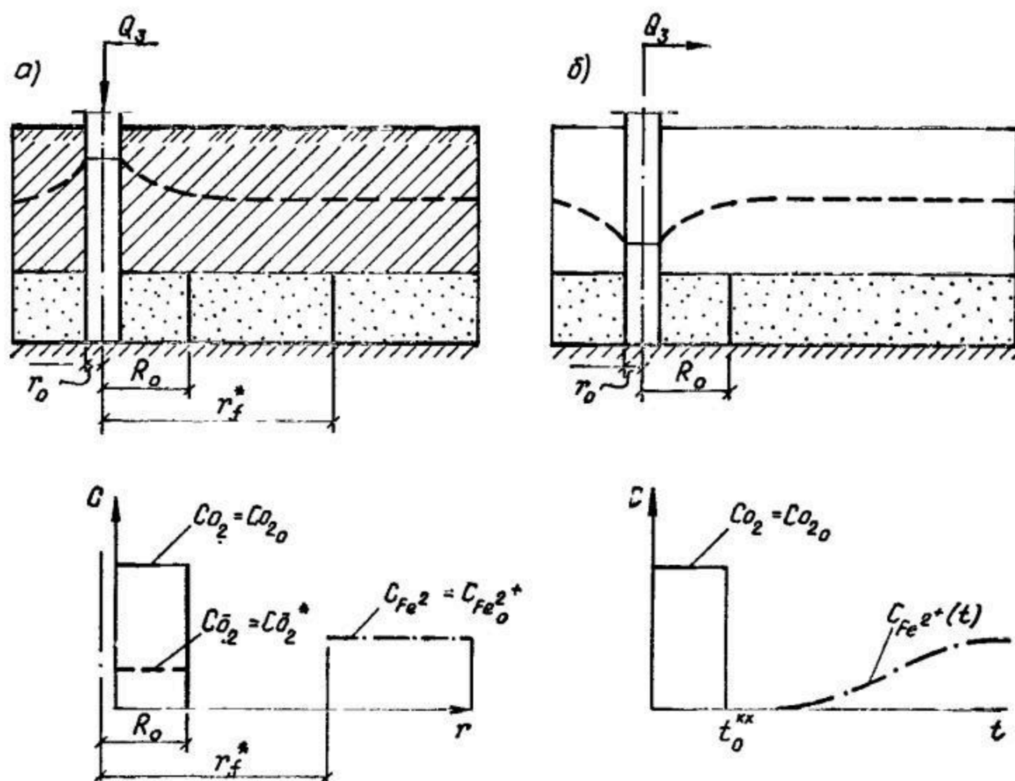
Рис. 21.4. Схема и графики гидродинамических и кинетических областей при работе установок обезжелезивания
