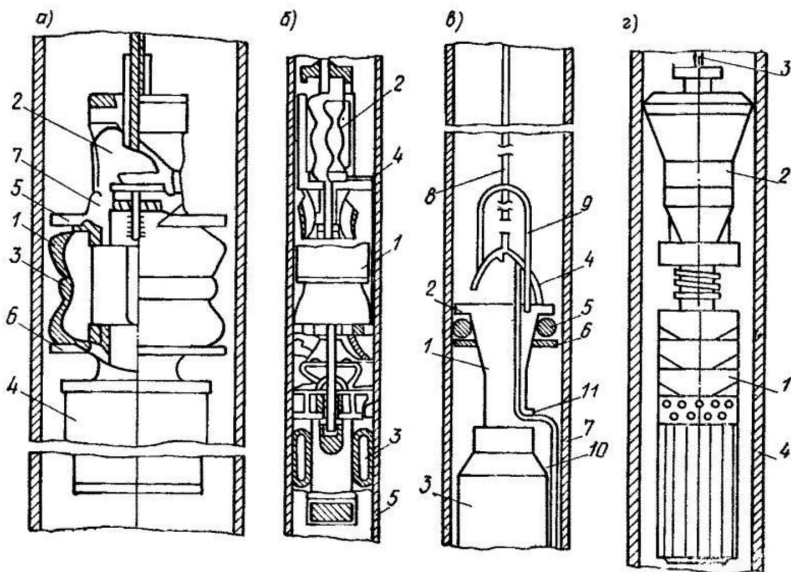
Рис. 5.6. Устройства беструбной подвески
