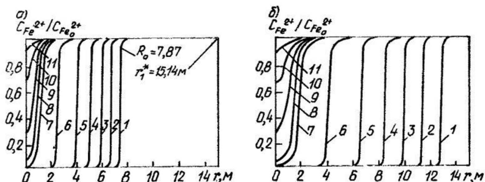
Рис. 21.7. Расчетные профили концентраций железа в зоне «зарядки»
