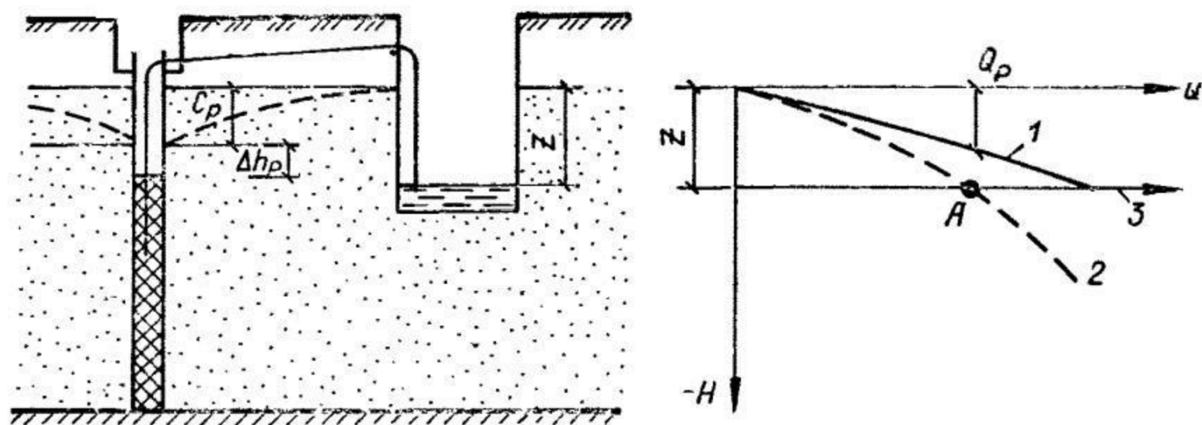
Рис. 7.4. Схема к расчету скважин при сифонном водоотборе
