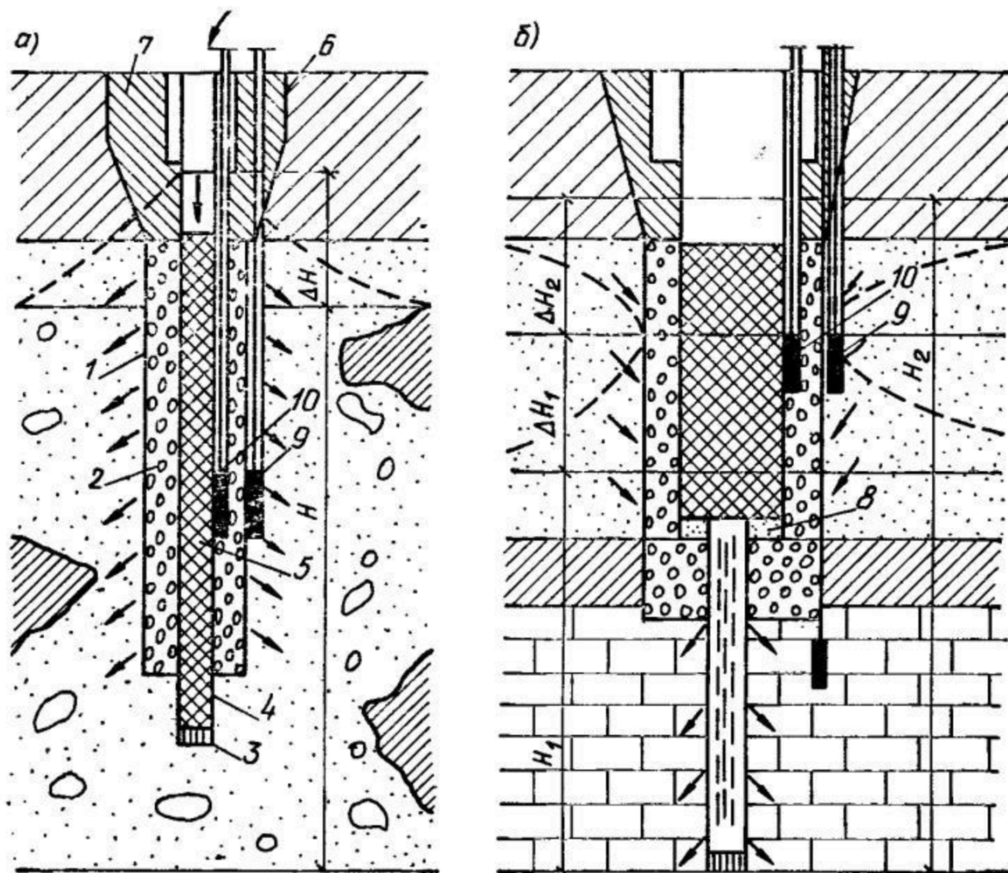
Рис. 13.10. Конструкции поглощающей и дренажно-поглощающей скважин a — поглощающая скважина; б — дренажно-поглощающая скважина: 1 — фильтровый каркас; 2 — обсадка; 3 — пробка; 4 — отстойник; 5 — эксплуатационная колонна; 6 — кондуктор; 7 — затрубная цементировка; 8 — сальник; 9 — наблюдательная скважина; 10 — затрубный пьезометр
