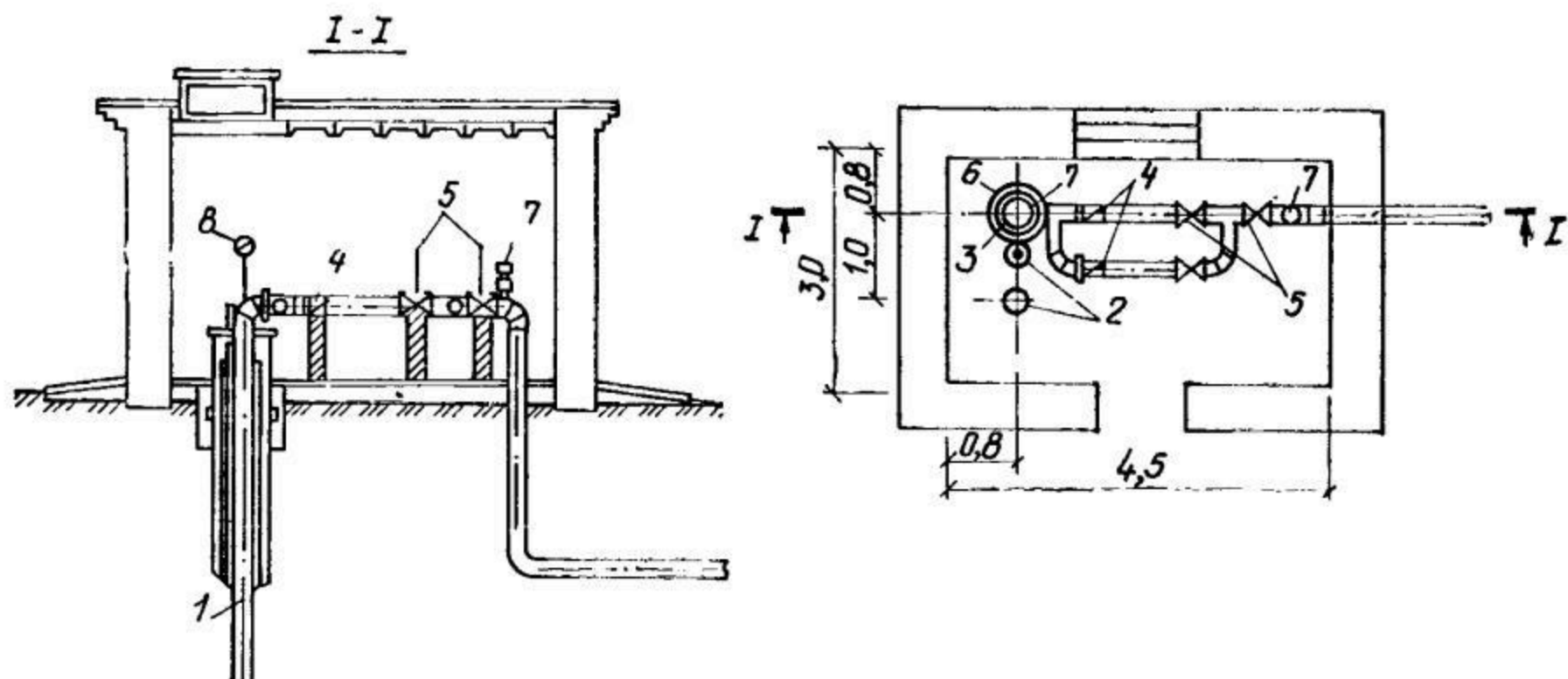
Рис. 13.11. Схема входного узла поглощающей скважины 1 — поглощающая скважина; 2 — наблюдательная скважина; 3 — пьезометр; 4 — водомер; 5 — задвижка; 6 — манометр; 7 — вантуз
