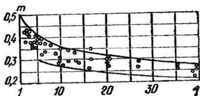
Рис. 4.5. Зависимость пористости породы от \eta
