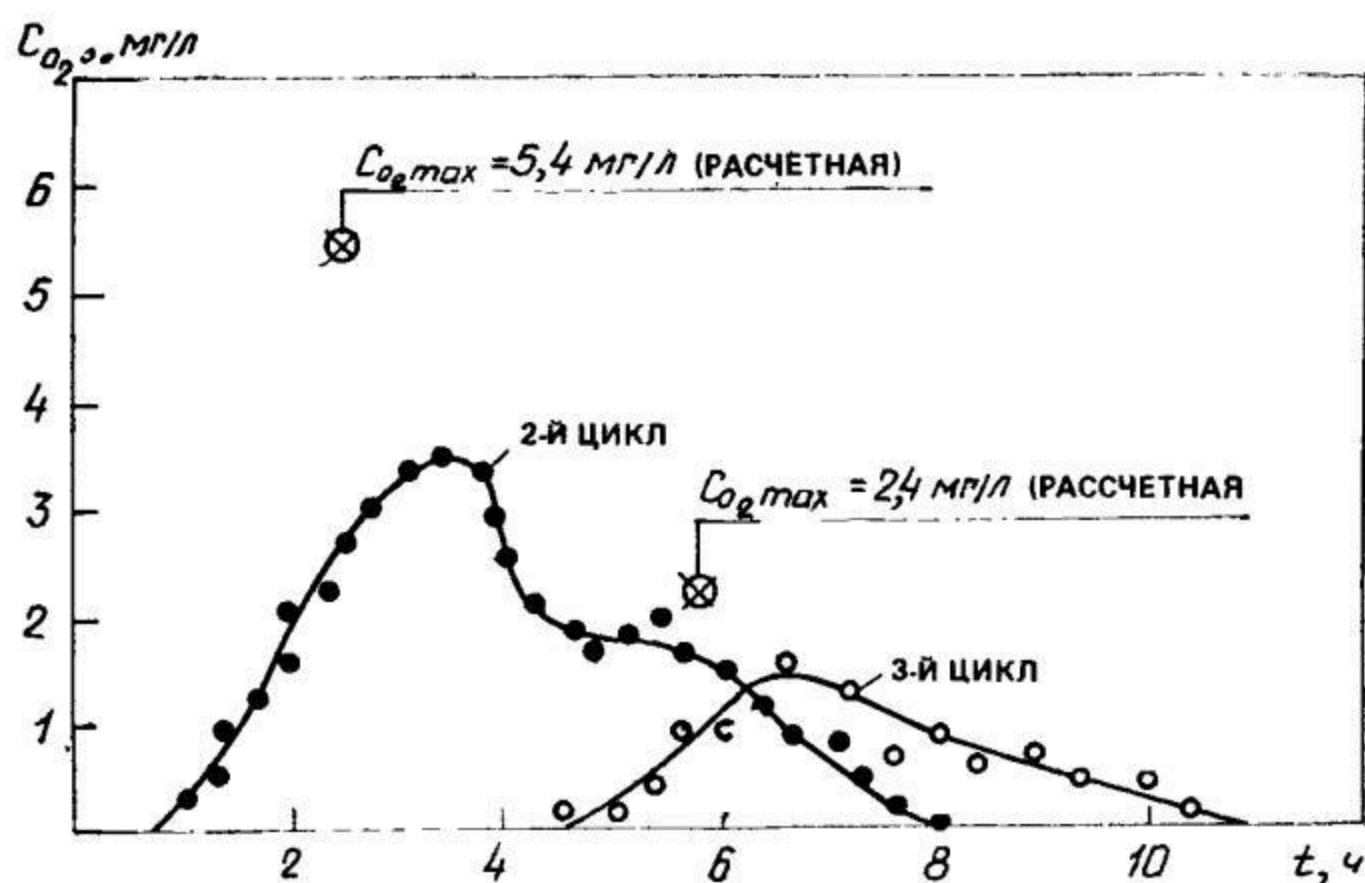
Рис. 21.19. Выходные кривые C_{O_2}(t)
