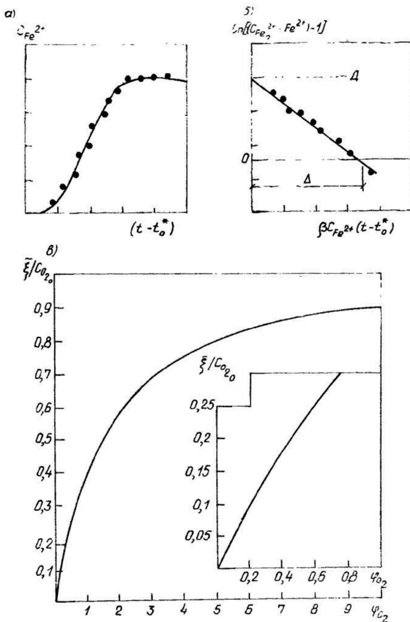
Рис. 21.8. Графоаналитический метод определения параметров процесса а — график выходной кривой C_{\text{Fe}^{2+}} ; б — вспомогательный график; в — график функции \bar{\xi}/C_{\text{O}_2} = f(\varphi_{\text{O}_2})
