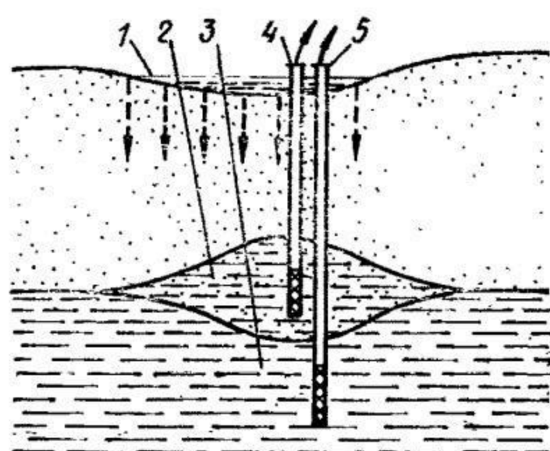
Рис. 13.2. Схема создания и использования линз пресных вод
