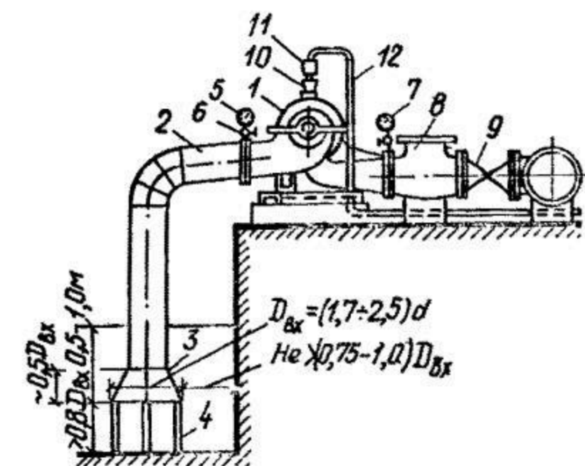
Рис. 5.4. Схема оборудования арматурой горизонтального центробежного насоса
