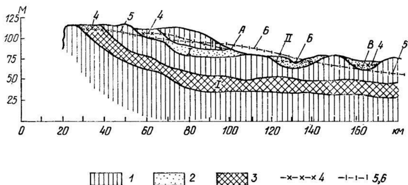
Рис. 1.1. Схема залегания подземных вод
