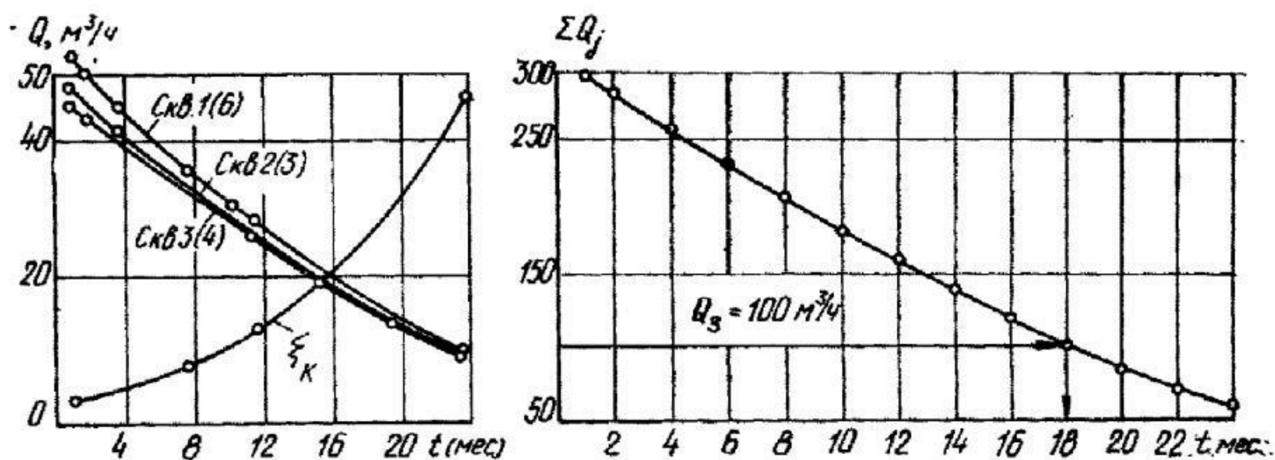
Рис. 7.7. Расчетные графики изменения во времени \xi_K(t) , Q_j(t) и \Sigma Q(t) при действии скважин в режиме S_j = \text{const}
