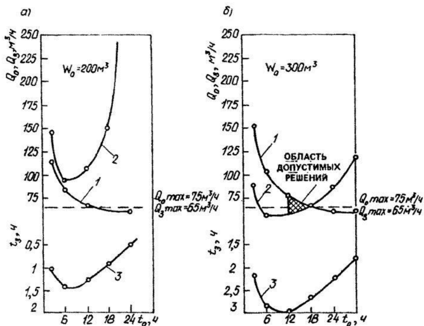
Рис. 21.20. Графоаналитический метод расчета установок на заданную производительность
