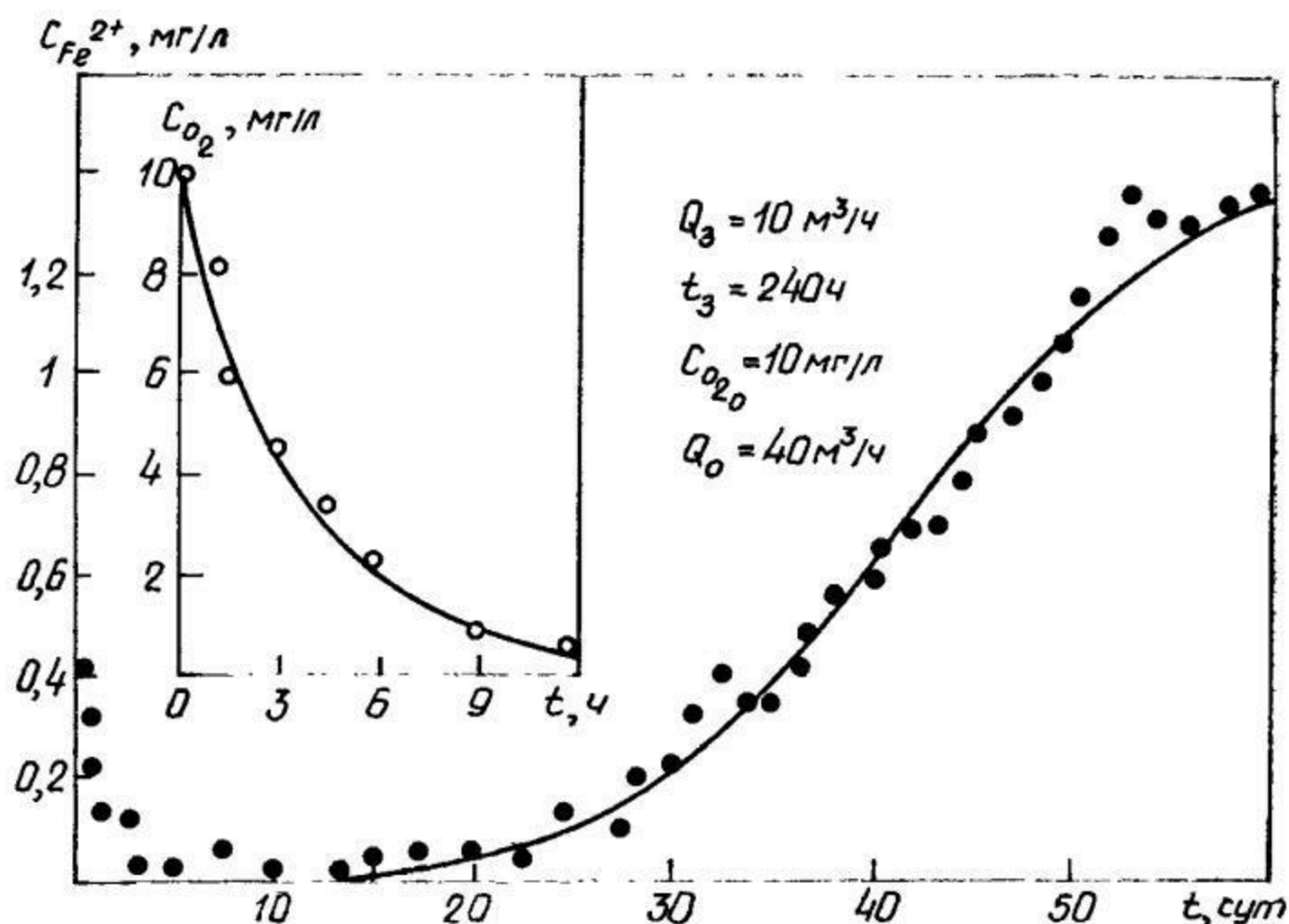
Рис. 21.18. Выходные кривые C_{O_2}(t) и C_{Fe^{2+}}(t)
