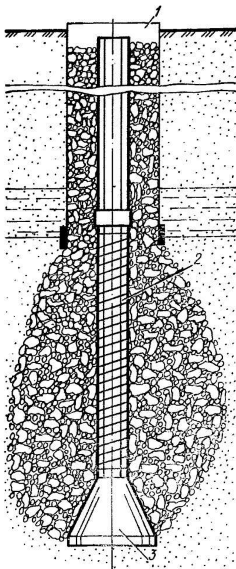
Рис. 14.7. Схема устройства гравийной обсыпки с применением башмака-конуса
