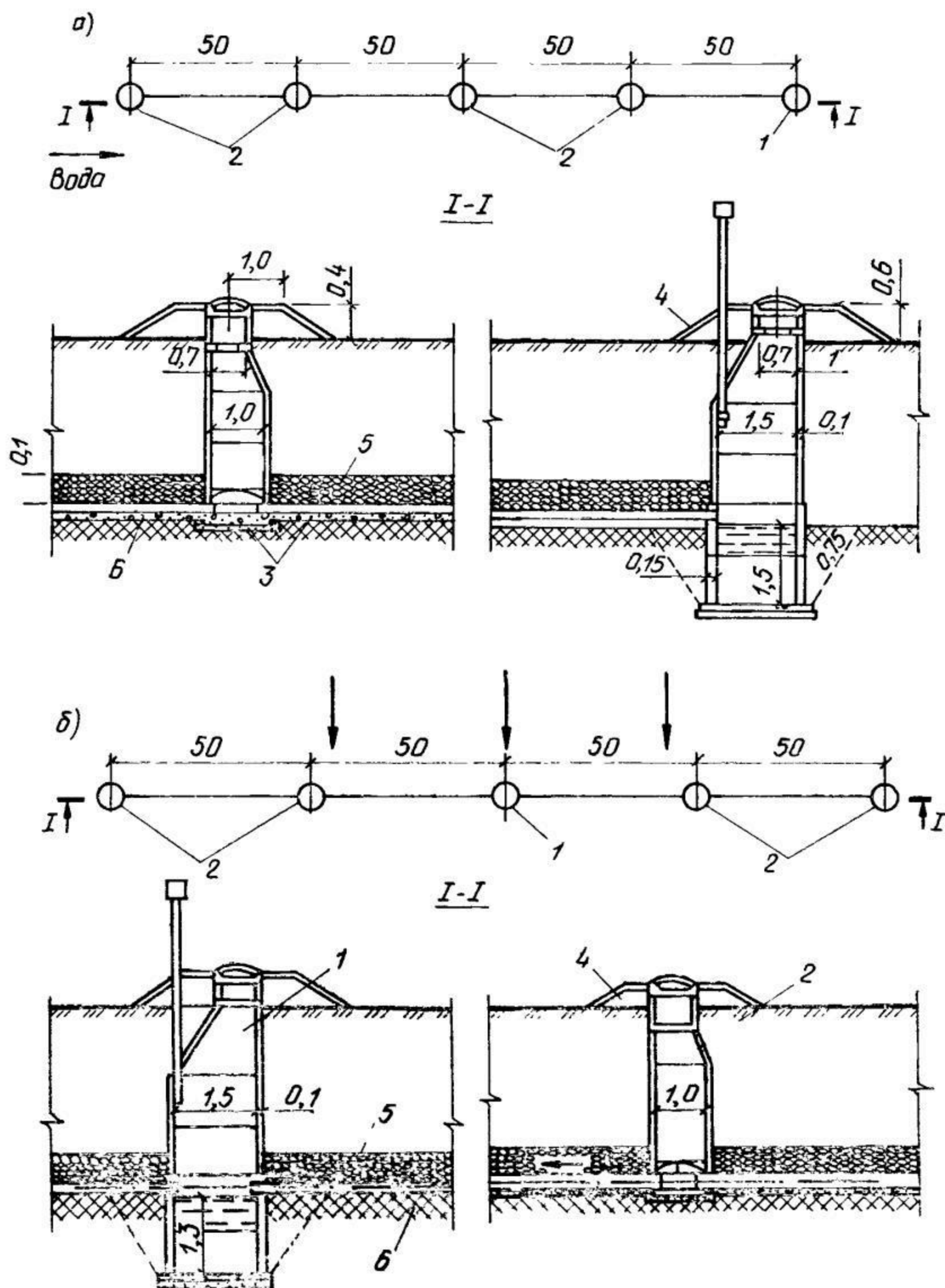
Рис. 9.2. Конструкции горизонтальных водозаборов трубчатого типа
