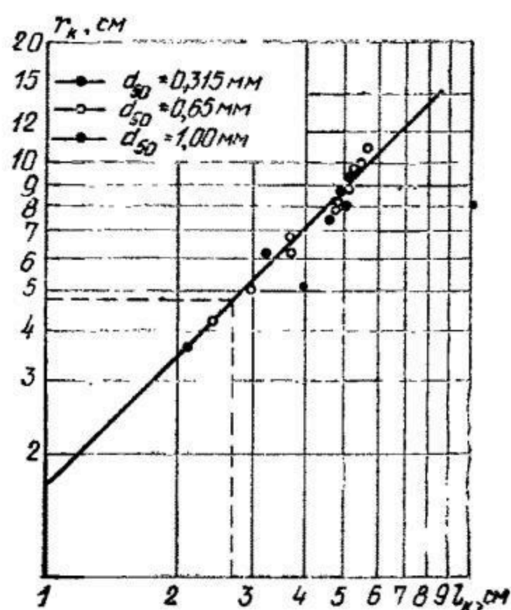
Рис. 14.3. Зависимость глубины каверны от ее радиуса
