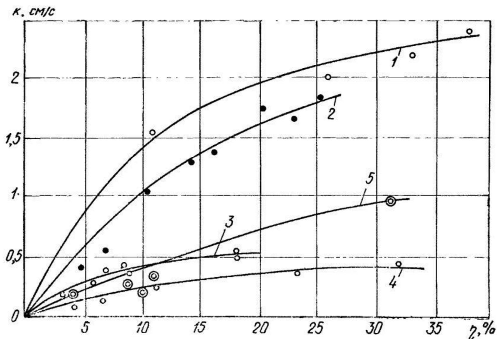
Рис. 4.2. Проницаемость фильтров различных типов в зависимости от скважности 1 — каркасно-стержневые; 2 — проволочные на трубчатом каркасе; 3 — с водоприемной поверхностью из штампованного листа; 4 — сетчатые фильтры с сетками галунного плетения; 5 — стеклопластиковые фильтры
