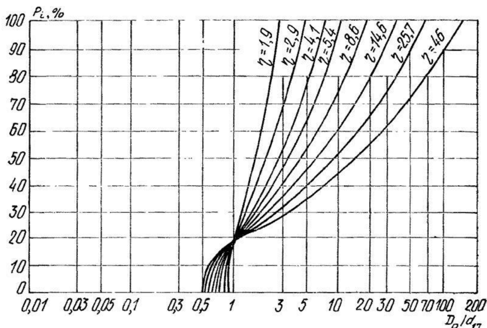
Рис. 4.9. Кривые зернового состава теоретически несuffозионных пород (по А. Н. Патрашеву)
