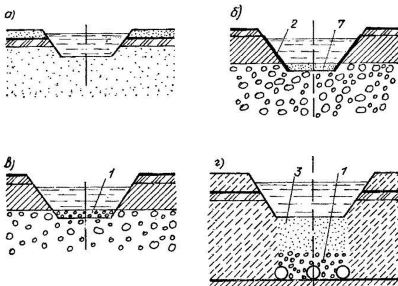
Рис. 13.5. Схемы инфильтрационных бассейнов
