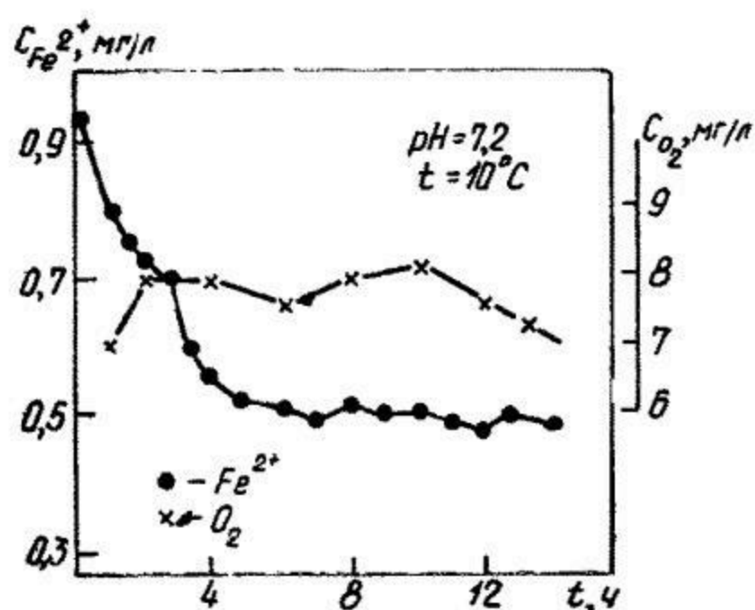
Рис. 21.10. Кривые окисления железа в свободном объеме
