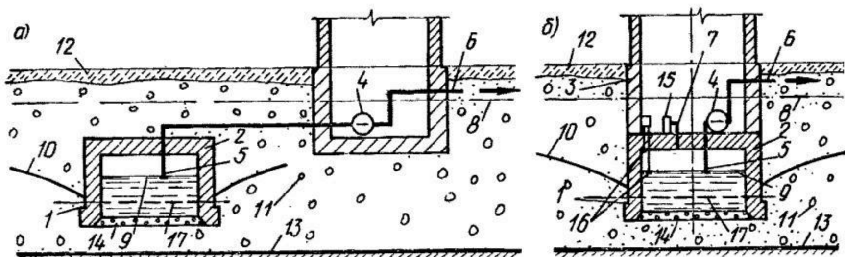
Рис. 12.1. Конструктивные схемы несовершенных шахтных колодцев
