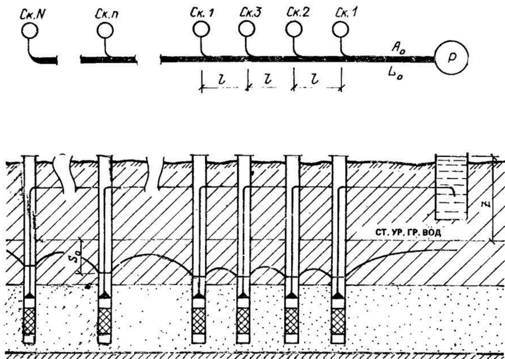
Рис. 7.5. Схема подсоединения скважин линейного ряда к сборному водоводу Q_n , при которых выполняется условие (7.8). После этого вычисляют s_n :
