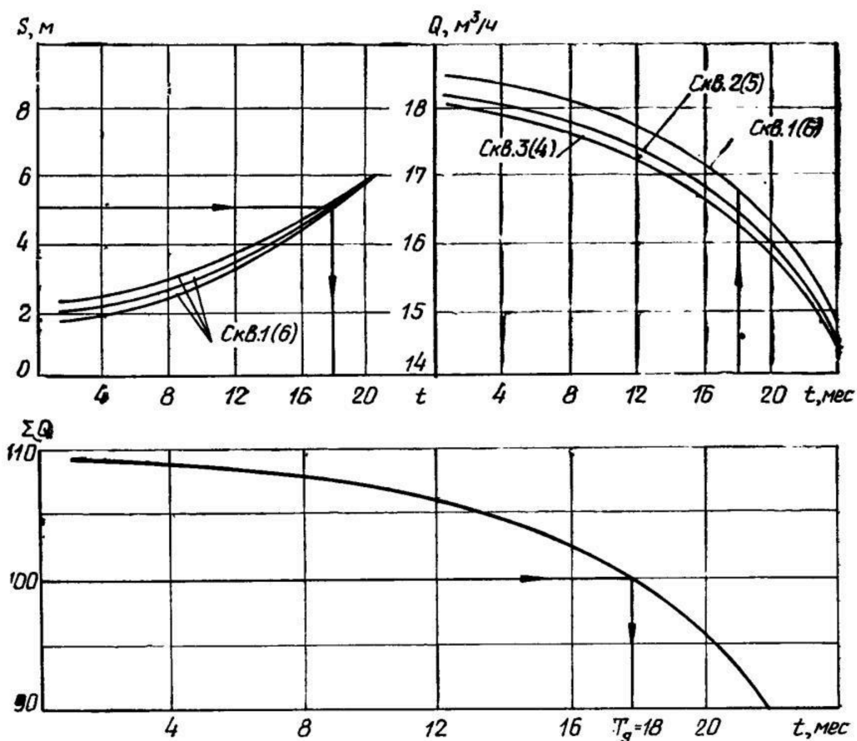
Рис. 7.9. Расчетные значения изменения S_i(t) , Q_i(t) и \Sigma Q_i(t) при насосной эксплуатации скважин
