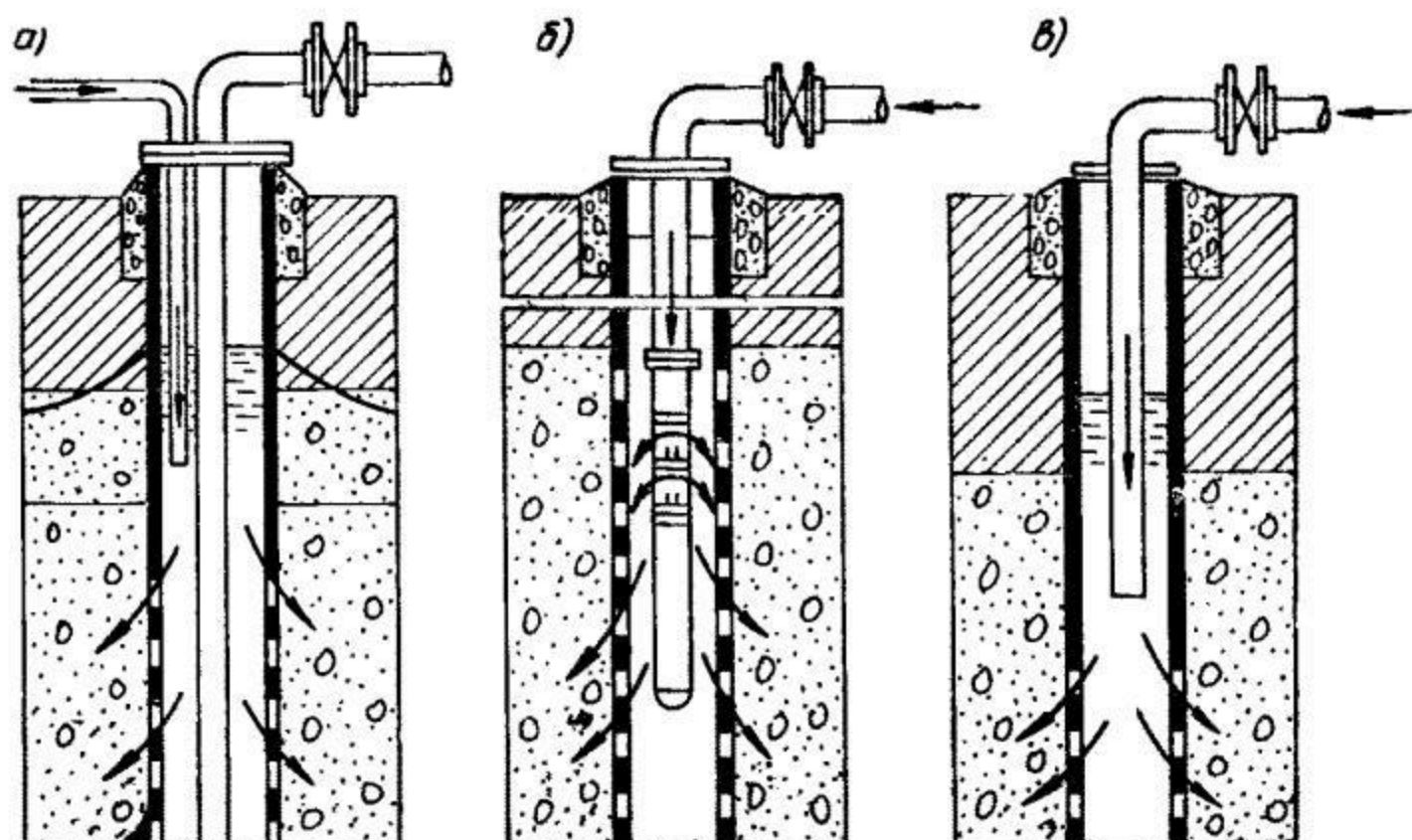
Рис. 13.12. Схемы подачи воды в скважины двойного назначения
