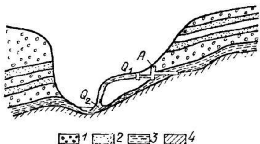
Рис. 11.1. Каптаж источника путем полного перехвата подземного потока
