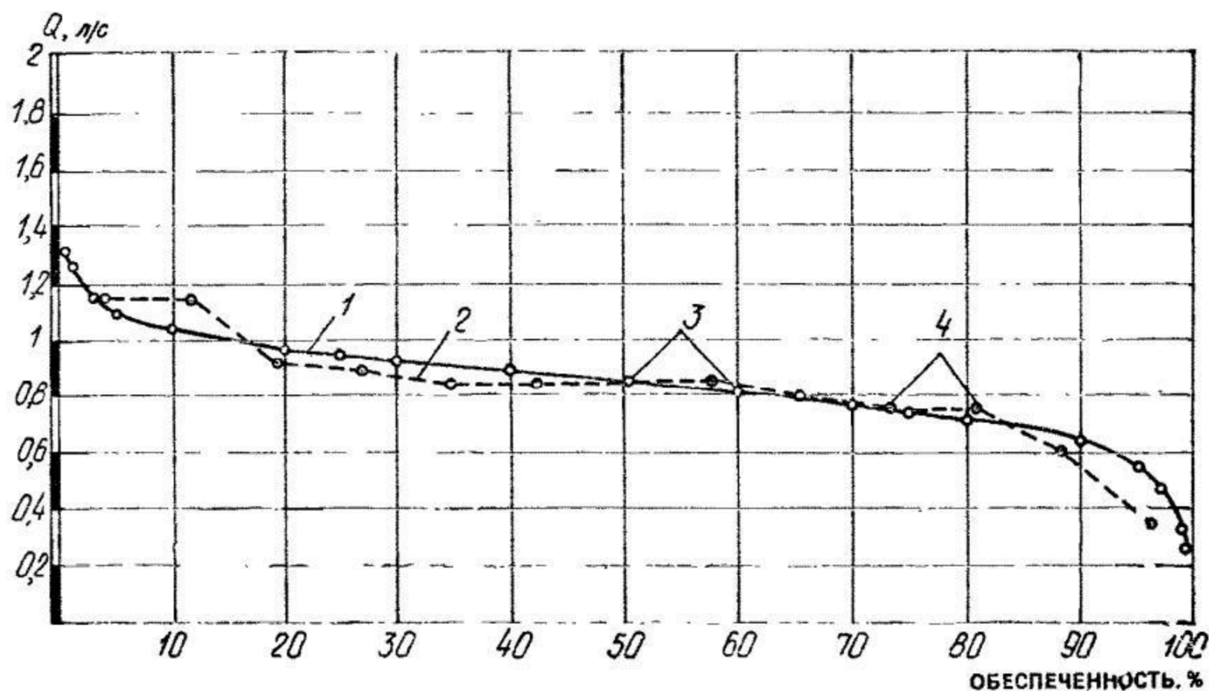
Рис. 11.5. Кривая обеспеченности минимальных дебитов источника
