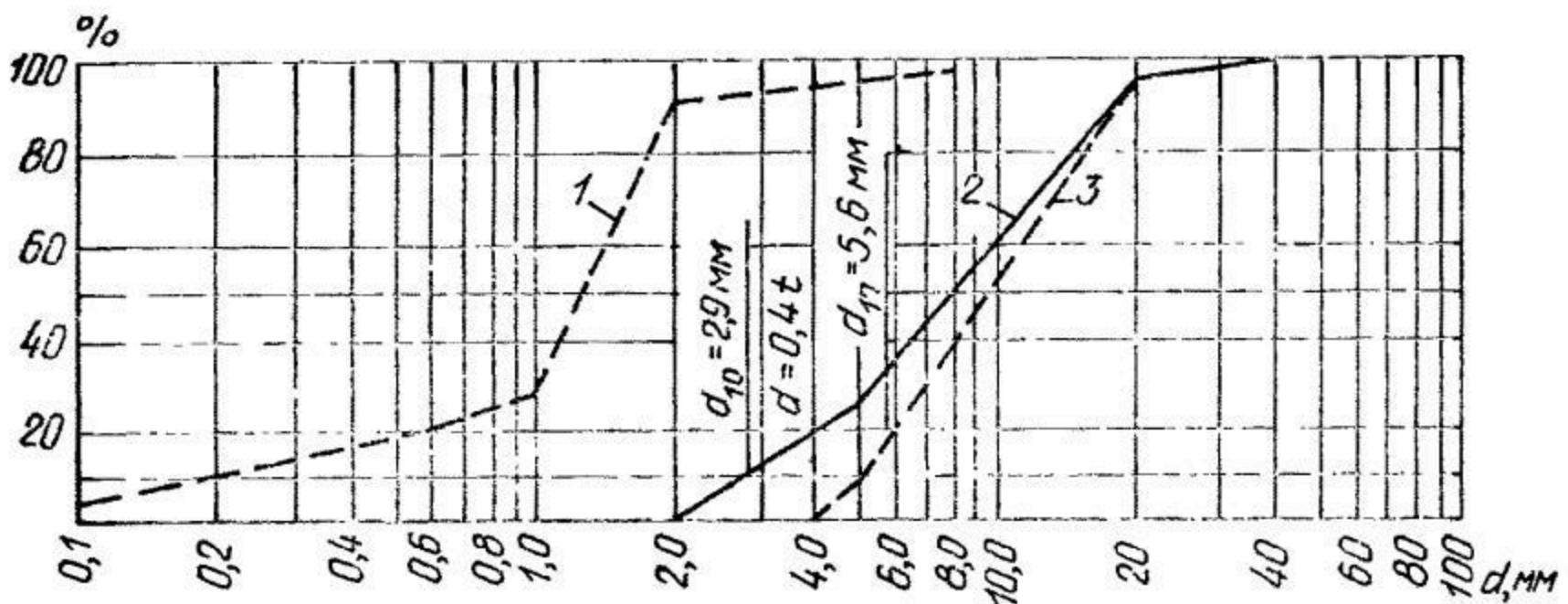
Рис. 9.11. Кривые гранулометрического состава
