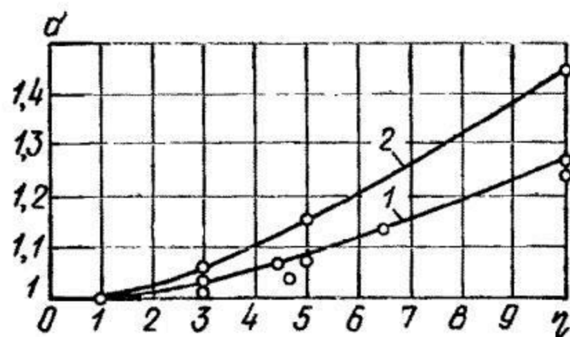
Рис. 4.8. Кривые зависимости поправочных коэффициентов для неоднородных обсыпок от \eta
