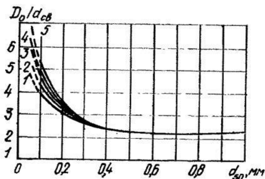
Рис. 4.7. Кривые зависимости допустимых межслойных коэффициентов от неоднородности породы
