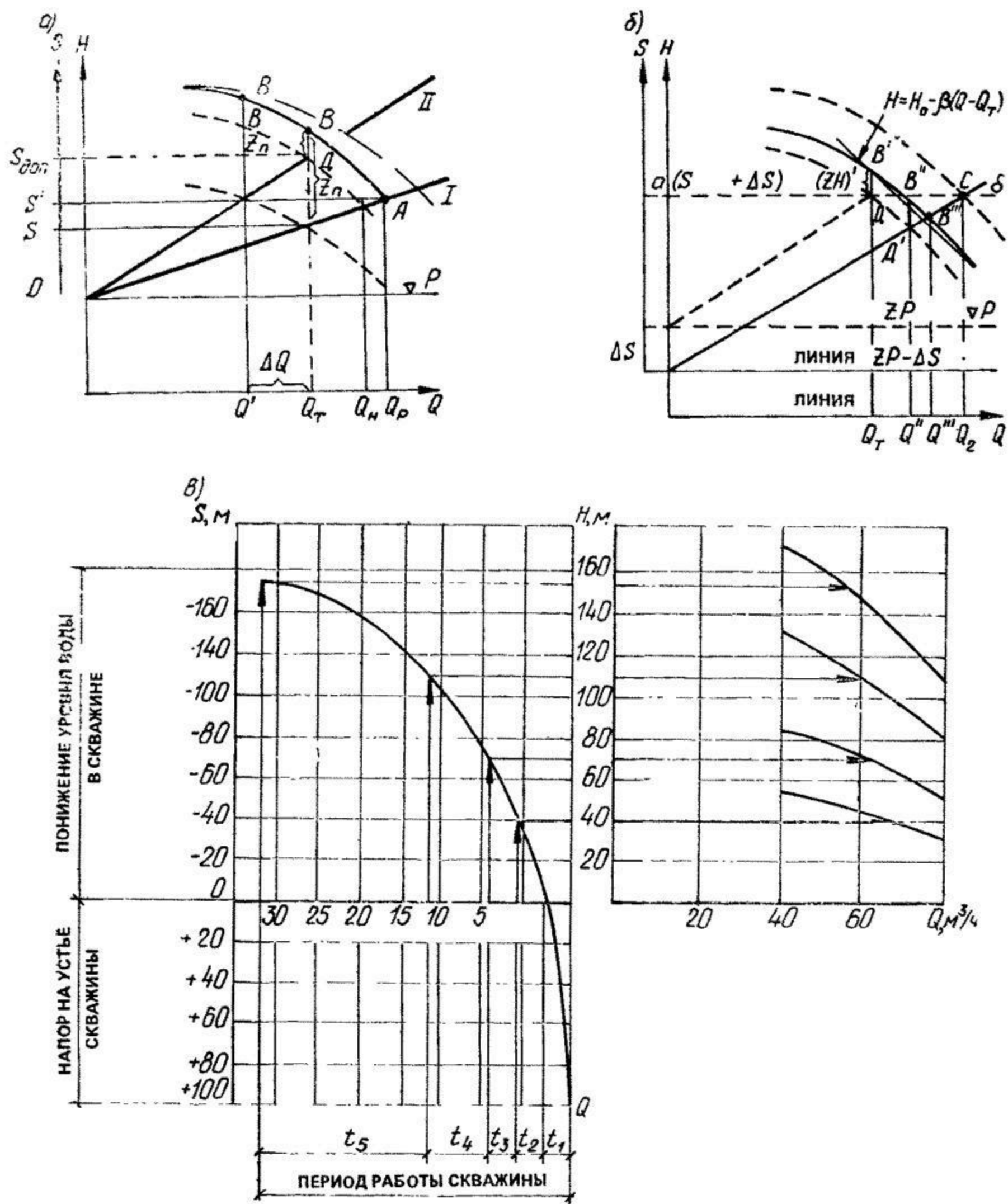
Рис. 7.3. Графоаналитический метод решения задач
