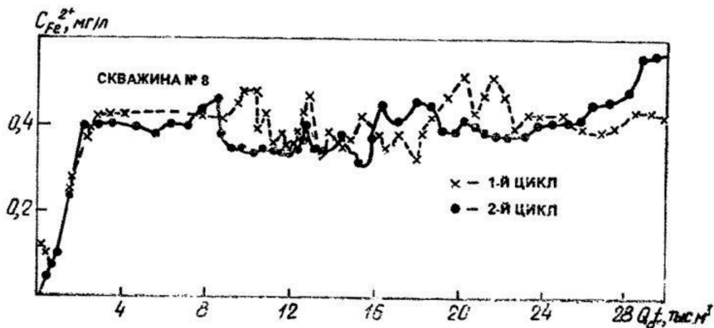
Рис. 21.15. Выходные кривые
