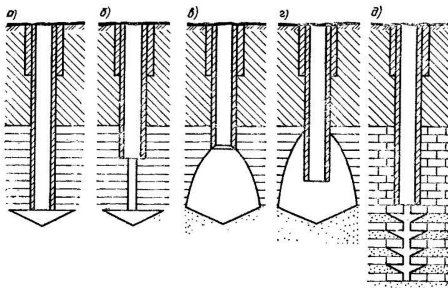
Рис. 14.1. Конструкции бесфильтровых скважин
