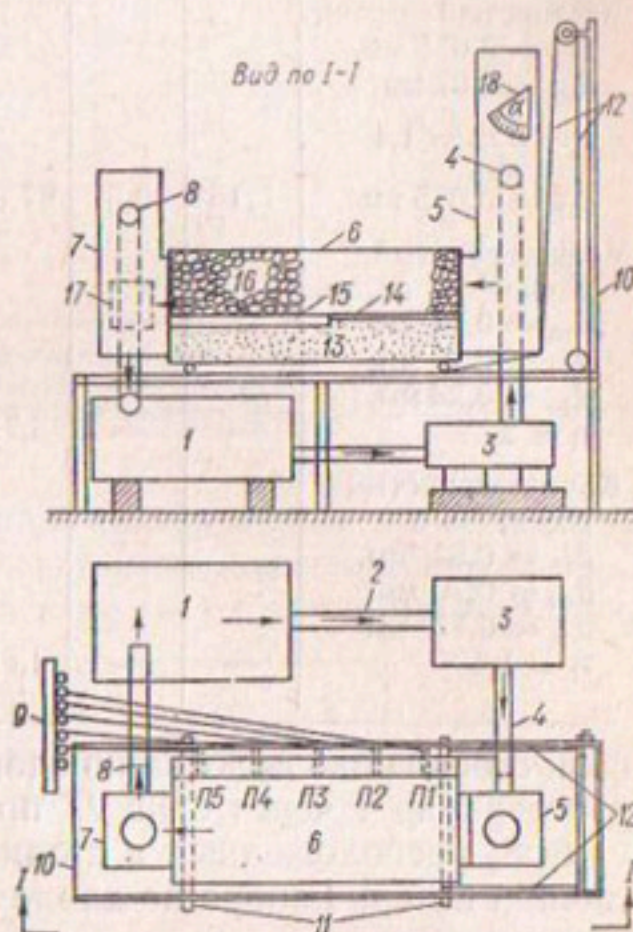
Рис. 92. Схема установки:
