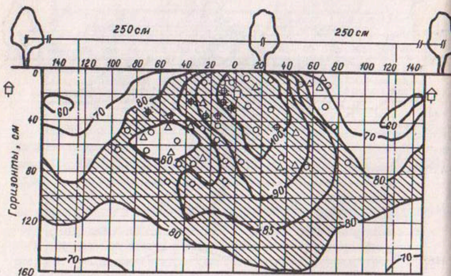
Рис.6. Карта распределения влажности почвы и корневой системы на варианте с расположением капельниц в пахотном слое почвы: ~ – гидроизоплеты, % от ШПВ; ○ – корни, диаметром 0–3 мм; △ – корни диаметром 3–10 мм; □ – корни диаметром 10–16 мм
