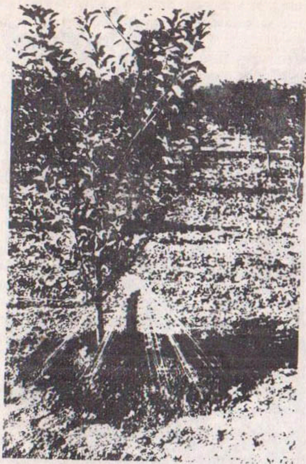
Рис. I. Капельно-импульсное орошение яблоневого сада с под- кroновым надпочвенным расположением капельниц (сов- хоз "Прут" Молдавской ССР)
