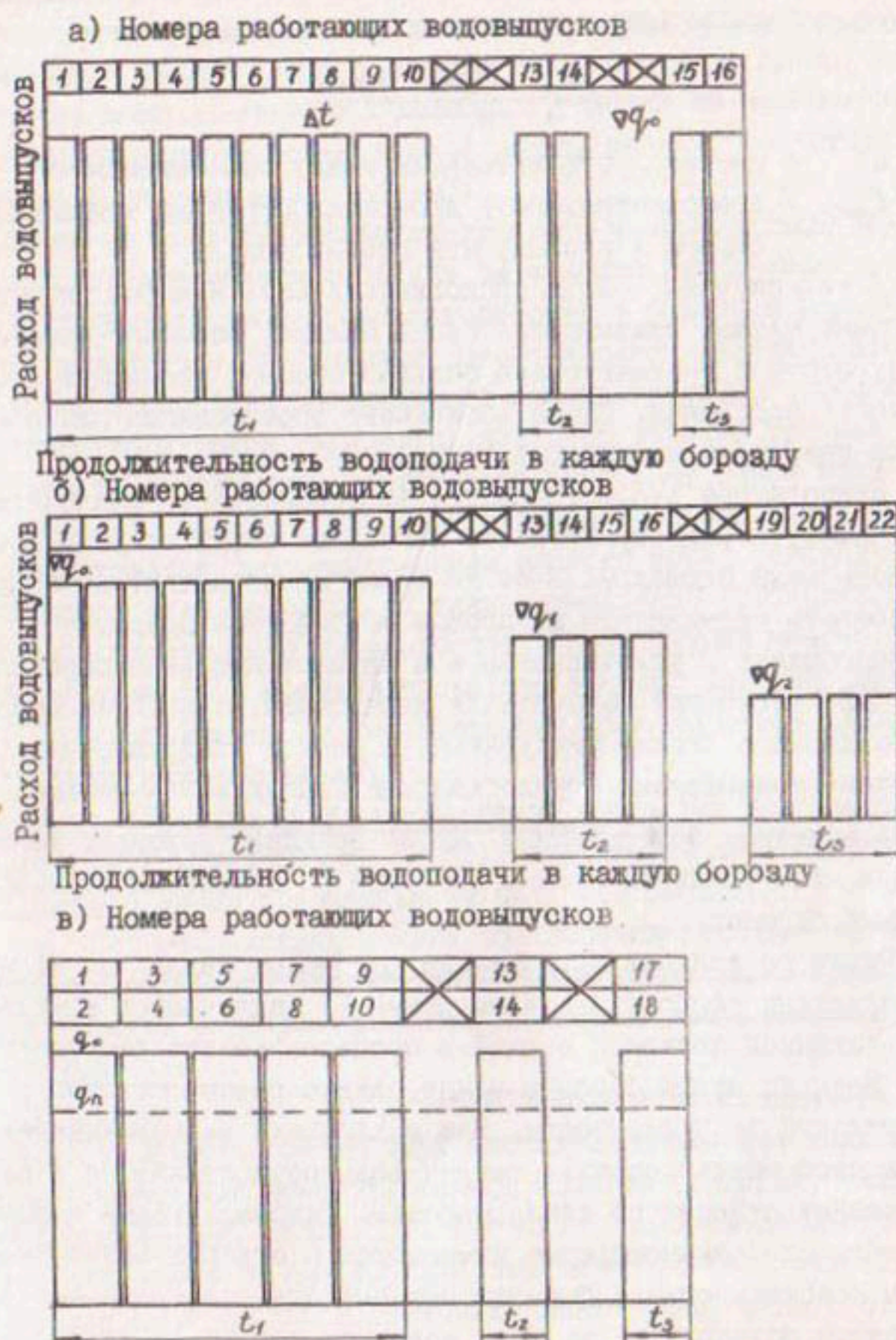
Рис.8. Схема возможного формирования цикличной водоподачи в борозду из водовыпусков самоходного плангового устройства при поливе прерывистой струей: а) постоянной по величине; б) уменьшающейся по величине; в) разной по величине для уплотненных и неуплотненных борозд
