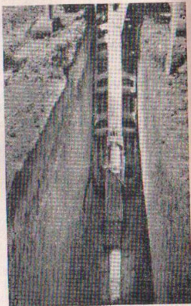
Рис. 110. Укладка глубокого дренажа из витых гибких поливинилхлоридных труб с фильтром из стеклохолста ВВГ дрепоукладчиком ДК-3,5: а — дрепоукладчик в работе; б — дрена в траншее.
