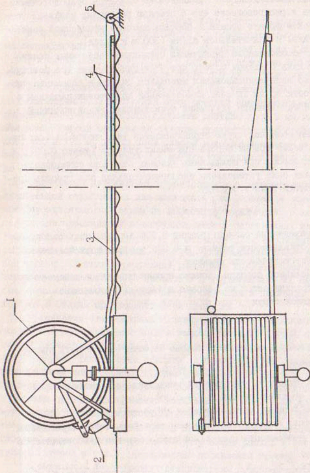
Рис. 6. Принципиальная схема самоходного шлангового устройства: 1 - барабан; 2 - шаговый гидродвигатель; 3 - полиэтиленовый шланг; 4 - регулируемые водовыпуски; 5 - разматывающее устройство
