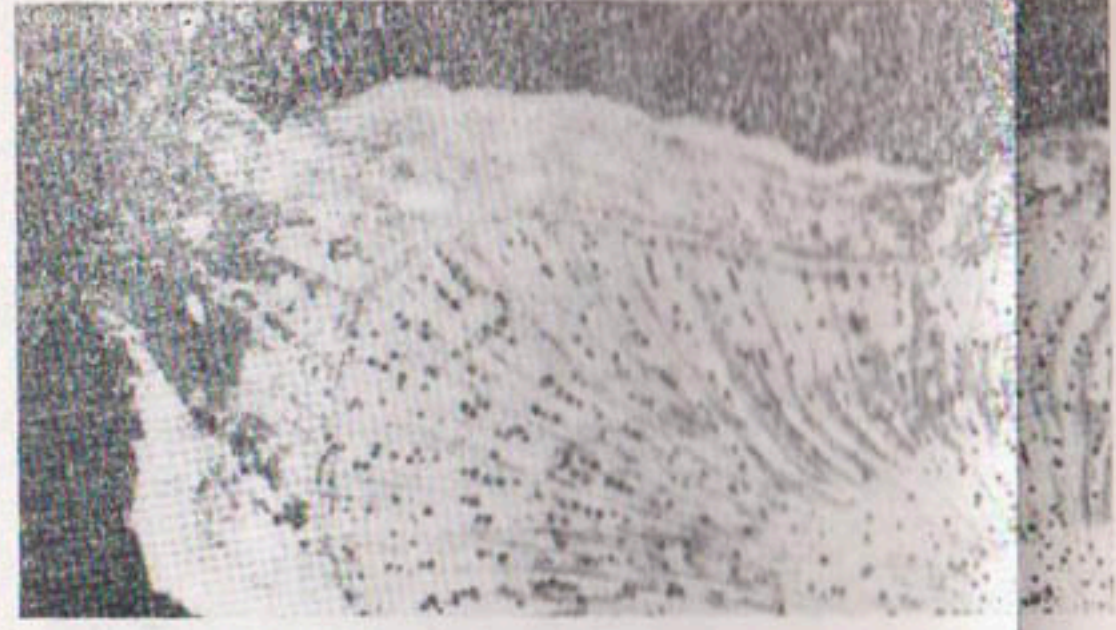
Рис. 5. Плотность 1,6 г/см 3 , влажность 40% от КВ.
