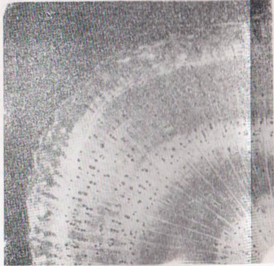
Рис. 4. Плотность 1,3 г/см 3 , влажность 80% от КВ.
