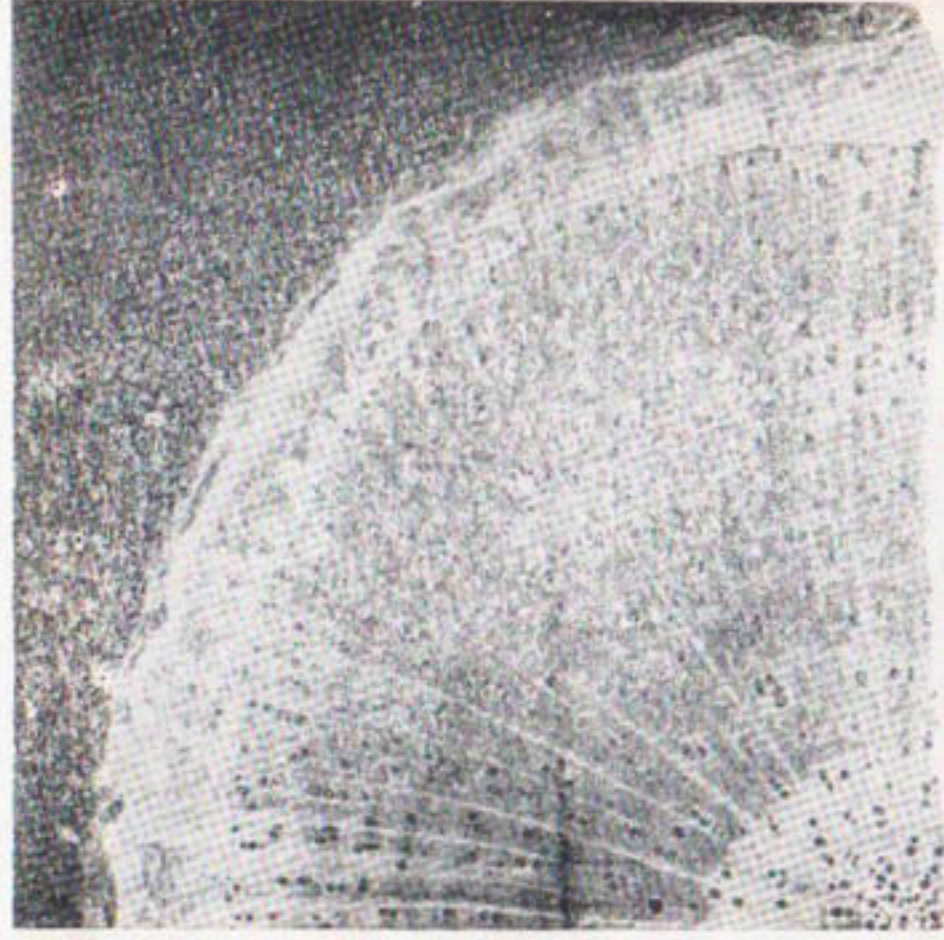
Рис. 3. Плотность 1,3 г/см 3 , влажность 60% от КВ.
