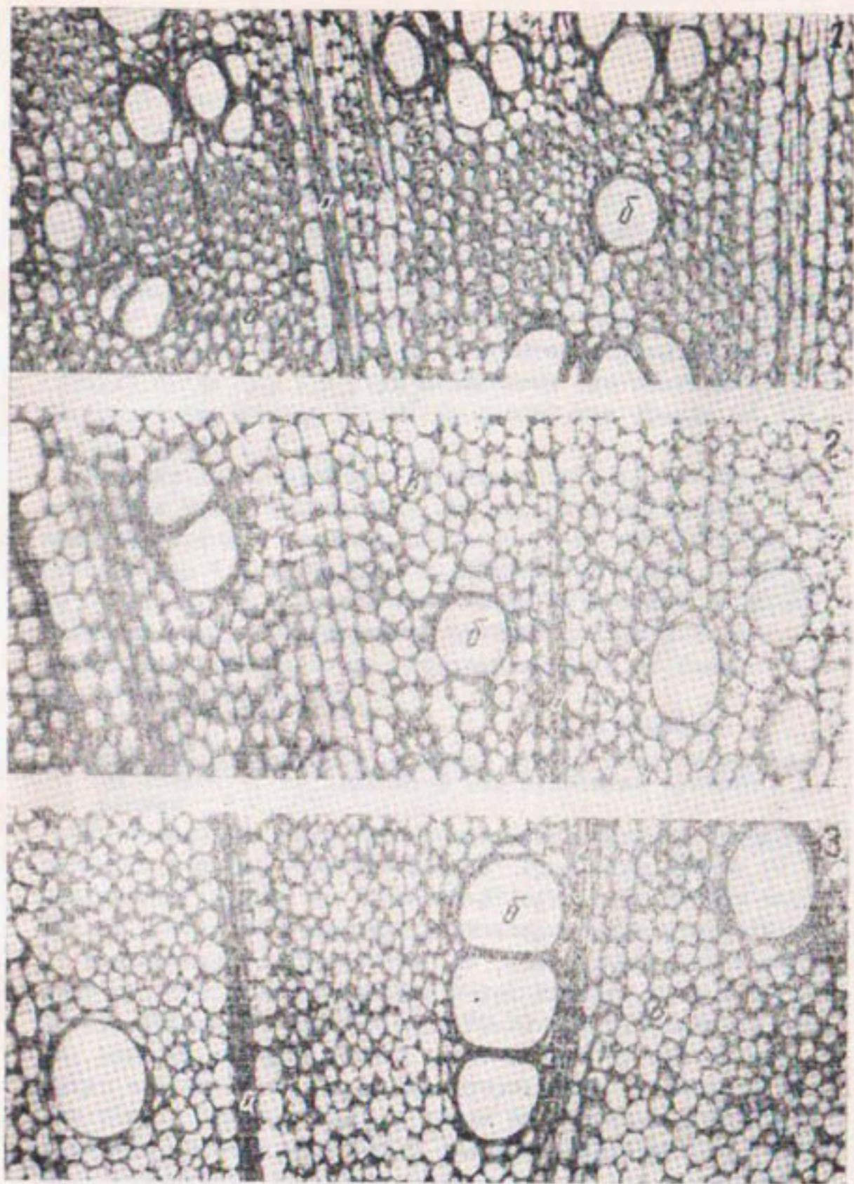
Рис. 8. Влияние плотности и влажности почвы на анатомическое строение корня хлопчатника (плотность 1,3 \text{ г/см}^3 : 1 — влажность 40\% от КВ; 2 — влажность 60\% от КВ; 3 — влажность 80\% от КВ. а—радиальный луч; б—проводящий сосуд; в—древесная паренхима (либриформ).
