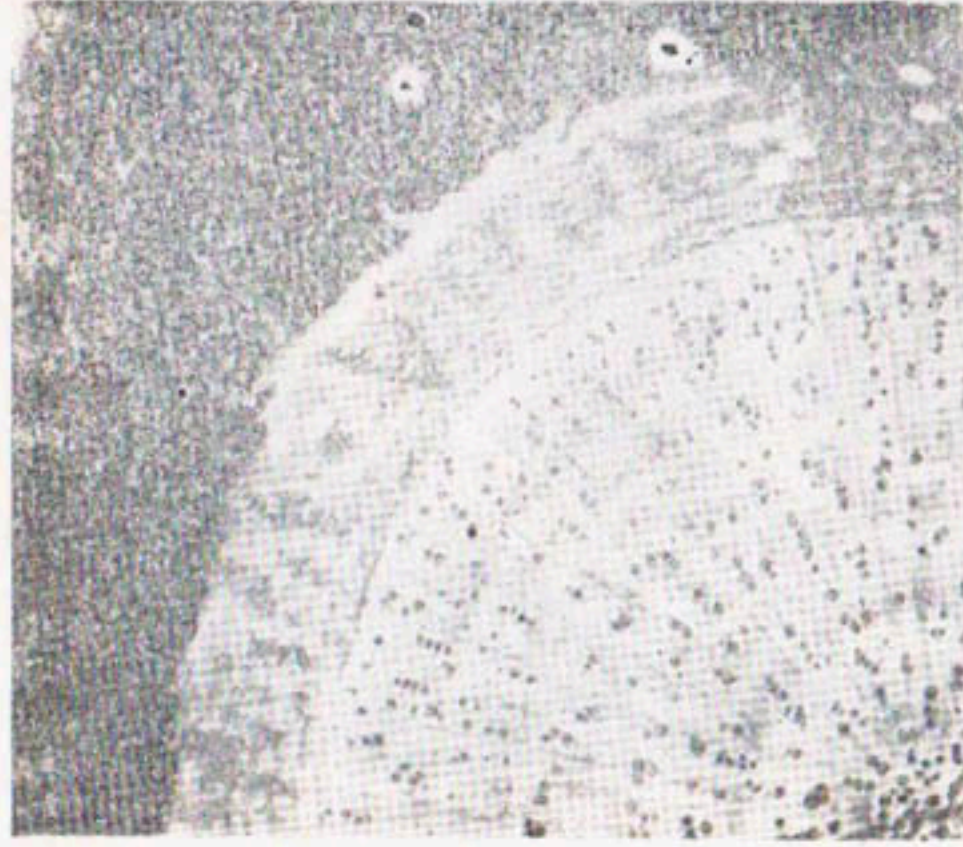
Рис. 2. Анатомическое строение корня хлопчатника (поперечный срез) при плотности 1,3 г/см 3 и влажности 40% от КВ.
