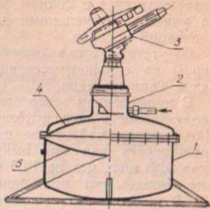
Рис. 2. Импульсный дождеватель «Колонна-15»:
