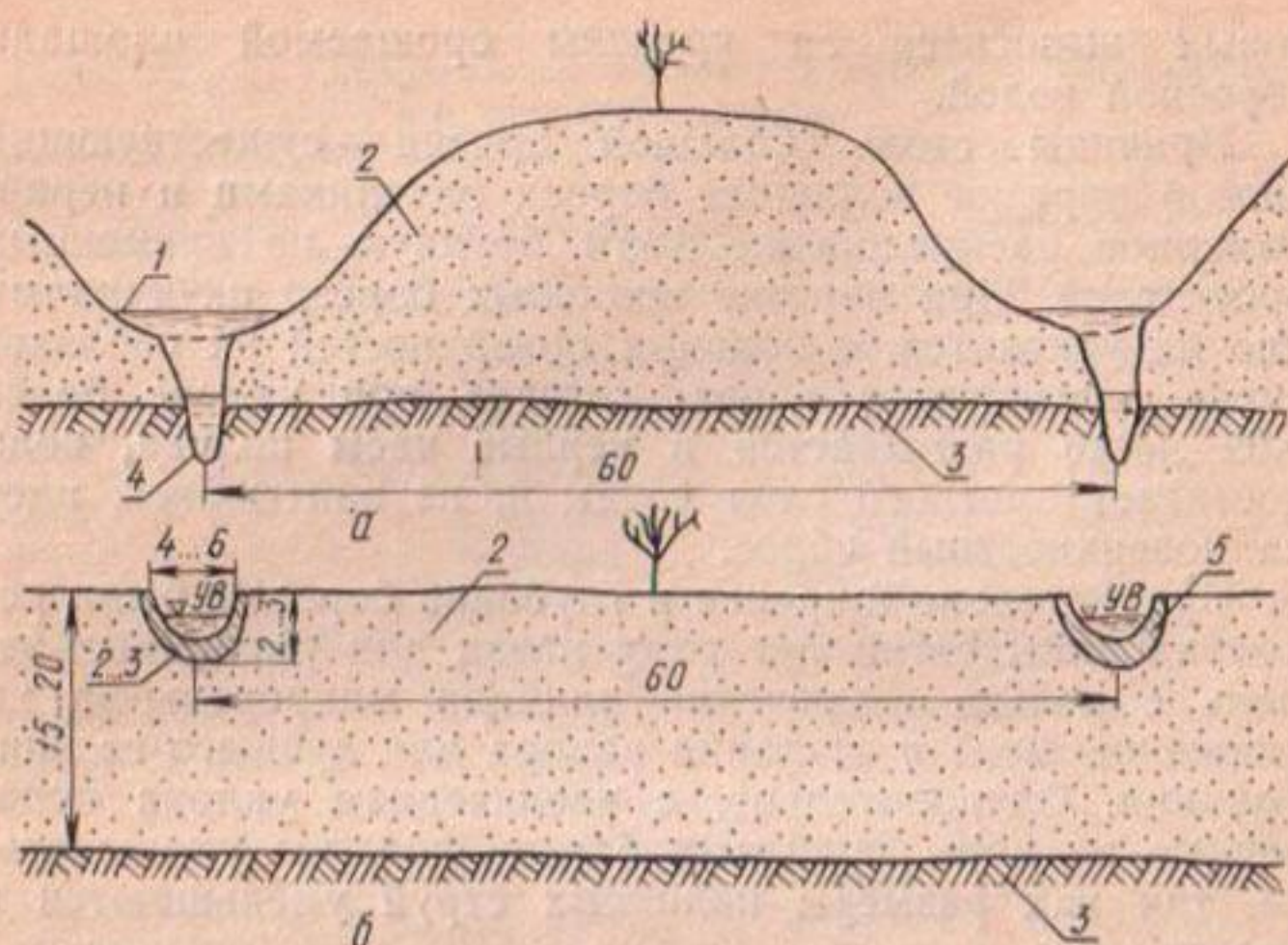
Рис. 2. Расположение и размеры поливных борозд, выполненных обычными окучками и катками-бороздоделателями (микроборозды): а — обычные поливные борозды; б — микроборозды; 1 — первоначальный уровень воды; 2 — пахотный слой; 3 — подпахотный слой; 4 — дно борозды после размыва; 5 — уплотненный слой (расстояния в метрах).
