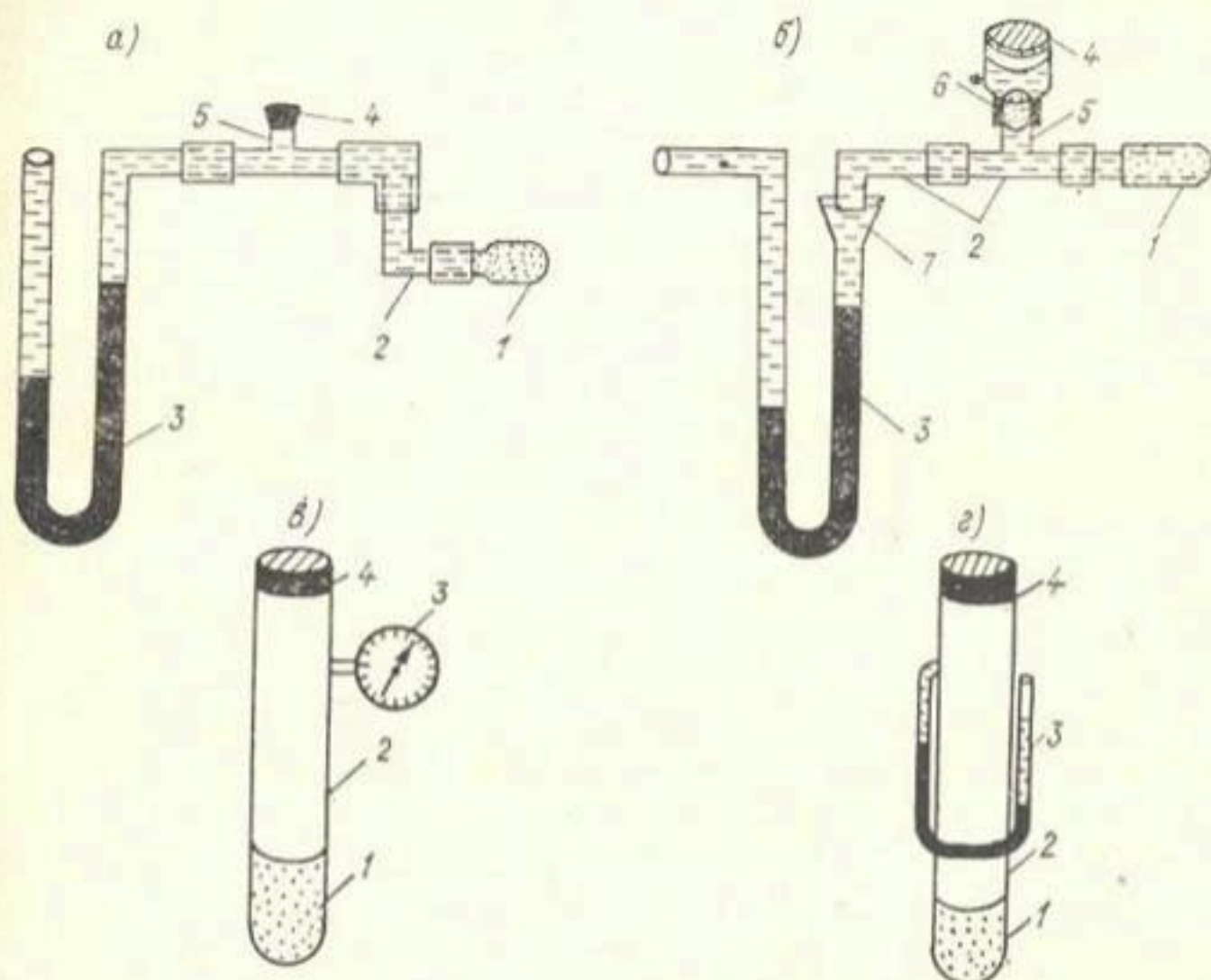
Рис. 2.1. Схемы тензиометров.
