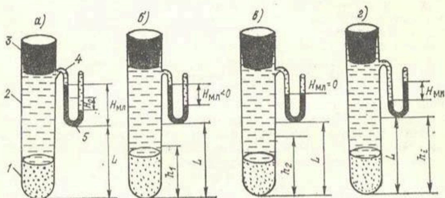
Рис. 2.8. Схема установки тензиометров в грунтовые воды и соотношение манометрических разностей ( H_{мл} и H_{мв} ) и гидростатической поправки ( H_0 ). 1 — датчик, 2 — корпус, 3 — пробка, 4 — ртутный манометр, 5 — поверхность почвы; L — глубина установки тензиометра в почву; h_1 , h_2 , h_i — УГВ от поверхности почвы.
