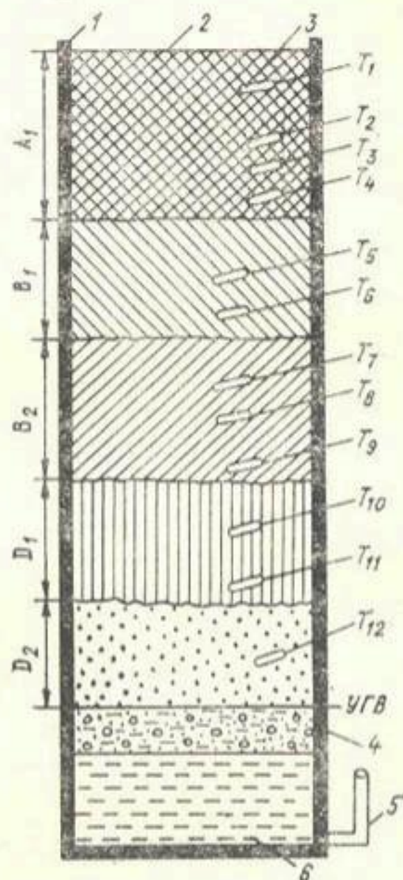
Рис. 4.1. Схема почвенной колонны. 1 — корпус, 2 — почва, 3 — датчик тензиометра, 4 — фильтр, 5 — пьезометр, 6 — грунтовые воды; T_1 — T_{12} — тензиометры.
