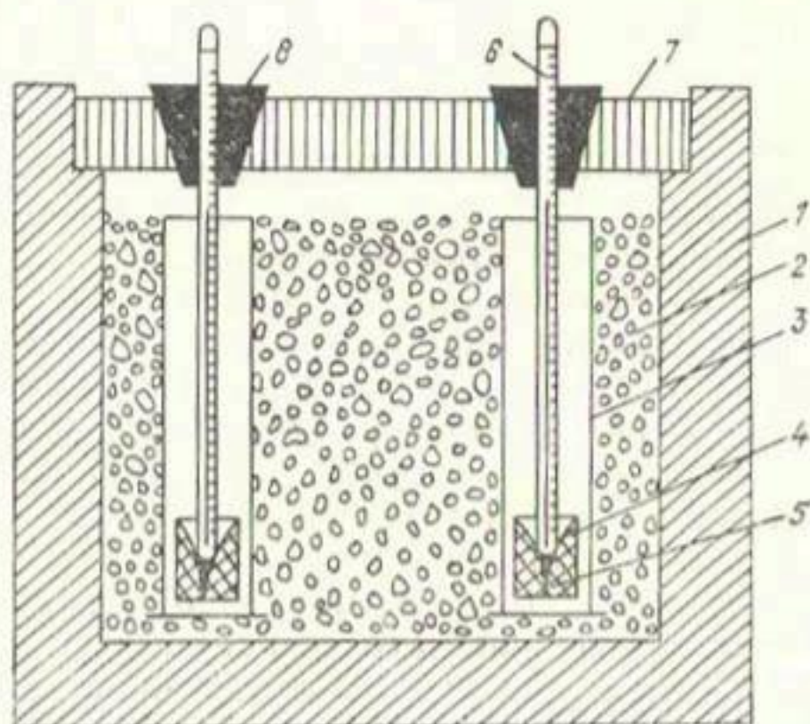
Рис. 2.10. Схема криоскопа.
