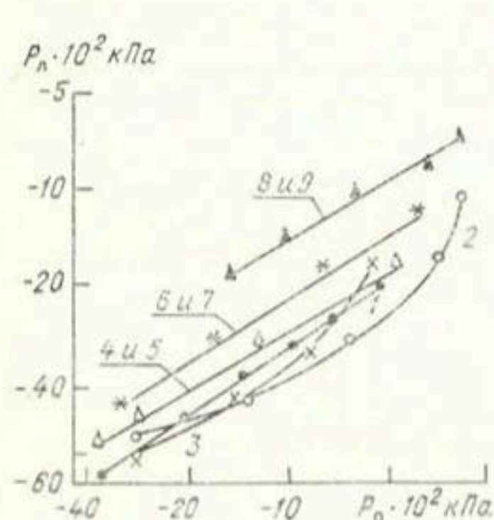
Рис. 5.1. Зависимость потенциала влаги в листьях различных растений ( P_{\text{л}} ) от потенциала почвенной влаги ( P_{\text{п}} ).
