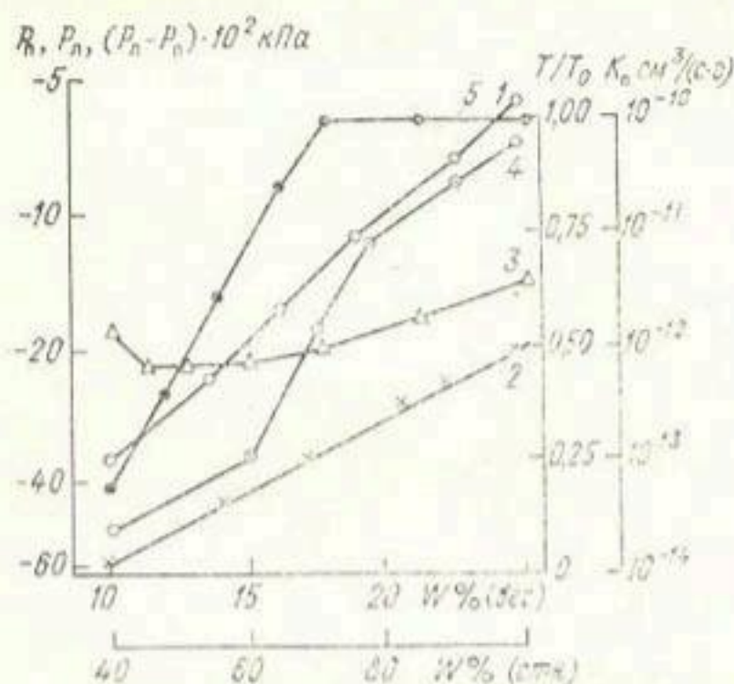
Рис. 5.4. Зависимость потенциала влаги в почве ( P_n ) и листьях проса ( P_l ), перепада потенциала ( P_l - P_n ), коэффициента влагопроводности почвы ( K_n ) и относительной транспирации ( T/T_0 ) от влажности черноземовидной суглинистой почвы.
