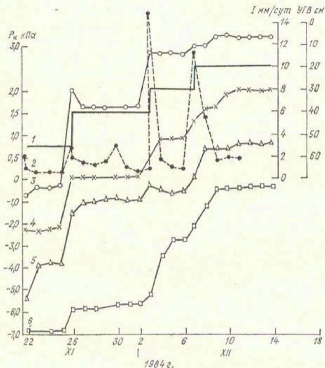
Рис. 4.7. Динамика потенциала влаги P_k , УГВ и интенсивности расхода грунтовых вод I .
