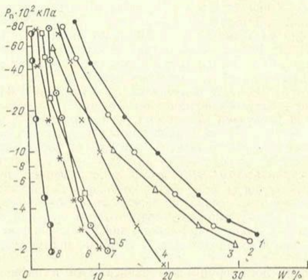
Рис. 3.2. Зависимость полного потенциала почвенной влаги P_{\text{п}} от влажности почвы W , полученная психрометрическим методом.
