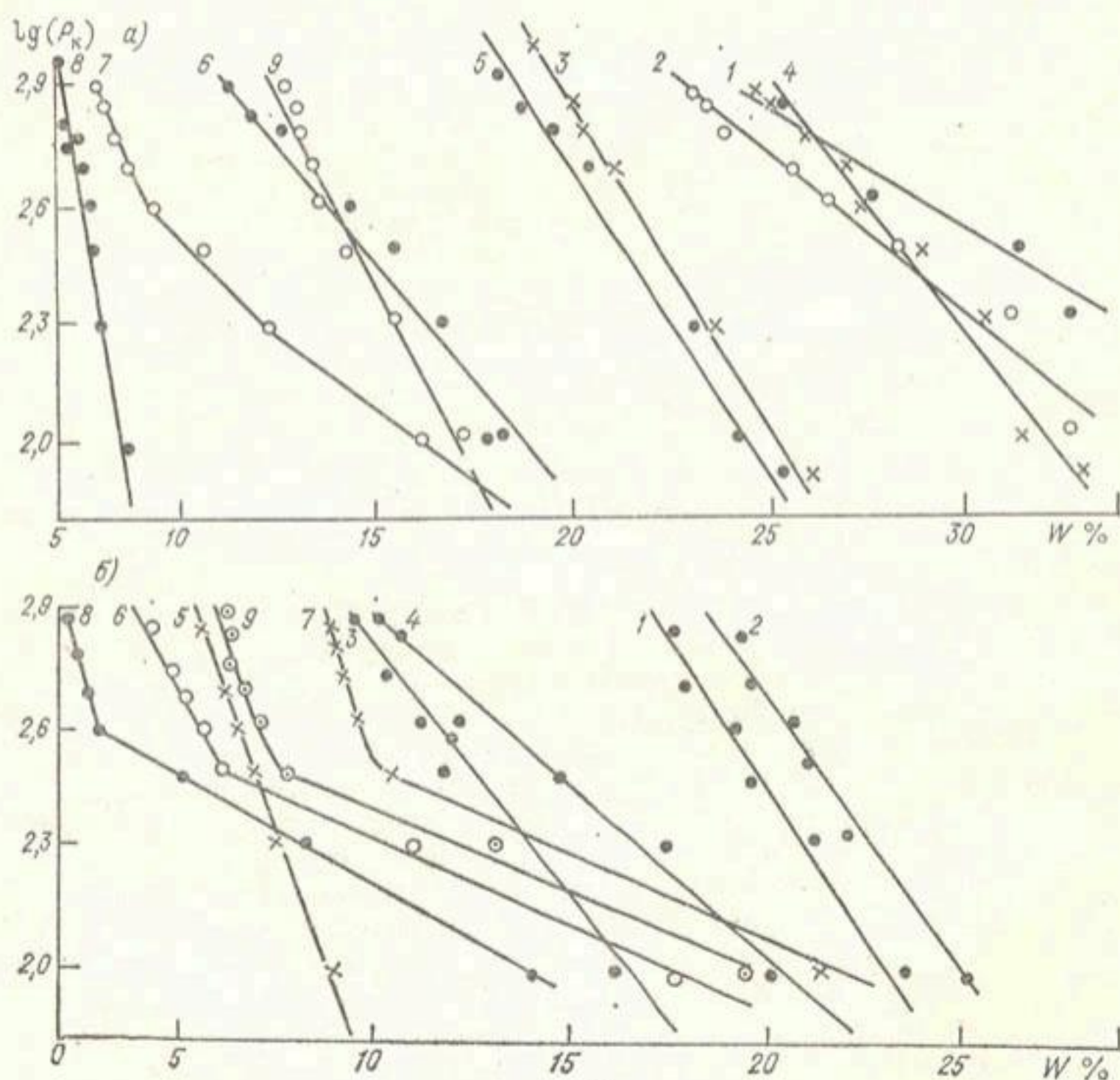
Рис. 3.1. Зависимость капиллярно-сорбционного потенциала почвенной влаги ново-подзолистой
