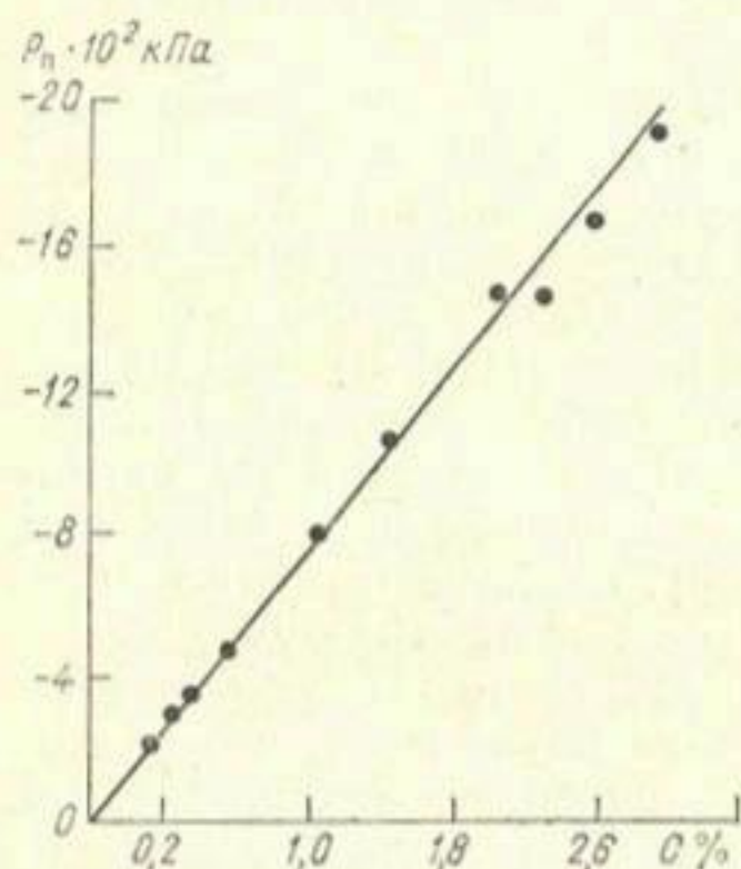
Рис. 3.10. Зависимость потенциала почвенной влаги P_n от содержания водорастворимых солей C .
