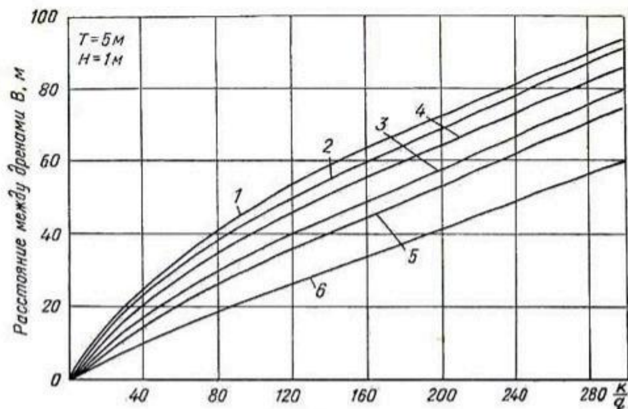
Рис. 21. Зависимость B = f\left(\frac{k}{q}\right) при T=5 м; H=1 м:
