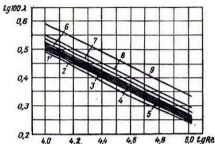
Рис. 30. Сводный график зависимости \lg 100\lambda = f(\lg Re) для полиэтиленовых гладкостенных неперфорированных труб:
