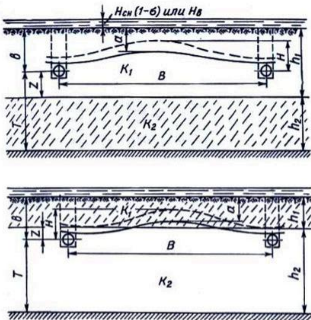
Рис. 20. Схемы к расчету расстояний между дренами в двухслойных грунтах.
