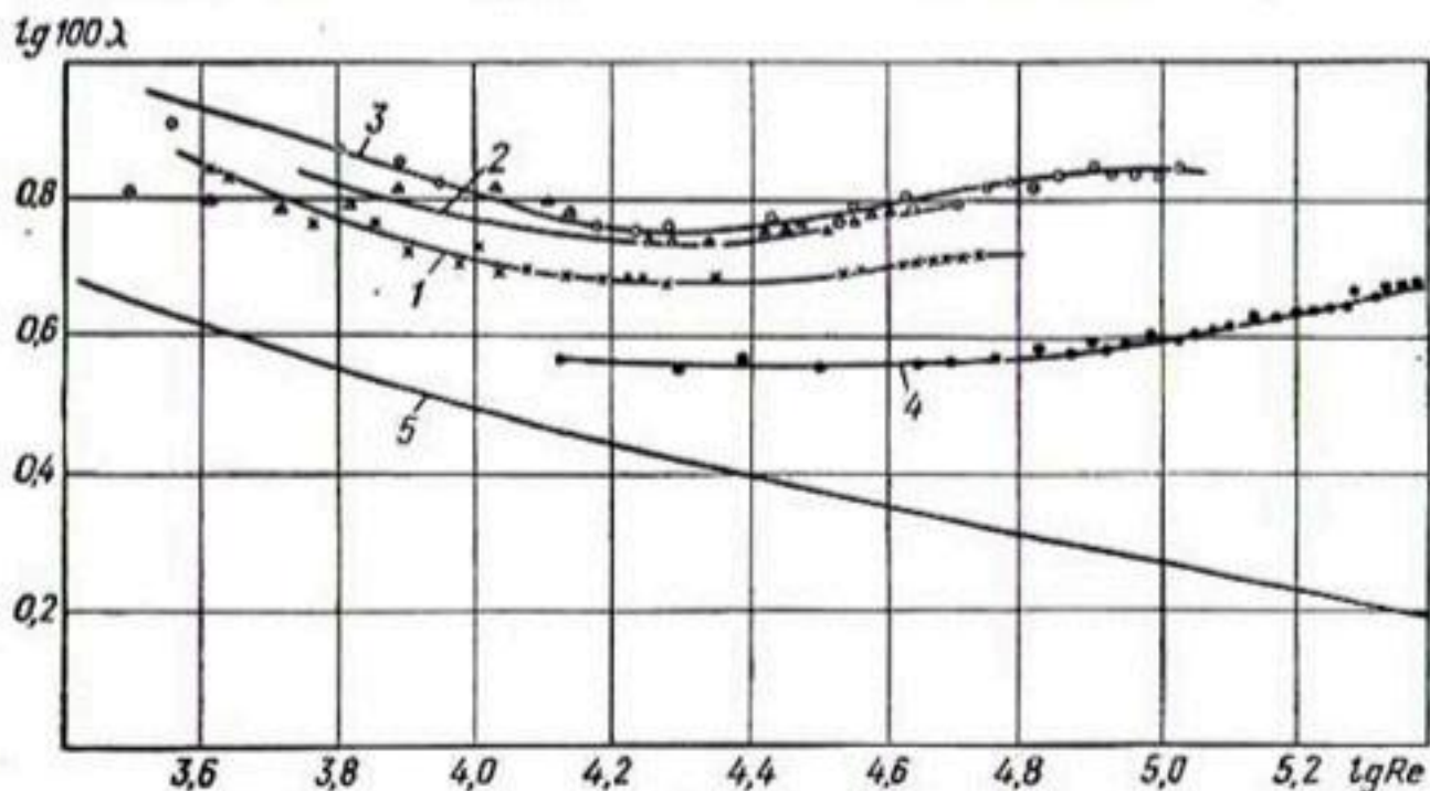
Рис. 37. Зависимость \lg 100\lambda = f(\lg Re) для полиэтиленовых гофрированных труб конструкции БелНИИМВХ:
