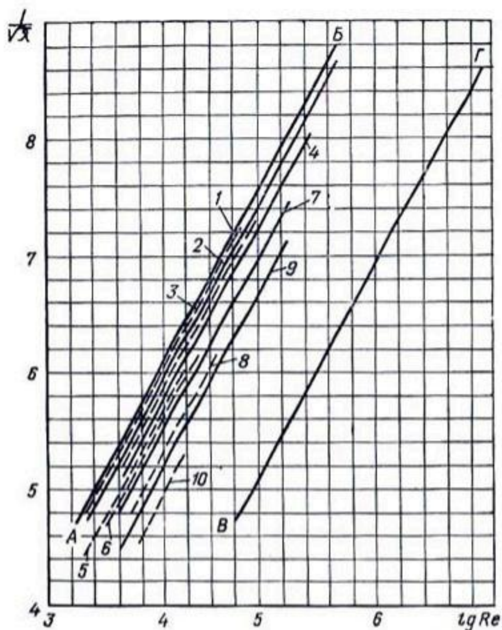
Рис. 32. Зависимость \frac{1}{\lambda} = \varphi(\lg Re) для гладкостенных полиэтиленовых труб:
