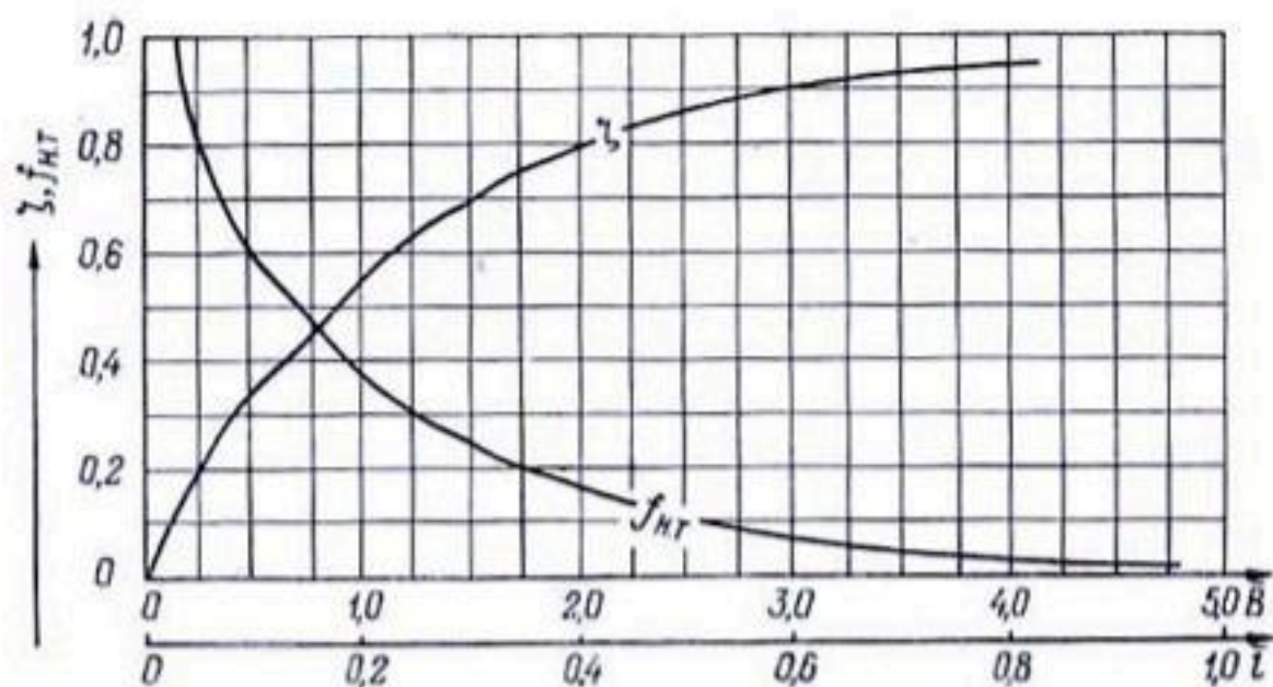
Рис. 24. Зависимость \xi = f(\bar{B}) .
