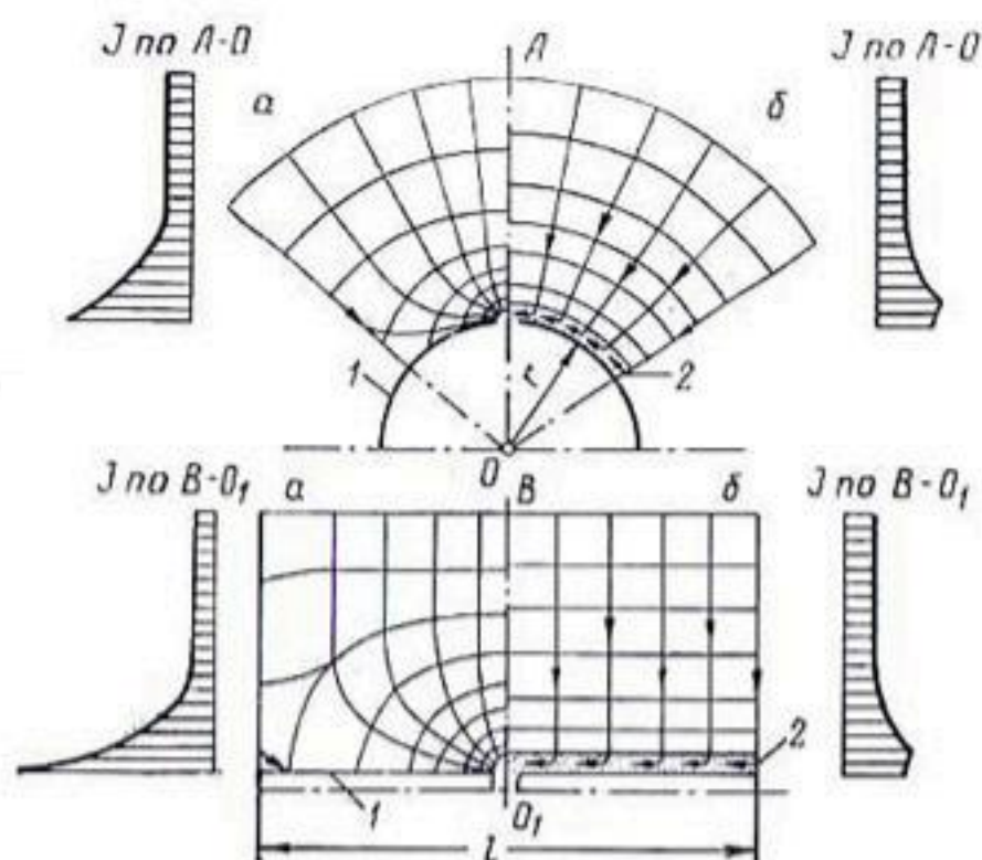
Рис. 13. Схемы притока воды к дренам и эпюры градиентов: сверху — к трубе с тремя рядами продольных щелей, внизу — с поперечными стыковыми зазорами (щелями); а — без фильтра, б — с фильтром; 1 — труба; 2 — фильтр.
