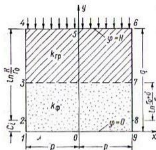
Рис. 19. Нормальный прямоугольник.
