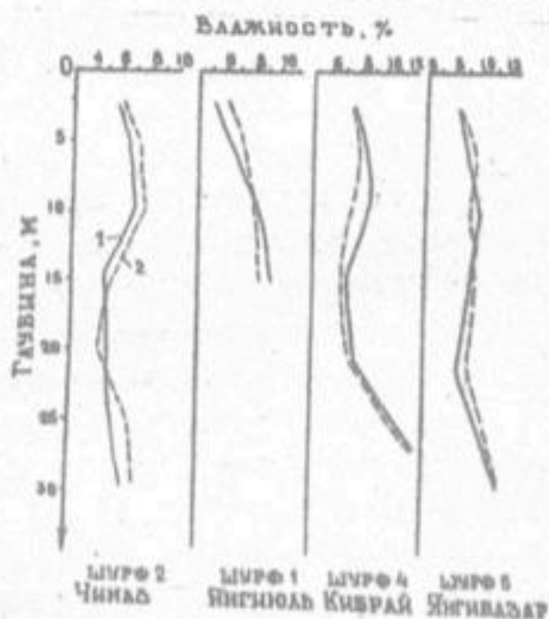
Рис. I. Сравнение естественной (1) и максимальной гигроскопической (2) влажности лессовых пород.
