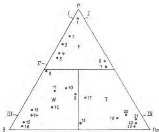
Рис. 1.6. Диаграмма, иллюстрирующая подразделение дельт на три типа по преобладанию влияния одного из трех факторов: реки (F), волнения (W) и приливов (Т) по У.Е.Галловейо [39]
