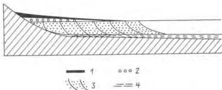
Рис. 1.4. Схема строения дельтовых отложений по Дж.Барреллу [176, 210]
