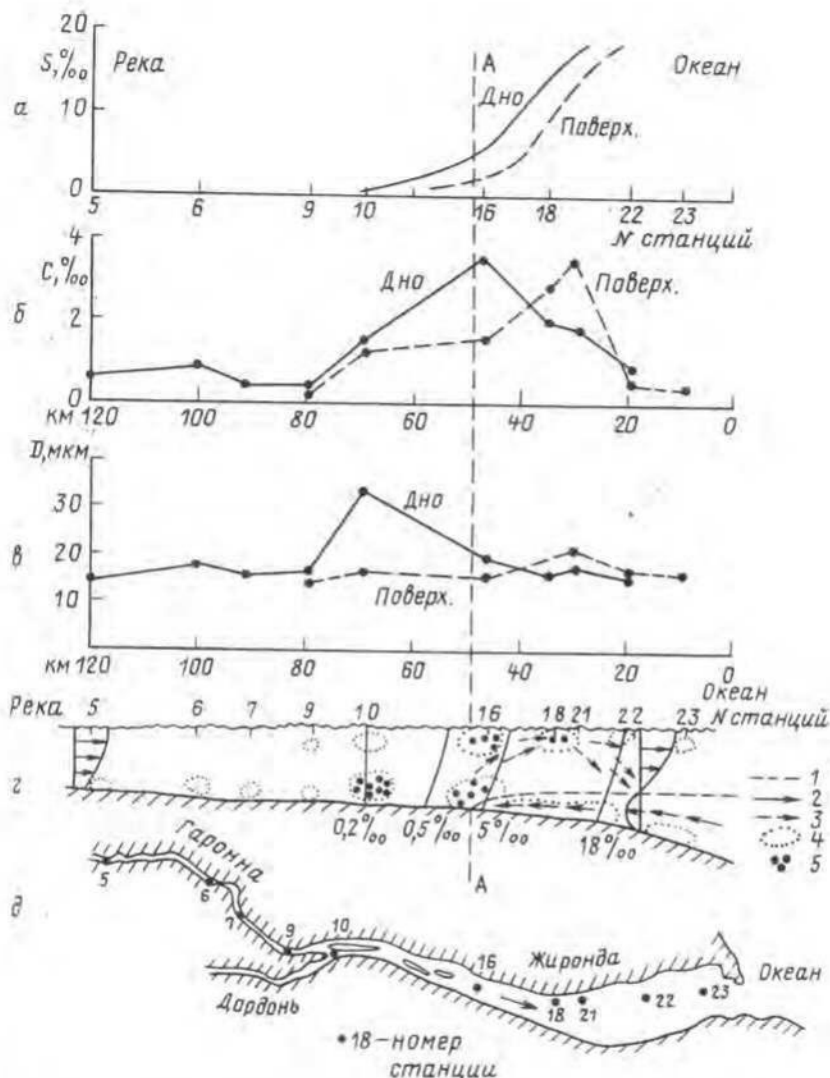
Рис. 3.2. Продольное изменение солености воды (в ‰) (а), концентрации взвешенных наносов в ‰ (б), крупности взвеси (в), а также продольный разрез русла (г) и схема русла в плане (д) с номерами станций в устье Жиронды по [241]
