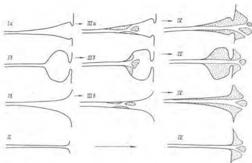
Рис. 1.3. Типы устьевых областей рек [124, 136]
