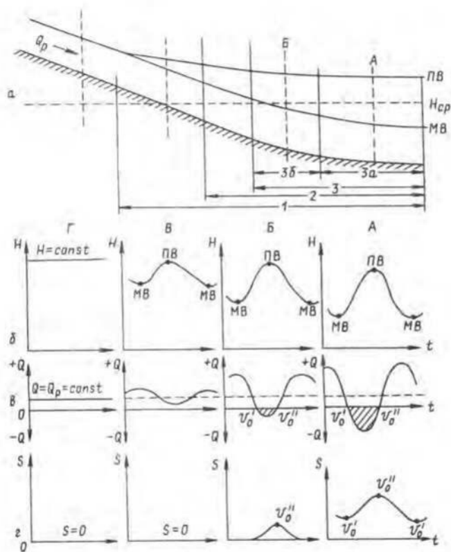
Рис. 2.4. Зоны на приливном устьевом участке реки (а): 1 – с приливными колебаниями уровня, 2 – с обратными течениями, 3 – с осолоненными водами ( 3a – в любую фазу прилива, 3b – в приливную фазу); графики изменения в течение приливного цикла уровней воды (б), расходов воды (в), солёности воды (г) на створах, расположенных на разном расстоянии от моря и в пределах различных зон; v'_0 и v''_0 – моменты смены течений (нулевой скорости), заштрихованы области графиков при обратных течениях. ПВ – полная вода, МВ – малая вода при приливах, H_{cp} – средний приливный уровень воды на устьевом взморе, Q_p – речной расход воды
