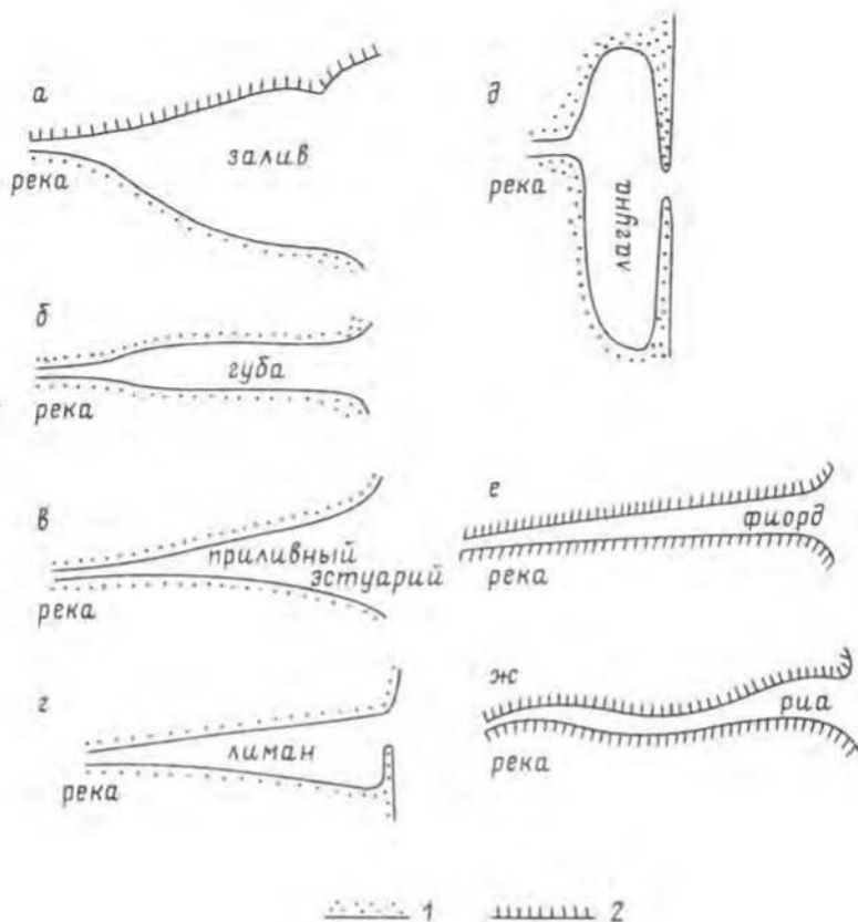
Рис. 1.8. Различные виды полужакрытых устьевых взморьев эстуарного типа а – залив, б – губа, в – собственно приливный эстуарий, г – лиман, д – лагуна, е – фиорд, ж – риа. Берега: 1 – низменные аккумулятивные, 2 – гористые
