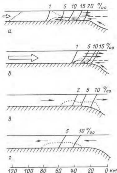
Рис. 3.1. Миграция зоны повышенной мутности воды ( \lambda > 1 \text{ кг/м}^3 ) в устье Жиронды а – половодье, б – межень [207]; в – отлив, г – прилив [208]. Стрелки показывают направление течений; наклонные линии – изогалины (в ‰)
