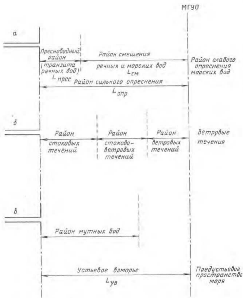
Рис. 1.12. Схема районирования устьевое взморья по характеру смешения речных и морских вод (а), течений (б), мутности воды (в)
