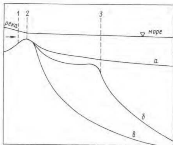
Рис. 1.2. Типы устьевых взморья в зависимости от глубины и рельефа дна [179] а – отмелое, б – отмелое со свалом глубин, в – приглубое; 1 – морской край дельты, 2 – устьевой бар, 3 – свал глубин
