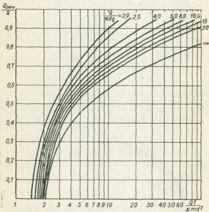
Рис. 20. График \frac{Q_{\text{реч}}}{Q} = f\left(\overline{T}, \frac{Q}{\pi dq}\right) для одиночного берегового водозабора при \beta = -\frac{\pi}{2} и \frac{d_0}{d} = 1
