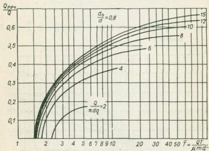
Рис. 16. График \frac{Q_{pеч}}{Q} = f\left(\bar{T}, \frac{Q}{\pi d q}\right) для одиночного берегового
