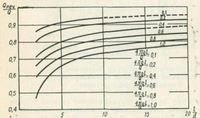
Рис. 9. График \frac{Q_{\text{реч. max}}}{Q} = f \times \left( \frac{4 \pi q l}{Q}; \frac{l}{d} \right) для определения максимального количества поверхностных вод, подтягиваемых к линейному водозабору при \beta = \frac{\pi}{2}
