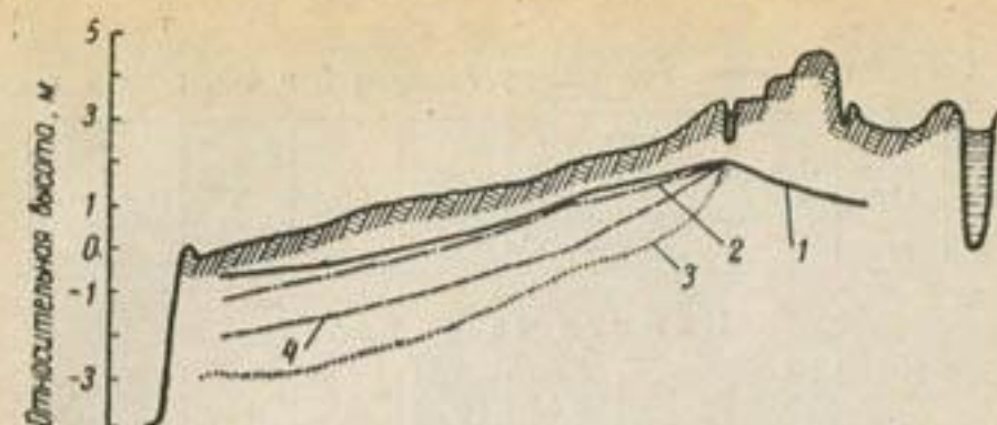
Рис. 24. Изменение уровня грунтовых вод под влиянием дренажа. Профиль по створу 1-1:
