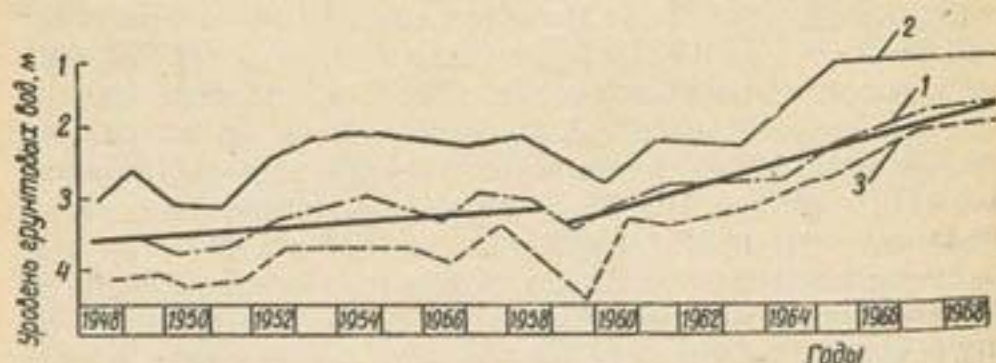
Рис. 21. Многолетняя динамика уровня грунтовых вод: 1 — среднегодовая; 2 — весна (март); 3 — осень (октябрь).
