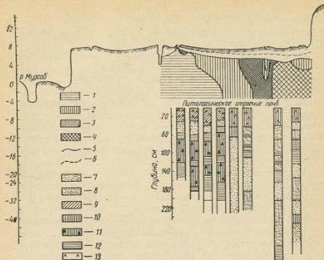
Рис. 20. Почвенно-гидрохимический профиль в верхней части Мургабской дельты:
