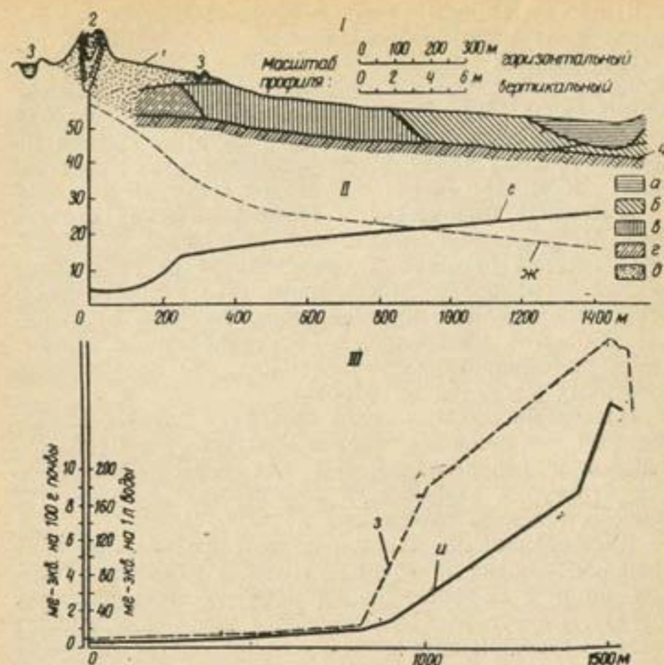
Рис. 11. Распределение и состав ирригационных отложений от канала к межканальному понижению:
