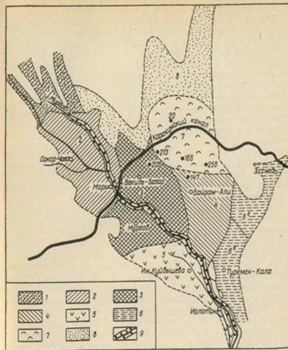
Рис. 19. Схема массивов разной давности орошения Мургабского оазиса:
