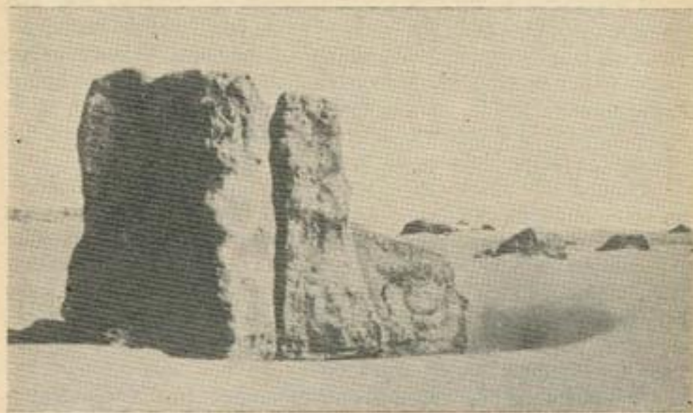
Рис. 9. Останцы из аллювиально-озерных отложений Харгинской депрессии.
