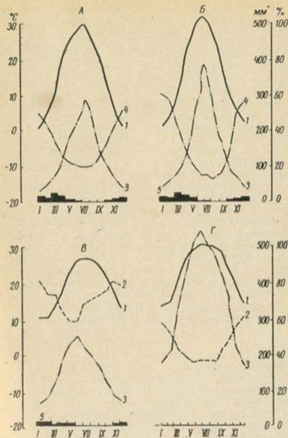
Рис. 4. Главнейшие климатические показатели по оазисам в Туркмении — Байрам-Али (А), Репетек (Б), в АРЕ — Тахта (В) и Харга (Г):
