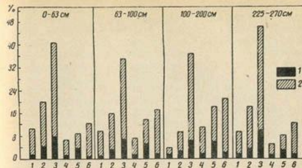
Рис. 13. Распределение карбонатов по фракциям в древнеорошаемой почве, % на сухую почву:
