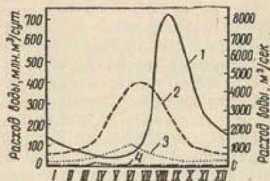
Рис. 6. Сток речных вод:
