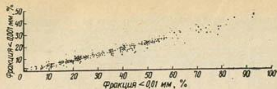
Рис. 12. Зависимость содержания ила от механического состава отложений Мургабской дельты.
