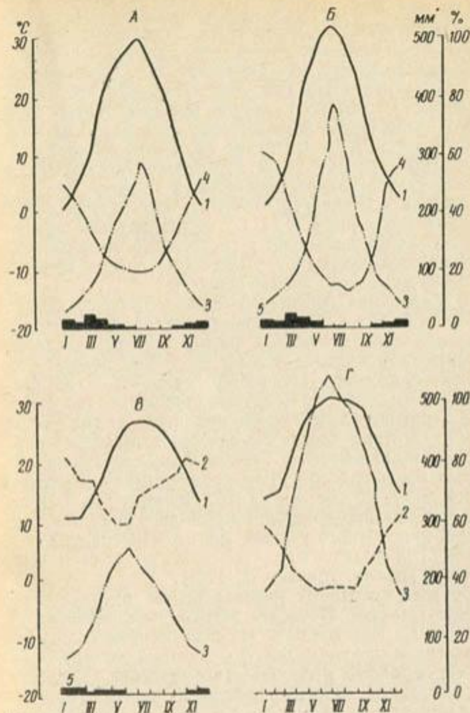
Рис. 4. Главнейшие климатические показатели по оазисам в Туркмении — Байрам-Али (А), Репетек (Б), в АРЕ — Ташта (В) и Харга (Г):
