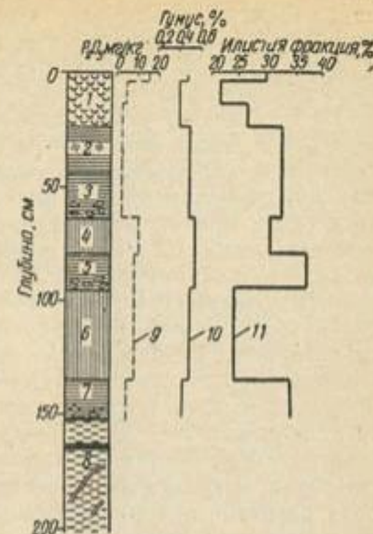
Рис. 1. Профиль геоксюрской почвы и распределение гумуса, подвижного фосфора и ила:
