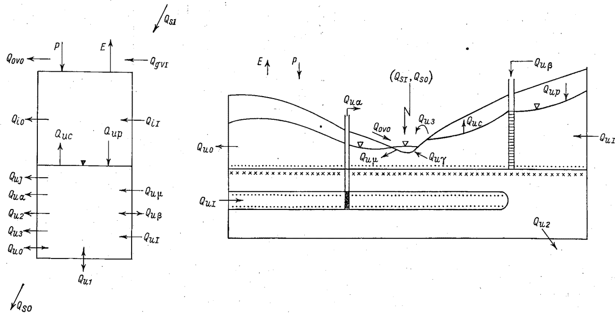
Рис. 12. Поперечный разрез речного бассейна, изображающий концептуальную модель баланса подземных вод. Обозначения даны согласно уравнениям (1), (104), (105) и (106).
