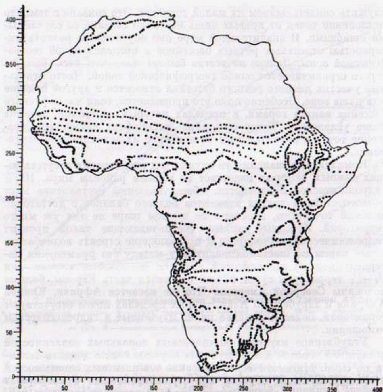
Рис. 3. Пример карты валового увлажнения территории Африки, построенной на графопостроителе [уменьшена более чем в 2 раза]
