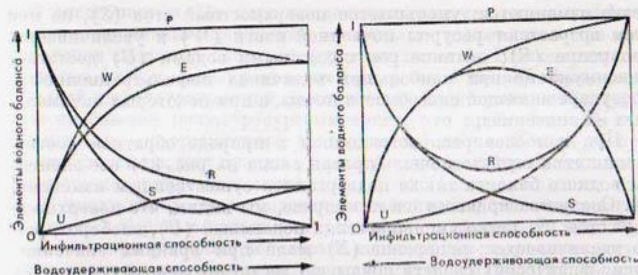
Рис. 21. Теоретические зависимости водного баланса от свойств почвы: P — атмосферные осадки; R — полный речной сток; U — подземный сток в реки; S — поверхностный (паводочный) сток; W — валовое увлажнение территории; E — испарение
