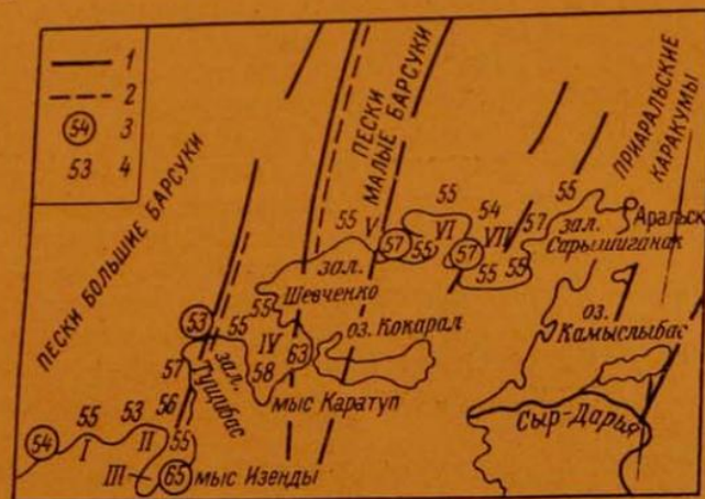
Рис. 2. Тектоническая схема Северного Приаралья.
