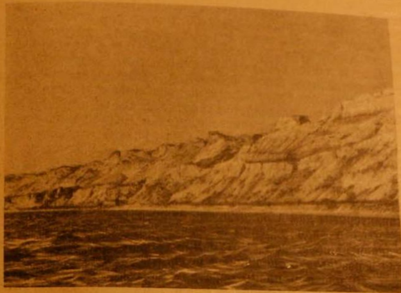
Рис. 34. Три уровня морских террас (к северу от мыса Актумсык).
