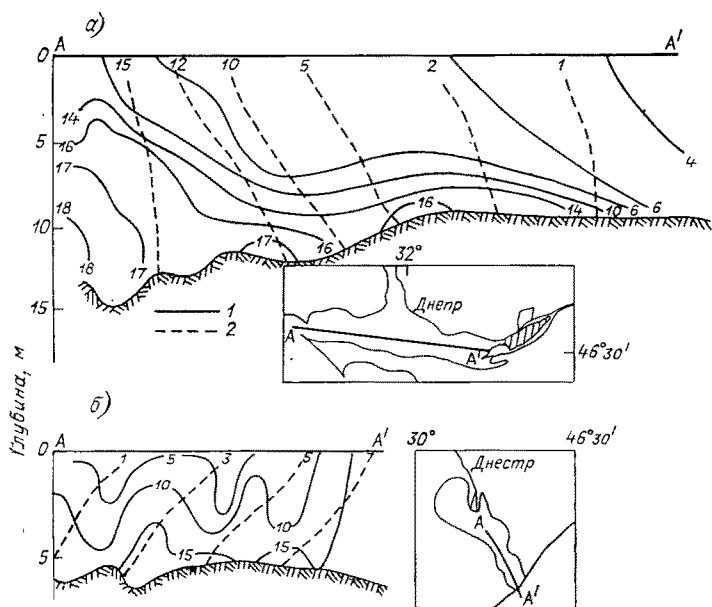
Рис. 34. Вертикальное распределение солености (‰) в лиманах Днепро-Бугском (а) и Днестровском (б) на осевых разрезах в маловодный 1972 г. (1) и средний по водности год (2) [436].
