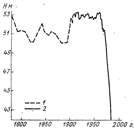
Рис. 3. Многолетние изменения уровня Аральского моря [321]. 1 — восстановленные по косвенным данным; 2 — наблюдаемые.
