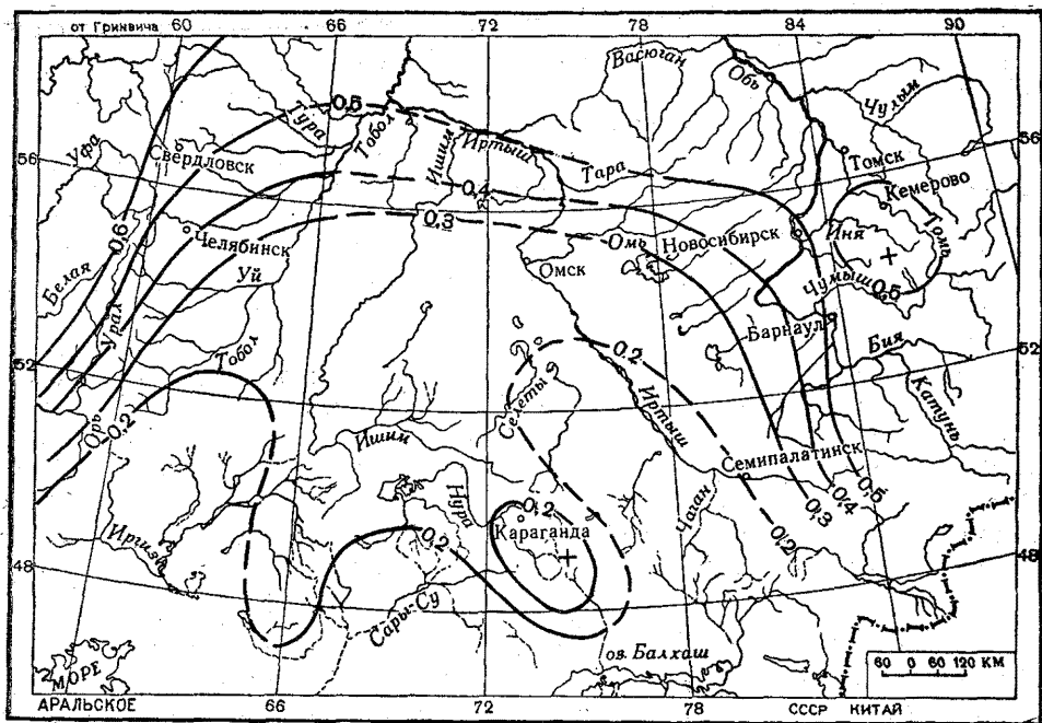
Рис. 30. Схематическая карта коэффициента зарегулированности стока \varphi(I)_{\text{пр}} .
