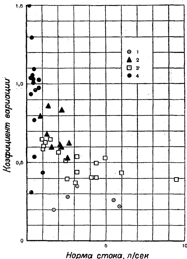
Рис. 17. Зависимость коэффициентов вариации ( C_v ) от нормы стока ( M_0 ).
