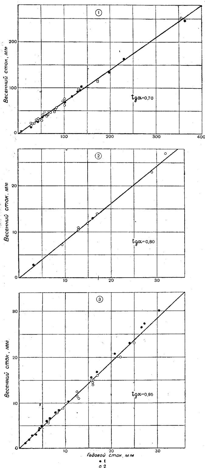
Рис. 13. Графики связи весеннего и годового стока. (1) — лесостепные районы, (2) — степные районы, (3) — полупустынные районы. 1 — за период наблюдений, 2 — за многолетний период.
