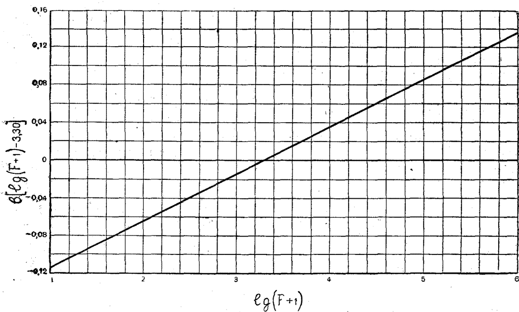
Рис. 31. Вспомогательный график зависимости b[\lg(F+1) - 3.30] = f[\lg(F+1)] .
