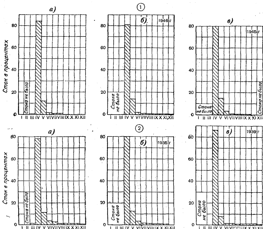
Рис. 26. Распределение стока на реках Казахского мелкосопочника. 1 — р. Ишим — г. Акмолинск ( F = 7400 \text{ км}^2 ), 2 — р. Нура — с. Сергипольское ( F = 11300 \text{ км}^2 ). а) средний фиктивный год, б) средний реальный год, в) маловодный год.
