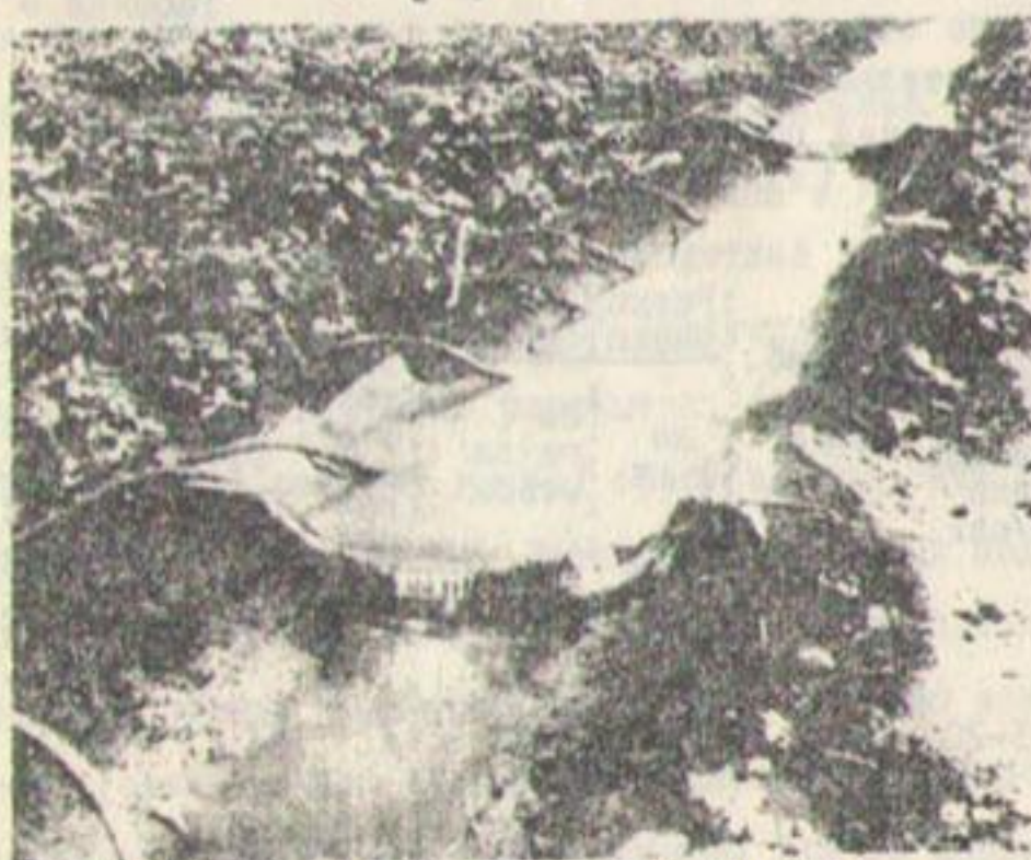
Рис.9. Полив по бороздам с помощью сифонов и брезентовых перемычек (совхоз им. Кирова)
