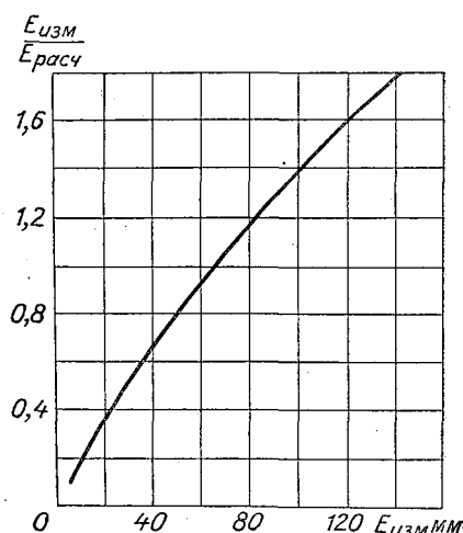
Рис. 67. Поправочный коэффициент к величинам испарения с почвы, измеренным с помощью испарителей ГТИ-500-50.
