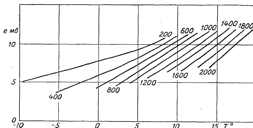
Рис. 61. График для расчета величин испарения (мм/сут.) за теплый сезон с водноиспарительного бассейна площадью 20 м² по средним годовым значениям температуры и влажности воздуха, измеренным на высоте 2,0 м.
