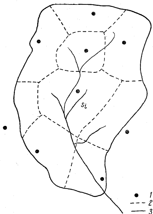
Рис. 74. Схема разбивки водосбора на участки.
