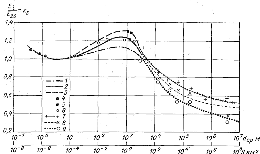
Рис. 87. Зависимость интенсивности испарения от среднего диаметра и площади водоема.
