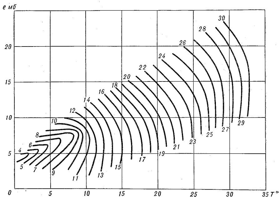
Рис. 90. График для расчета среднесуточной (за декаду, месяц) температуры поверхности водноиспарительного бассейна площадью 20 м 2 , глубиной 2,0 м по исправленным средним значениям температуры и влажности воздуха (т. е. с учетом величин \Delta T_{\text{в}} и \Delta e_{\text{в}} ).
