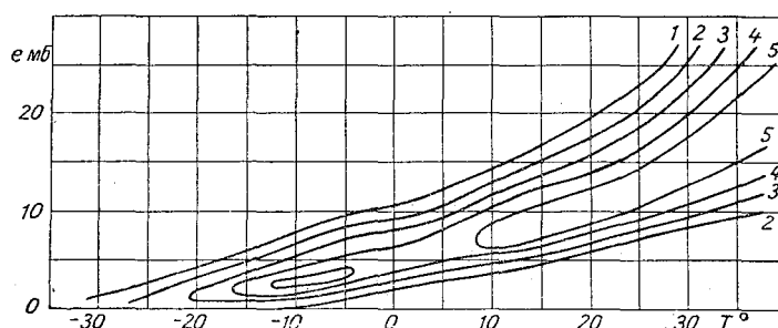
Рис. 54. Зависимость скорости ветра на высоте флюгера u_f за отдельные сроки от исправленных значений температуры и влажности воздуха на высоте 2,0 м.
