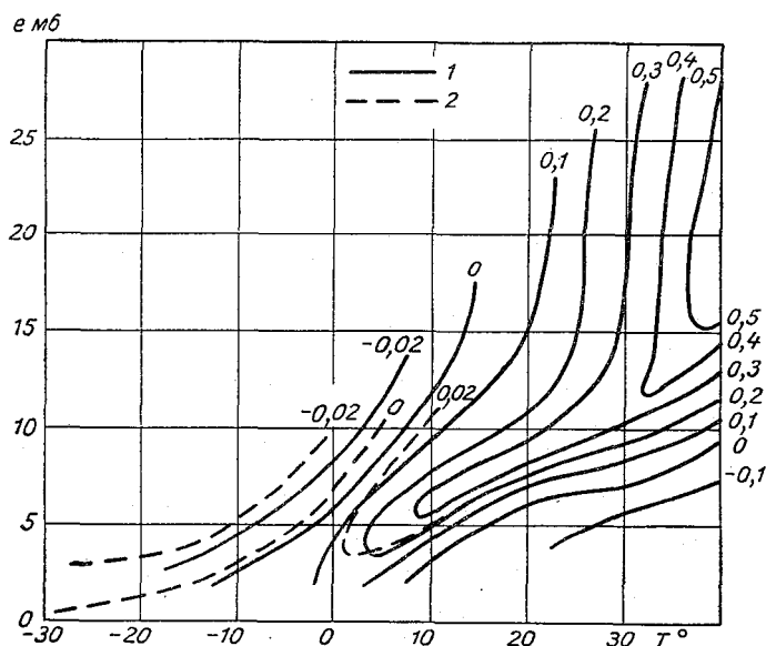
Рис. 56. Зависимость интенсивности испарения (мм/час) с почвы (1) и снега (2) от исправленных срочных значений температуры и влажности воздуха (т. е. с учетом величин \Delta T , \Delta e и \delta e ).
