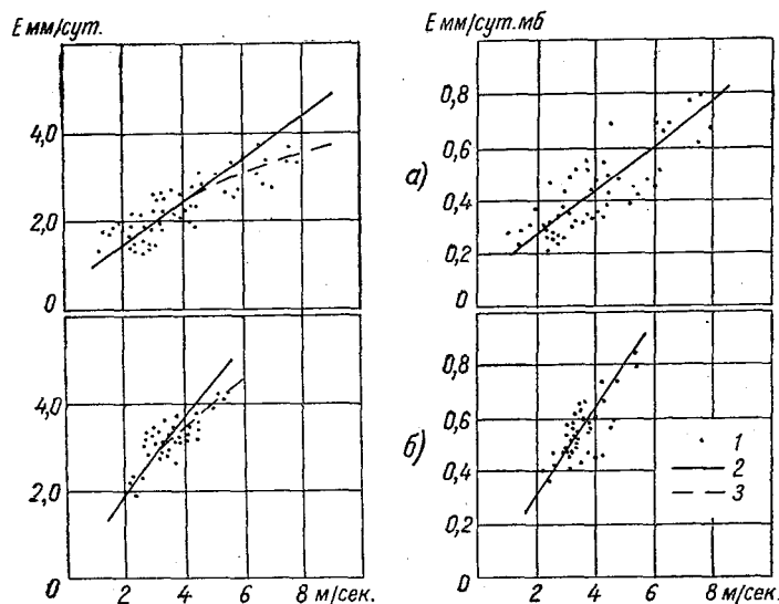
Рис. 95. Зависимость интенсивности испарения (мм/сут.) и ее величины, отнесенной к дефициту влажности (мм/сут. мб), от скорости ветра для бассейна площадью 20 м 2 (а) и Валдайского озера (б).
