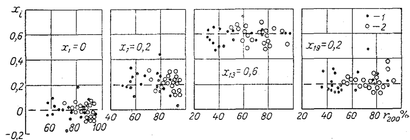
Рис. 118. Зависимость коэффициентов x_i , характеризующих суточный ход испарения с почвы, от влажности почвы и воздуха.
