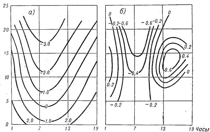
Рис. 78. Поправки \delta T_v и \delta e_v на суточный ход температуры (а) и влажности (б) воздуха (используемой при расчете испарения с водной поверхности) в зависимости от исправленных значений температуры на ее сезонный ход (т. е. с учетом величины \Delta T_v ).
