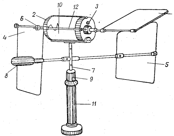
Рис. 13. Схема трехлопастного анемомографа.
