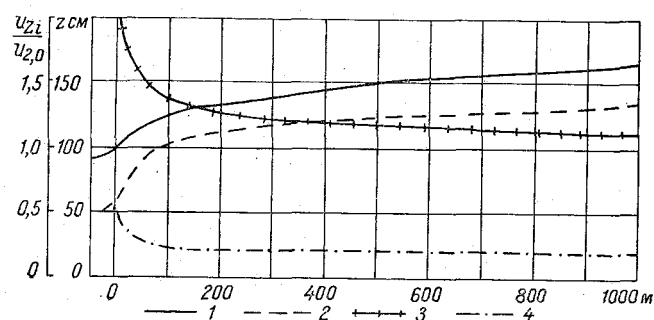
Рис. 82. Трансформация скорости ветра и опускание линий тока над водоемом.
