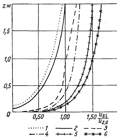
Рис. 81. Профили ветра в различных пунктах измерений по створу. 1 — 50 м от уреза, 2 — урез, 3, 4, 5 и 6 — 50, 100, 500 и 1000 м от уреза, u_{zi} — скорость ветра на высоте z в i -том пункте измерения, u_{2,0} — скорость ветра на высоте 2,0 м на урезе.
