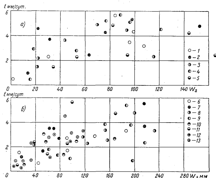
Рис. 130. Примерный вид зависимости суммарного испарения с некоторых сельскохозяйственных полей от активных влагозапасов слоя почвы мощностью 0,5 м для ВНИГЛ и 1,0 м для ДНИГЛ. а — лен, ВНИГЛ; б — яровая пшеница, ДНИГЛ; 1 — всходы; 2 — начало роста стебля, 3 — образование соцветий, 4 — цветение, 5 — зеленая спелость, 6 — всходы, 7 — 3-й лист, 8 — кущение, 9 — выход в трубку, 10 — колошение, 11 — цветение, 12 — молочная спелость, 13 — восковая спелость.
