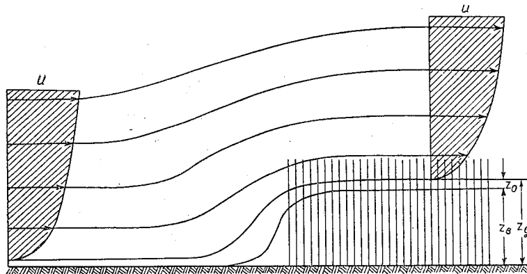
Рис. 31. Схема набегания воздушного потока на густой и высокий травостой.
