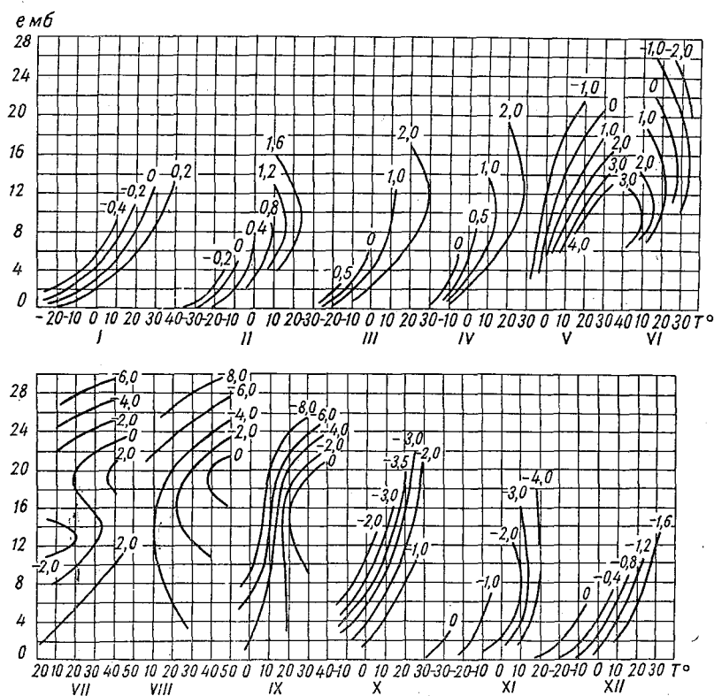
Рис. 48. Поправки \Delta e на сезонный ход влажности воздуха по месяцам в зависимости от измеренных значений температуры и влажности воздуха.
