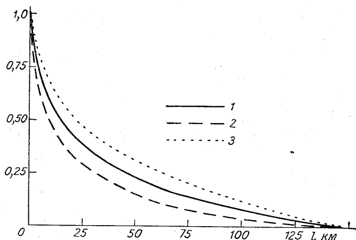
Рис. 71. Зависимость величин \frac{T_{l,и} - T_{c,и}}{T_{m,и} - T_{c,и}} и \frac{e_{l,и} - e_{c,и}}{e_{m,и} - e_{c,и}} от расстояния l выбранного пункта наблюдений до берега. 1 — среднее положение кривой трансформации; 2 — кривая трансформации для весенне-летнего периода; 3 — кривая трансформации для осенне-зимнего периода.
