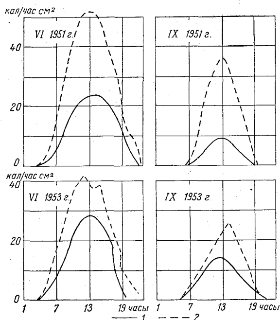
Рис. 119. Средний за месяц суточный ход суммарной радиации и затраты тепла на испарение с луга при различной влажности почвы.
