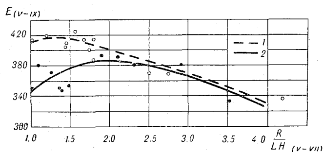
Рис. 113. Зависимость испарения с леса (1) и поля (2) от индекса сухости \frac{R}{LH} (за май—июль).
