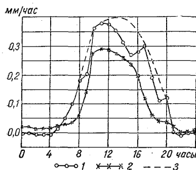
Рис. 117. Суточный ход испарения с луга.
