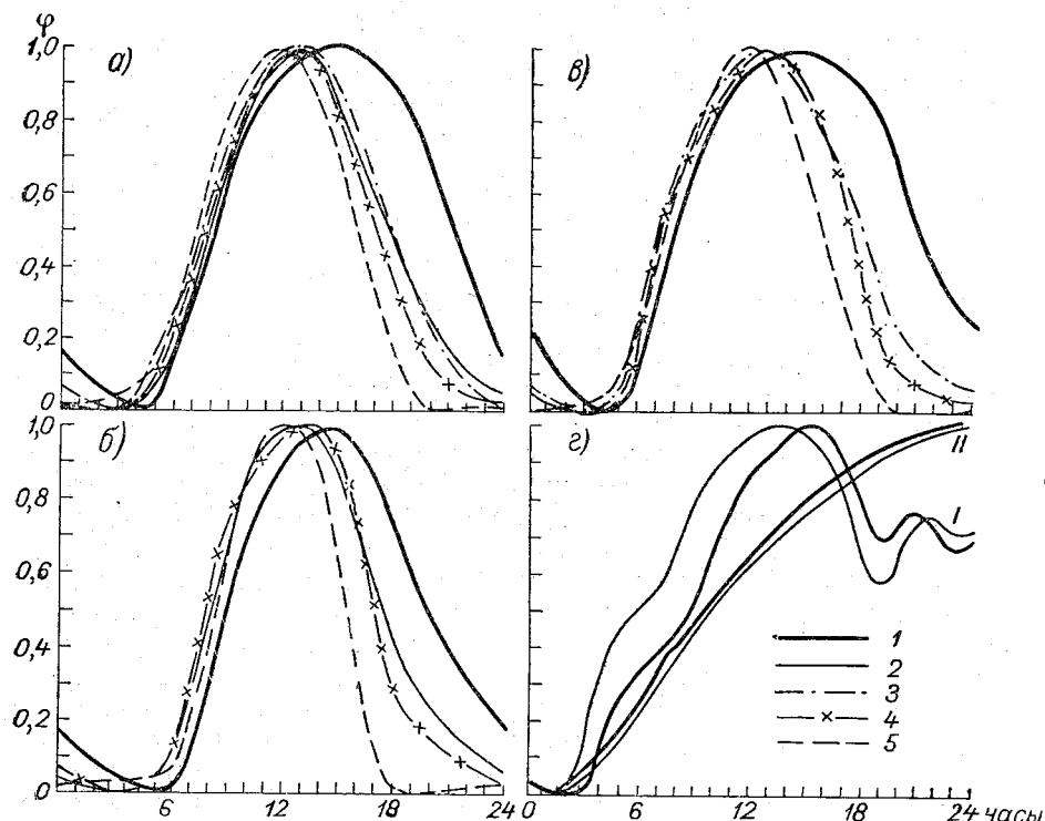
Рис. 44. Суточный ход температуры воздуха T^{\circ} (1), эффективного излучения E_{\text{эф}} (4), радиационного баланса R (5) и температуры почвы, измеренной ртутными термометрами T_{\text{п. рт}} (2) радиационным методом T_{\text{п. рад}} (3). а — оголенная почва и б — степная растительность при ясном небе в июне 1962 г.; в — оголенная почва при ясном небе в сентябре 1961 г.; г — снежный покров 30/1 1963 г. (II).
