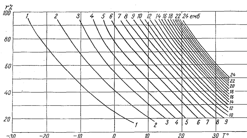
Рис. 75. Связь между среднемесячными величинами абсолютной и относительной влажности воздуха.
