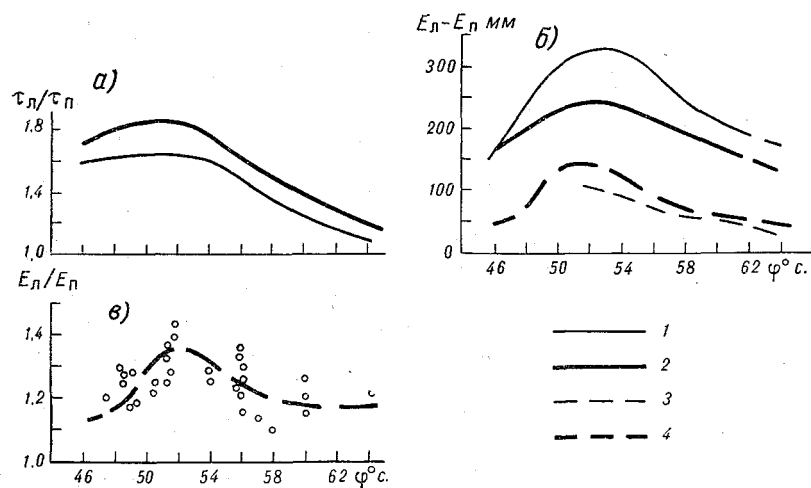
Рис. 116. Зависимость отношения продолжительности периодов вегетации леса \tau_{\text{л}} и поля \tau_{\text{п}} (а), разности величин испарения с леса и поля (б), отношения испарения с лиственного леса к среднему испарению с окружающей территории (в) от широты местности \varphi . 1 — лес — озимые; 2 — лес — яровые; 3 — лес — болотная растительность; 4 — лес — поверхность суши.
