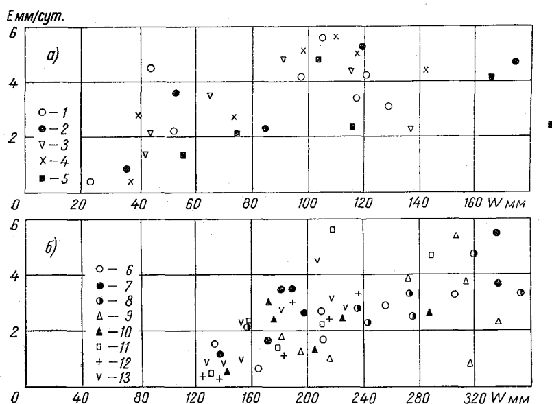
Рис. 129. Примерный вид зависимости суммарного испарения с некоторых сельскохозяйственных полей от общих влагозапасов слоя почвы мощностью 0,5 м для ВНИГЛ и 1,0 м для ДНИГЛ.
