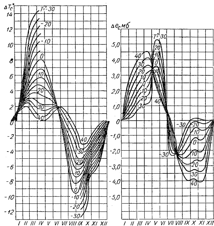
Рис. 68. График поправок на сезонный ход температуры \Delta T_c и влажности \Delta \epsilon_c воздуха над сушей.
