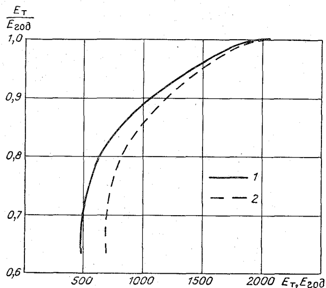
Рис. 62. График связи отношения испарения с водной поверхности за теплый период E_{\text{т}} к годовой величине E_{\text{год}} с величинами испарения за теплый период (1) и за год (2).
