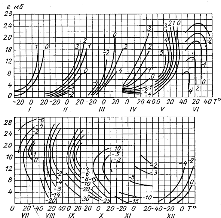
Рис. 46. Поправки \Delta T на сезонный ход температуры воздуха по месяцам в зависимости от измеренных значений температуры и влажности воздуха.
