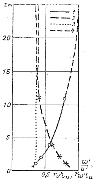
Рис. 17. Зависимость от- ношения вертикальной пульсации скорости w' к горизонтальной пульса- ции u' , величины коэф- фициентов корреляции r_{u'l_u} и r_{w'l_w} , а также
