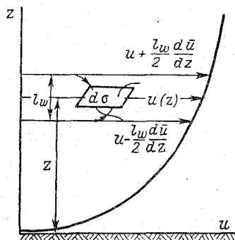
Рис. 21. Схема вертикального турбулентного переноса количества движения в атмосфере.
