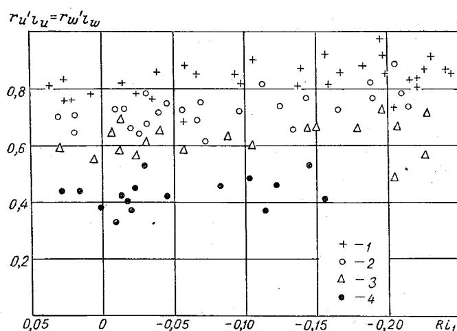
Рис. 20. Зависимость коэффициента корреляции r_{u'l_u} на различных уровнях от устойчивости стратификации атмосферы. Термоанемограф на высотах: 1) 1 м; 2) 2 м; 3) 4 м; 4) 11,5 м.
