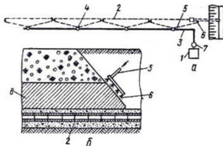
Рис. 21. Схема способа уплотнения засыпки грунта дрена.
