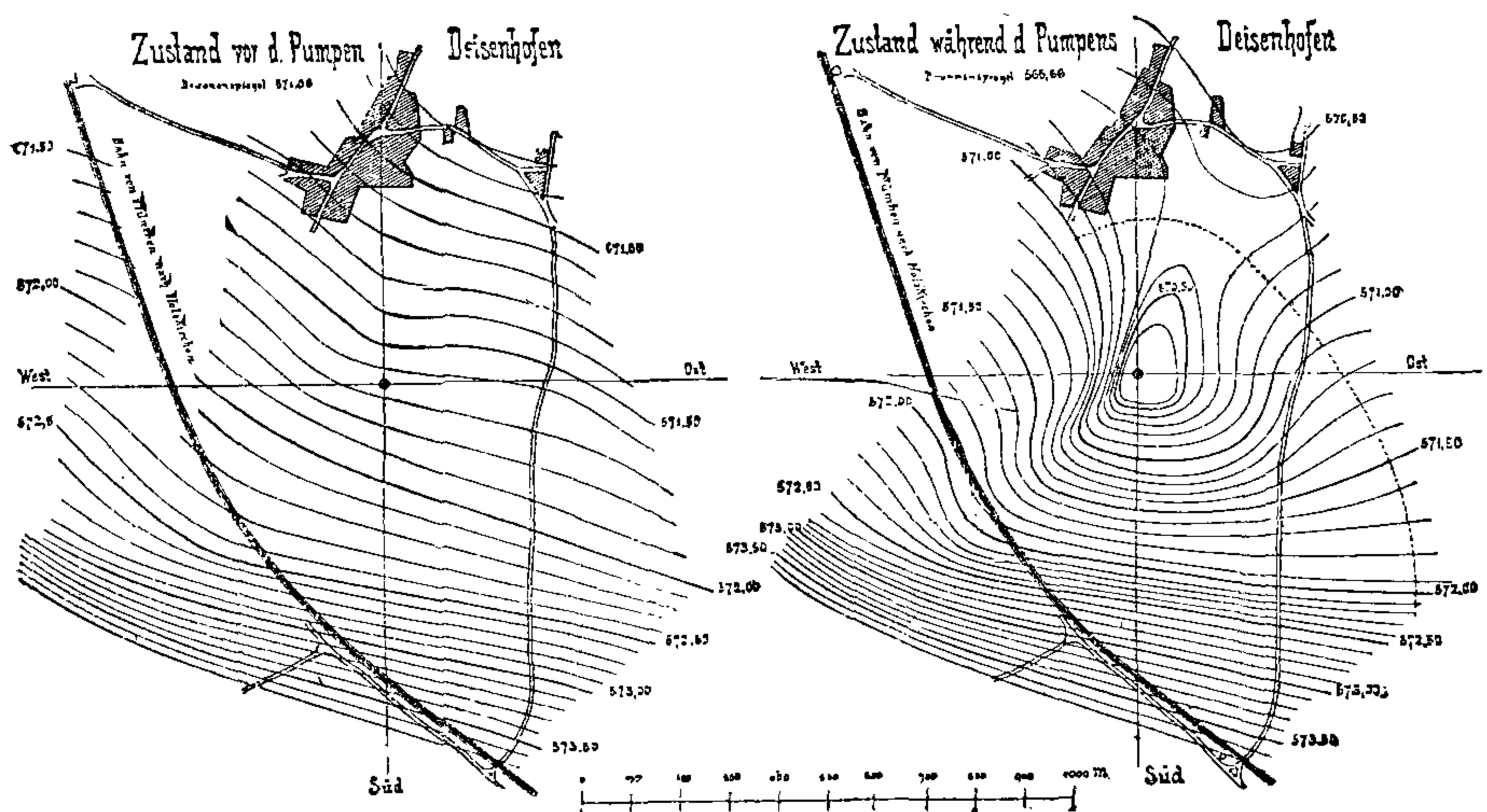
Фиг. 113. Горизонталы грунтовыхъ водъ въ области Дейзенгофскаго колодца.
