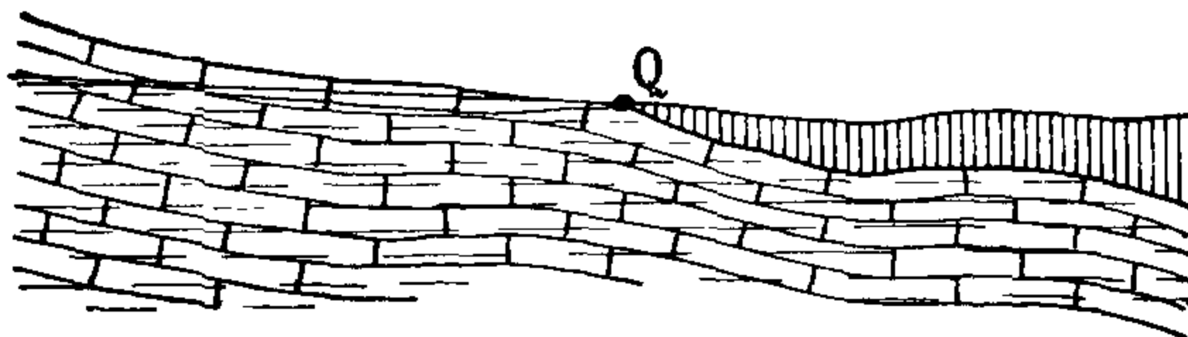
Пленерскій известнякъ Эмскій мергель
