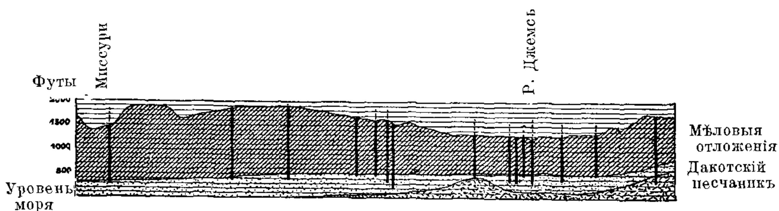
Фиг. 155. Поперечный профиль по линіи а—b на фиг. 153.
