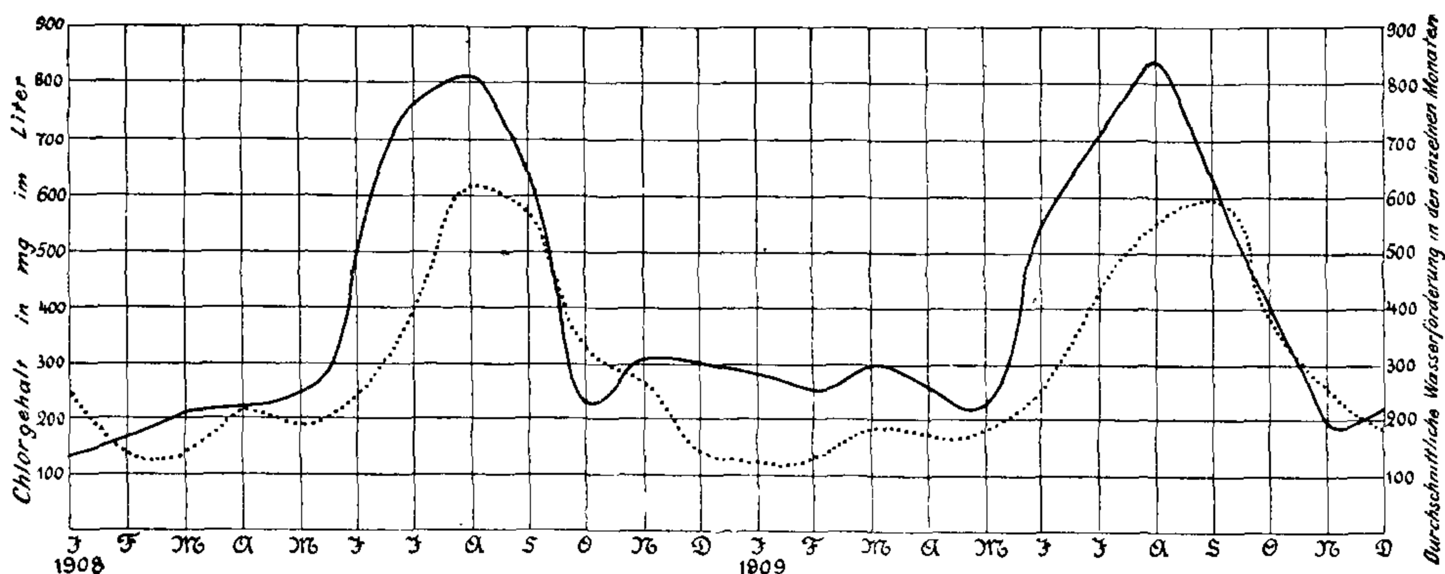
Фиг. 82. Зависимость между содержаніемъ хлора (пунктиръ) и расходомъ воды (сплошная).
