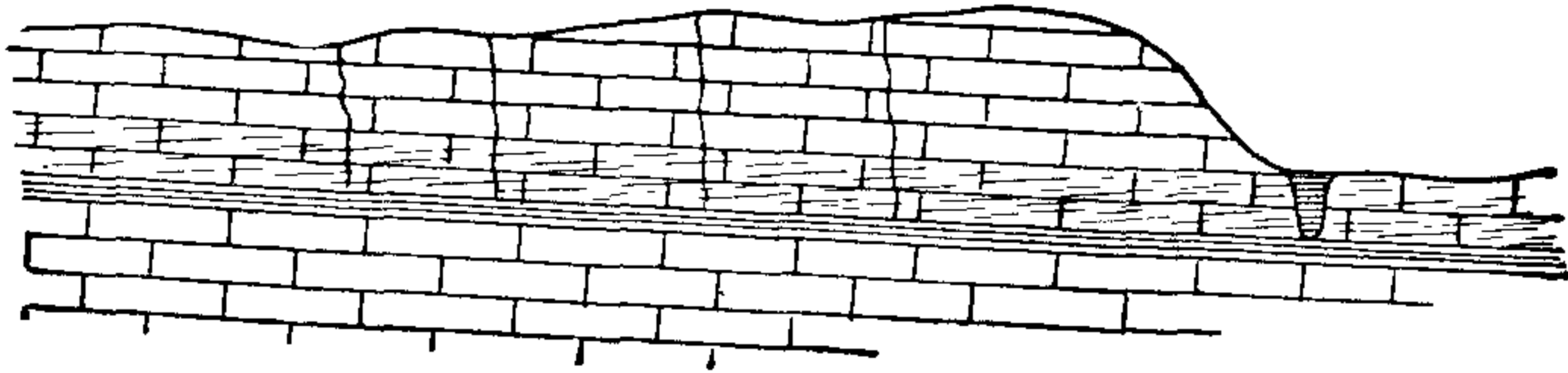
Фиг. 185. Блаутопфъ близъ Блаубёрена.
