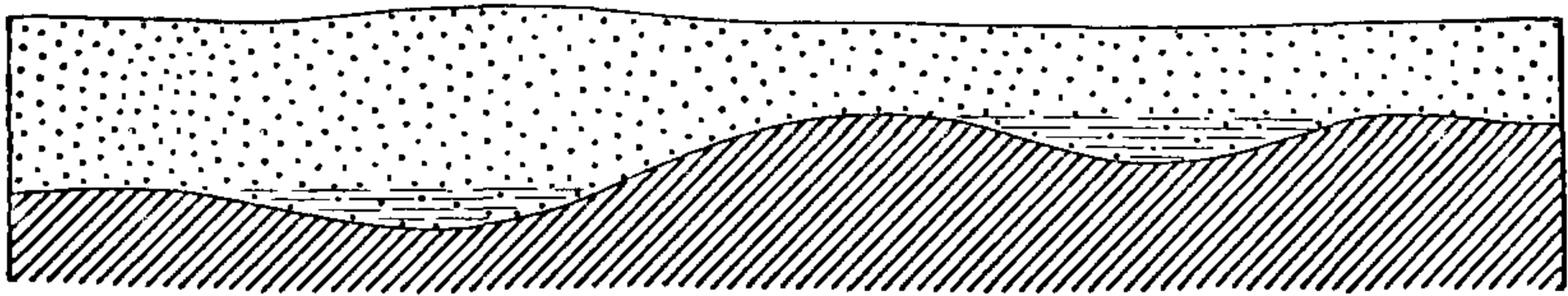
Фиг. 60. Озера грунтовой воды.
