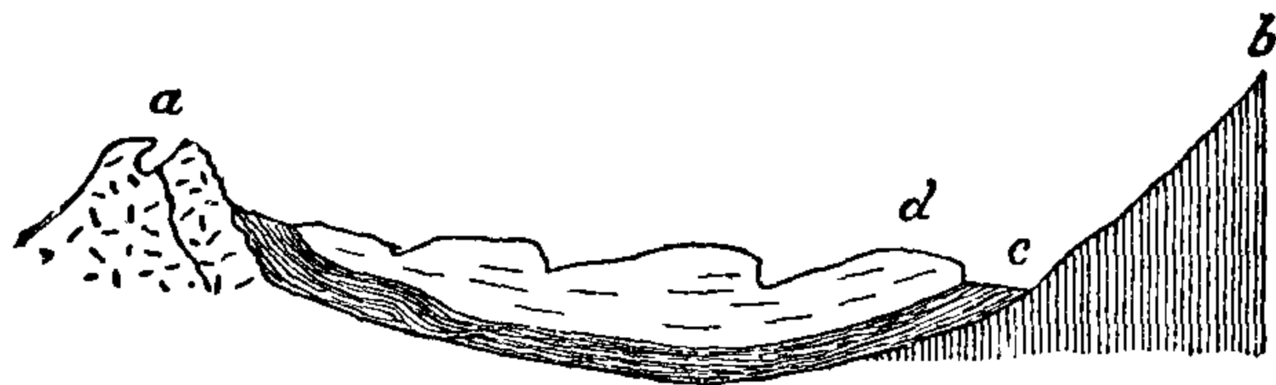
Фиг. 105. Профиль окрестностей Фюрстенфельда (по Д. Штуру).
