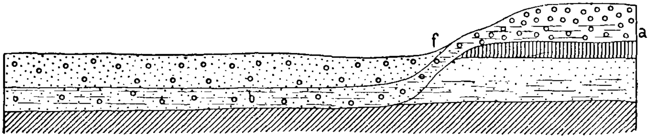
Фиг. 62. Подземный водопадъ.
