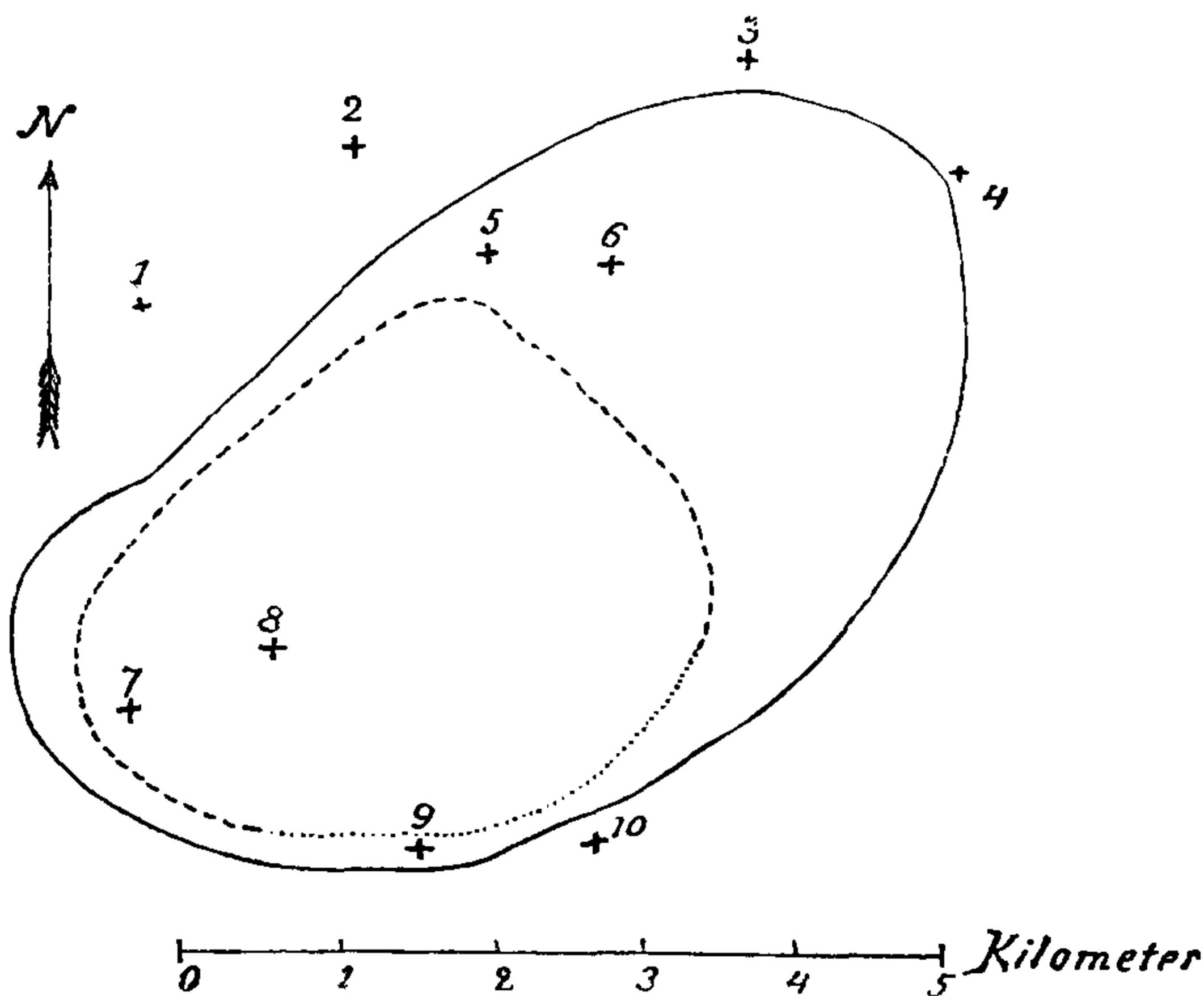
Фиг. 107. Torrent d'Anzin, по Добря.
