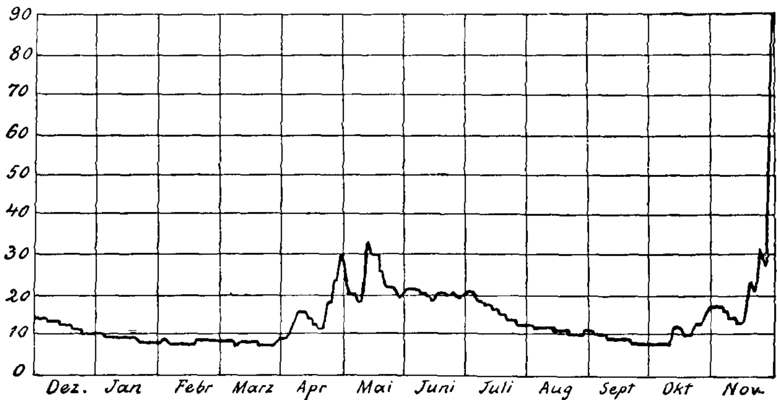
Фиг. 193. Дебитъ источника Воклюзъ въ 1877 г.
