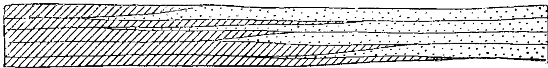
Фиг. 15. Переменно выклипывающееся напластованіе.
