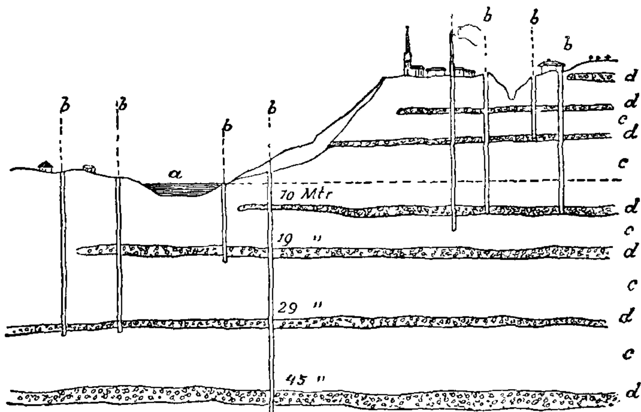
Фиг. 106. Разрѣзъ мѣстности Фюрстенфельдъ въ Штейермаркѣ (по Д. Штуру).
