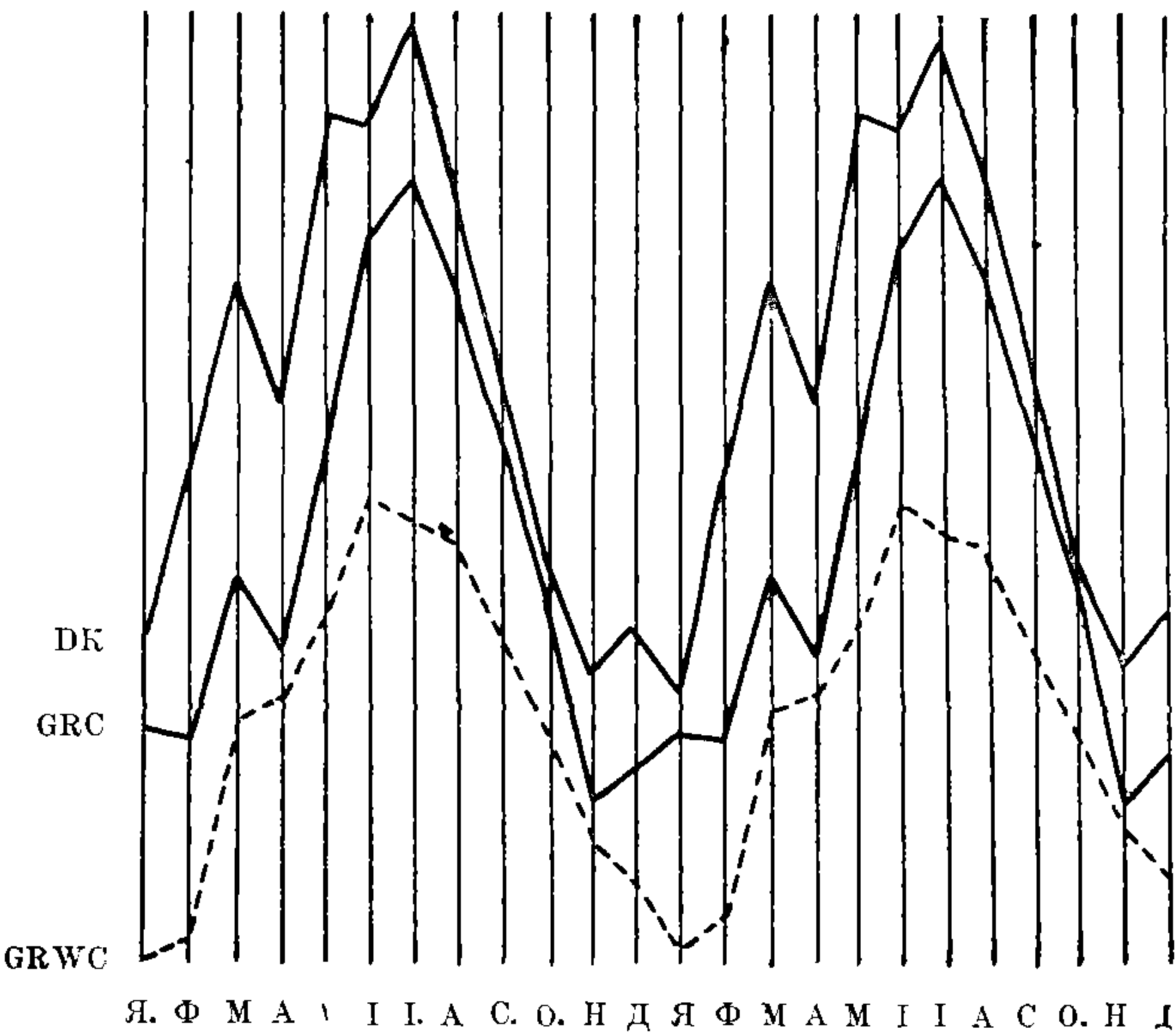
Фиг. 92. Двухгодовой періодъ колебаній уровня Дунайскаго канала (DK) и грунтовыхъ водъ въ Россауской казармѣ (GRC) и въ Реннвегской казармѣ (GRWC) въ Вѣнѣ.
