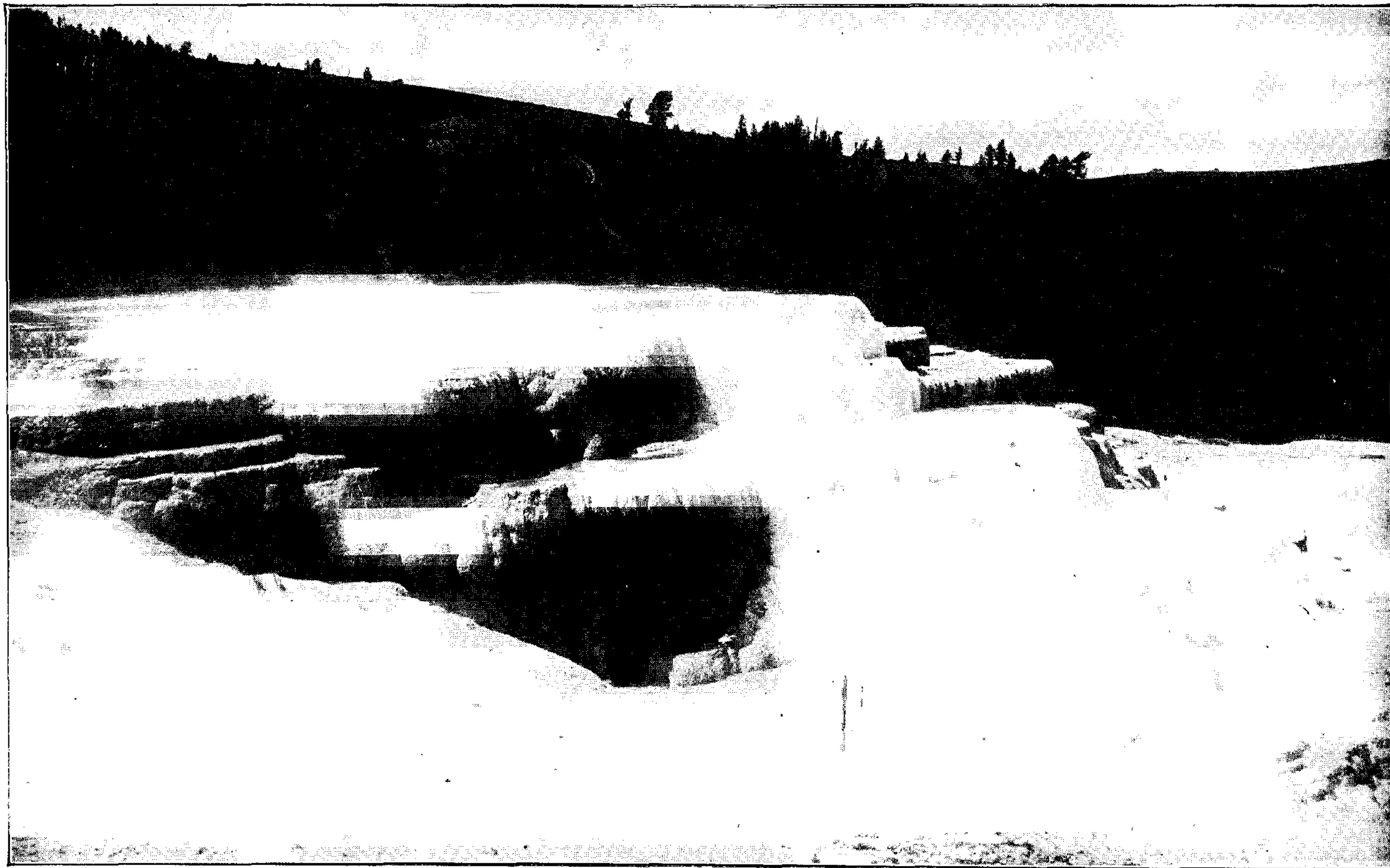
Фиг. 229. Террасы известковаго туфа въ области Мамонтоваго источника (Mammoth Hot Spring) въ Йеллоустонскомъ паркѣ.
