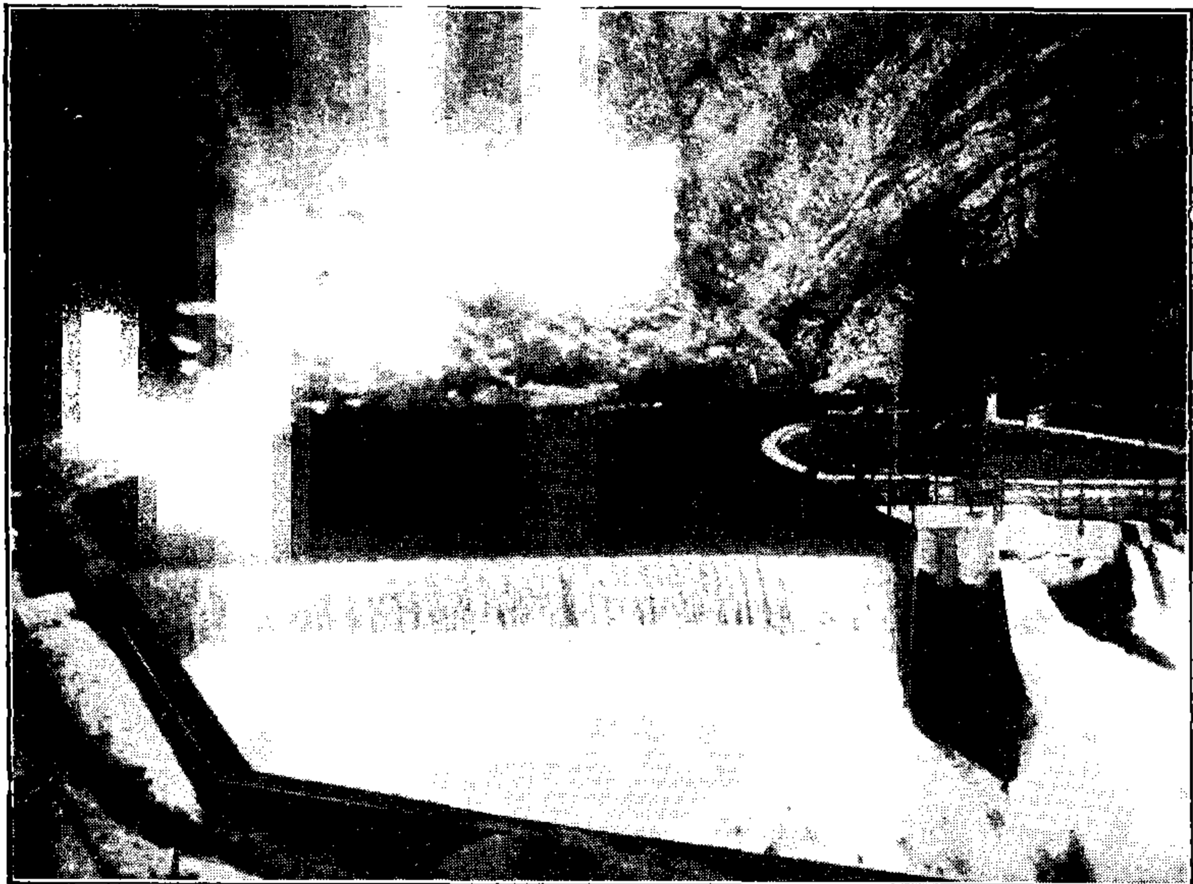
Фиг. 205. Источникъ Areuse (La Doux) близъ С. Сюльписъ, Валь де Траверъ, Невшатель. Трещинный источникъ. Фот. Шардта.
