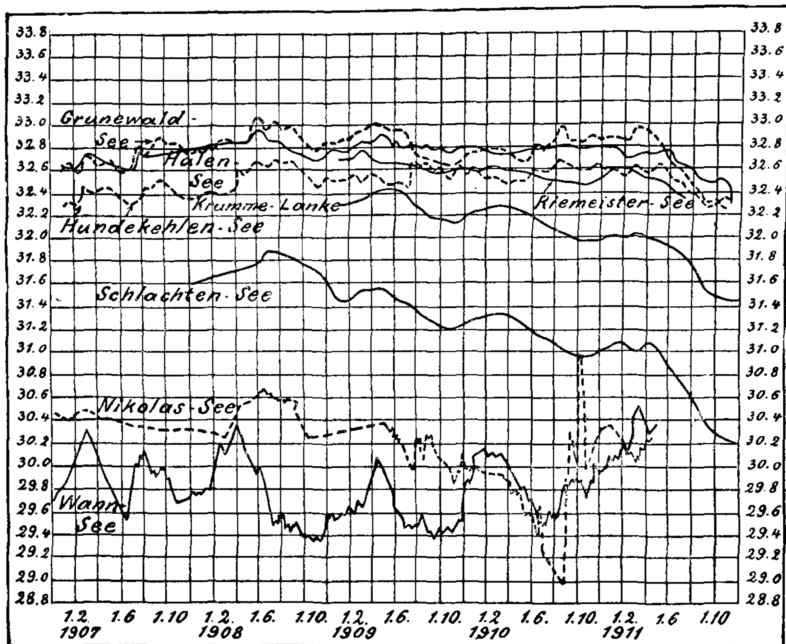
Фиг. 118. Кривыя колебанія зеркала озеръ въ Груневальдѣ близъ Берлина.
