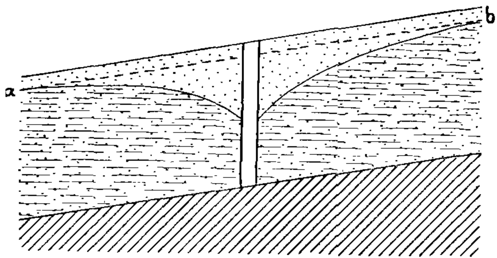
Фиг. 112. Воронка пониженія при сильномъ уклонѣ зеркала грунтовыхъ водъ.
