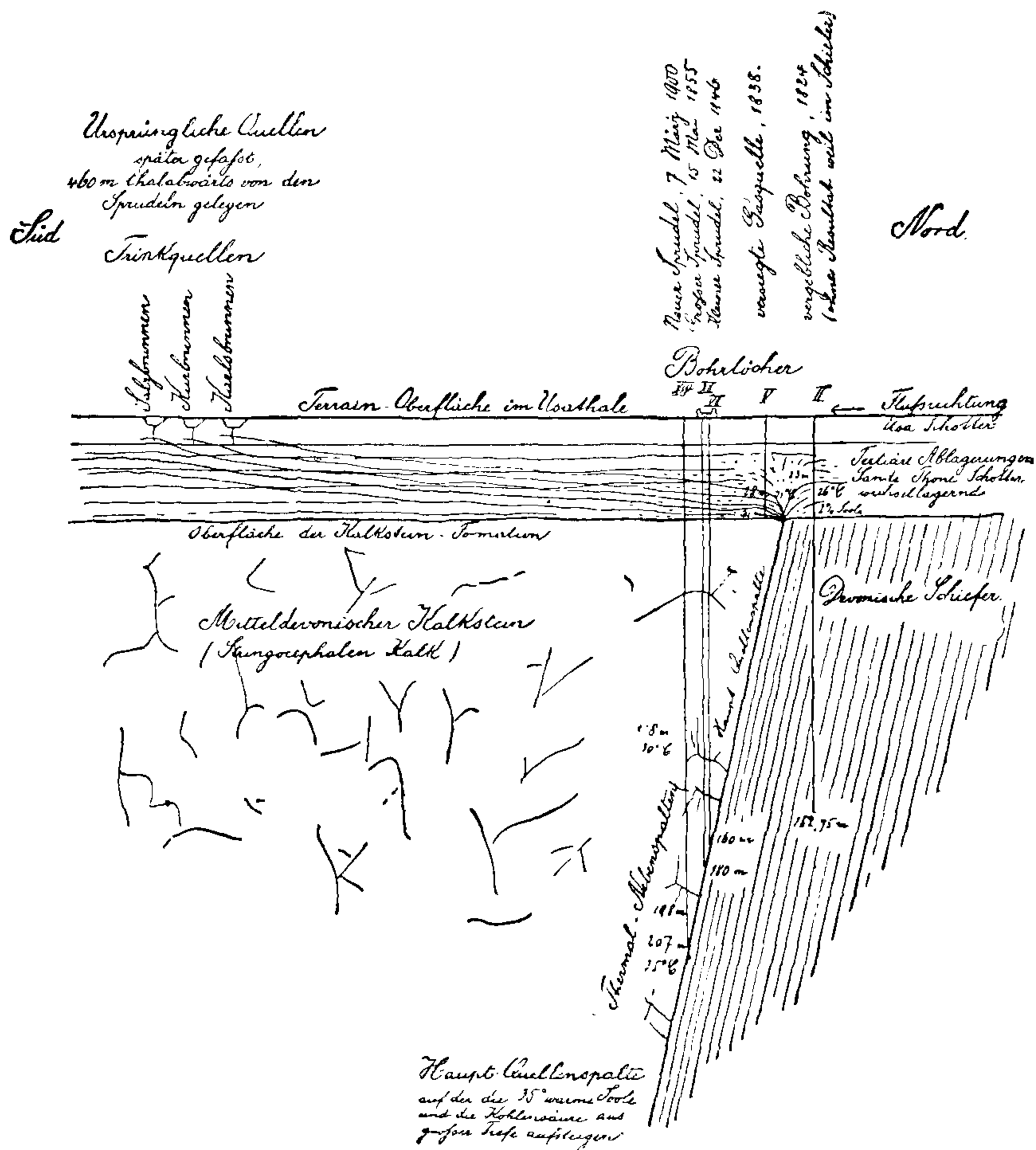
Фиг. 224. Разрѣзъ шпруделя въ Наугеймѣ, по Л е п с і у с у.
