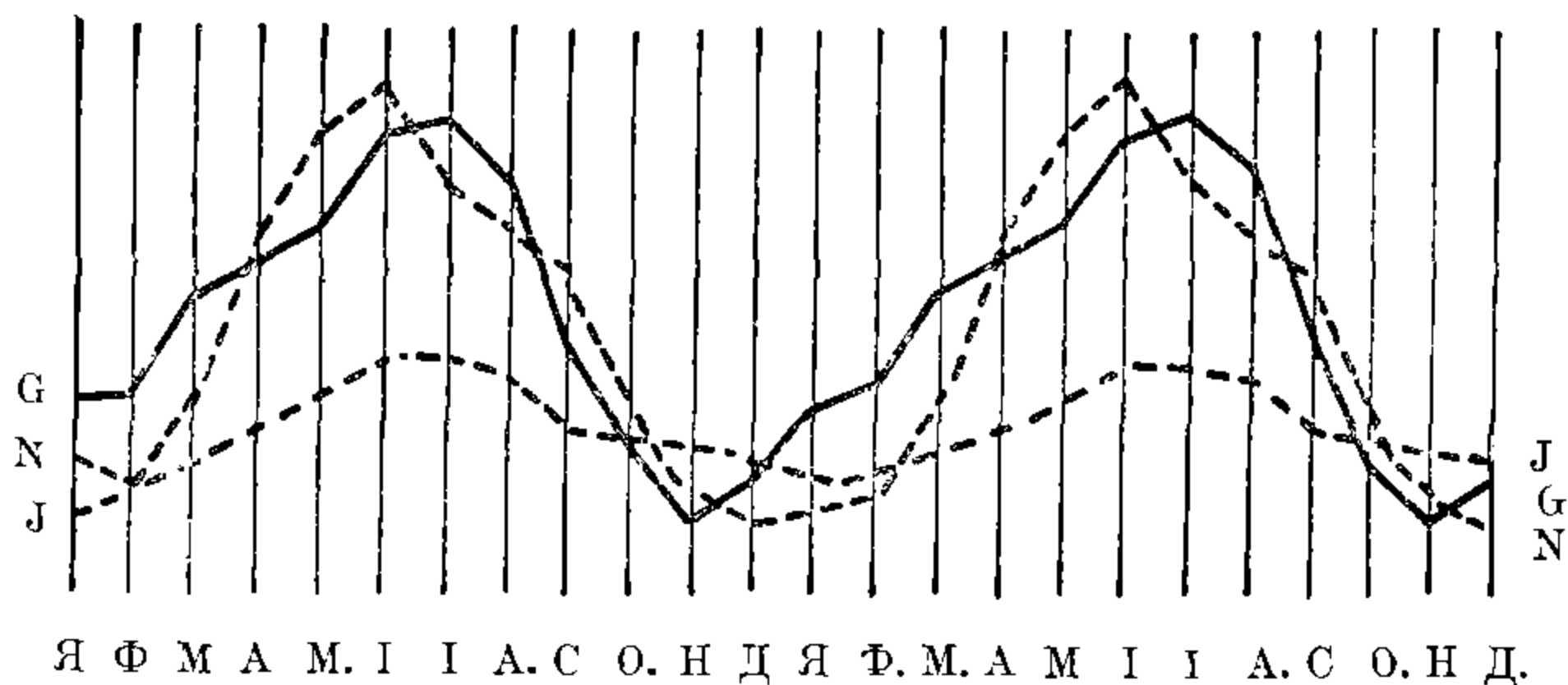
Фиг. 87. Двухгодичный періодъ колебаній грунтовыхъ водъ (G), осадковъ (N) и рѣки Изара въ Мюнхенѣ.
