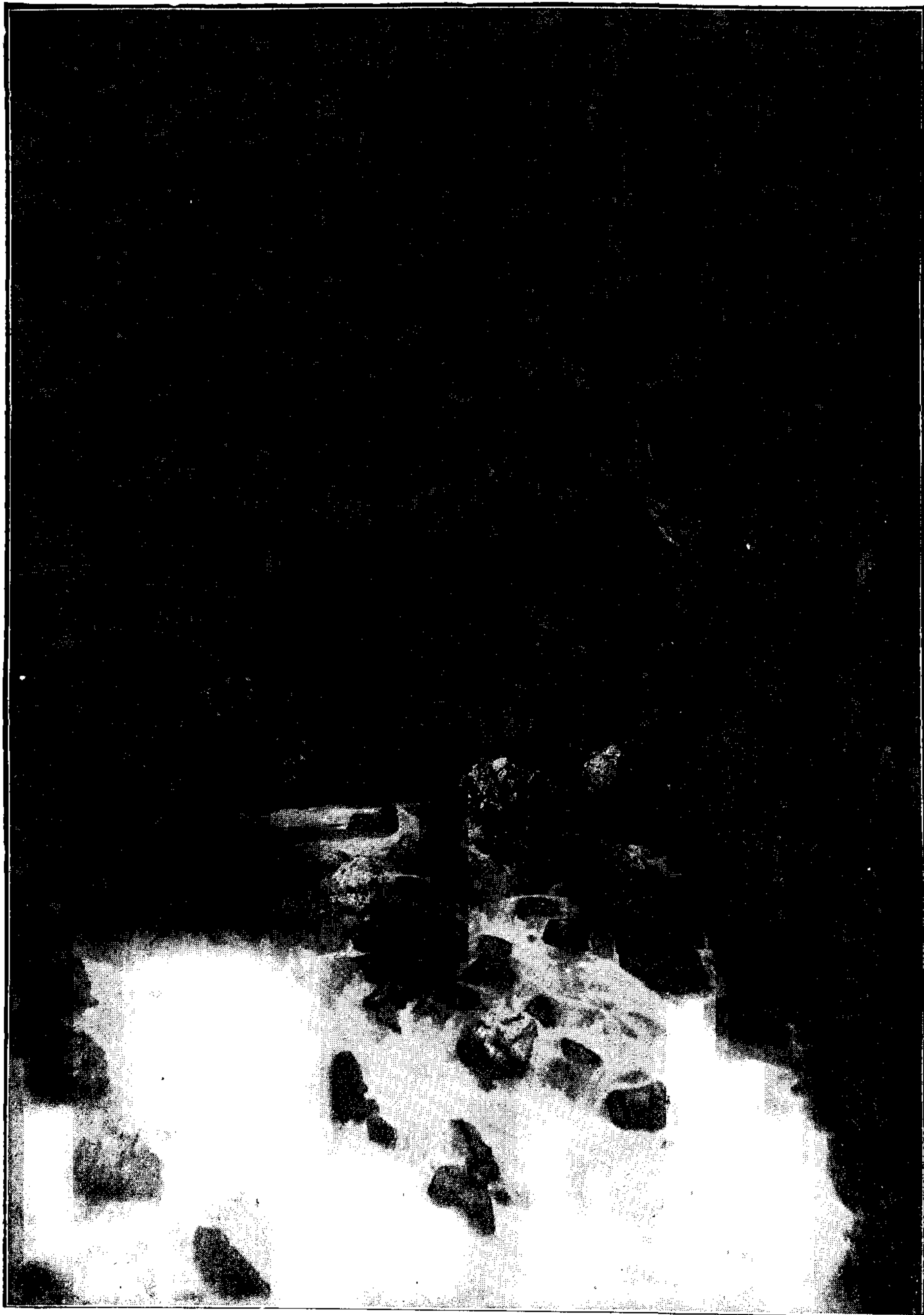
Фиг. 131. Тихальинскій источникъ.
