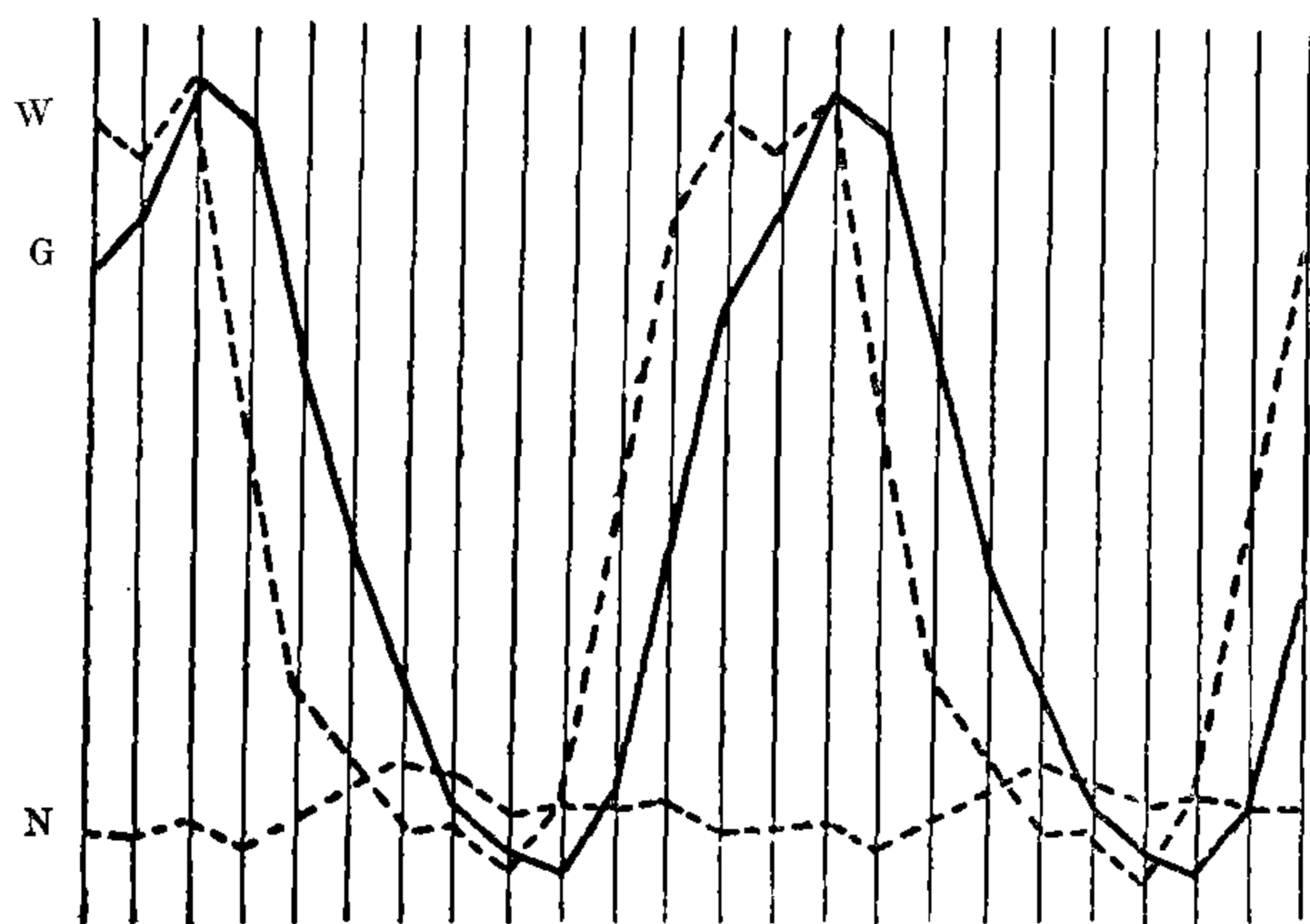
Фиг. 90. Двухгодичный періодъ уровня Везера (W), грунтовой воды (G) и атмосферныхъ осадковъ (N) въ Бременѣ. (Масштабъ Везера относится къ масштабу грунтовыхъ водъ и осадковъ какъ 3,5:1).
