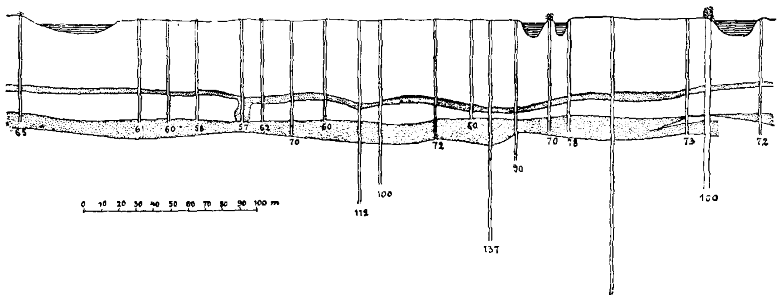
Фиг. 167 (по Добре).
