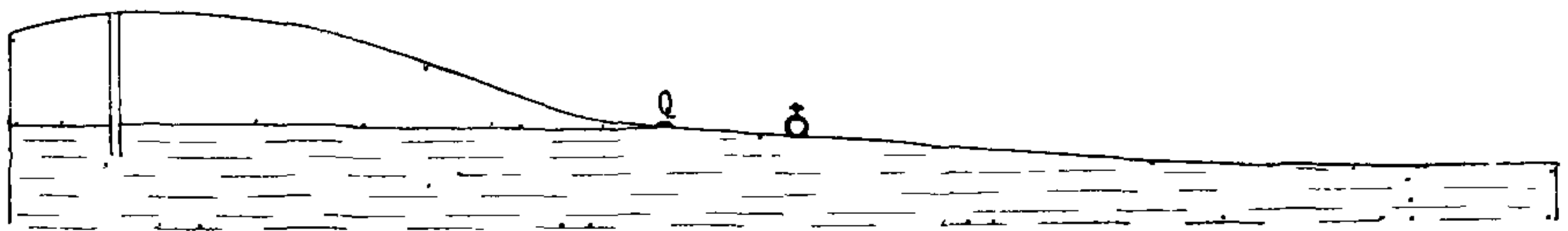
Фиг 76. Водныя условія Флеминга
