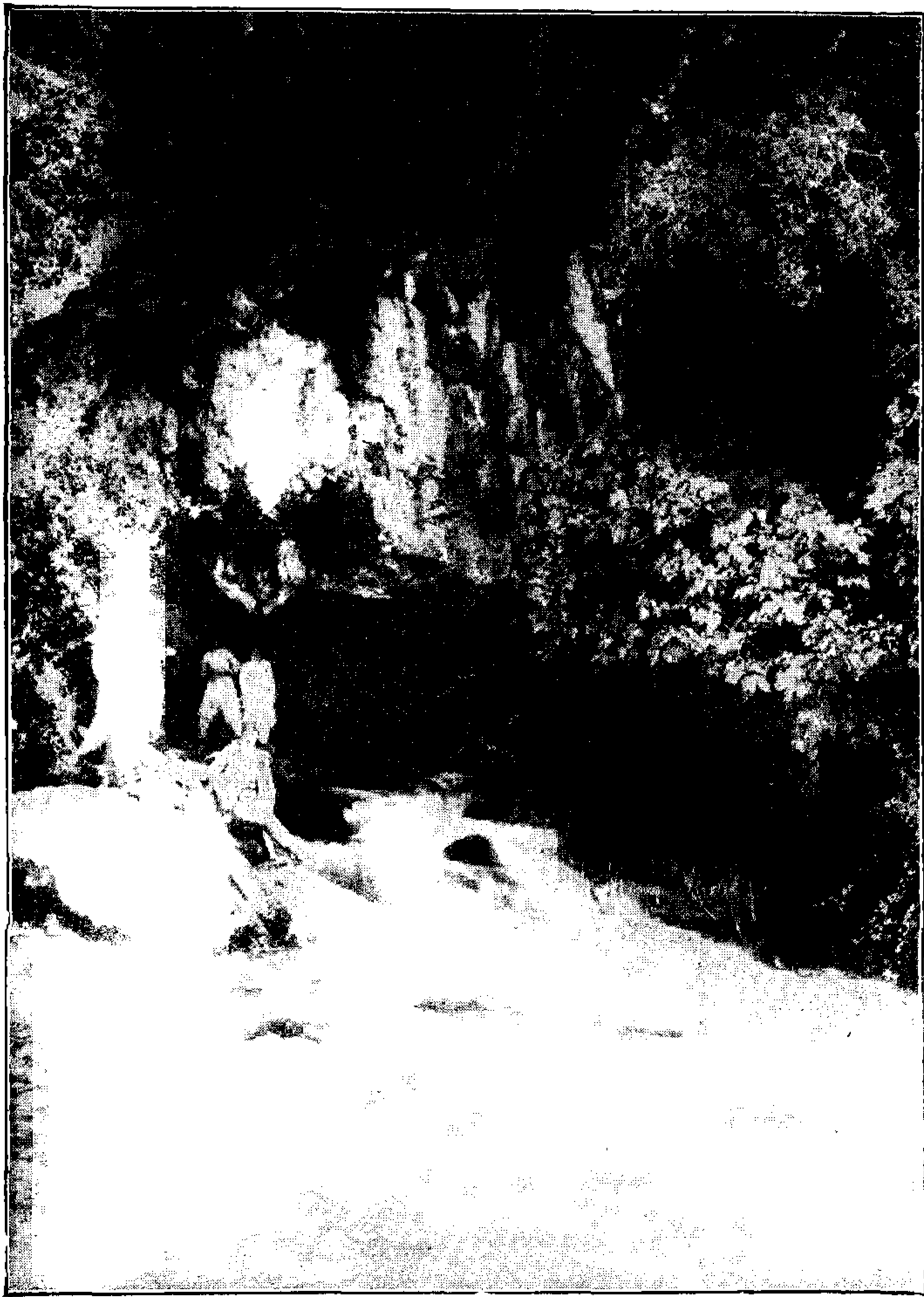
Фиг. 130. Источникъ Вріюштика.
