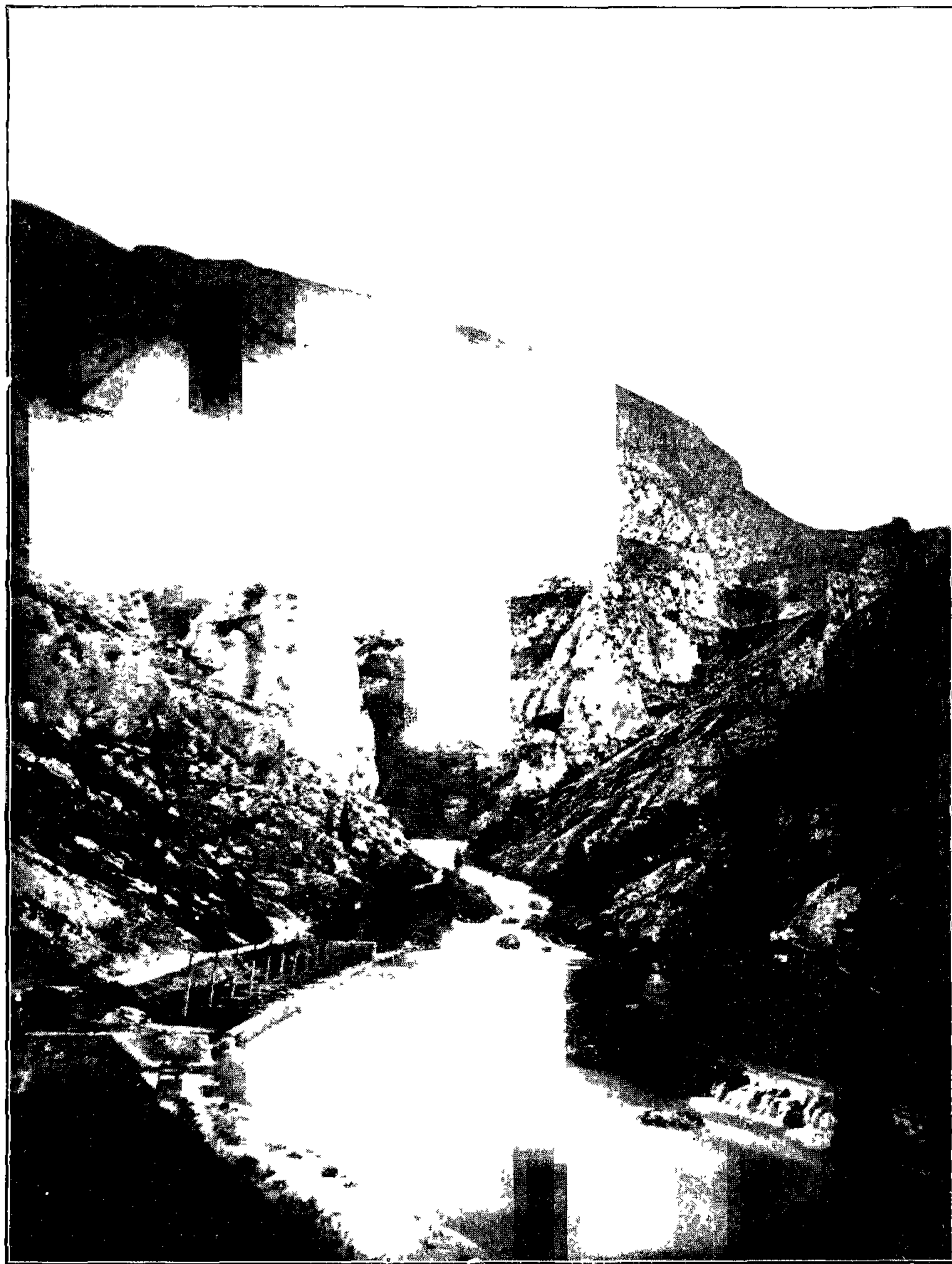
Фиг. 191. Источникъ Воклюзъ.
