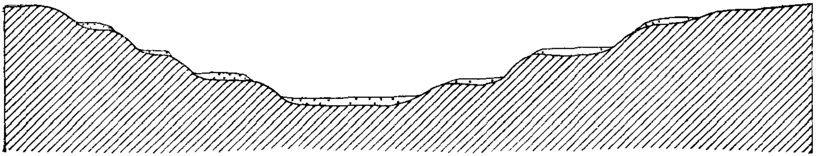
Фиг. 7. Эрозіонныя террасы.
