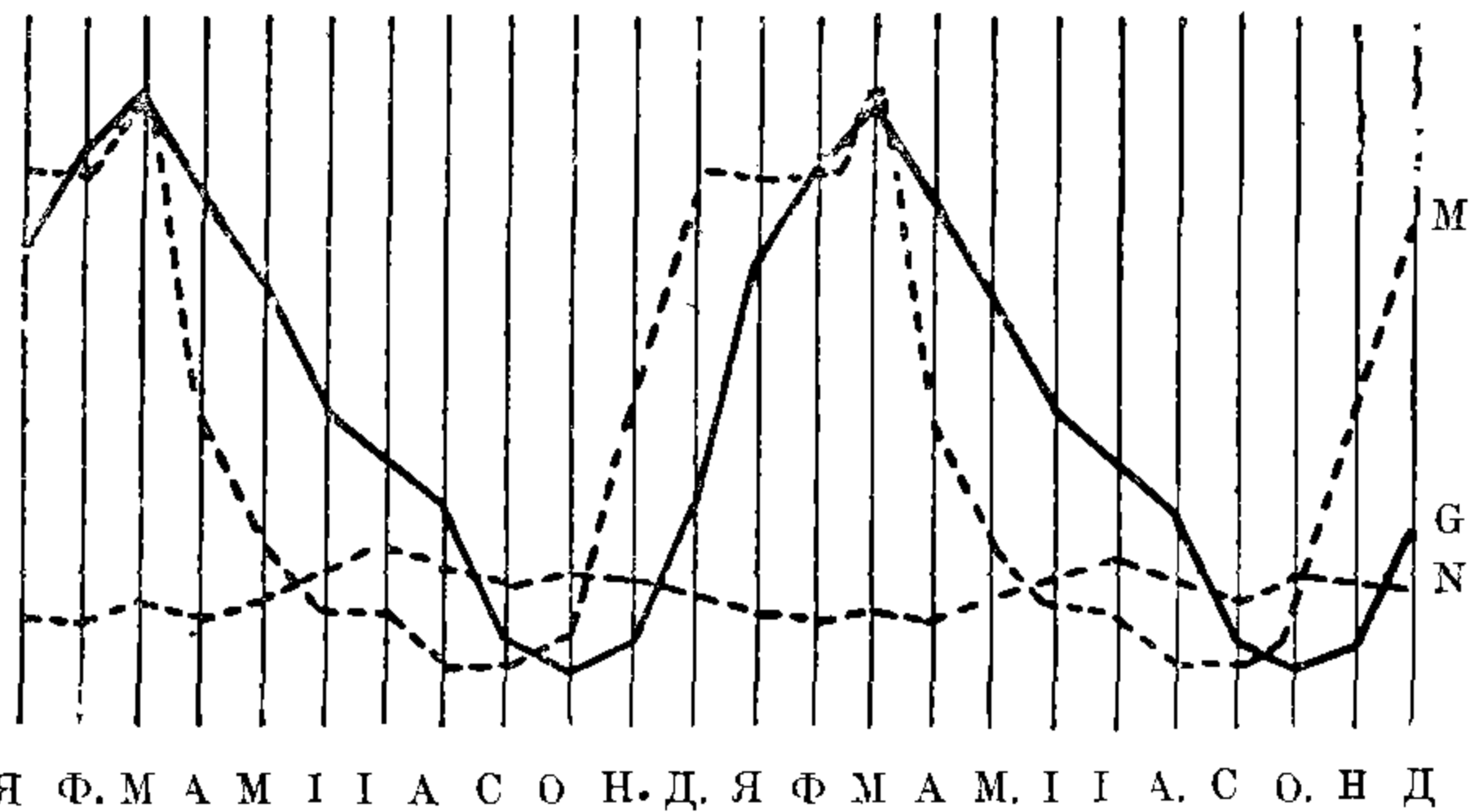
Фиг. 91 Двухго́дичный періодъ стоянія Майна (М), грунтовыхъ водъ (G) и атмосферныхъ осадковъ (N) во Франкфуртѣ на М. Масштабъ стояній Майна относится къ масштабу грунтовыхъ водъ и осадковъ, какъ 2,5 : 1.
