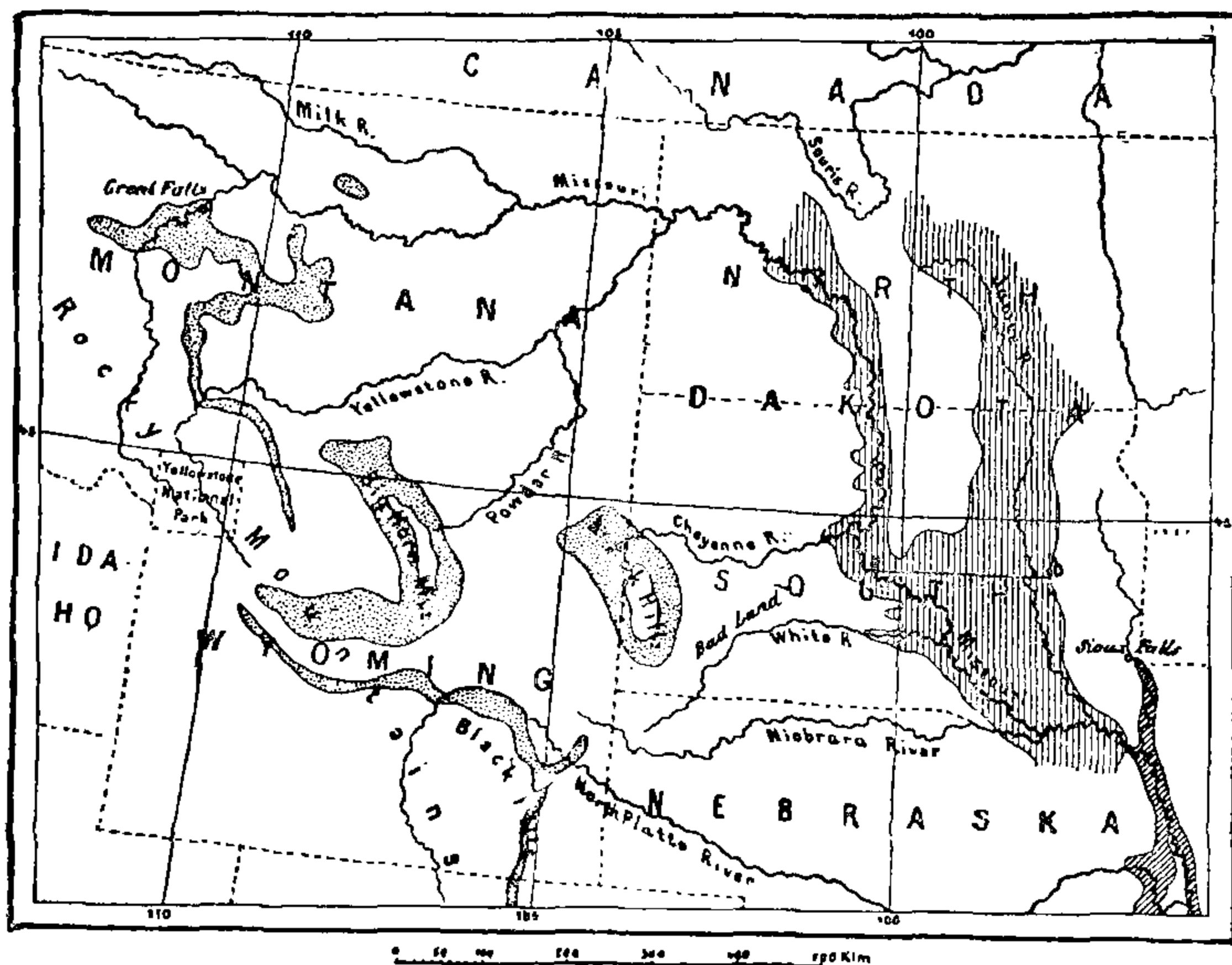
Фиг. 153. Карта выходовъ на поверхность Дакотскаго песчаника въ Скалистыхъ горахъ (площади покрыты точками) и часть артезианскаго бассейна Дакоты съ положительнымъ пьезометрическимъ уровнемъ (вертикальная штриховка).
