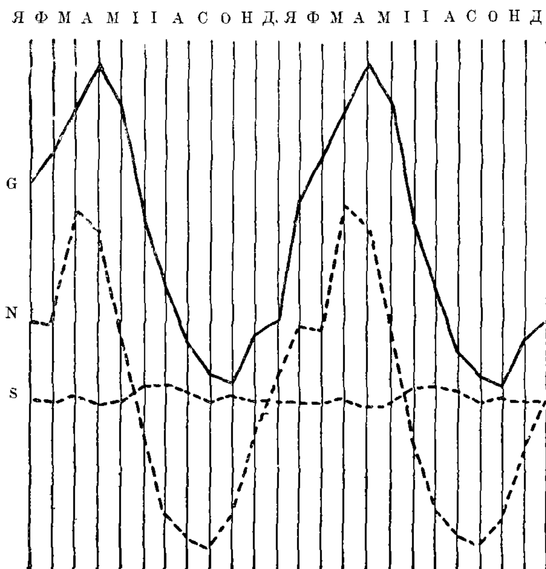
Фиг. 89. Двухгодичный періодъ грунтовыхъ водъ (G), уровня рѣки Шпре (N) и атмосферныхъ осадковъ (S) въ Берлинѣ.
