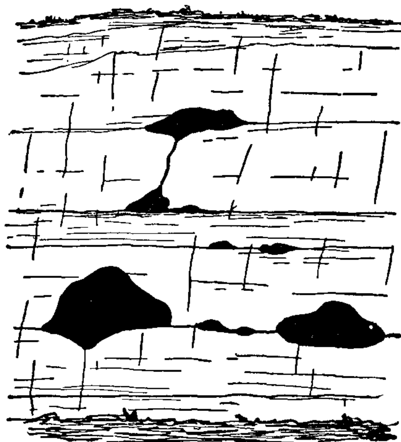
Фиг. 127. Каналы въ слоевыхъ трещинахъ.
