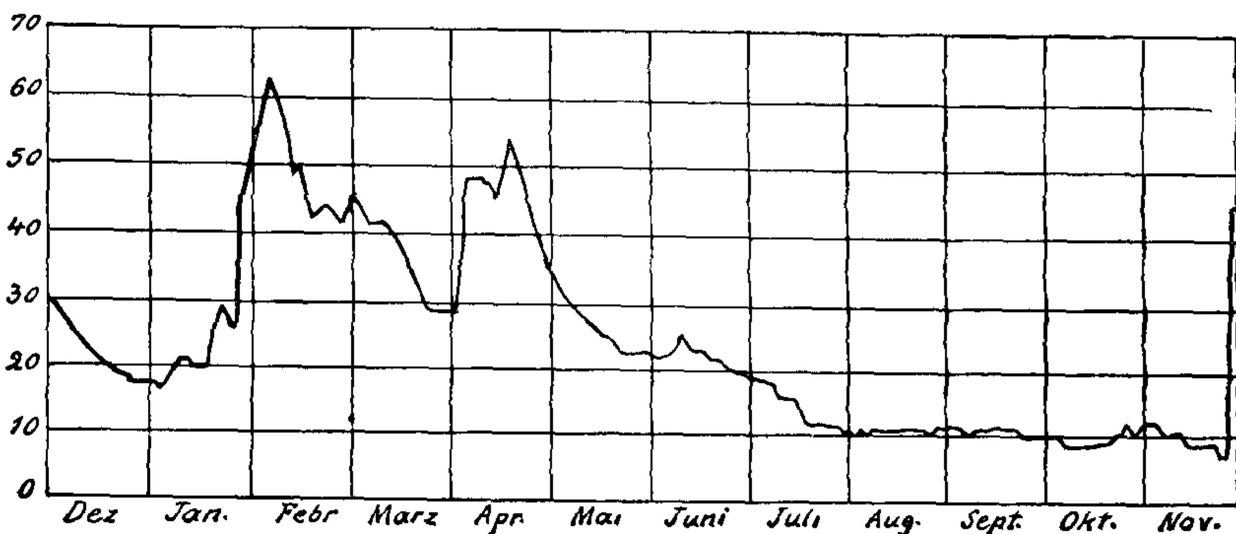
Фиг. 194. Дебитъ источника Воклюзъ въ 1880 г.
