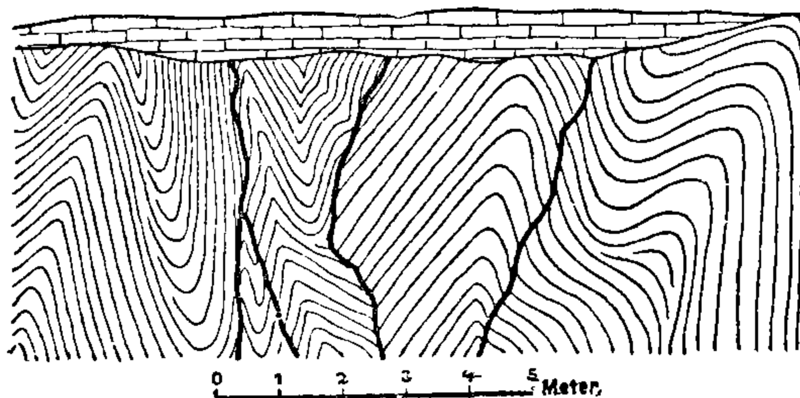
Фиг. 18. Цехштейновые слои, налегающіе на изогнутые кульмскіе кремнистые сланцы (Зап. Гарцъ).
