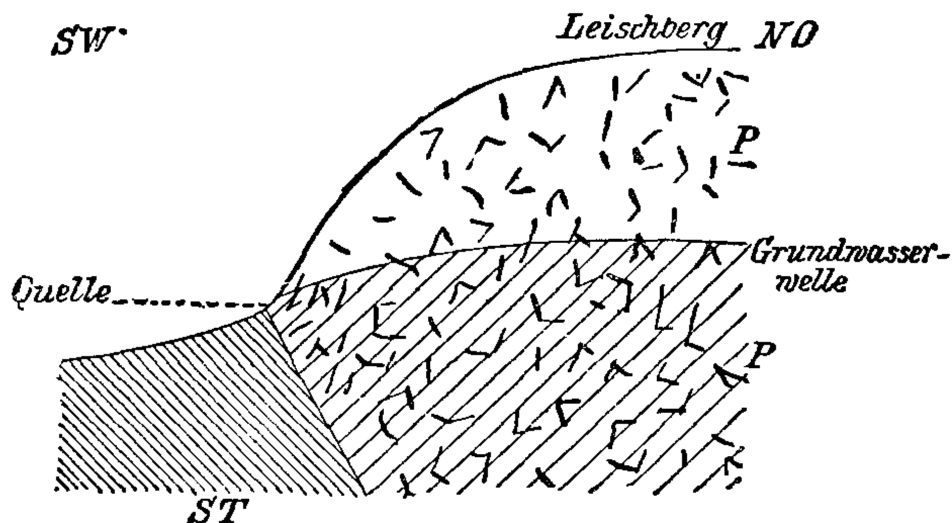
Фиг. 198. ST — слои Tholeyer, P — фельзитовые порфиры.
