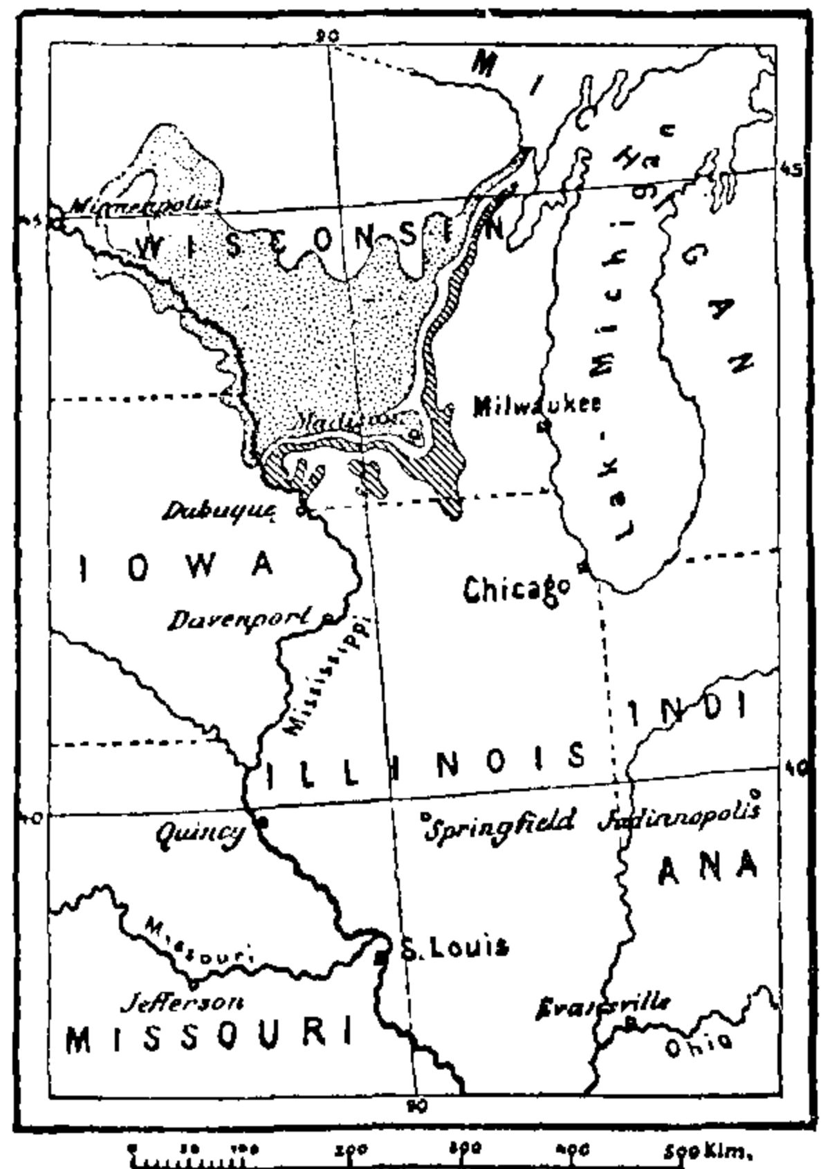
Фиг. 162. Высота кембріійскихъ и силурійскихъ песчаниковъ въ Уисконсинѣ (покрытая точками площадь — кембріійскій, заштрихованная — силурійскій песчаникъ).
