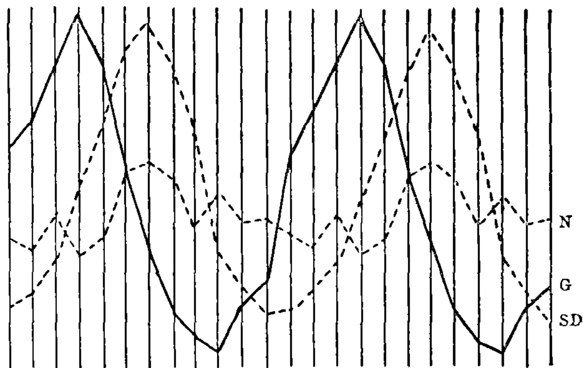
Фиг. 94. Двухгодовой періодъ грунтовыхъ водъ (G), осадковъ (N) и недостатка насыщенія (SD) въ Берлинѣ.
