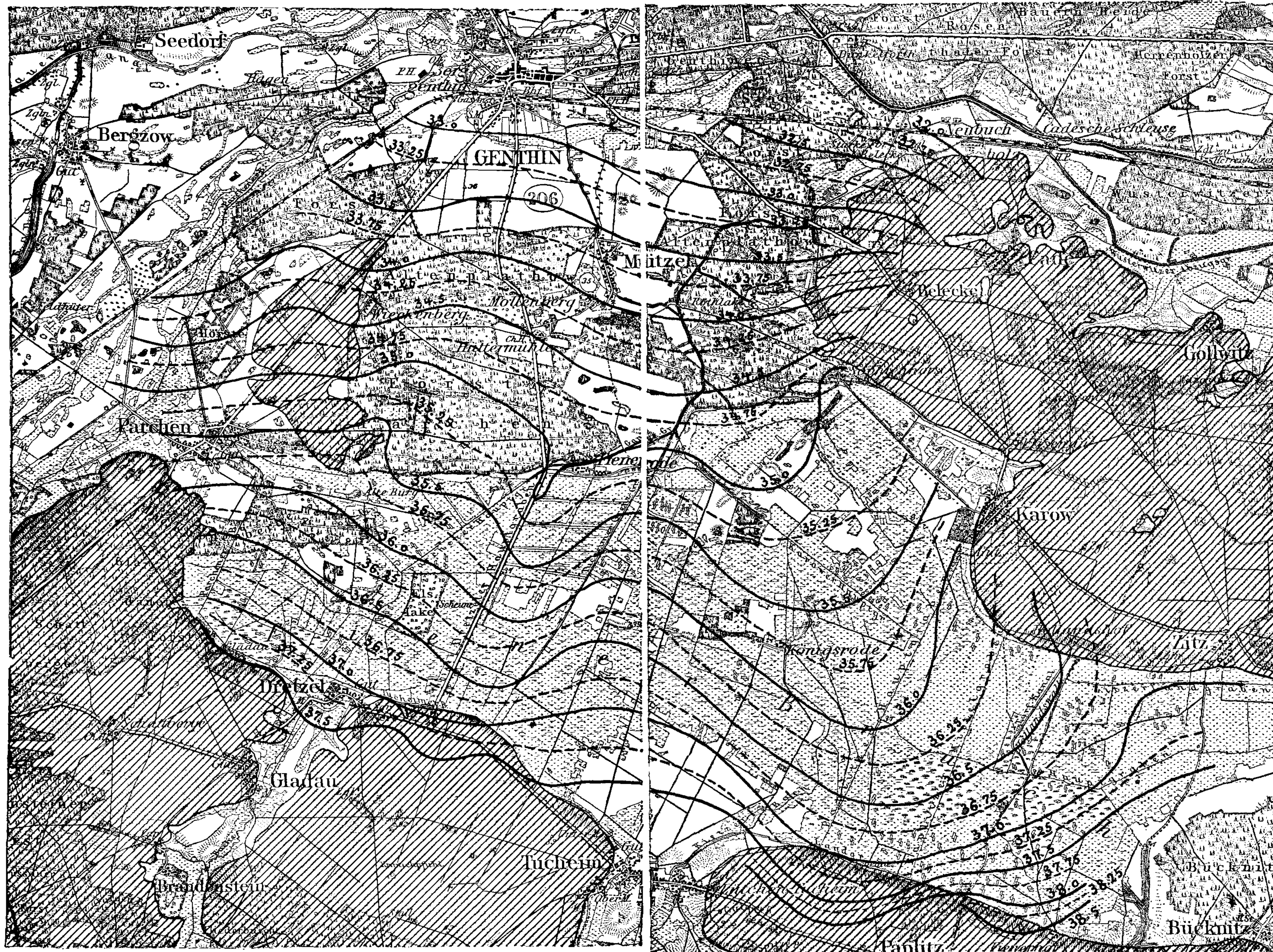
Фиг. 53. Горизонталы уровня грунтовых водъ через \frac{1}{4} м. въ области Фиерер Bruch. Масштабъ 1 : 100000.
