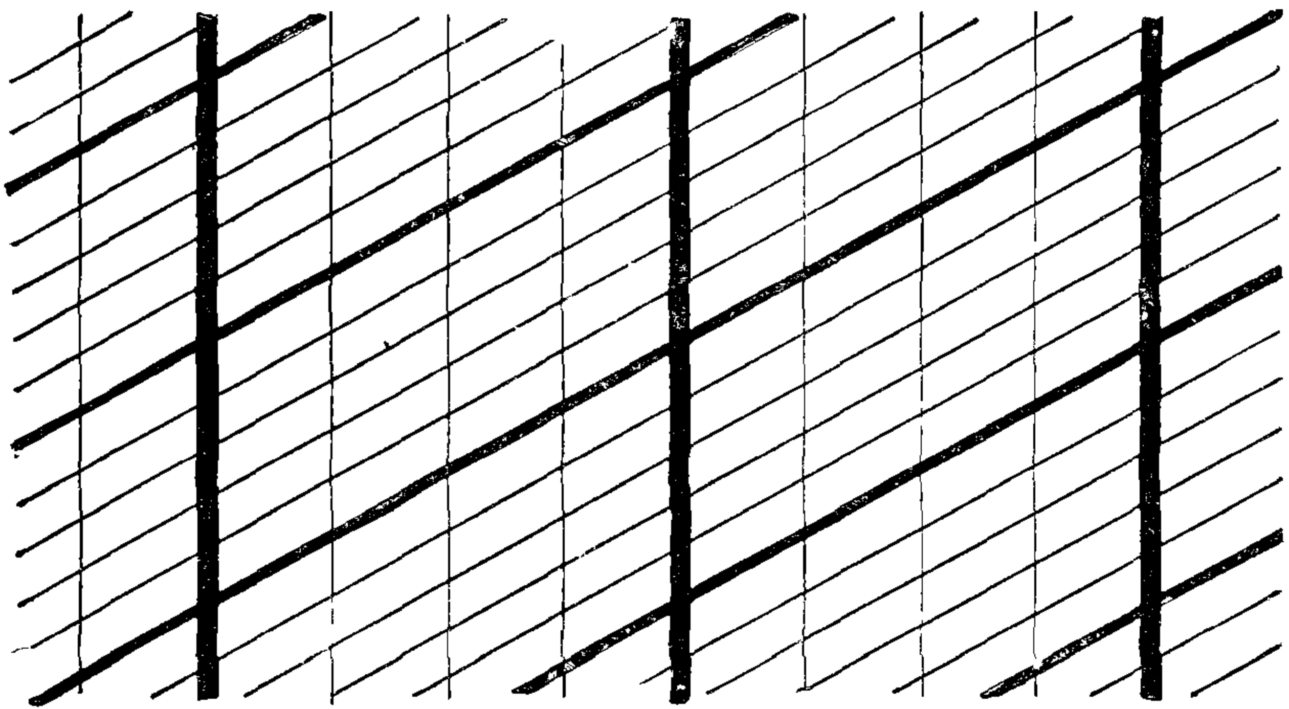
Фиг. 32. Система трещинъ въ раковистомъ известнякѣ Бернбурга
