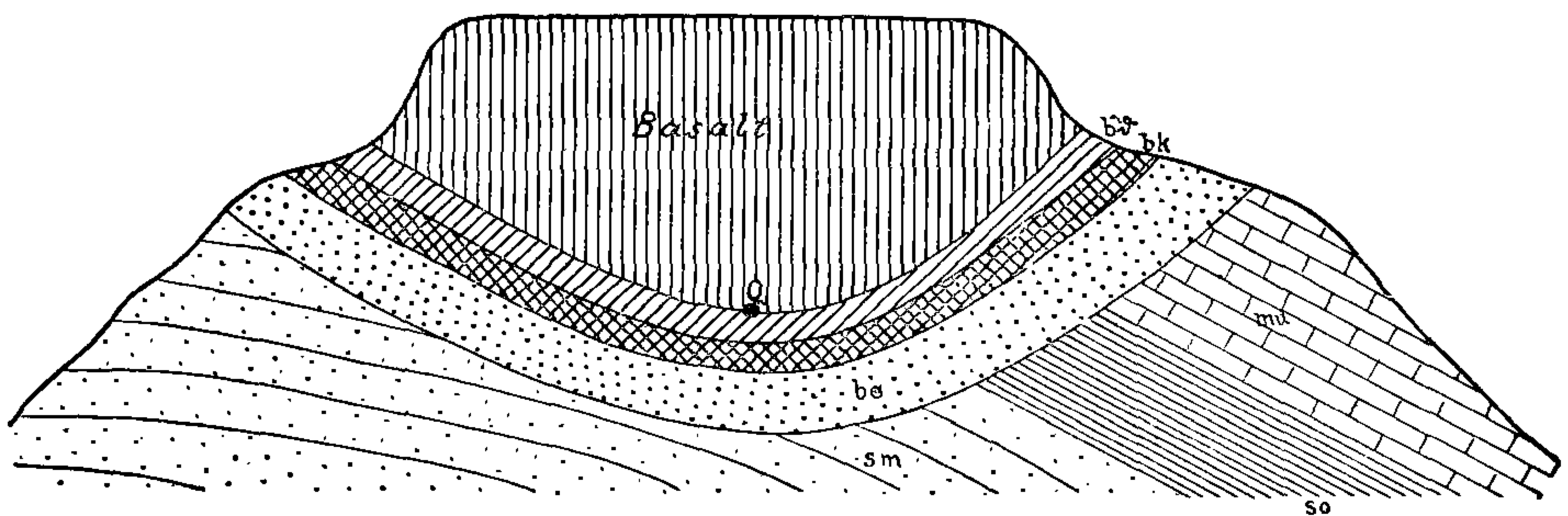
Фиг. 199. Переливающийся источникъ въ массивѣ Мейсснера.
