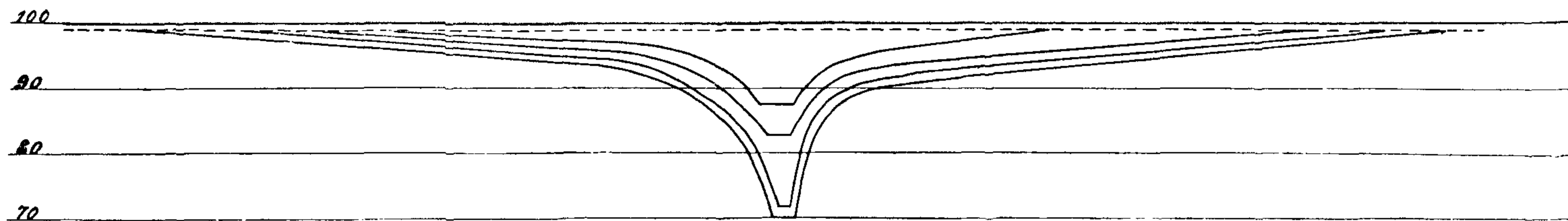
Фиг. 116. Поперечный разръзъ четырехъ воронокъ пониженія фиг. 114.
