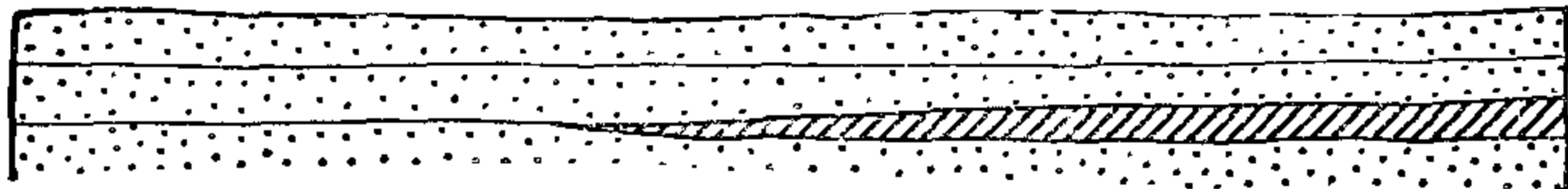
Фиг. 14. Выклиниваніе.
