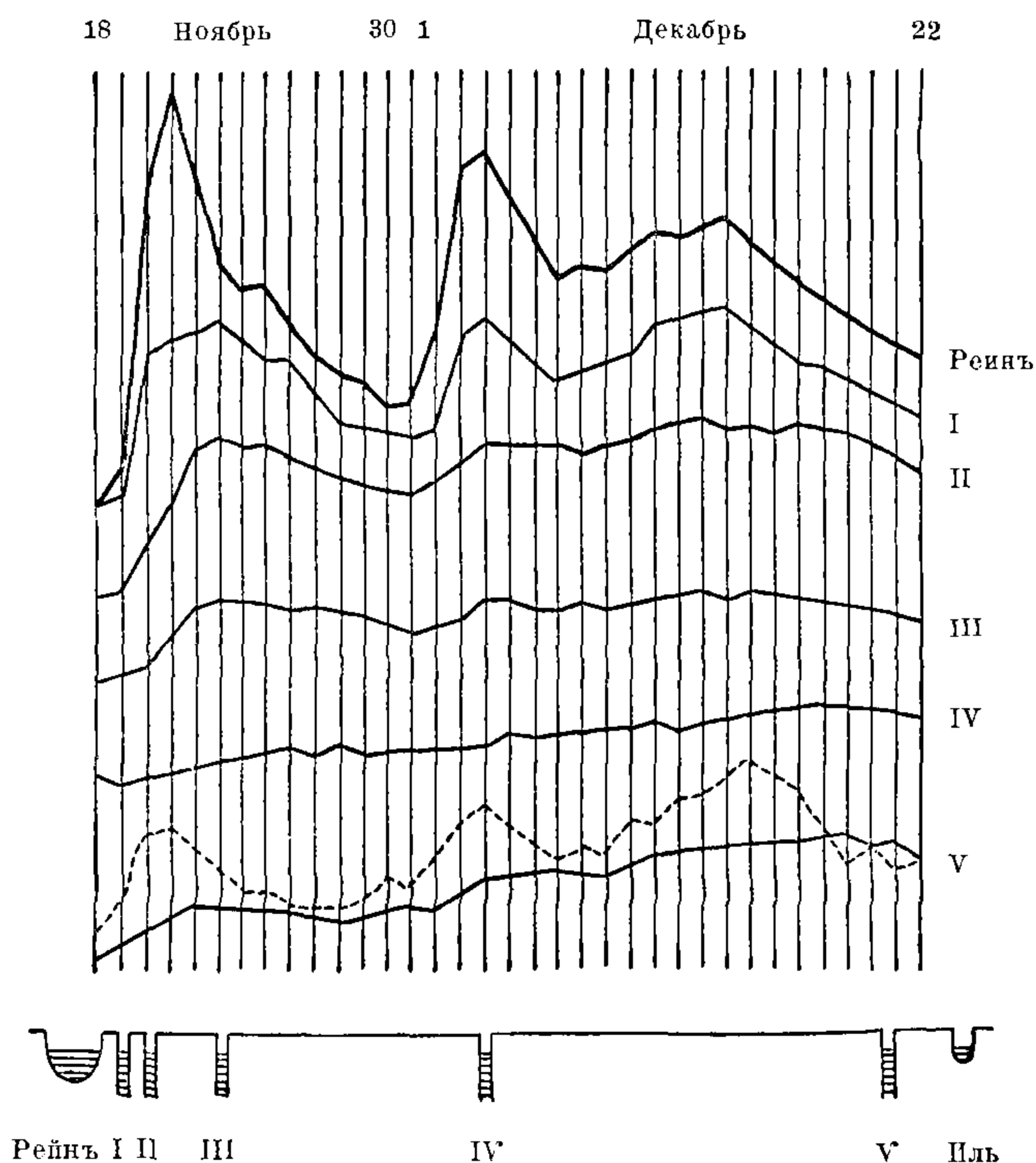
Поперечный профиль отъ Рейна къ Илю съ уровнями грунтовыхъ водъ.
