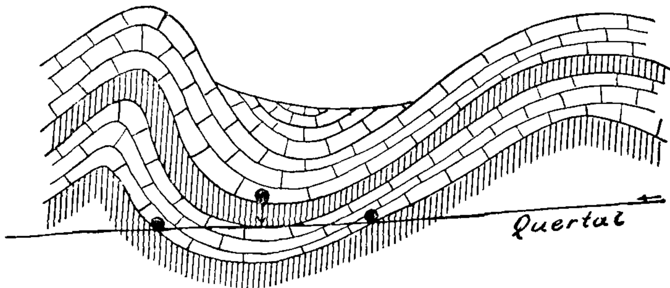
Фиг. 186 (по А. Гейму).
