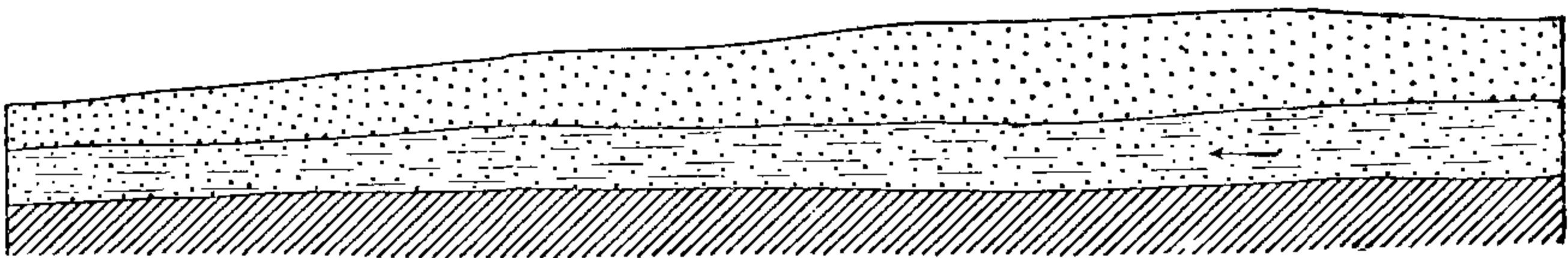
Фиг. 61. Потокъ грунтовой воды.
