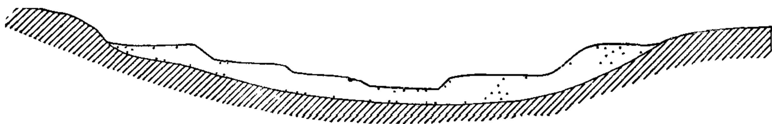
Фиг. 9. Долинные террасы.
