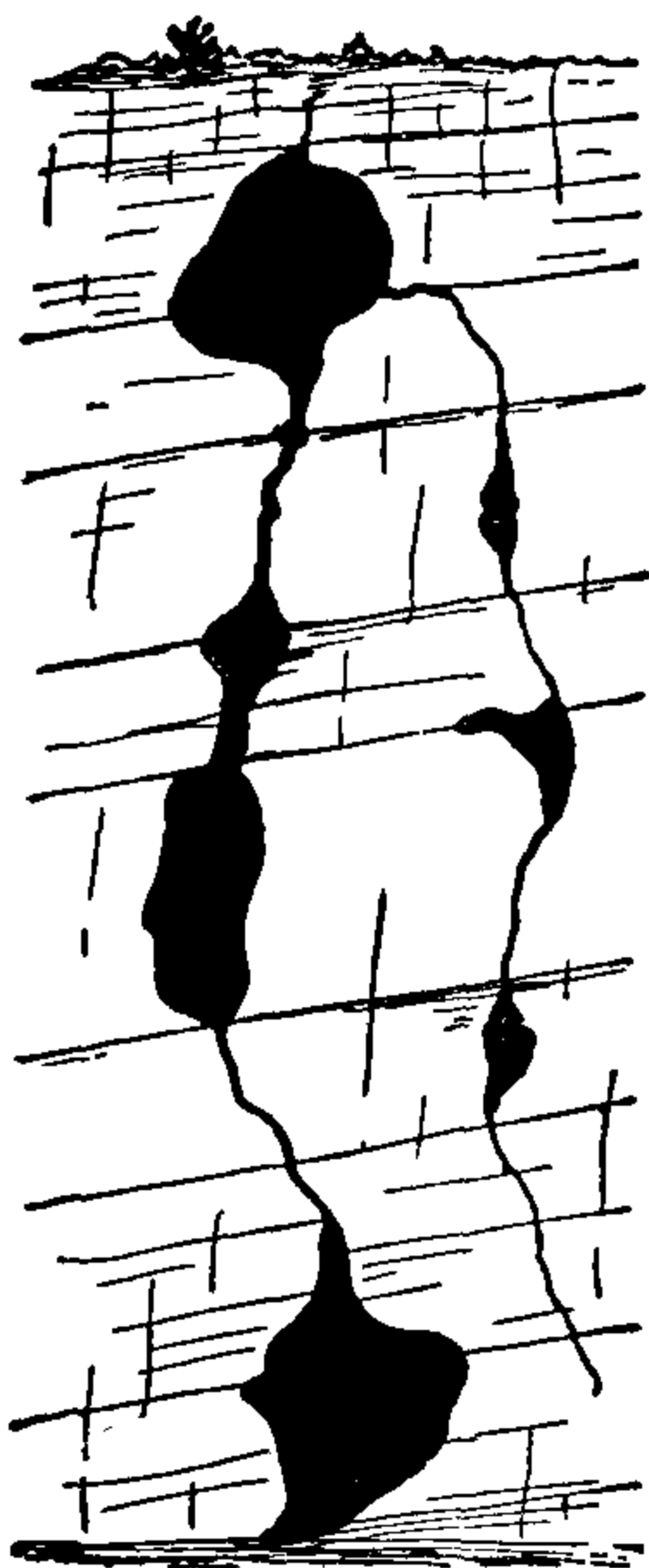
Фиг. 126. Трещинный каналъ.
