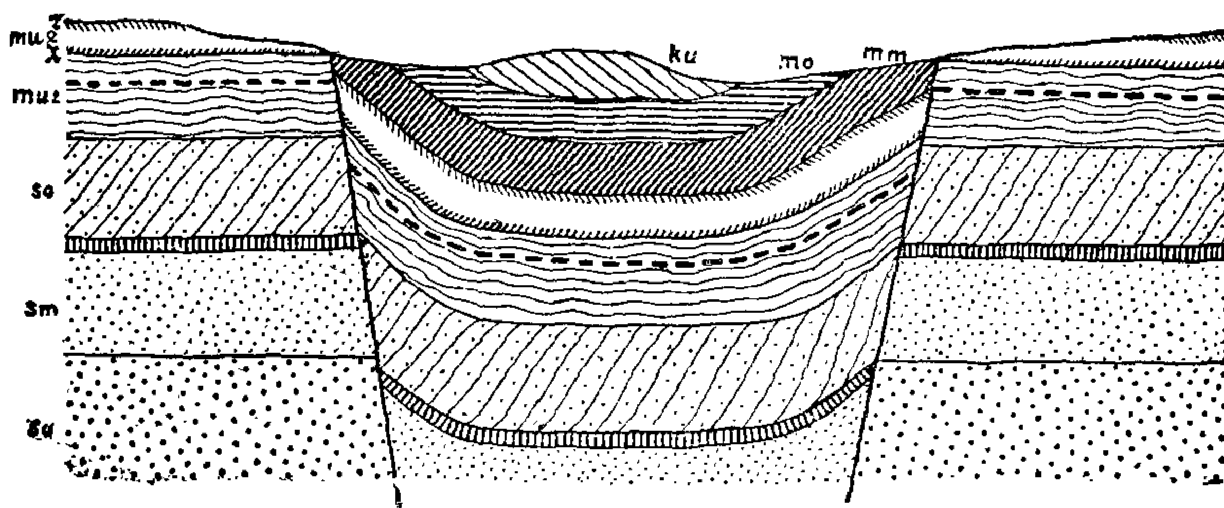
Фиг. 43. Простой грабенъ.
