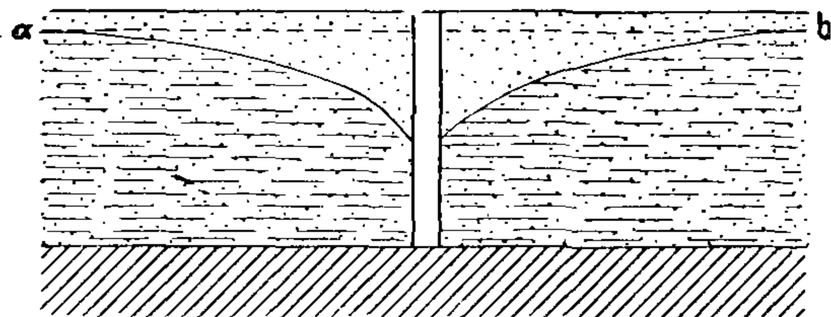
Фиг. 111. Воронка пониженія при ровной поверхности грунтовыхъ водъ.
