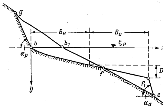
Рис. 39. Формирование береговой линии водохранилища ( z_p — расчетный уровень).
