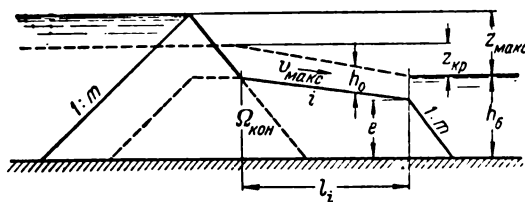
Рис. 50. Расчетная схема для приближенного определения единичного объема наброски, вышедшей из воды.
