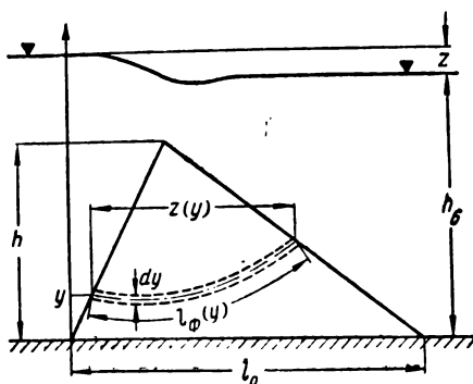
Рис. 55. К определению фильтрационной способности наброски.
