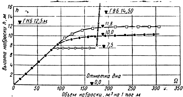
Рис. 33. Сравнение роста кубатуры наброски на 1 пог. м фронта в зависимости от типа материала наброски: каменной, массивовой и каркасной при q = 11 м 2 /сек.
