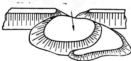
Рис. 39. Характер расположения материалов на- броски в плане при пионерном методе перекрытия русел.
