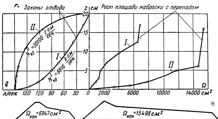
Рис. 11. Сопоставление площадей и профилей наброски в зависимости от закона изменения удельного расхода (отвода расхода).
