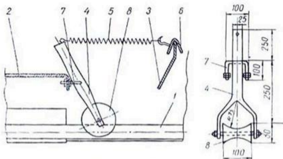
Рис. 6. Прижимное приспособление:
