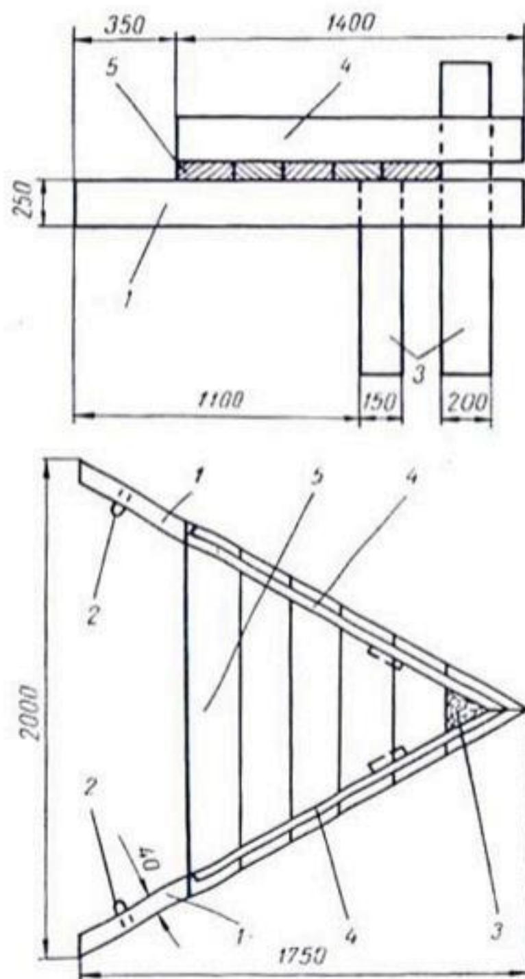
Рис. 7. Присыпающее устройство:
