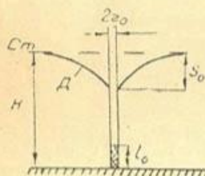
Рис. 15. Схема несовершенного колодца; C_m — статический уровень подземных вод; Д — динамический уровень подземных вод.
