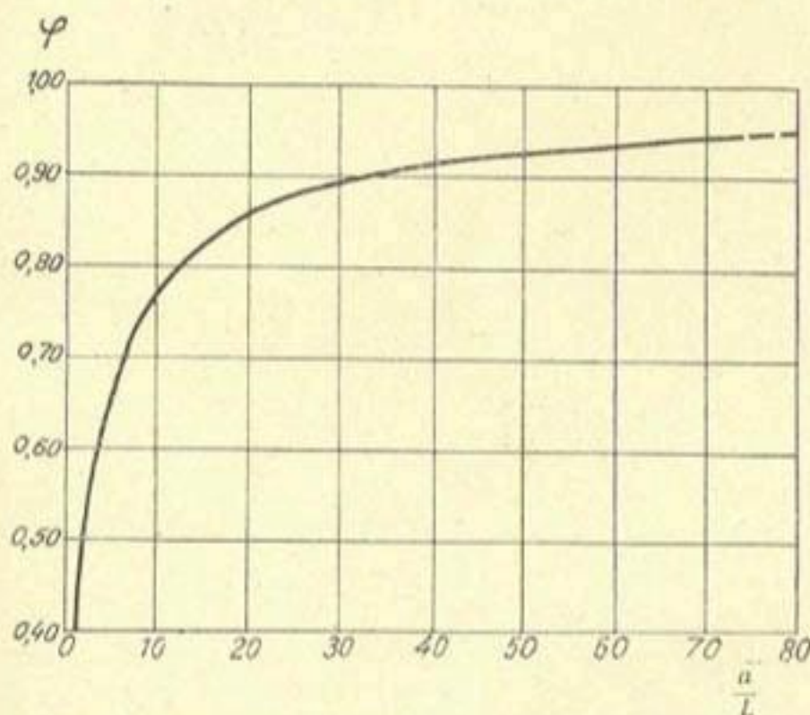
Рис. 3. График для определения поправочного коэффициента \varphi = f\left(\frac{a}{L}\right) к формуле притока в длинную совершенную траншею или котлован.
