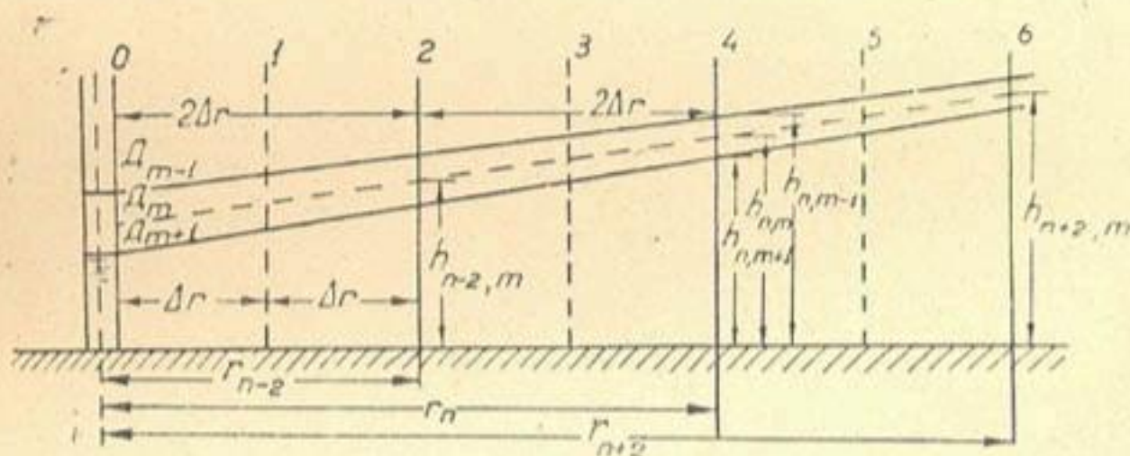
Рис. 4. Схема к расчету неустойчивого радиального потока безнапорных вод к одиночному совершенному колодцу методом конечных величин: 0, 2, 4, 6 — основные сечения; 1, 3, 5 — промежуточные сечения; D_{m-1} , D_m , D_{m+1} — положение депрессионных поверхностей, соответствующее расчетным интервалам времени m-1 , m , m+1 .
