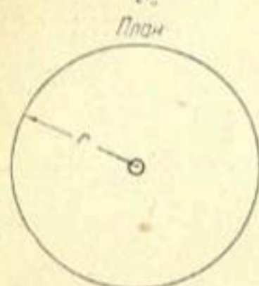
Рис. 5. Схема к расчету неустановившегося радиального потока безнапорных вод к одиночному совершенному колодезю по аналитическим формулам Соколова: 1—первоначальное положение уровня подземных вод; 2—положение депрессионной поверхности в момент времени t (от начала откачки).
