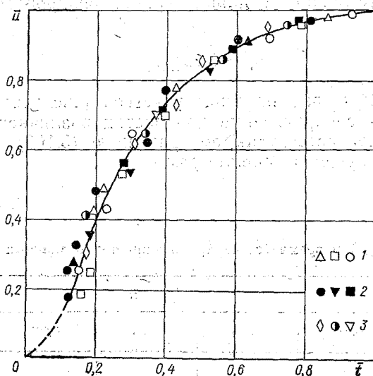
Рис. 5.16. Зависимость \bar{u} = \bar{u}(\bar{t}) на участке синхронизации в каналах разных сечений при различных диаметрах частиц d_T .
