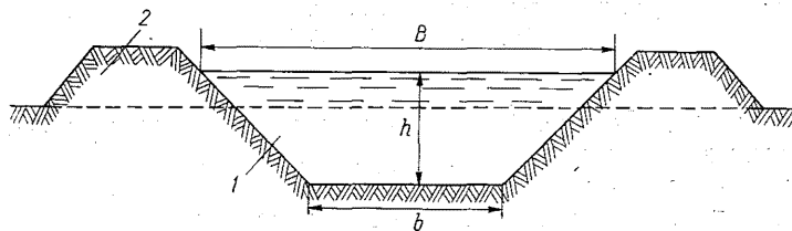
Рис. 1.3. Трапецеидальное поперечное сечение канала в полувыемке-полунасыпи.
