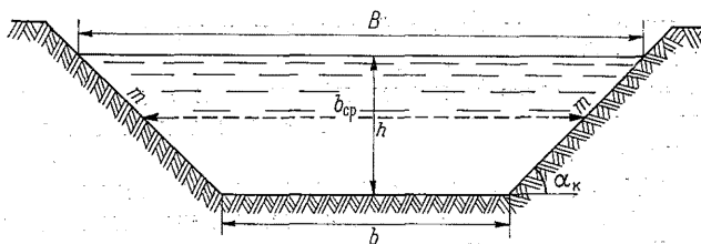
Рис. 1.1. Трапецеидальное поперечное сечение канала.
