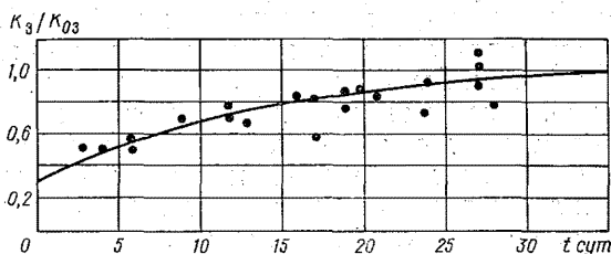
Рис. 7.10. Изменение K_3/K_{03} в зависимости от числа суток после ледостава t , р. Ока у г. Калуги.
