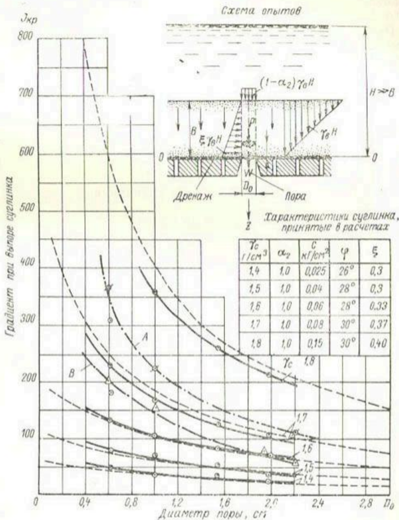
Рис. 18. Графики зависимостей между критическим градиентом фильтрационного потока и диаметром отверстия при контактном выпоре лессового суглинка с оптимальной начальной влажностью W_n = 16-18\% :
