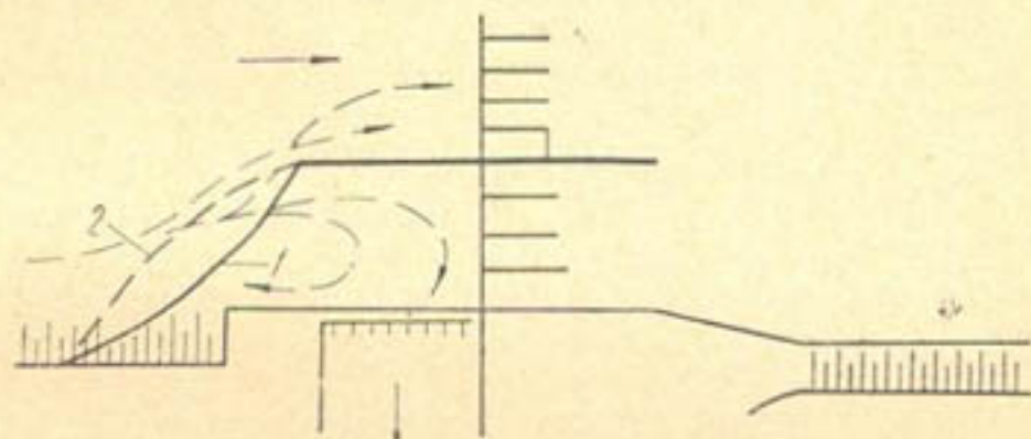
Рис. 58. Два варианта наносоотбойного порога промывного кармана головного регулятора:
