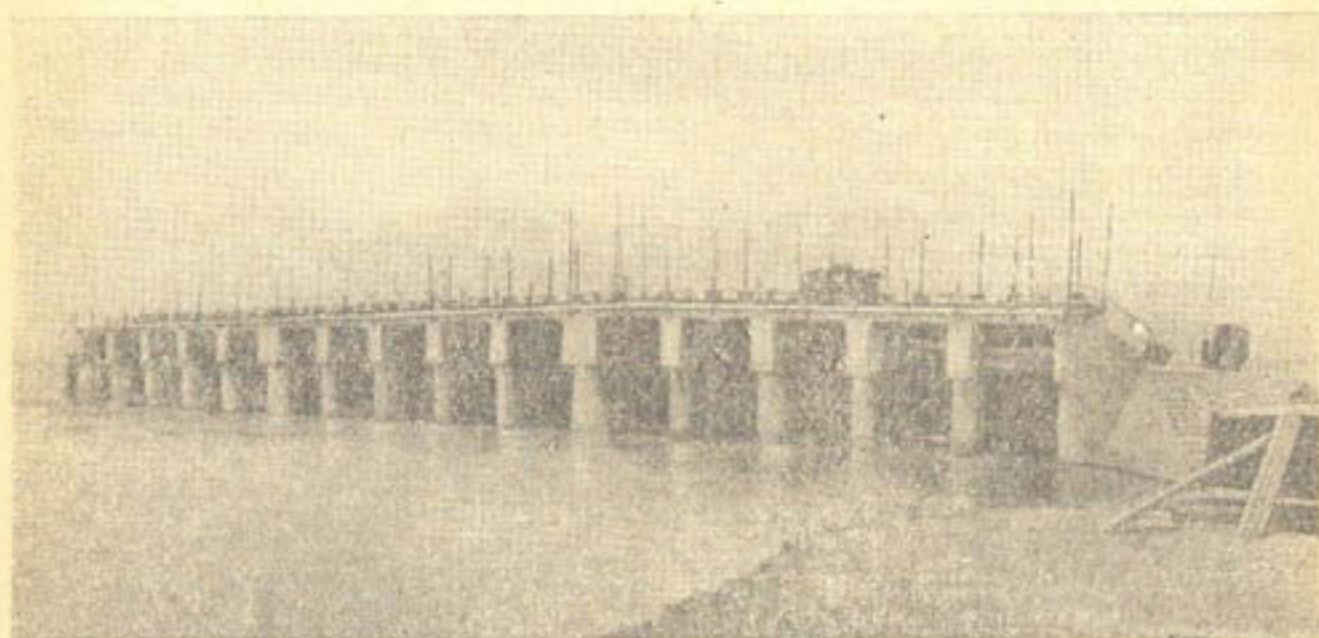
Рис. 29. Головной регулятор Кызкеткен на Амударье у Тахиаташа.
