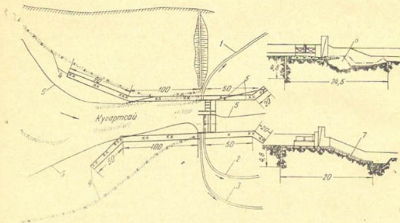
Рис. 4. Схема водозабора на Кугартсае, КиргССР:
