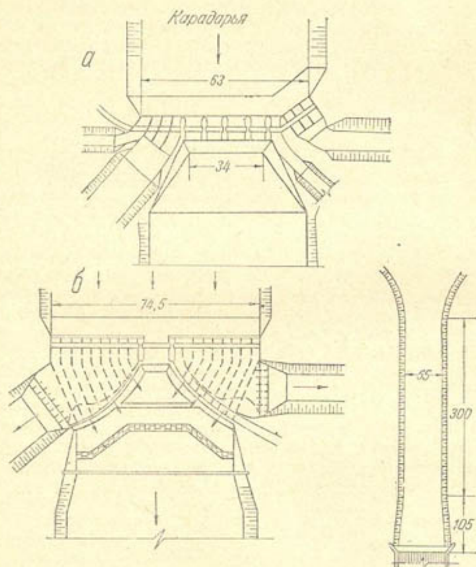
Рис. 19. Первоначальные варианты Дамходжинской плотины: а — Верхнеизарский тип водозабора; б — центральный двухсторонний водозабор С. И. Зиновьева.
