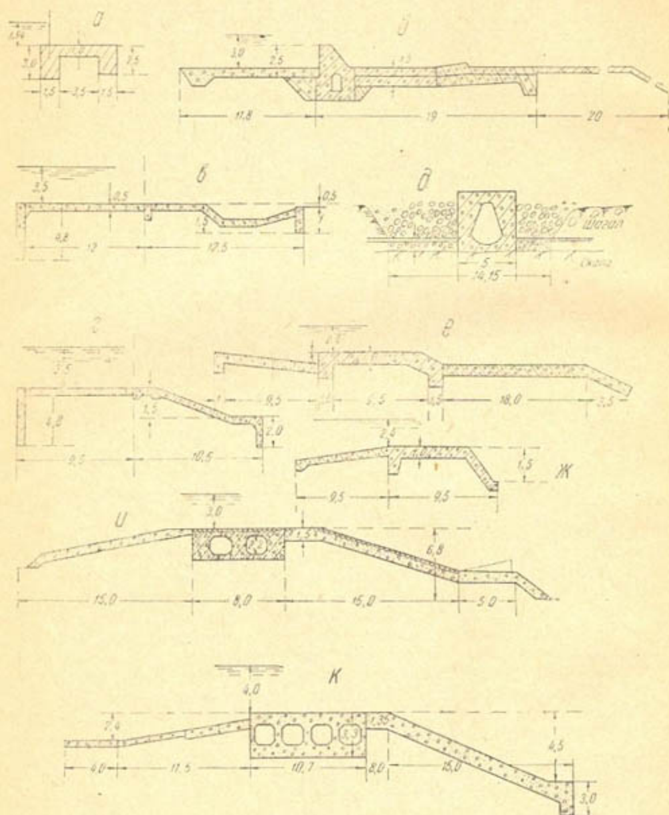
Рис. 59. Флютбеты водозаборных плотин:
