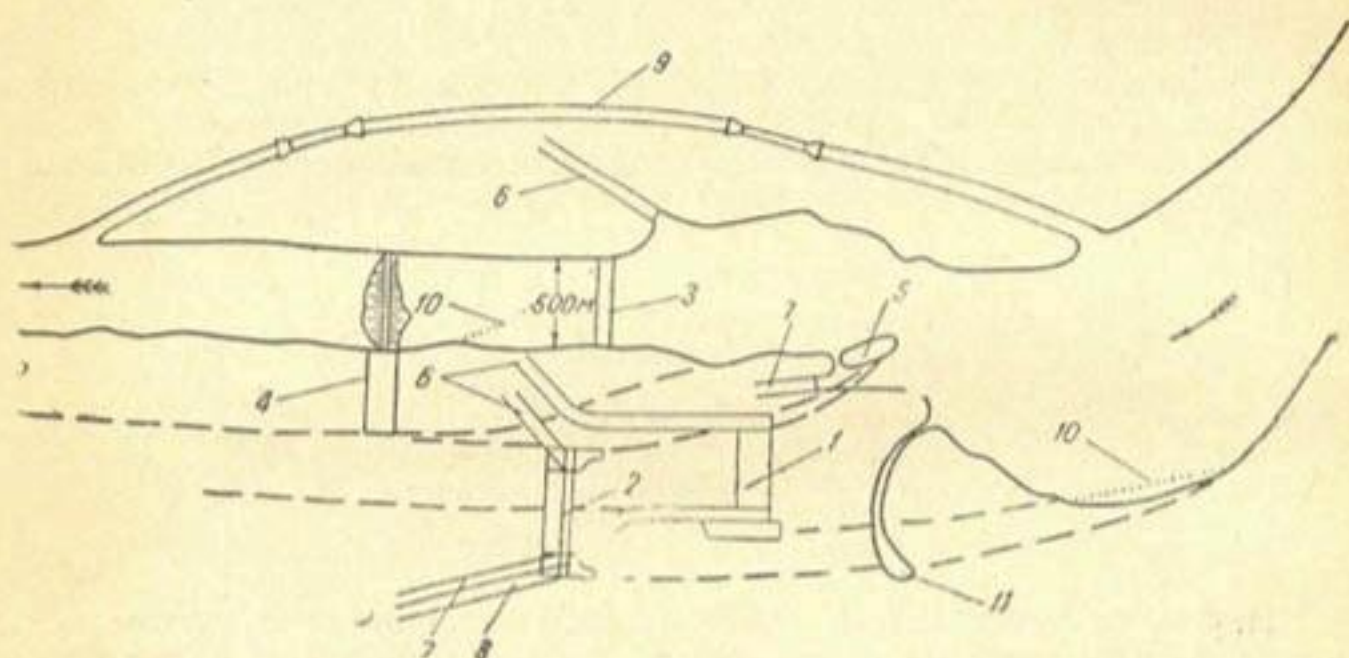
Рис. 24. Схемы водозаборов у мыса Тахияташ на Амударье.
