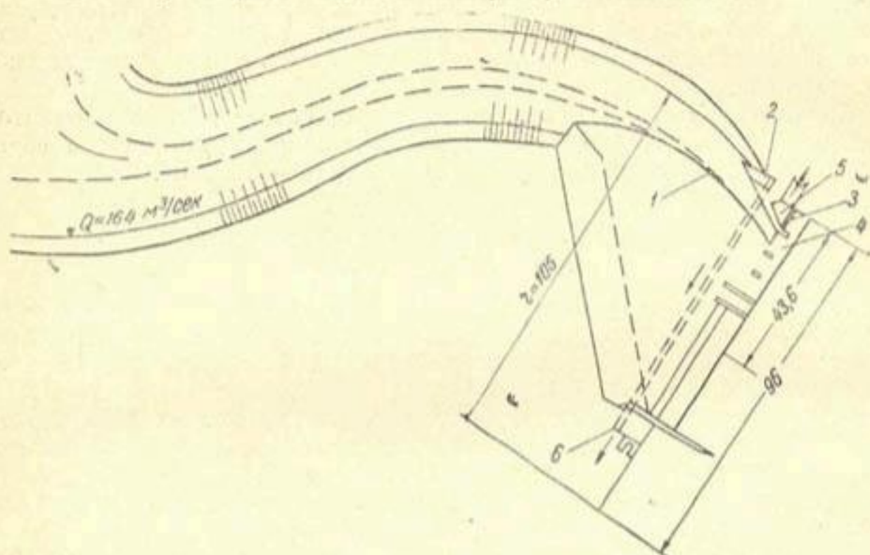
Рис. 23. Неосуществленный вариант водозабора ферганского типа, разработанный для реконструкции плотины на Кугартсае:
