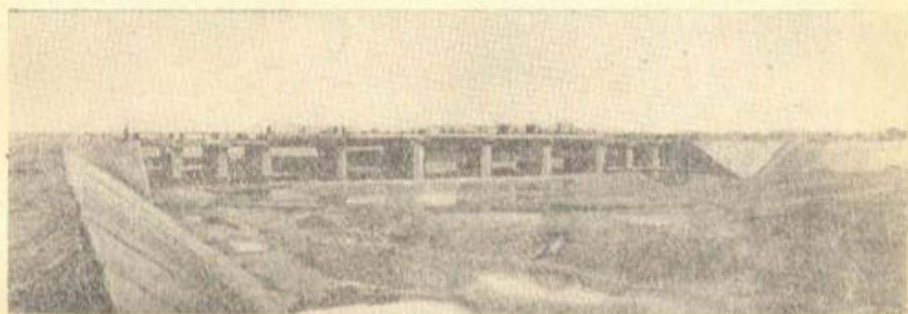
Рис. 46. Тешикташская плотина на Карадарье до монтажа затворов.
