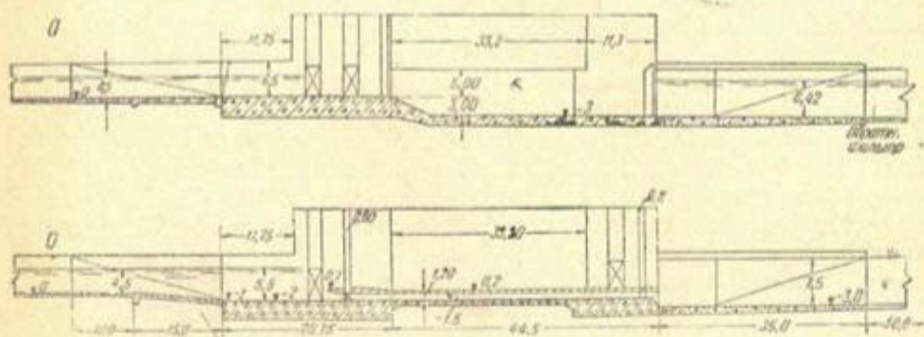
Рис. 44. Продольные разрезы Казалинской плотины на Сырдарье:
