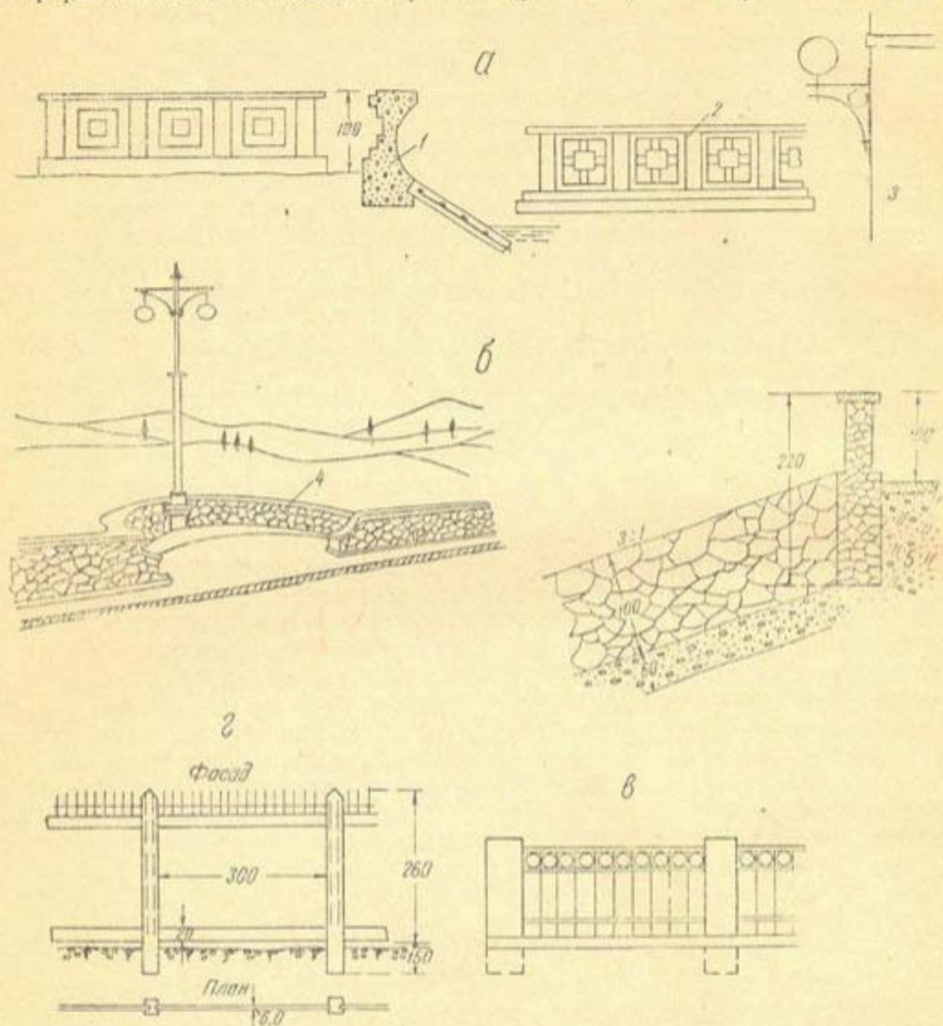
Рис. 63. Архитектурные эскизы некоторых деталей плотины Средней Азии:
