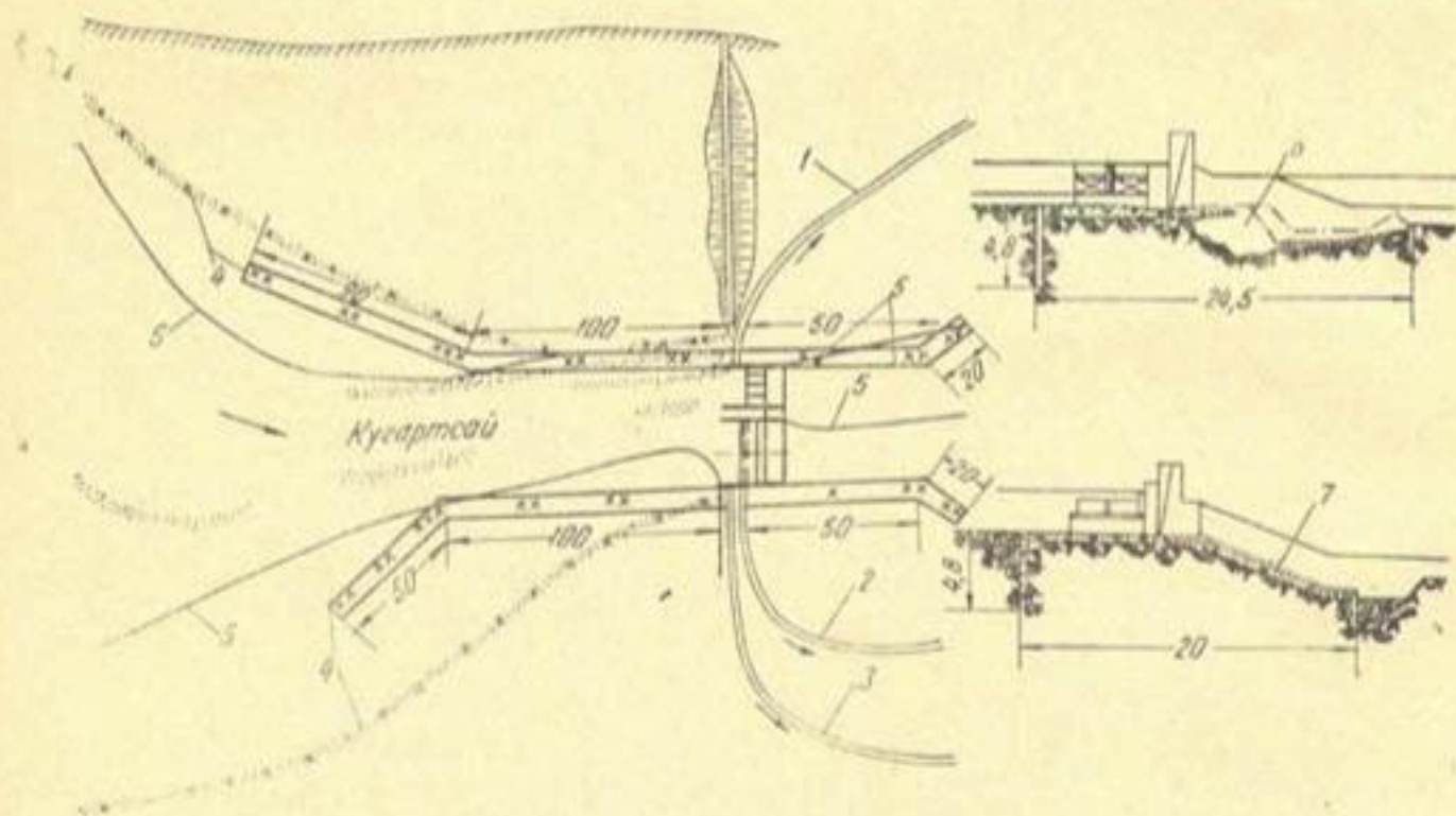
Рис. 4. Схема водозабора на Куяртсае, КиргССР:
