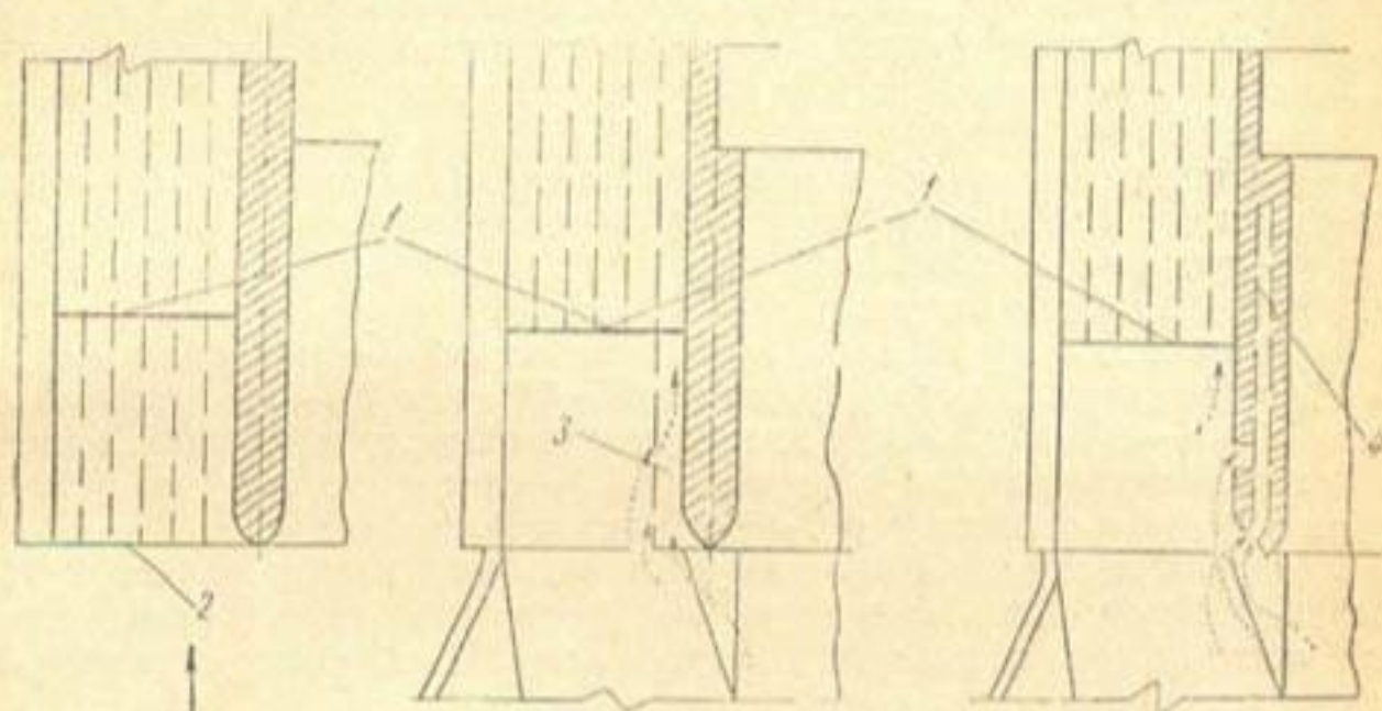
Рис. 45. Схемы конструкций по борьбе с завихрениями на Казаинской плотине, предложенные САНИИРИ:
