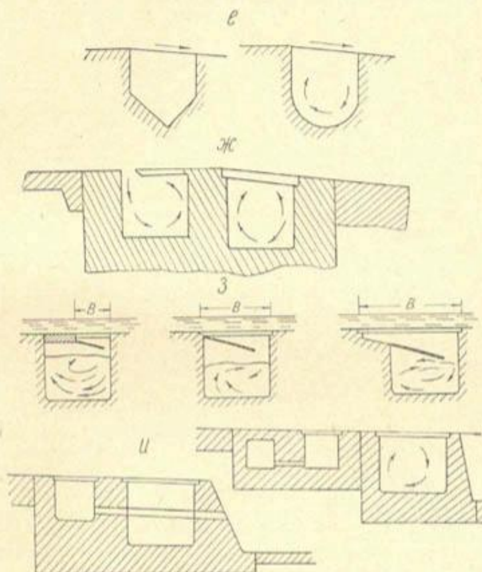
Рис. 53. Развитие конструкций водозахватных и наносоперехватывающих галерей плотин решетчатого типа; варианты а, ж, з, и.
