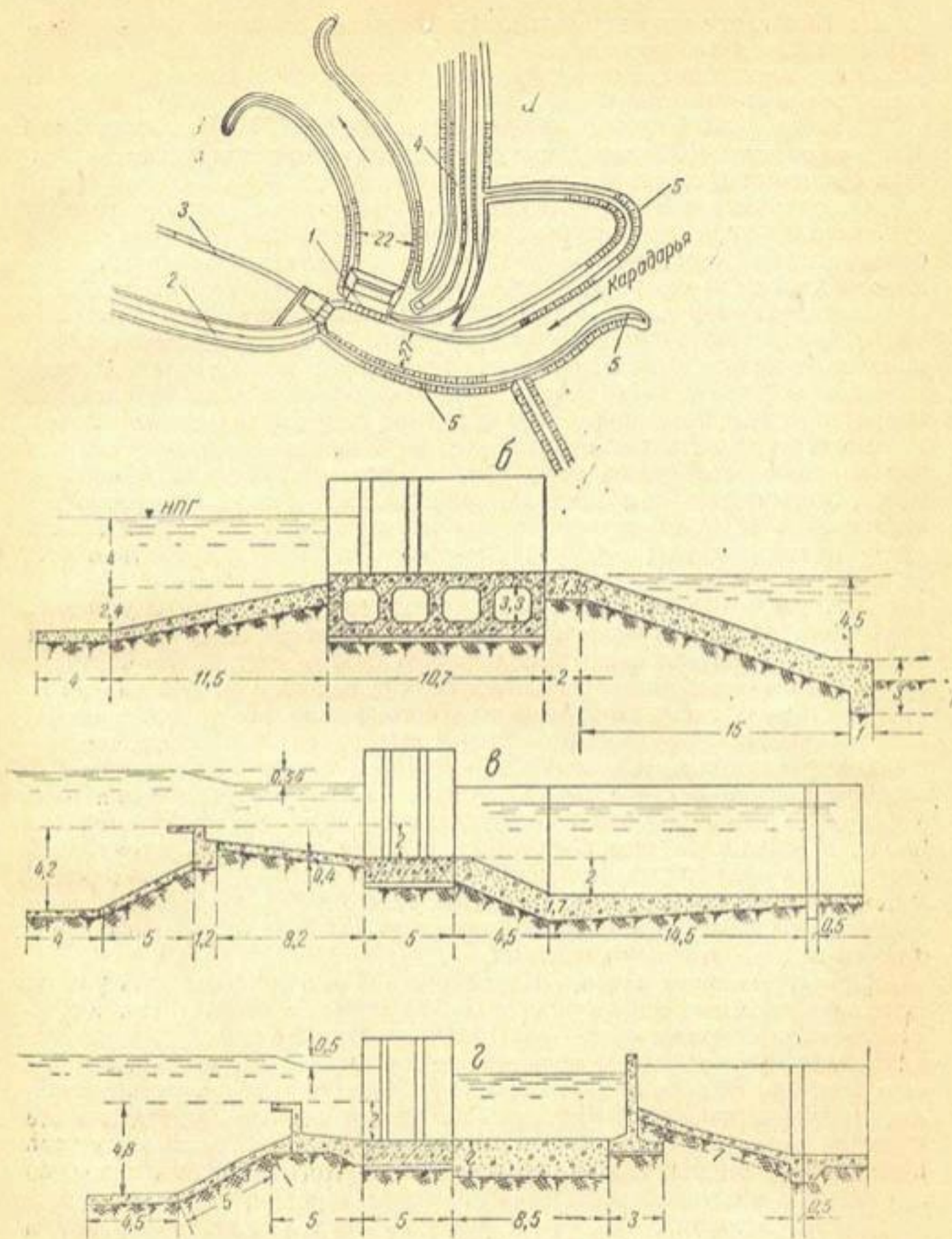
Рис. 21. Схема Дамходжинского гидроузла:
