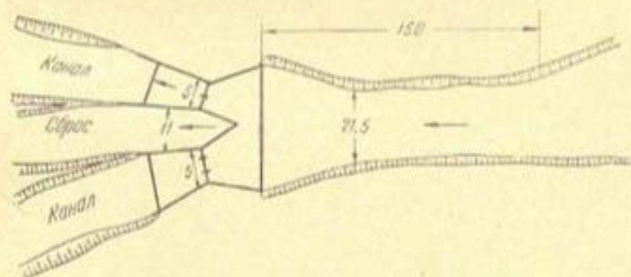
Рис. 9. Двухсторонний водозабор стрельчатого типа на Бешалышсае в Ферганской долине (размеры в метрах).
