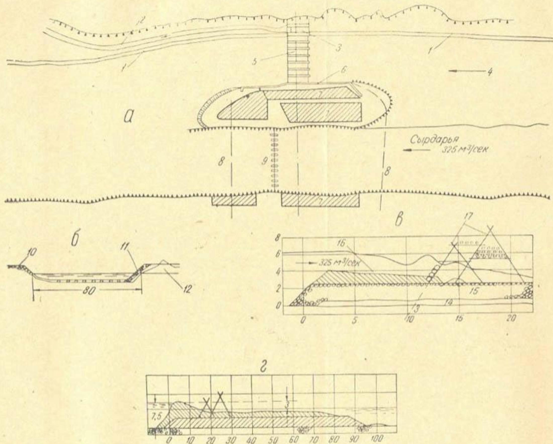
Рис. 37. Перекрытие Сырдарьи на Фархадстрое:
