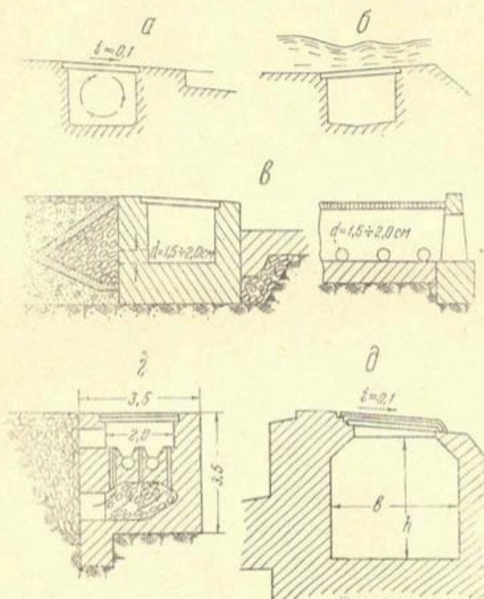
Рис. 52. Различные конструкции водозахватных и наносоперехватывающих галерей плотины решетчатого типа; варианты а, б, в, г, д (размеры в метрах).
