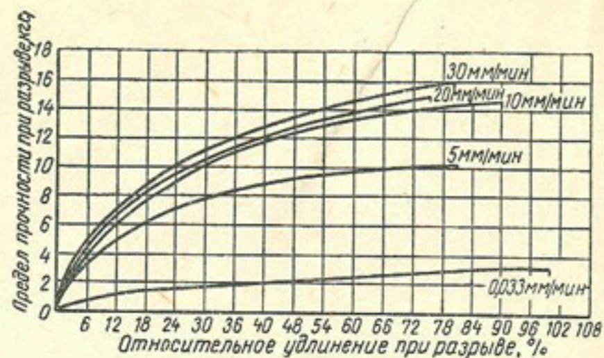
Рис. 13. Влияние скорости нагружения образцов на результаты определения прочности и деформативности мастики ГС-1.
