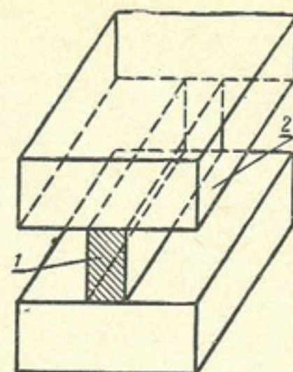
Рис. 14. Образец для определения деформативности и прочности мастики:
