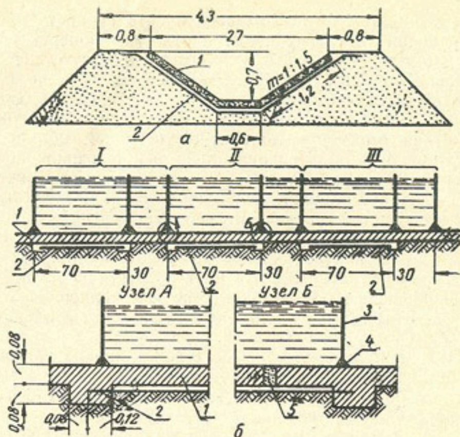
Рис. 6. Схема канала I-P-6 Татарбунарской системы с пленочным экраном и монолитным бетонным покрытием:
