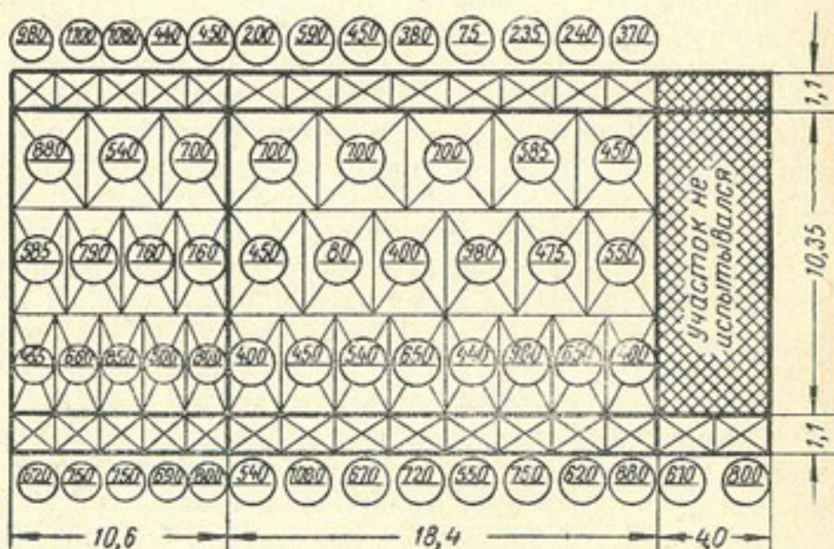
Рис. 26. Результаты испытаний полимербетонной облицовки пролетов 1 и 2 Яккабагского гидроузла:
