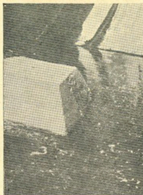
Рис. 27. Кавитационное разрушение на шашке-гасителе водосливной плотины Волжской ГЭС им. В. И. Ленина.
