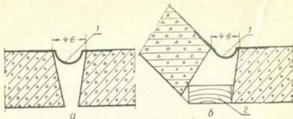
Рис. 18. Конструкции швов в сборных облицовках каналов: а — герметизация шва армогерметиком; б — герметизация шва примыкания откосной плиты к донной армогерметиком; 1 — армогерметик слоем 0,5 см; 2 — монтажная деревянная подкладка (размеры в см).
