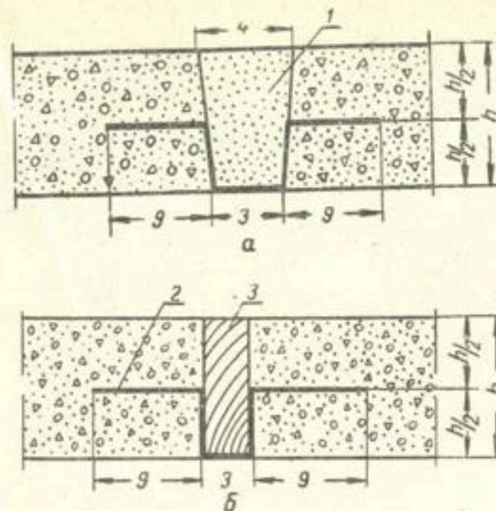
Рис. 19. Пленочная шпонка в облицовке канала из монолитного бетона толщиной менее 10 см (а) и более 10 см (б): 1 — цементный раствор; 2 — полиэтиленовая пленка; 3 — антисептированная доска (размеры в см).
