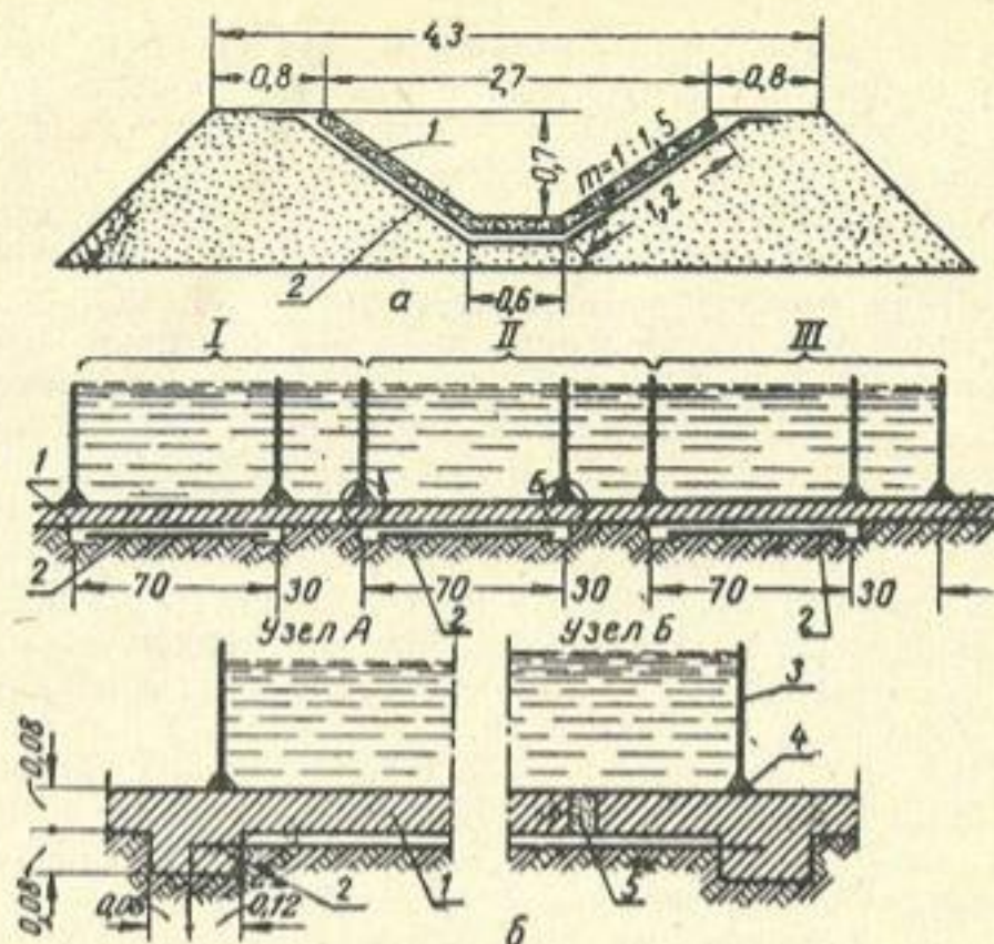
Рис. 6. Схема канала I-P-6 Татарбунарской системы с пленочным экраном и монолитным бетонным покрытием: а — сечение канала; б — схема устройства отсеков при фильтрационных измерениях; 1 — монолитный бетон; 2 — пленка; 3 — щит; 4 — раствор; 5 — цементный раствор (размеры в м).
