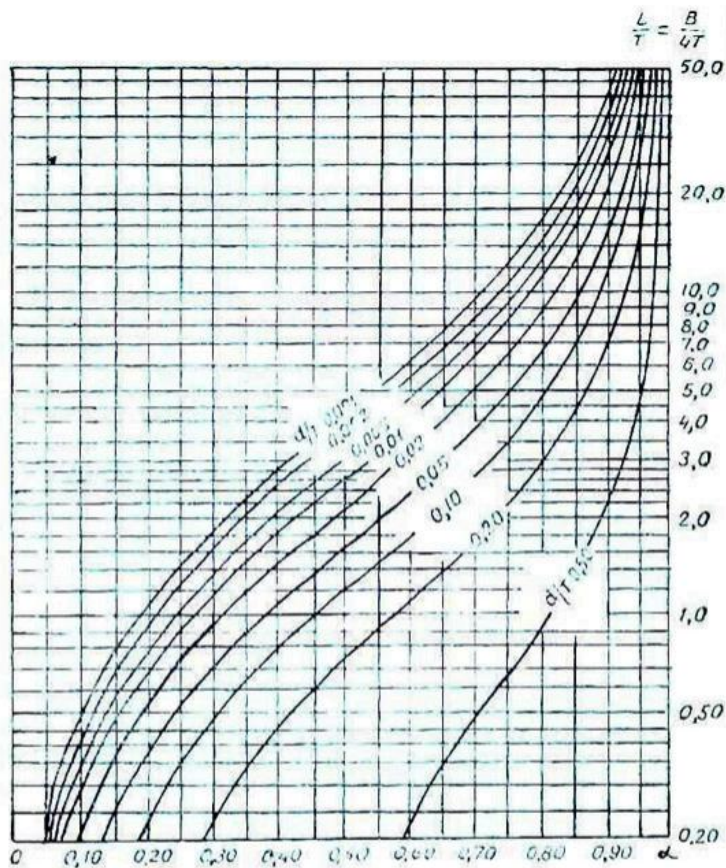
Рис. 9. График С. Ф. Аверьянова для определения коэффициента влияния дренажа \alpha .
