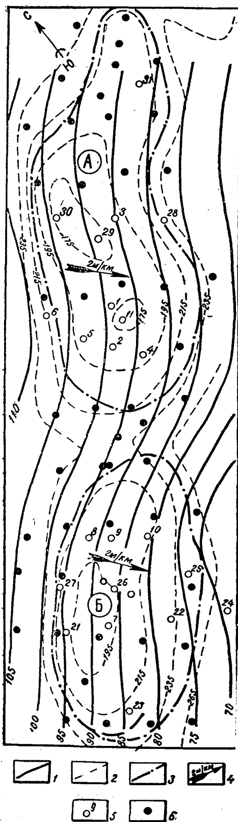
Рис. 1. Схематическая структурно-гидрогеологическая карта Базайского поднятия: А — Жаксыкоянкуласское, Б — Жаманкоянкуласское месторождения. 1 — гидроизогипс; 2 — изогипсы по кровле кумского горизонта; 3 — контур газоносных залежей; 4 — гидравлический уклон пьезометрической поверхности подземных вод кумского горизонта; 5 — структурные скважины; 6 — разведочные скважины.
