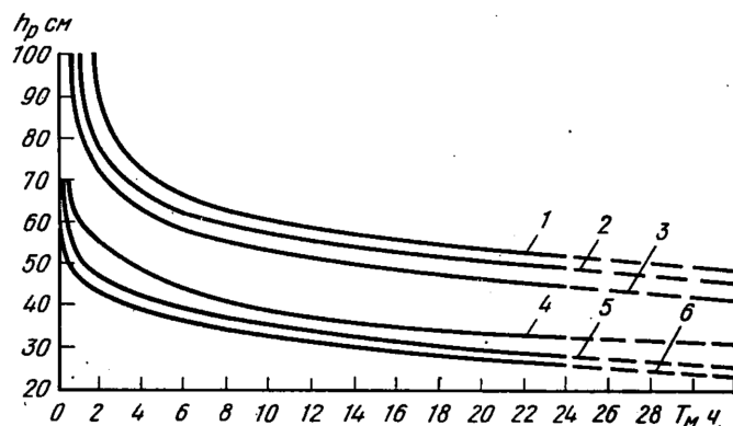
Рис. 2. Номограмма для расчета начала лавиноопасного периода при метелях по данным наблюдений на снеговальной станции Серебрянск (1, 2, 3) и метеостанций Бухтарма (4, 5, 6):
