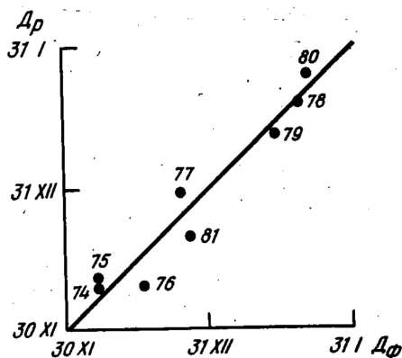
Связь рассчитанных D_p и фактических D_{\phi} дат замерзания Капчагайского водохранилища
