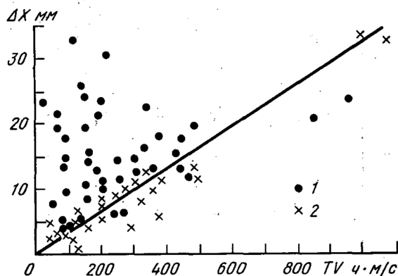
Рис. 4. Связь дефицита осадков ( \Delta X ), необходимых для схода лавин свежевыпавшего снега и определяемых по рис. 1 \sigma , с характеристикой TV для метеостанции Лениногорск:
