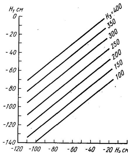
Зависимость сглаженных за 5 сут уровней воды у г. Гурьева ( H_1 ) от осредненных за этот же период уровней у пос. Пешной ( H_2 ) и уровней у пос. Махамбет ( H_3 )
