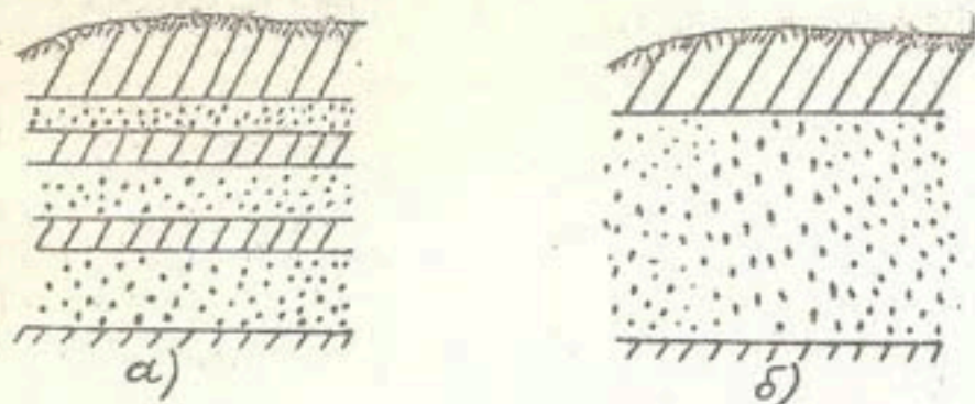
Рис. Вертикальные разрезы водонесных горизонтов: а) многослойный водонесный горизонт; б) двуслойный водонесный горизонт
