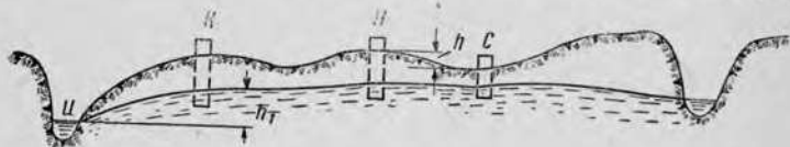
Рис. 7. Схема размещения существующего и проектируемого колодца в рельефе.
