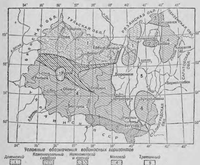
Рис. 5. Схематическая карта распространения и использования подземных вод Среднерусской возвышенности.
