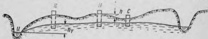
Рис. 7. Схема размещения существующего и проектируемого колодца в рельефе.
