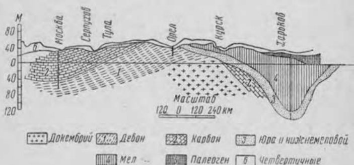
Рис. 4. Геологический разрез по линии Москва—Харьков.
