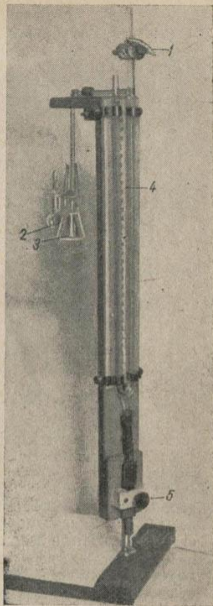
Рис. 18. Рабочая часть респирометра Варбурга (общий вид). 1 — верхний край манометра, 2 — рабочий сосудик, 3 — цилиндрик для щелочи, 4 — учетная шкала, 5 — нижний зажим.
