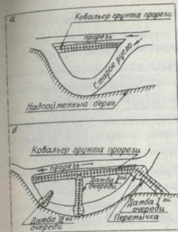
Рис. I. Схемы производства русловыправительных работ на р. Амударье:
