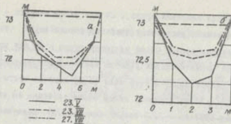
Рис. 3. Изменение поперечного сечения русла канала по времени: а - Большой Керисьяб, 2,7 км; б - Малый Керисьяб, 0,3 км.
