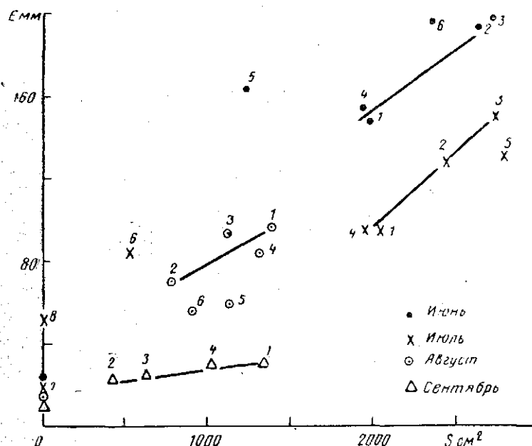
Рис. 1. Зависимость суммарного испарения ( E \text{ мм} ) от площади листьев ( S \text{ см}^2 ) на монолитах испарителей; горизонтальная площадка
