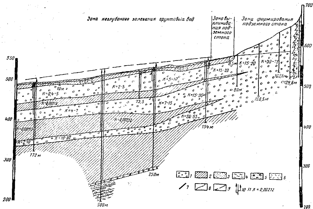
Рис. 1. Геолого-гидрогеологический разрез в меридиональном направлении: 1 — валунисто-галечники, галечники, гравийно-галечники; 2 — су глины; 3 — пески; 4 — глины; 5 — щебень; 6 — туфы, порфи- риты; 7 — разлом; 8 — уровень грунтовых вод; 9 — пьезометрический уровень IV водоносного горизонта; 10 — скважина гидро- геологическая; стрелки соответствуют напору подземных вод; 11 — коэффициент фильтрации
