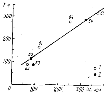
Рис. 3. Зависимость между величинами снегозапасов в руслах логов ( W_3 ) и продолжительностью метелей ( T ) за зиму:
