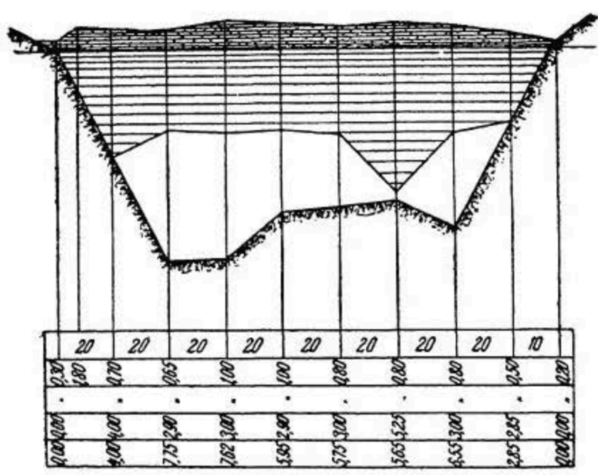
Рис. 135. Уменьшение живого сечения р. Свири донным льдом 10 ноября 1931.
