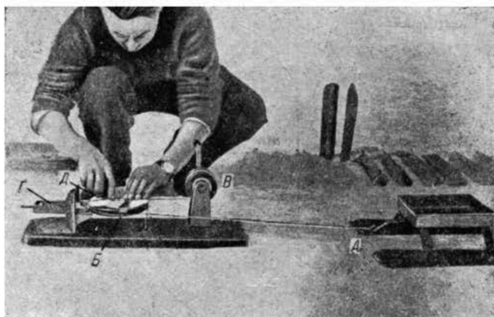
Рис. 207. Опыты Н. А. Павлова над сопротивлением движения лыж.
