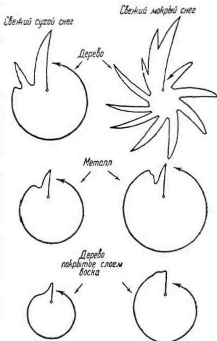
Рис. 208. Вектор-диаграммы зависимости сопротивления лыж.
