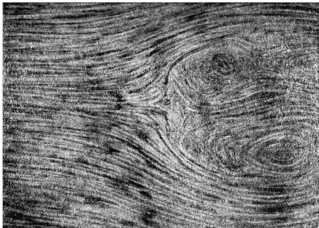
Рис. 159. Профиль движения воды (линии тока с их завихрениями), обнаруживаемый с помощью порошка лycopодия вокруг тонкой пластинки, поставленной перпендикулярно потоку.
