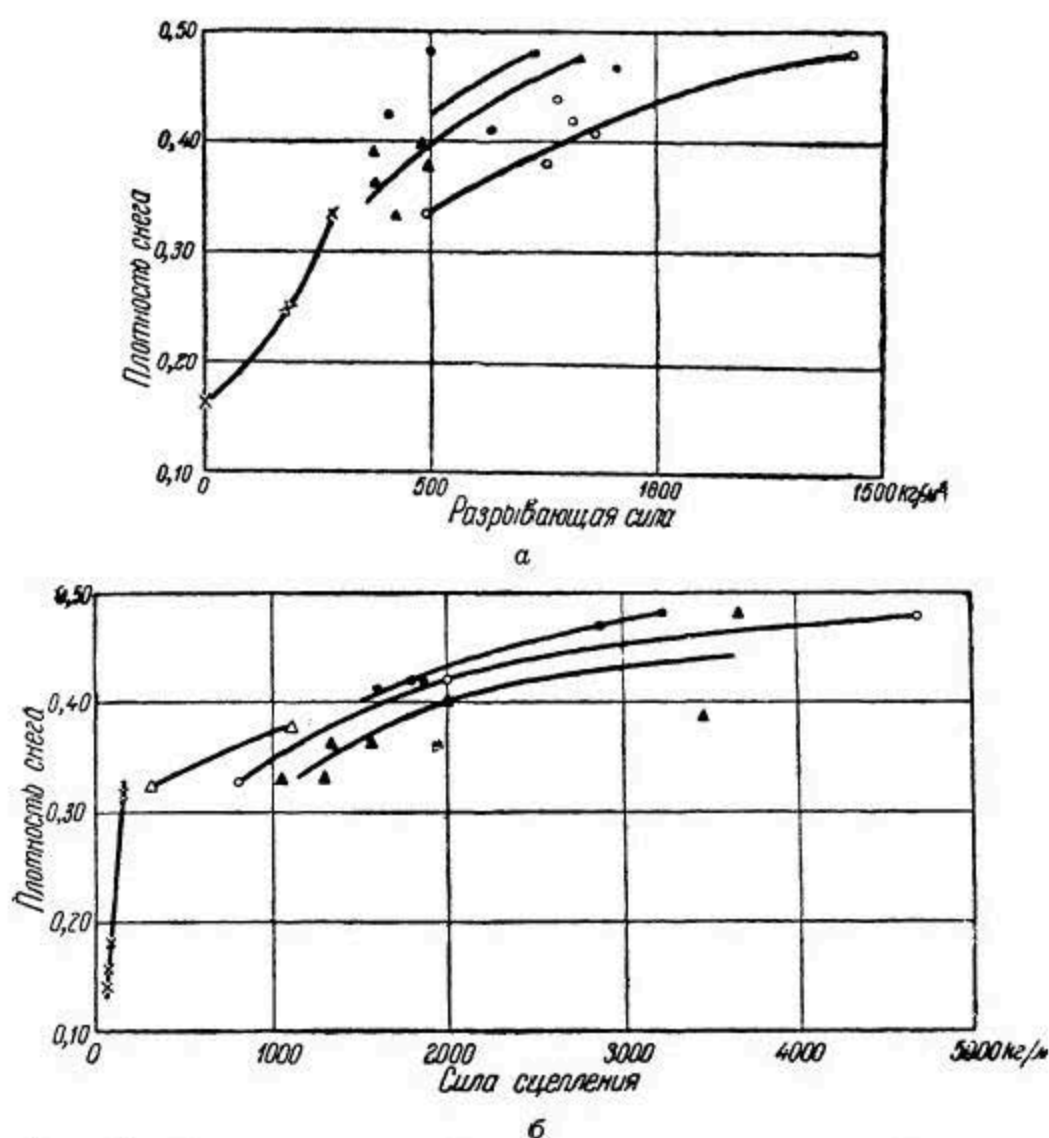
Рис. 72. Сила сцепления (а) и сопротивление разрыву (б) снега различной плотности (по Гоффу и Оттену).
