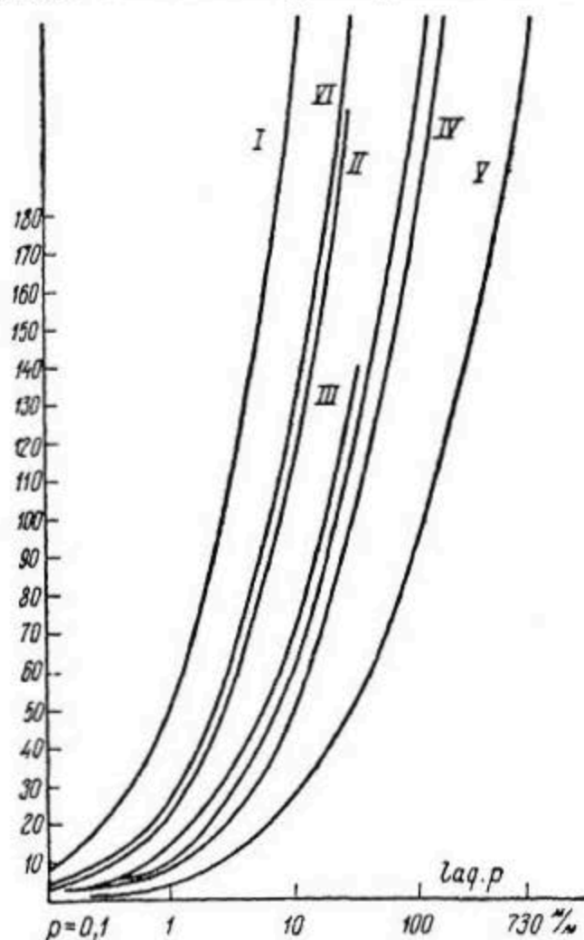
Рис. 71. Зависимость коэффициента теплопроводности хорошо проводящих материалов от давления находящегося в них воздуха по Смолуховскому.
