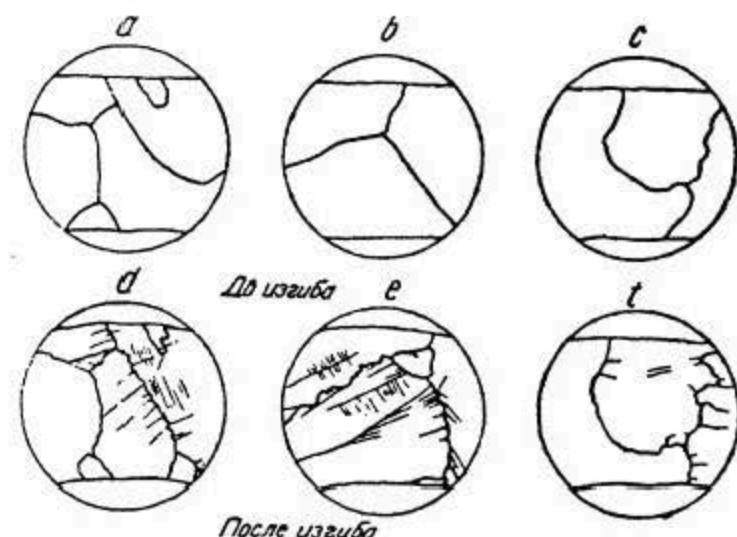
Рис. 55. Трещины отдельных зерен при изгибе (по Матсуяма).
