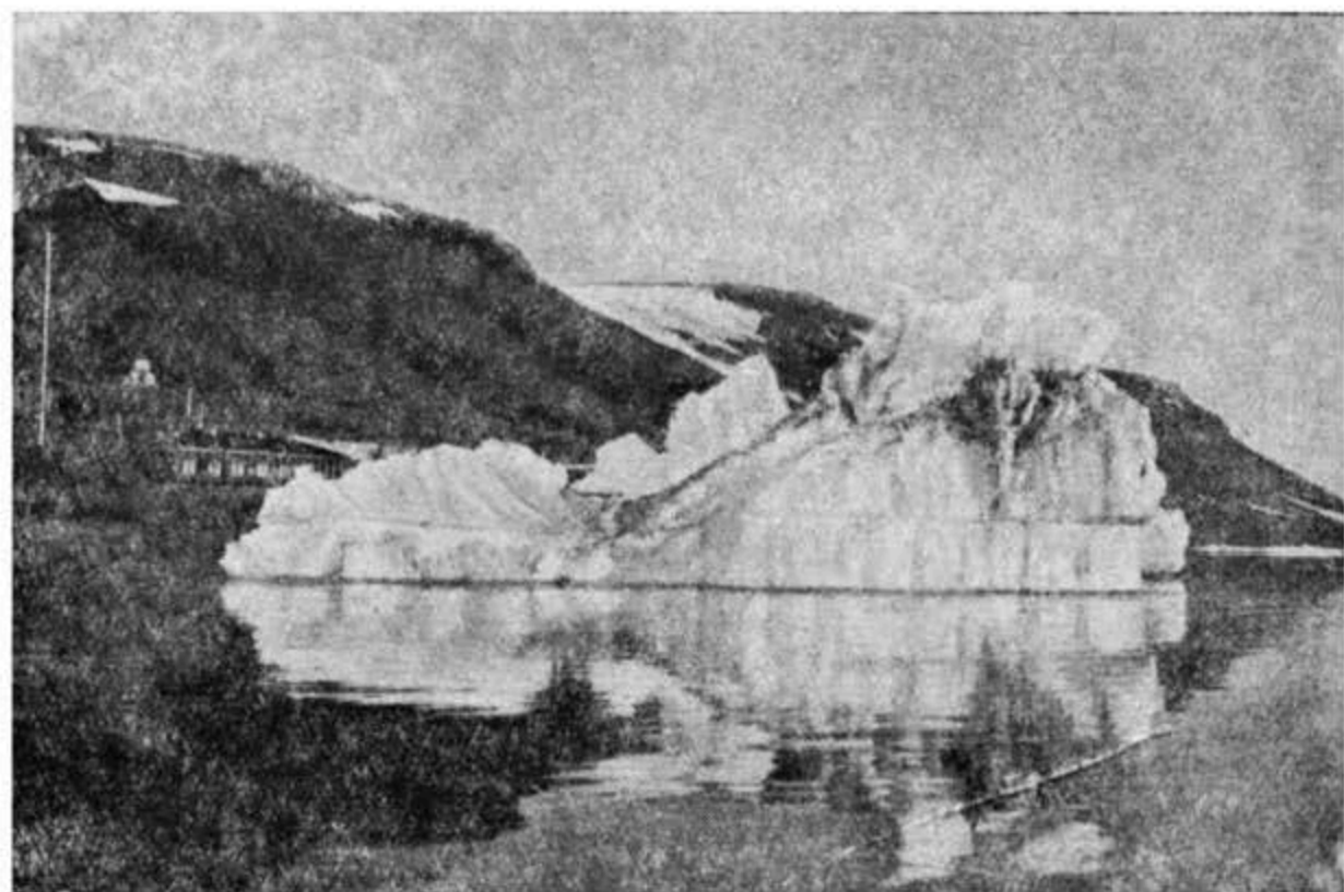
Рис. 144. Обломок айсберга — «щенок» — в бухте Тихой у Земли Франца-Иосифа (снимок Моргуна, 1935).
