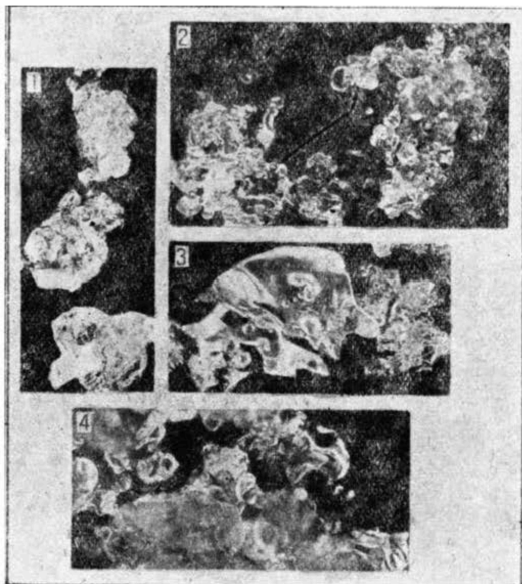
Рис. 153. Последовательные стадии фирнизации снега от частичного плавления зерен (снимки Зелигмана).
