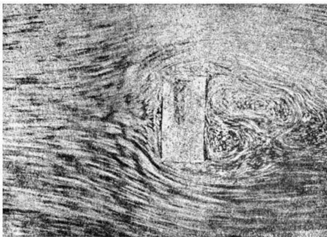
Рис. 161. То же — для поставленного на пути прямоугольного параллелепипеда.
