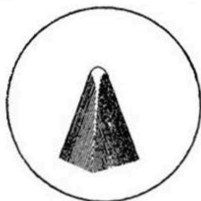
Рис. 99. Тригонально-пирамидальные кристаллы льда надземных вод (о. Вайгач, штольня; нат. велич. рисунок Головкина).
