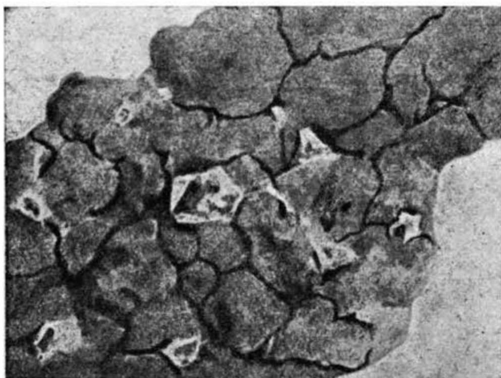
Рис. 201. Кристаллы льда в мерзлом грунте (Игарка; рис. Н. И. Быкова).
