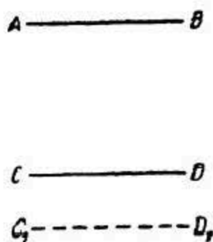
Рис. 20. Передача тепла посредством теплопроводности в случае перемещения поверхности раздела двух фаз.
