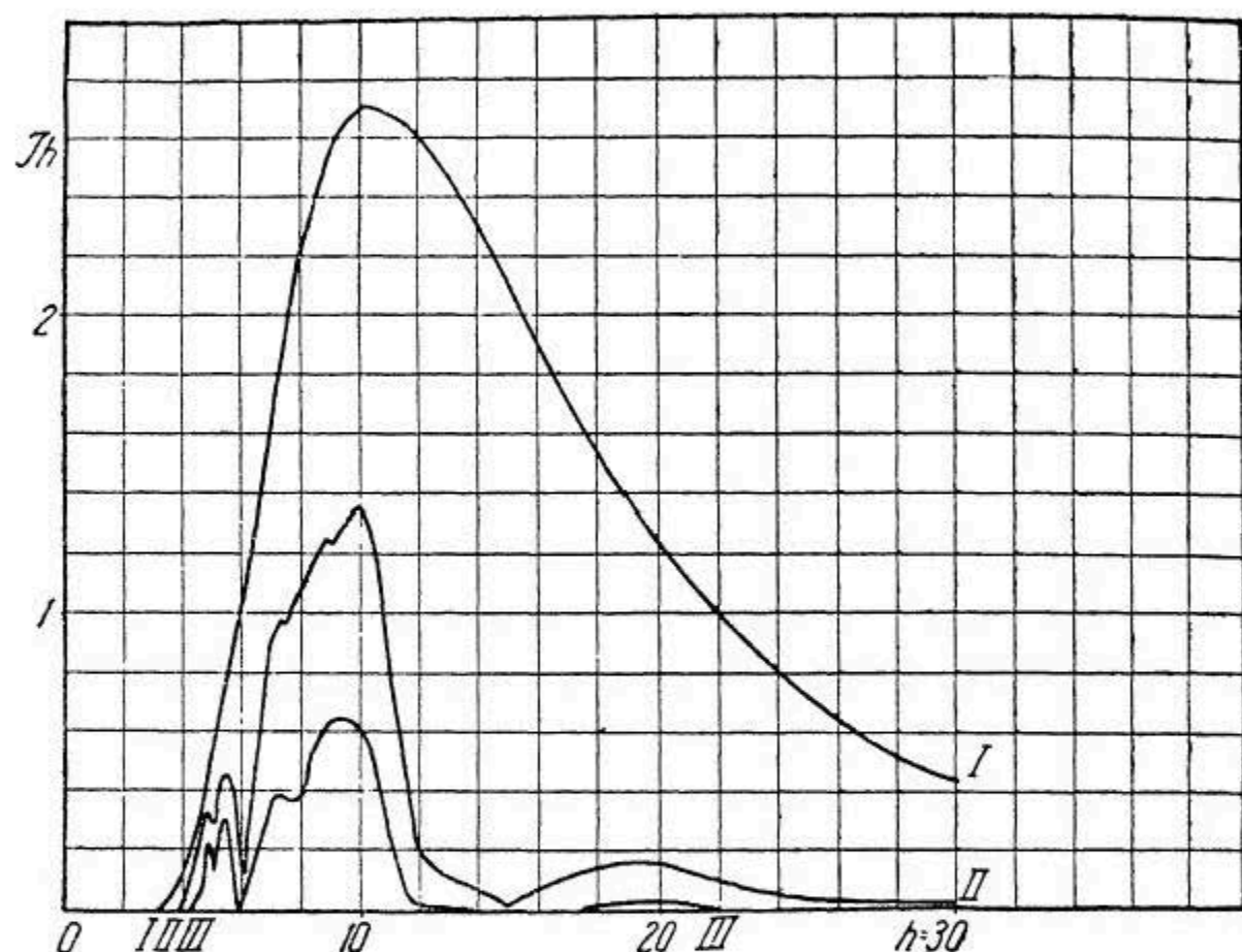
Рис. 62. Распределения энергии в спектре излучения абсолютно черного тела, с температурой 0^\circ (кривая I), после прохождения сквозь слой воды в 1 м (кривая II) и в 10 м (кривая III).
