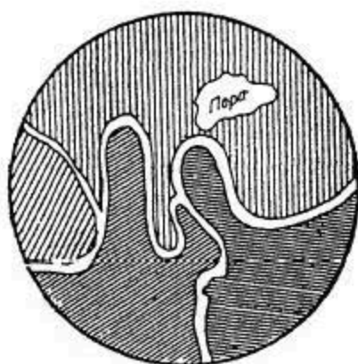
Рис. 101. Вращение кристаллов льда друг в друга (возможно вследствие метаморфических процессов) в сформировавшемся ледяном покрове (Карское море), имеющем скрытозернистую текстуру (шлиф; вид под микроскопом; рисунок Головкова).
