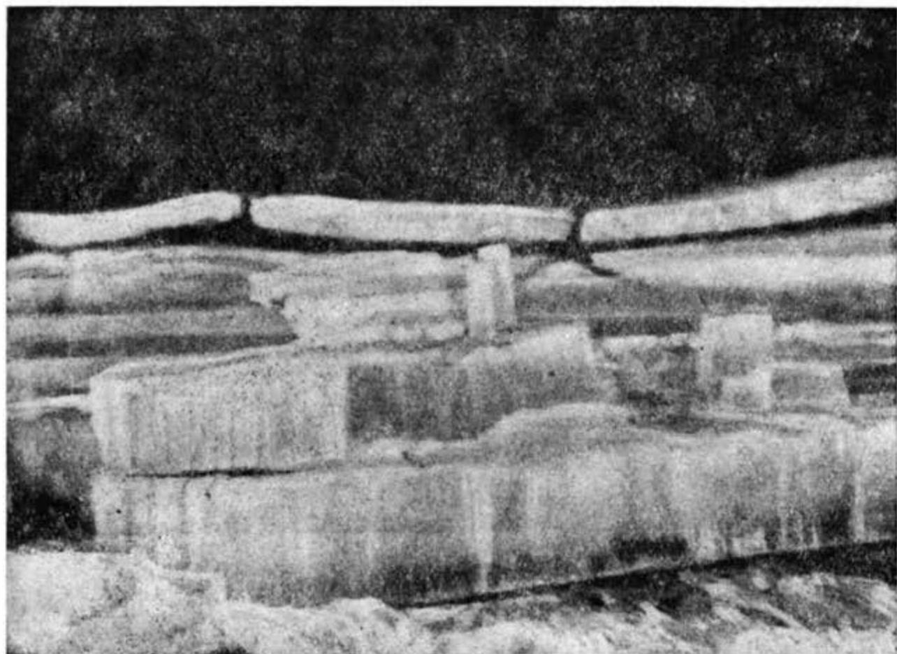
Рис. 146. Распад льда весной на р. Пилипе. Март 1928 (снимок А.-Б. Добровольского).
