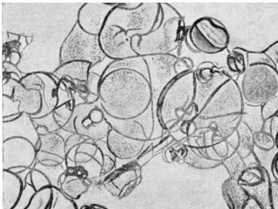
Рис. 41. Элементы кристаллизации воды по Альтбергу.
