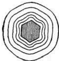
Рис. 12. Эквitemпературные поверхности вокруг шестигранного кристалла льда, находящегося в переохлажденной воде.
