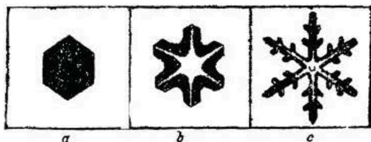
Рис. 16. Последовательные формы роста кристалла нодоформа (по Догелю).
