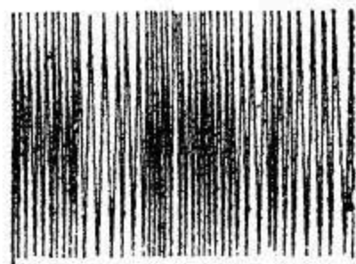
Рис. 35. Строение льда из соленого озера по Листову: а — горизонтальное; б — вертикальное сечение.
