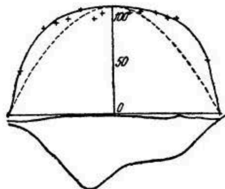
Рис. 197. Форма среднего сечения Хинтерейсфернера и распределение скоростей на его поверхности (сплошная линия) и на поверхности полуэллиптического канала (пунктирная линия).
