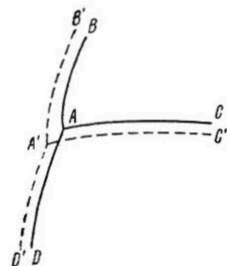
Рис. 6. Влияние осмотического давления на тройную точку.
