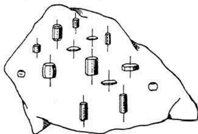
Рис. 73. Внутренние полости в речном льду в виде «отрицательных кристаллов» по Лейдольту.
