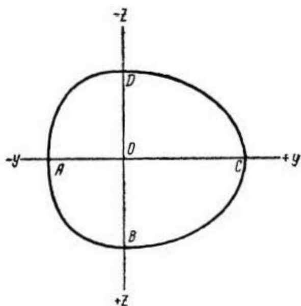
Рис. 195. Схема связи теорий ламинарного течения жидкости по каналу и по трубе.
