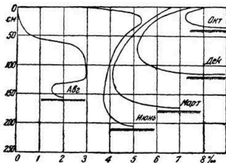
Рис. 36. Соленость льда на различных расстояниях от поверхности в различные месяцы.
