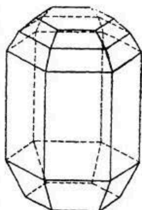
Рис. 97. Призматический кристалл льда перистых об- лаков (по Хессу).
