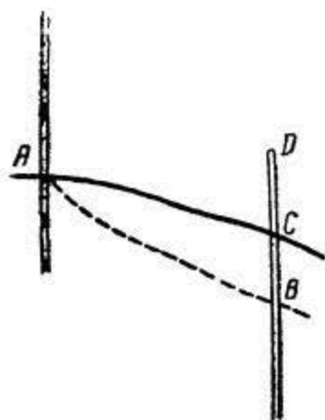
Рис. 188. Путь снежинок фирна и воткнутой в фирн палки.
