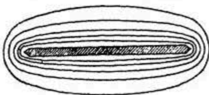
Рис. 13. Сечение эквitemпературных поверхностей вокруг пластинки льда в переохлажденной воде, перпендикулярное плоскости пластинки.
