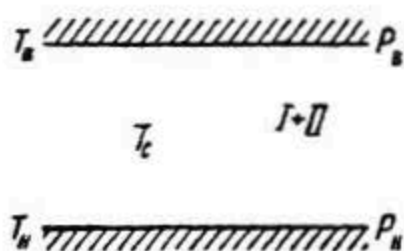
Рис. 17. Схема расположения слоев при превращении двухфазной системы.
