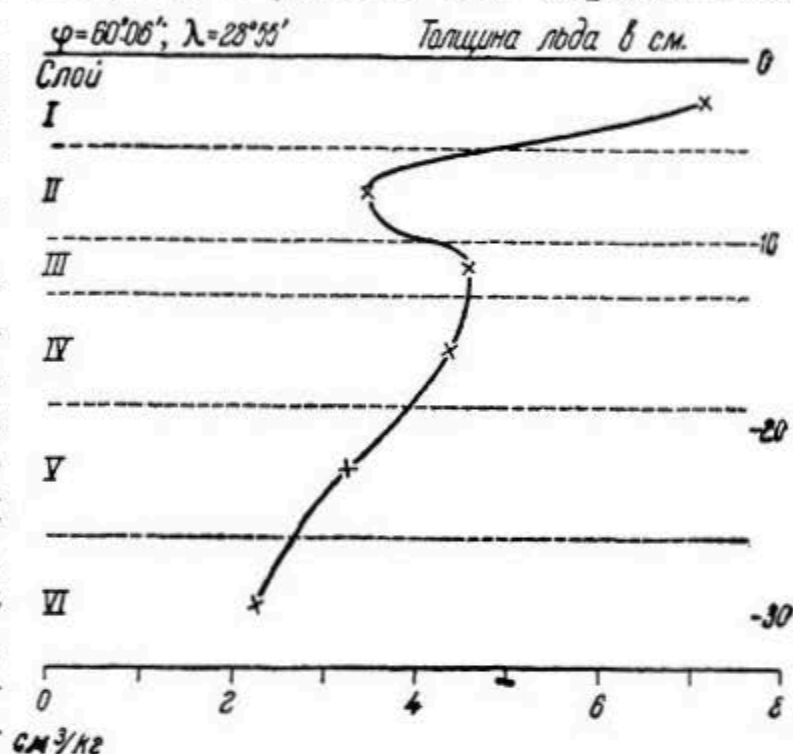
Рис. 148. График вертикального распределения полостей во льде в см³ на кг льда (по В. И. Арнольду-Алябьеву).
