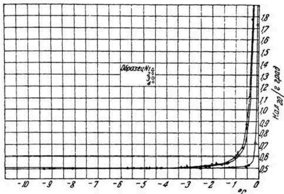
Рис. 32. Зависимость теплоемкости льда от температуры от -10^{\circ} до 0^{\circ} по Диккинсону и Осборну.
