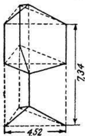
Рис. 64. Элементарная ячейка решетки льда.
