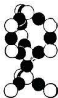
Рис. 65. Расположение атомов в элементарной ячейке решетки льда.
