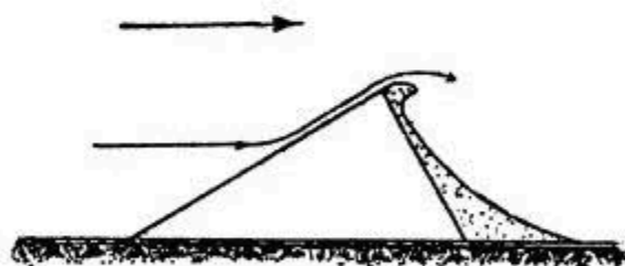
Рис. 165. Завихрение и даносы в случае клинообразного препятствия, обращенного пологим склоном к ветру (по Волькенбаху).
