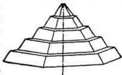
Рис. 74. Фигуры плавления на поверхности речного льда по Лейдольту.
