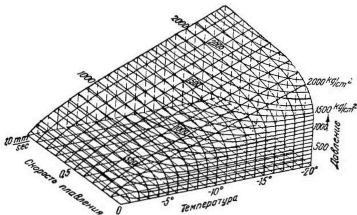
Рис. 59. Соотношения между быстротой плавления, температурой и давлением по Хессу.
