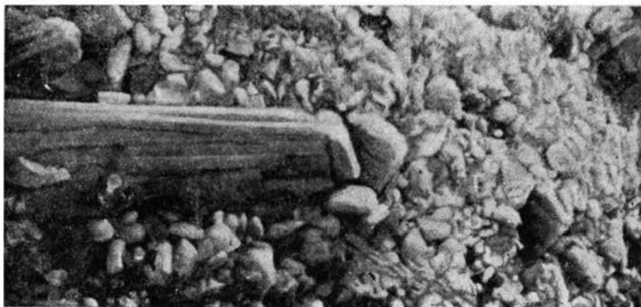
Рис. 147. Слоистая льдина у борта ледокола «Ермак», поставленная им на ребро в густой ледяной наше (вид сверху с борта). Балтийское море. Март 1923 (снимок В. А. Воротилова).
