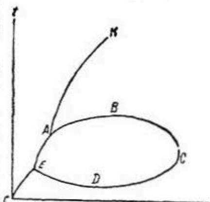
Рис. 3. Диаграмма изменений состояния по Тамману-Вейнбергу.
