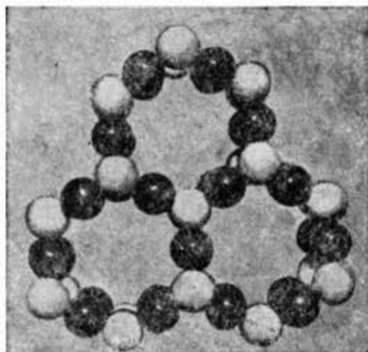
Рис. 66. Модель кристалла льда.
