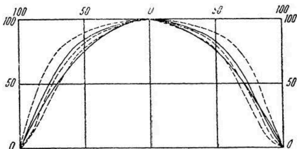
Рис. 183. Распределение скорости на поверхности различных ледников.
