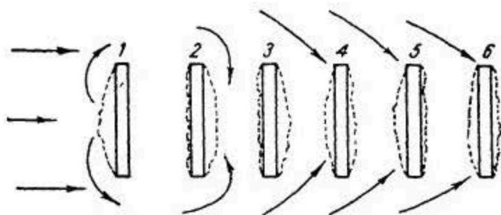
Рис. 44. Отложения «донного льда» на поставленных одна за другую сетках в опытах Зильбермана и Жемчугова.
