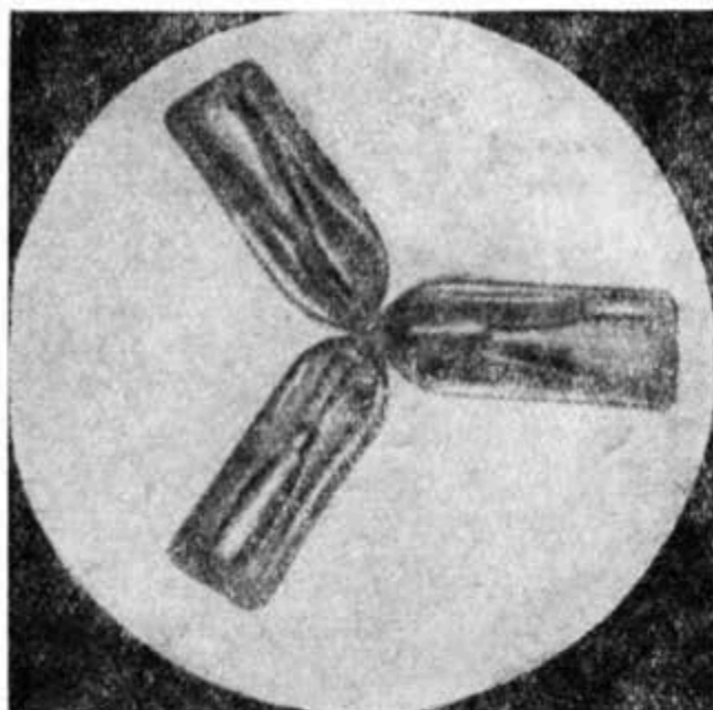
Рис. 90. Сужение внутренних пустот к пирамидальному концу заостренных стержневидных кристаллов льда (снимок Халльберга).
