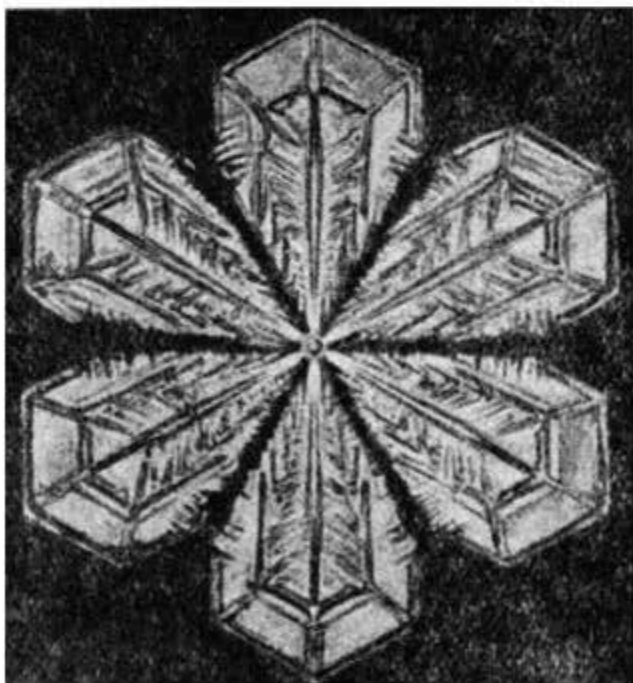
Рис. 84. Шестилопастный кристалл снега (снимок Бентлея).
