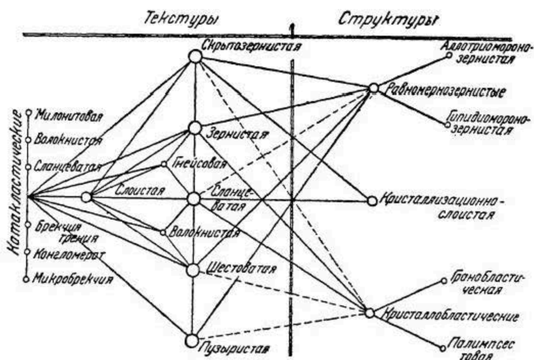
Рис. 100. Схема взаимоотношений текстур и структур льда Карского моря.
