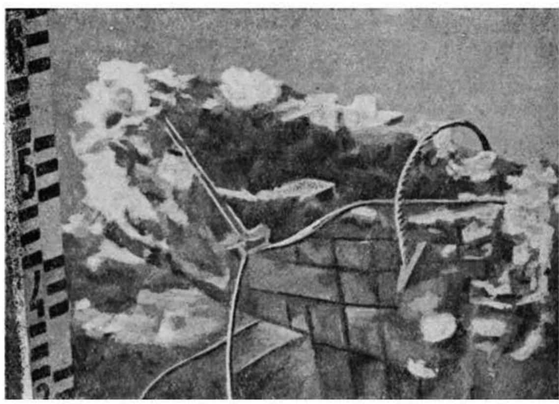
Рис. 134. Бельевая корзина с пластинками донного льда (снимок В. Я. Альтберга).
