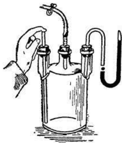
Рис. 105. Опыт Томсона с получением искусственного тумана.
