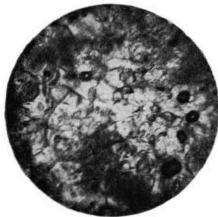
Рис. 103. Изометрические кристаллы льда, имеющие неправильную форму. Сформировавшийся ледяной покров Карского моря, имеющий сланцеватую текстуру (шлиф; микрофотография Головкова в проходящем свете; \times 40 ).
