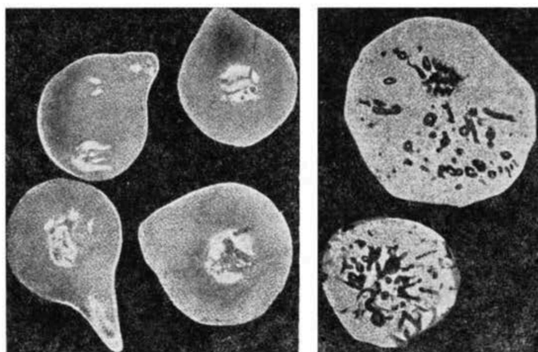
Рис. 108. Крупа, расплавившаяся с поверхности и снова замерзшая («зимний град», снимки Бентлея).
