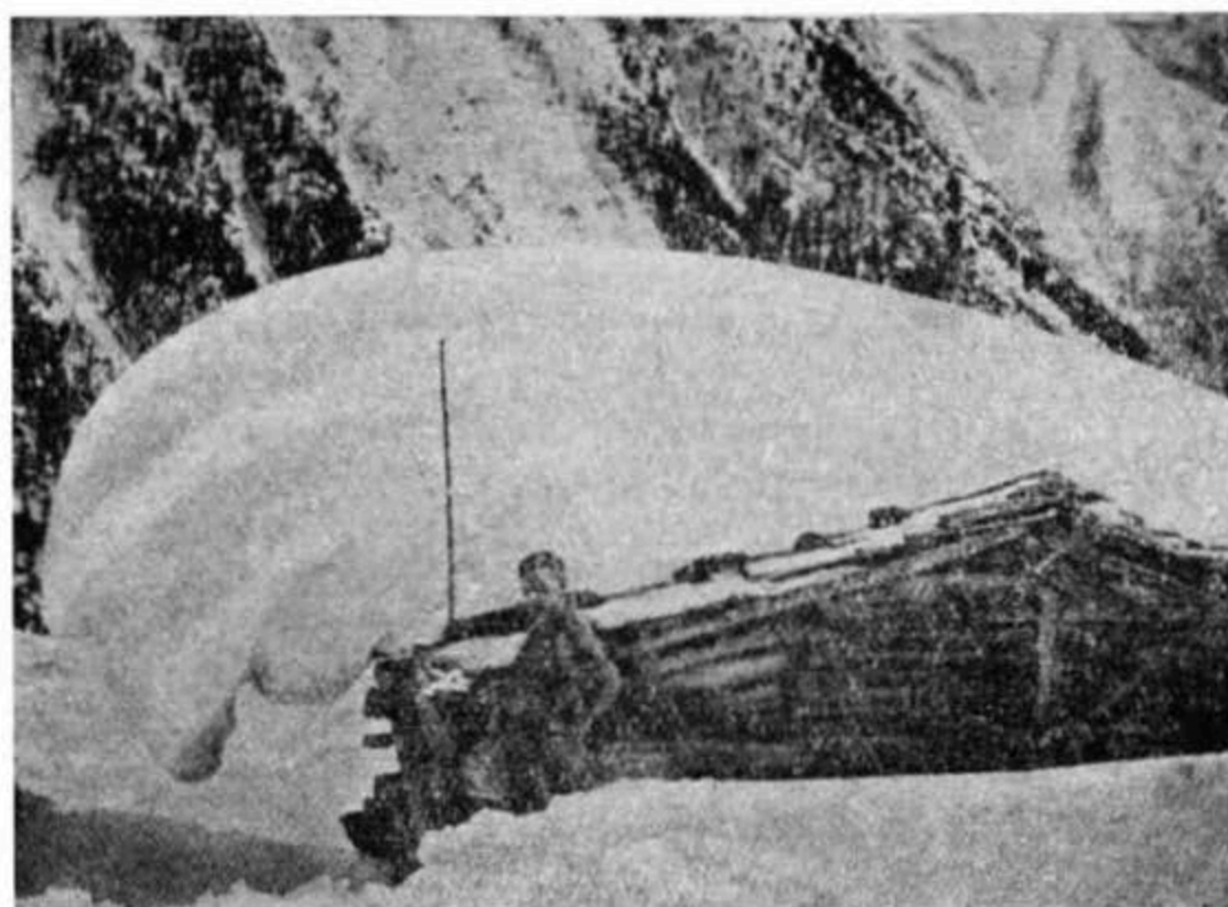
Рис. 22. Снежный навес за краем крыши.
