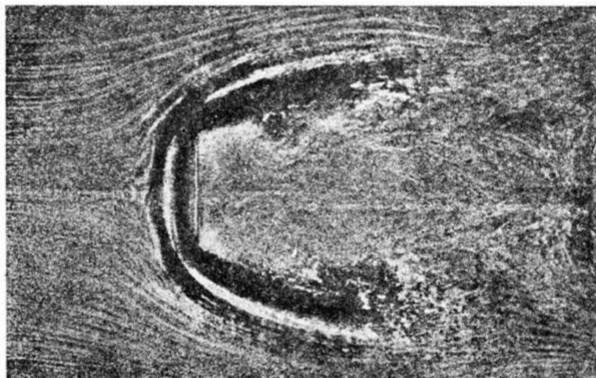
Рис. 171. Линии тока за перпендикулярной к направлению потока пластиной (снимок Рябушинского).
