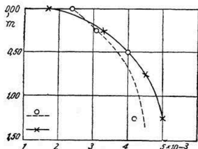
Рис. 53. Коэффициент теплопроводности на различных слоях соленого льда по Мальмгрену.
