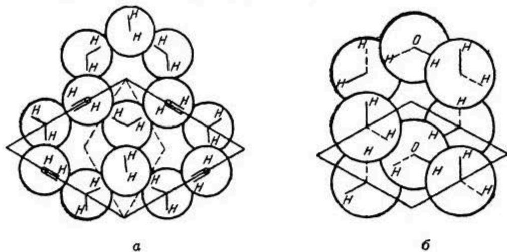
Рис. 70. Структура льда (а) и воды (б) по Берналю и Фаулеру.
