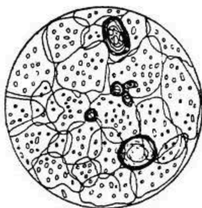
Рис. 102. Округлые изометрические кристаллы льда в сформировавшемся ледяном покрове (Карское море), имеющем зернистую текстуру (шлиф; вид под микроскопом, рисунок Головкова).
