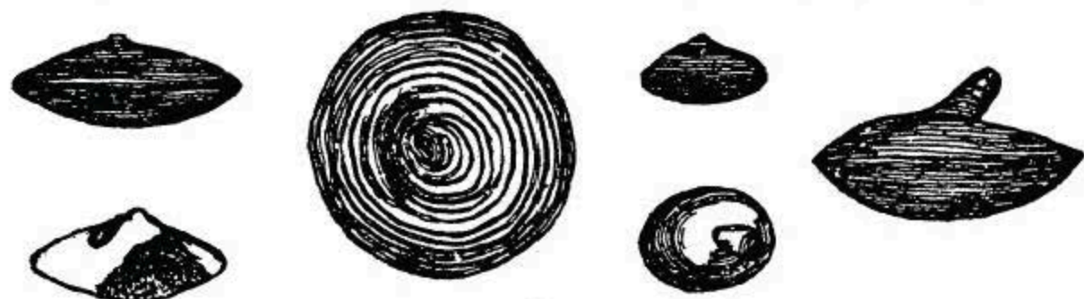
Рис. 126. «Искусственные градинки» Гезехуса — застывшие капельки расплавленной сурьмы.
