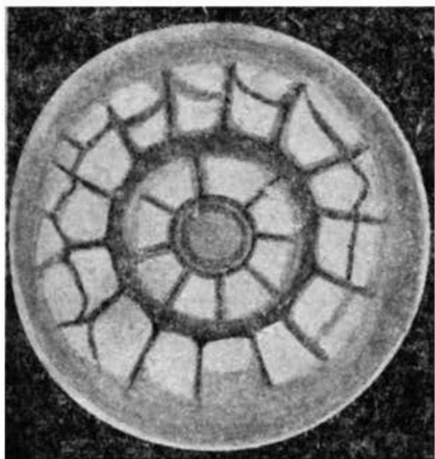
Рис. 123. Градины зернистого строения.
