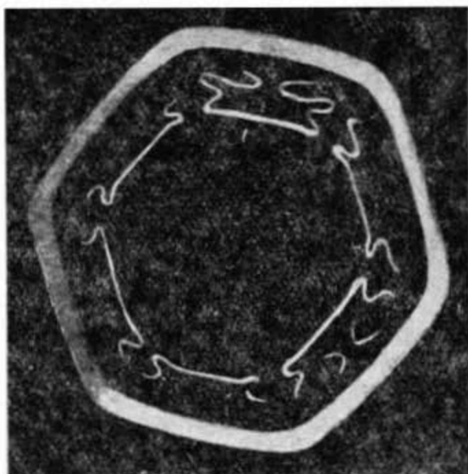
Рис. 96. Шестиугольный пластинчатый кристалл снега с признаками пирамидального строения в виде узких полосок по краям основания (снимок Г. Норденшельда).
