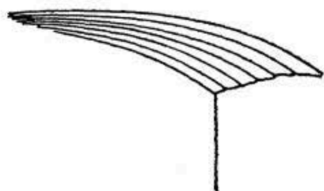
Рис. 167. Схема образования ветровых козырьков (козырьков давления по Волькенбаху).
