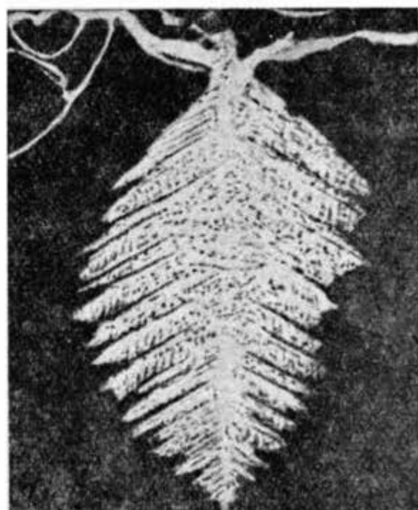
Рис. 115. Дендритовый морозный узор на окне (снимок Сигсона).
