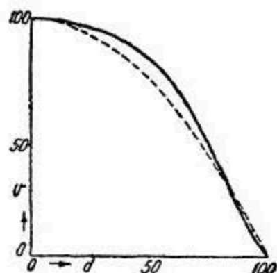
Рис. 199. Типовое распределение скоростей на поверхности ледника.
