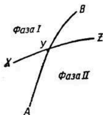
Рис. 8. Схема неустойчивых состояний по две стороны кривой перехода.
