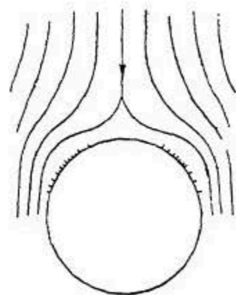
Рис. 110. Осаждение изморози на цилиндрах большого радиуса.
