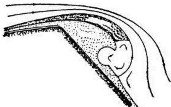
Рис. 168. Перекрытие наносного козырька козырьком давления по Волькенбаху.
