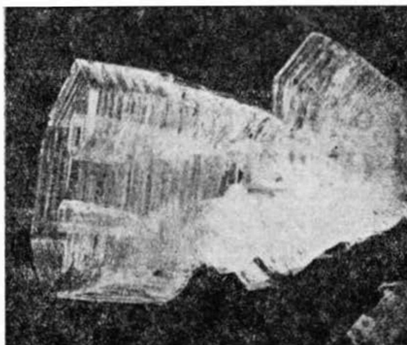
Рис. 119а и 119б. Пещерные кристаллы иней (снимок Вегенера в Гренландии). Обратите внимание, что одна сторона воронки открыта и заворачивается внутрь в виде шестиугольной спирали; увеличение: рис. 119а в 6 раз, рис. 119б — в 4 раза.
