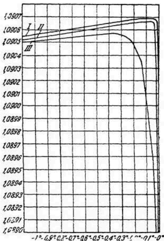
Рис. 39. Изменяемость удельного объема льда с температурой по Петтерсону.
