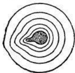
Рис. 11. Эквипотенциальные поверхности вокруг изолированного проводника с острием.
