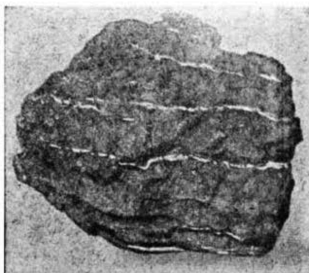
Рис. 202. Кусок глины (толщиной 15 см) с прослойками льда.
