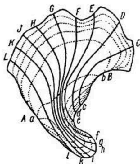
Рис. 185. Проекция на дно ледника линий тока и линий одинакового возраста льда.
