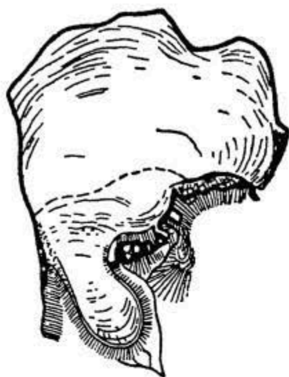
Рис. 184. Область питания, фирновая линия и область таяния ледника.
