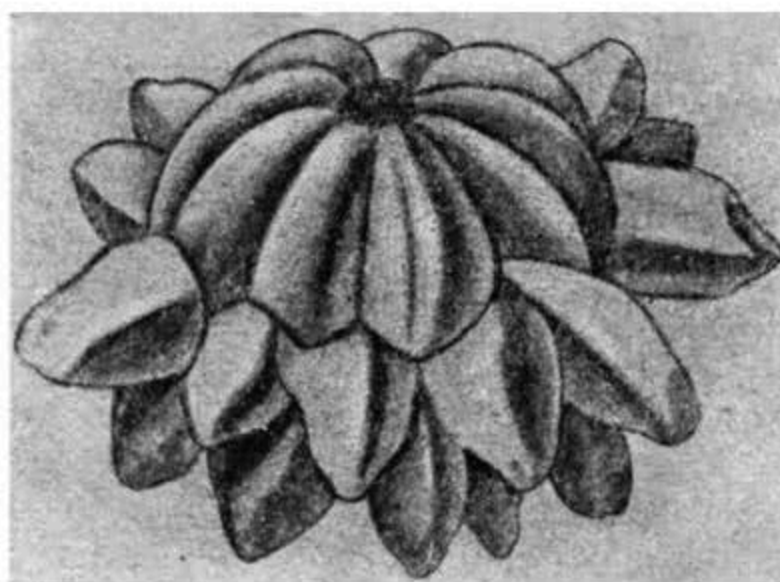
Рис. 129—131. Различные формы градин.
