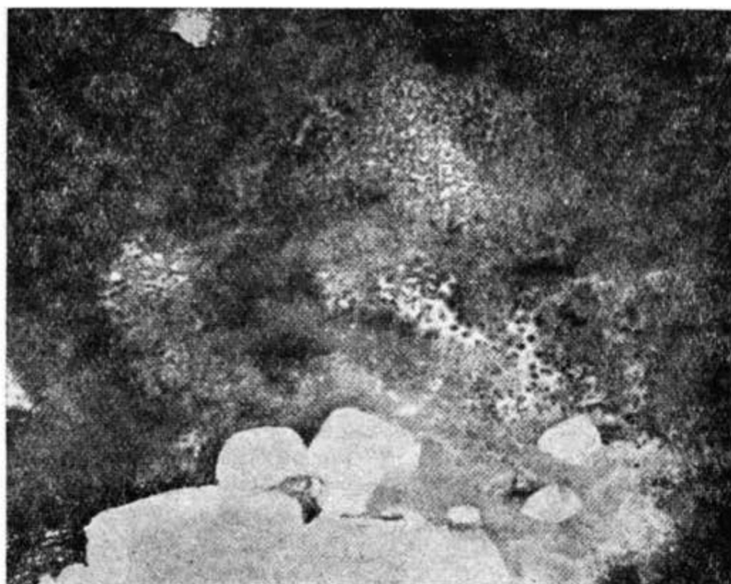
Рис. 152. Тающая льдина ноздреватого вида (сверху), сама льдина находится в воде, над водой видны лишь белые куски. Апрель 1923 (снимок В. А. Воротилова).
