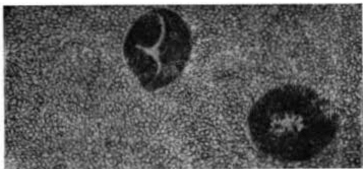
Рис. 4. «Дворик» вокруг более крупного кристалла инея на оконном стекле.
