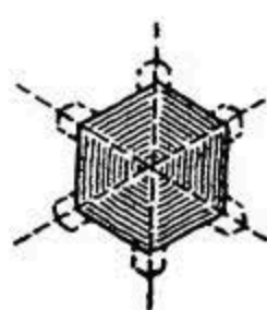
Рис. 14. Четырехгранные лопасти, образующиеся на ребрах шестигранного кристалла в переохлажденной жидкости.
