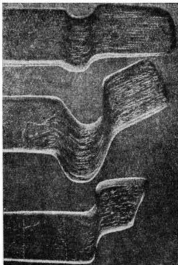
Рис. 54. Скольжения при изгибе пластинки льда (по Мюгге).
