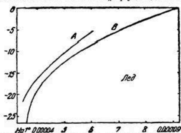
Рис. 38. Изменяемость коэффициента кубического расширения льда с температурой по Эндрюсу и Сойеру.
