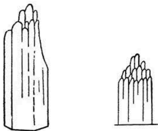
Рис. 91. Стерженьки с заостренным концом, растрепанным в виде пучка иголок (снимок Добровольского).
