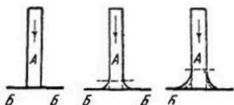
Рис. 28. Схема примерзания ледяной призмы к горизонтальной подставке.
