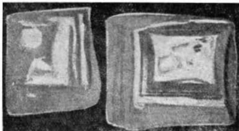
Рис. 98. Кристаллы инея формы прямоугольных параллелепипедов (снимок Бентлея).
