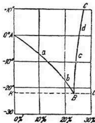
Рис. 7. Кривые затвердевания водного раствора хлористого натрия.
