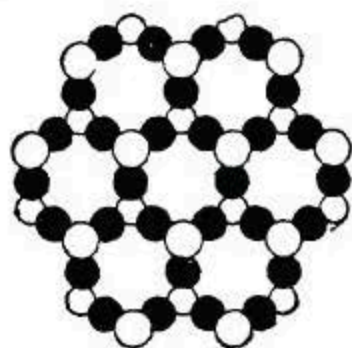
Рис. 63. Расположение кислородных (белые шары) и водородных (черные шары) атомов в зоне, вырезанной параллельно основанию кристалла льда.
