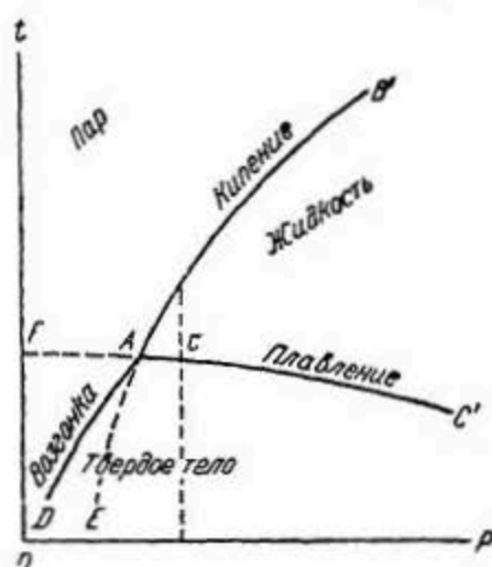
Рис. 1 и 2. Схематическая диаграмма фаз: 1) тело, которое при плавлении расширяется и температура плавления которого повышается при увеличении давления (обыкновенный случай — левая диаграмма); 2) тело, которое при плавлении уменьшается в объеме и температура плавления которого понижается при увеличении давления (случай, встречающийся значительно реже — правая диаграмма).
