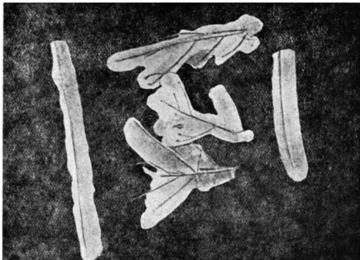
Рис. 132. Гололед на ветках.
