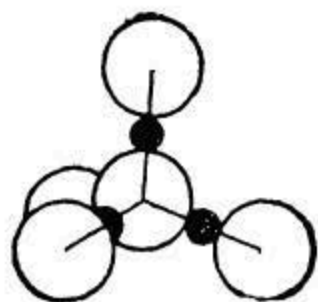
Рис. 69. Тетраэдрическое строение воды.
