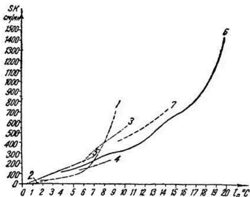
Рис. 51. Сводка определений линейной скорости кристаллизации. 1 — Тумлирц, 2, 3, 4 — Уолтон и Джедд, 5 — Хартман, 6, 7 — Лилиенталь.
