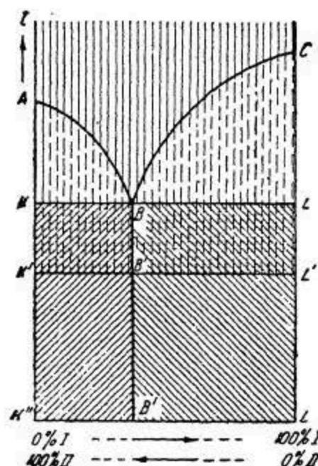
Рис. 10. Схема неустойчивых состояний растворов двух тел друг в друге.
