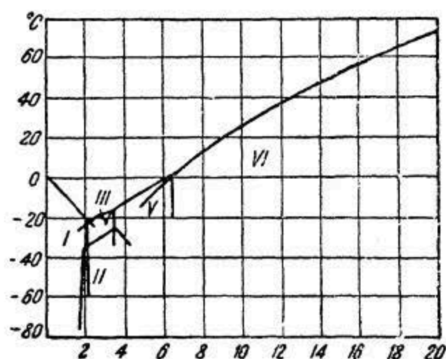
Рис. 30. Диаграмма состояний воды — жидкая вода и льды I, II, III, IV, V и VI — по Бриджмену.
