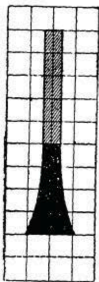
Рис. 33. Вероятная толщина соляных прослоек в слое льда, образовавшегося при -40^{\circ} .
