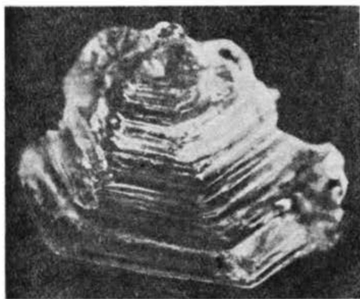
Рис. 112. Кристаллы инея: (a) — снимок Бентлена; \times 20 , (b) — снимок Зелигмана; (c) — схема различных кристаллов инея.
