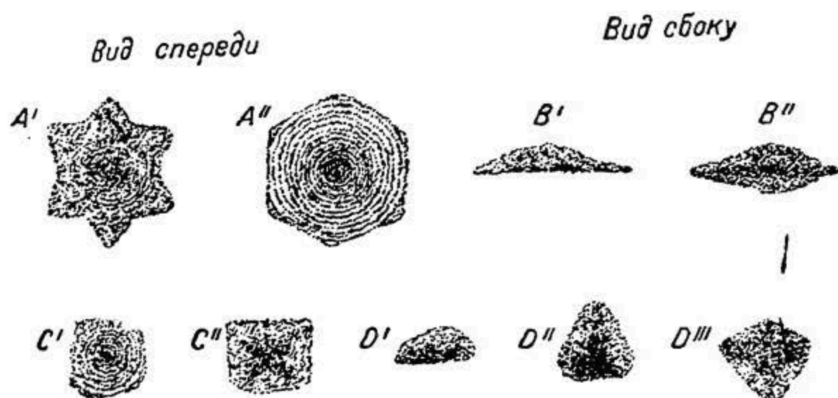
Рис. 107. Снежинки, покрытые инеем (снимки Бентлея).
