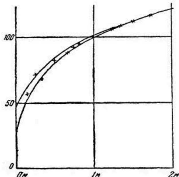
Рис. 56. Зависимость модуля сдвига льда от времени по Вейнбергу.
