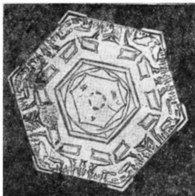
Рис. 75 и 76. След якобы гексагонального стержня ( 1\bar{1}20 ), обнаруженного во внутренних фигурах пластинки снега (снимки Бентлея).
