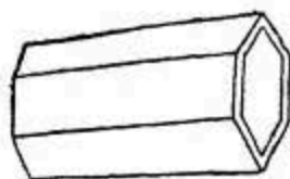
Рис. 112. Кристаллы инея: (a) — снимок Бентлена; \times 20 , (b) — снимок Зелигмана; (c) — схема различных кристаллов инея.
