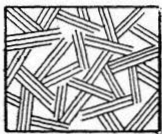
Рис. 150. Схема строения природного льда (в плане), образующегося в морской воде океанской солености (по В. И. Арнольду-Алябьеву).
