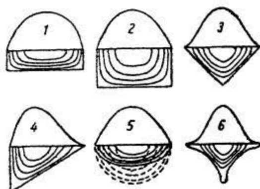
Рис. 196. Распределение скоростей при ламинарном течении жидкости по различным каналам.
