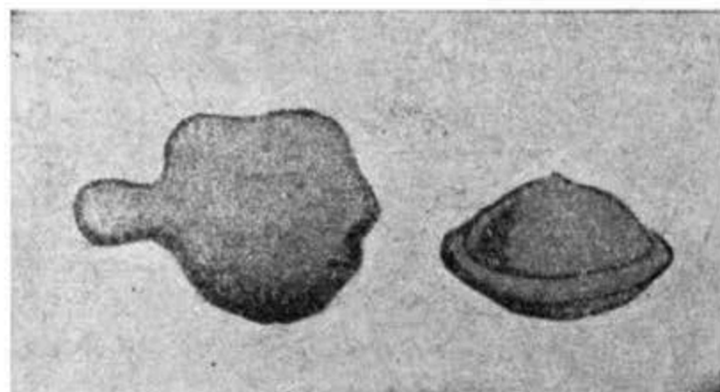
Рис. 125. Градины с наростами.
