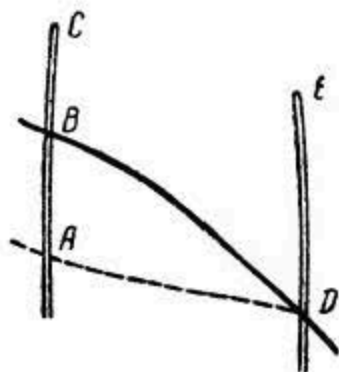
Рис. 189. Путь частицы ледника и вставленной в лед палки.
