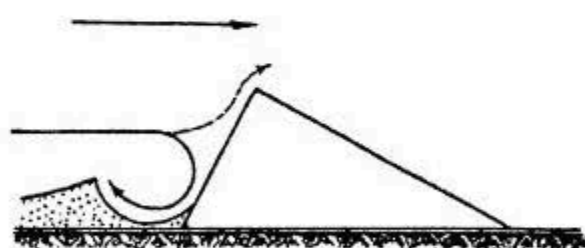
Рис. 166. То же — при обращении к ветру круто поднимающимся склоном препятствия.
