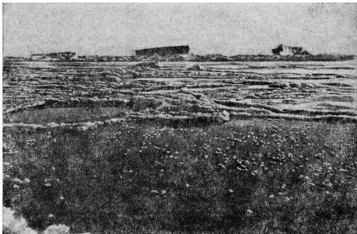
Рис. 138. Молодик в Антарктических водах. На переднем плане на гладкой поверхности прозрачного льда видны пучки инея. На фоне — ледяные горы (айсберги) (снимок Пристлея, 1912).
