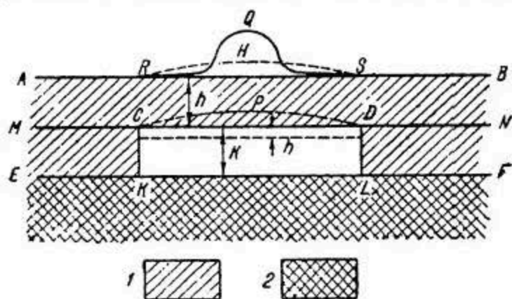
Рис. 204. Схема образования наледного бугра.
