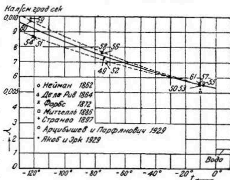
Рис. 52. Зависимость коэффициента теплопроводности льда от температуры по опытам Якоба и Эрка и других исследователей.
