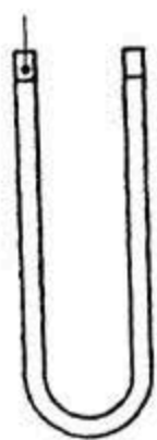
Рис. 50. Схема опытов по определению линейной скорости кристаллизации.
