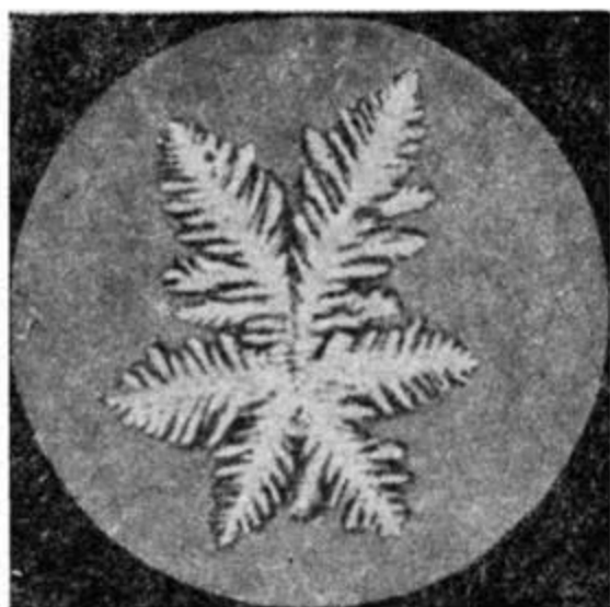
Рис. 40. Получение одиночной звездчатой пластинки льда из переохлажденной воды.
