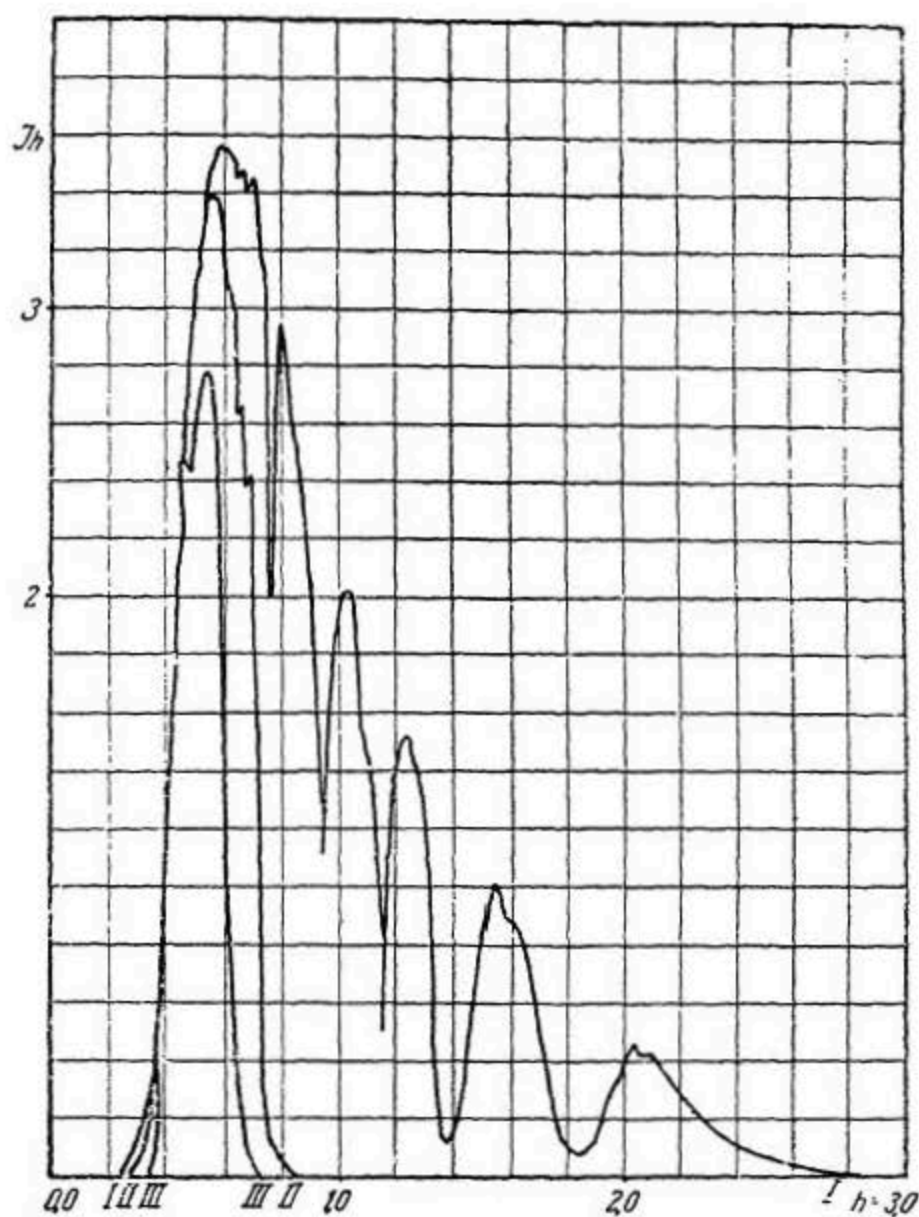
Рис. 61. Распределения энергии в спектре солнечного излучения, падающего на воду (кривая I) и прошедшего через слой воды толщиной в 1 и 10 м (кривые II и III).
