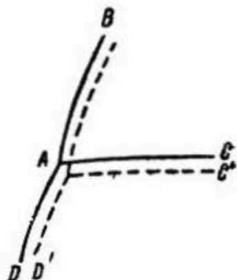
Рис. 5. Влияние нормального давления на тройную точку.
