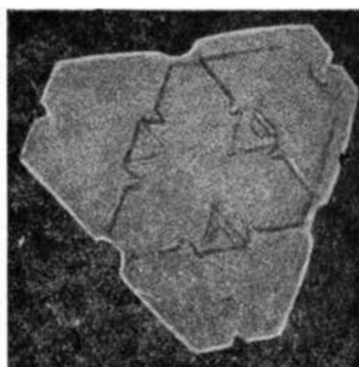
Рис. 78. Пластинчатый кристалл снега: поворот относительного развития двух тригональных стержней на некоторой стадии роста кристалла (снимок Бентлея).
