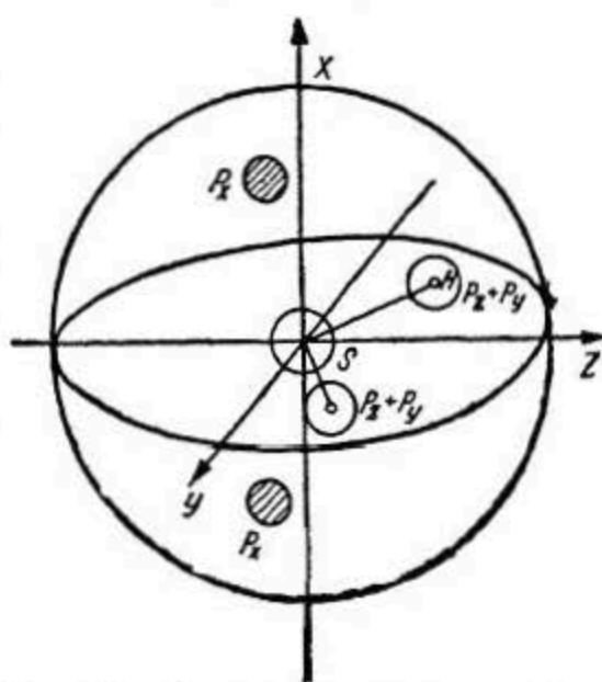
Рис. 68. Модель электронного облака молекулы воды по Милликэну.
