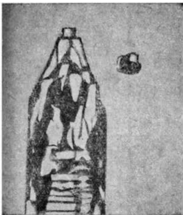
Рис. 88. Заостренный стержневидный кристалл льда (снимок Вестмана).
