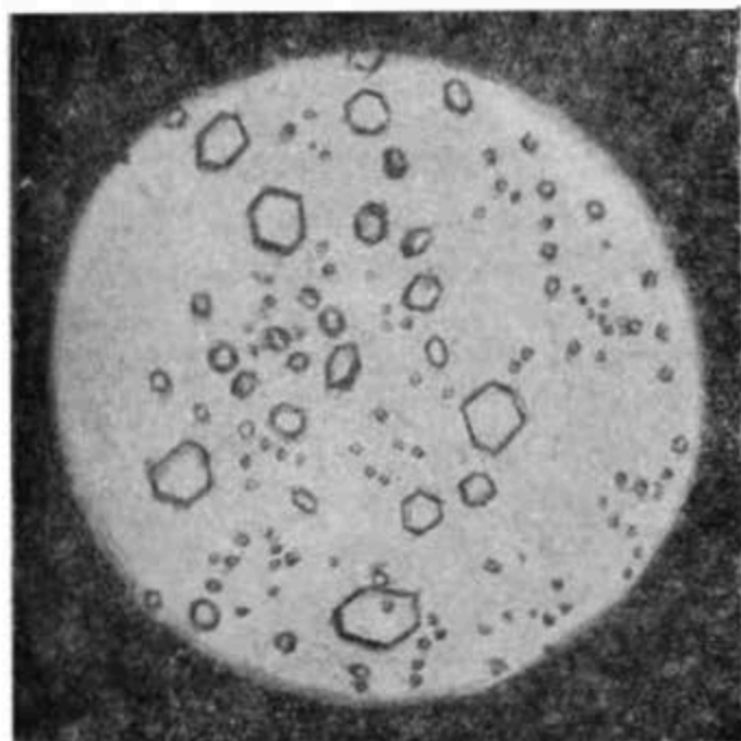
Рис. 47. «Отрицательные кристаллы», полученные вторичным замораживанием «ледяного цветка», подобного рис. 46 (увеличение в 8 раз). Адамс и Дэвис обращают внимание на точный параллелизм соответствующих границ.
