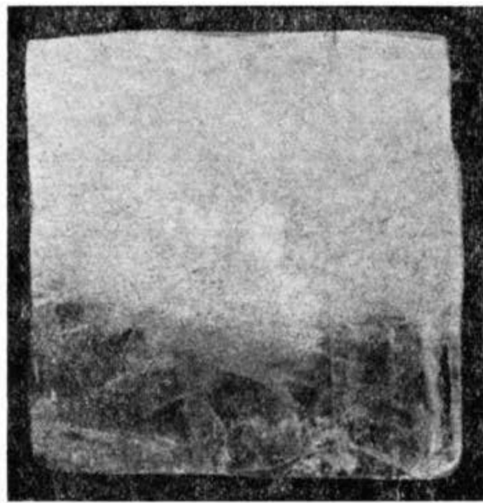
Рис. 149. Образец, вятый из верхней части ледяного покрова Невы: вверху мутный лед с обильными полостями, внизу — прозрачный чистый со следами деформаций и неправильностей в процессе намерзания (снимок С. А. Кадлеца).
