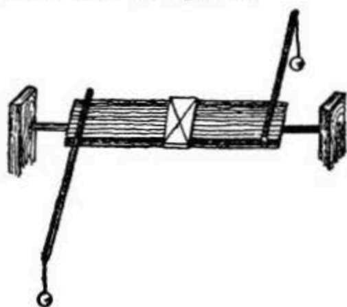
Рис. 57. Прибор Бианкони для кручения пластинки льда и результаты воздействия закручивающей пары.
