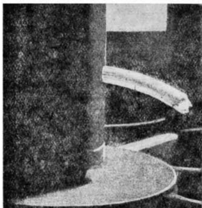
Рис. 58. Опыты Энгельна по выдавливанию льда через боковое отверстие.
