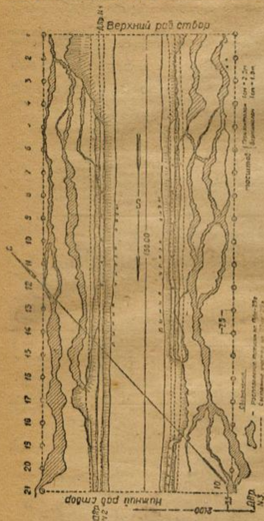
Рис. 19. План участка Старого Дзуга с показанием размывов на 12/VI 1926 г.
