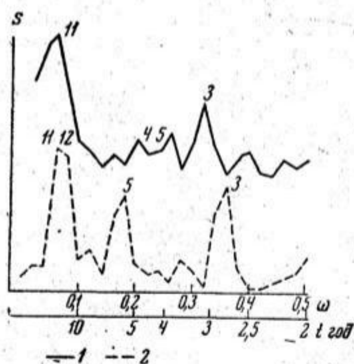
Рис. 4. Спектральная функция суммарного стока: 1 — первая группа рек; 2 — вторая группа рек
