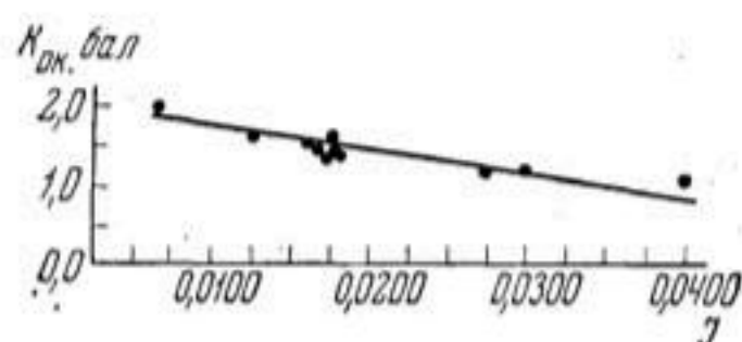
Рис. 2. Связь уклонов рек с окатанностью галечников
