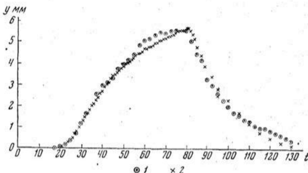
Рис. 2. Сопоставление наблюдаемого и вычисленного гидрографов: 1 — наблюдаемый; 2 — вычисленный гидрограф
